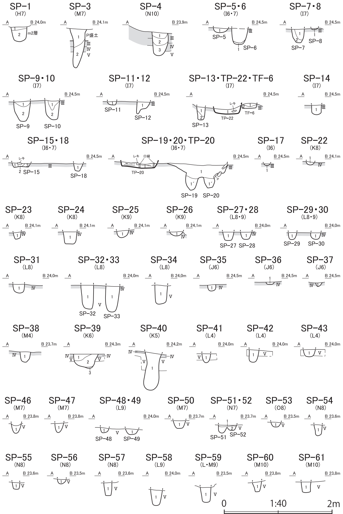
図IV-323 小ピット断面図 (1)
