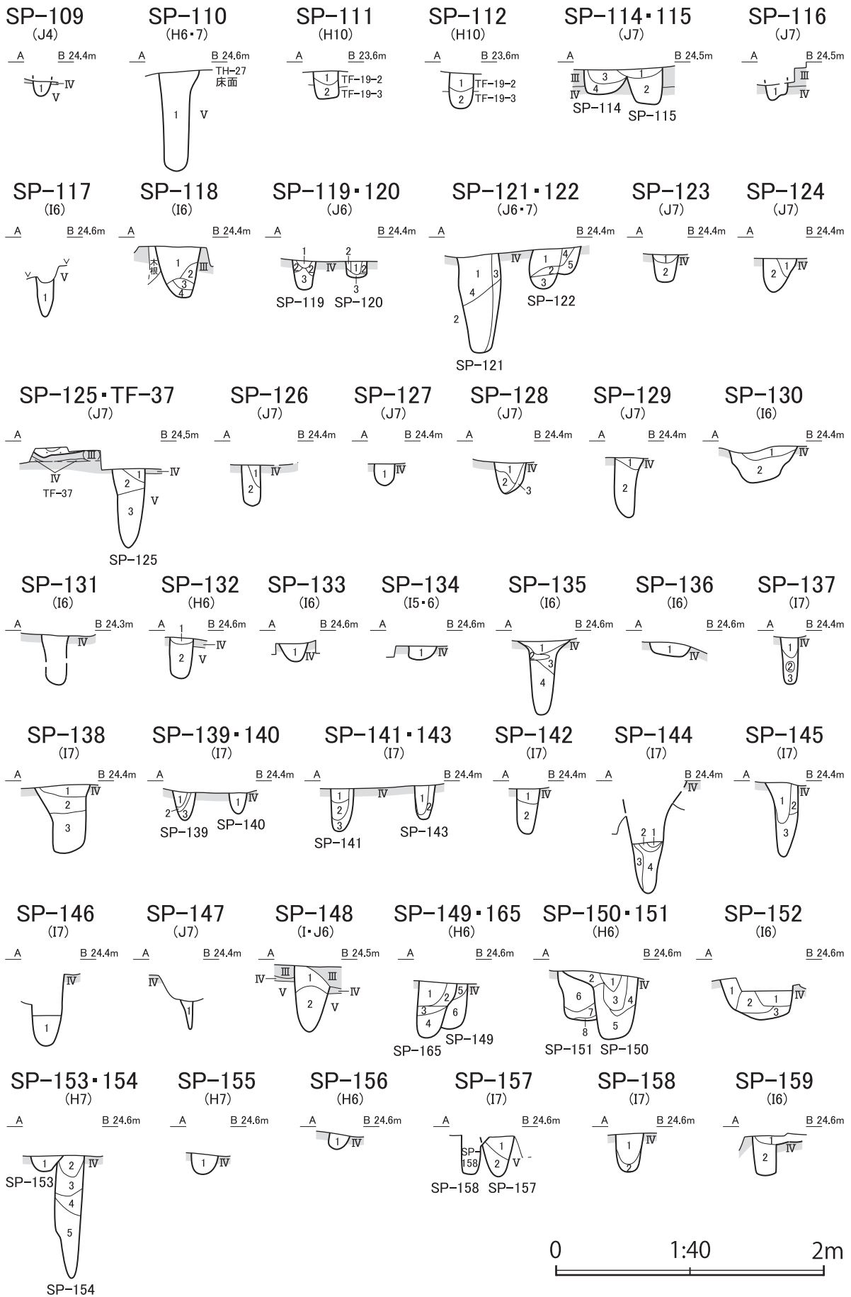
図IV-325 小ピット断面図 (3)
