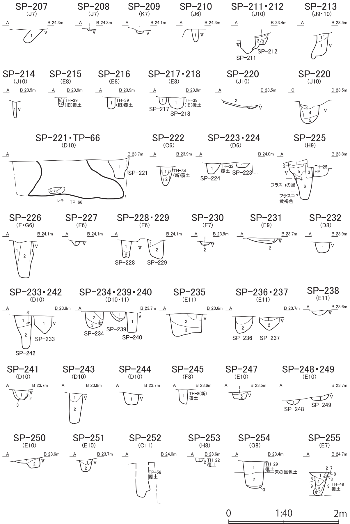
図IV-327 小ピット断面図 (5)
