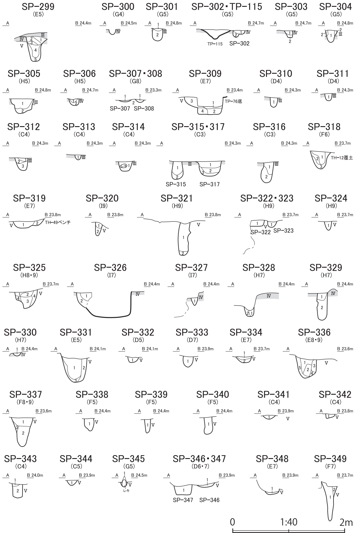
図IV-329 小ピット断面図 (7)
