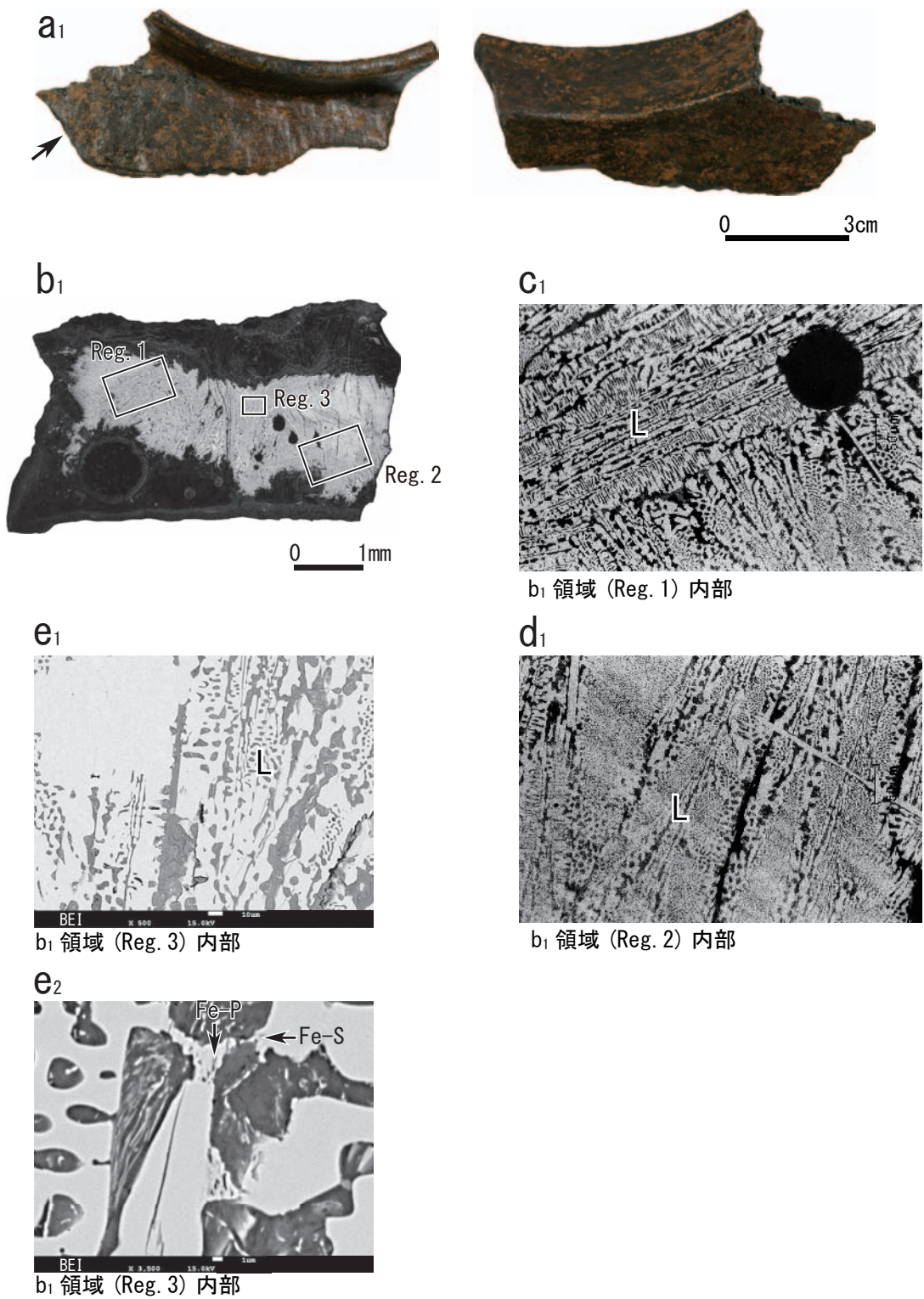
図5 No. 8の組織観察結果
