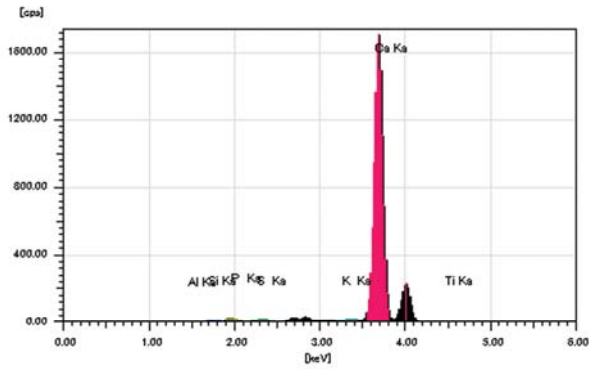
図1 蛍光 X 線分析結果
