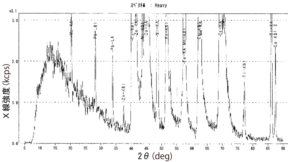
図 26(2) No. 72 および No. 113 の蛍光 X 線定性チャート
