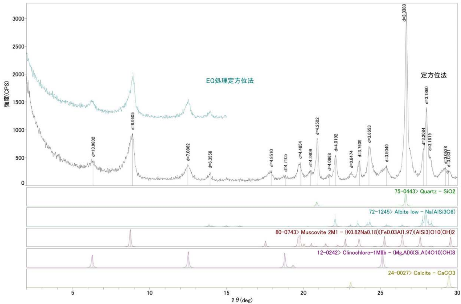
図16. 試料64(笏谷石)の定方位法・EG処理定方位法X線回折図
