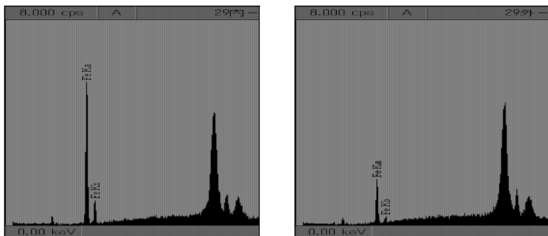
図 145. 漆塗椀 No.29 の XRF 測定結果（左図：29-内赤、右図：29-外黒）
