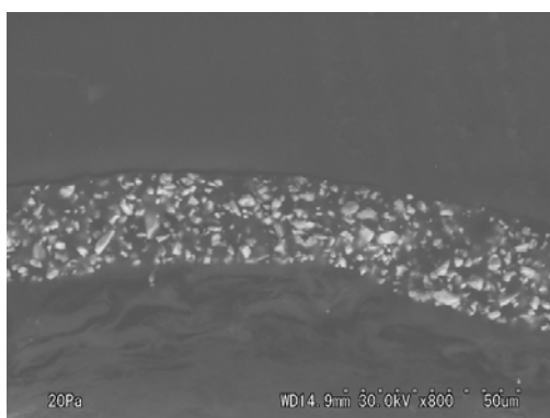
図 204. 漆塗串 No.11 の塗膜断面 SEM 画像 漆塗串 No.11 における朱の粒径は 2.6\sim 8.2\mu\text{m} で、大きさは比較的均質であった（図 204）。
