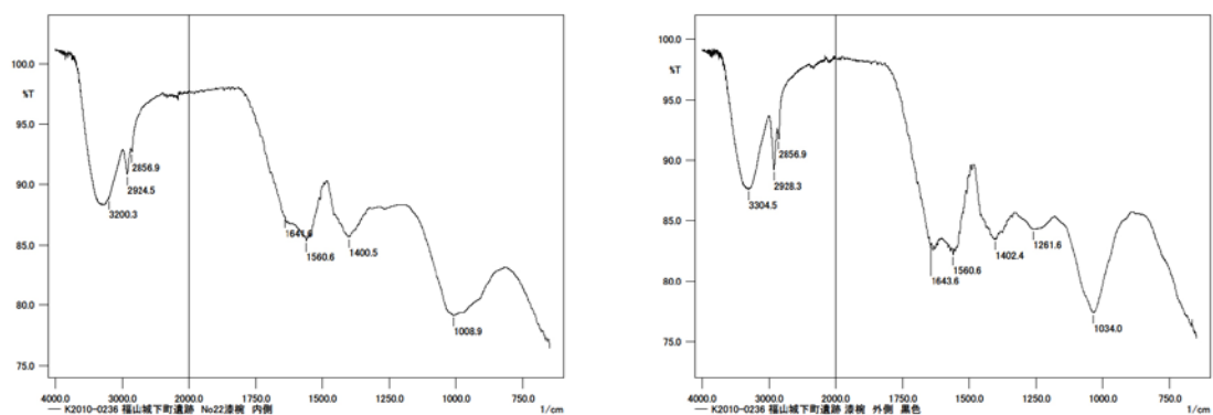
図 109. 漆塗椀 No.22 の ATR-FTIR 測定結果（左図：22-内赤、右図：22-外黒）
