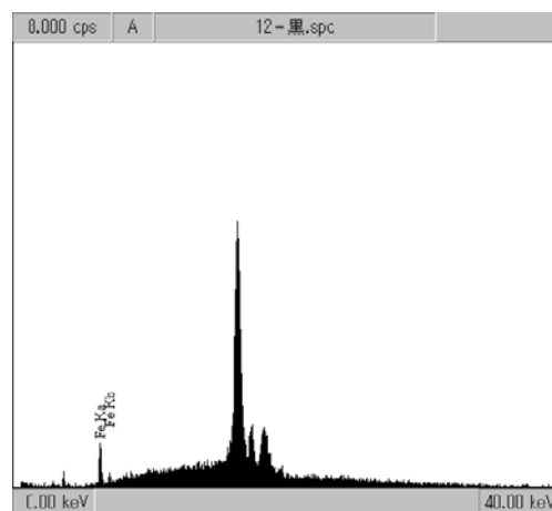
図 60. 漆塗部材 No.12 の XRF 測定結果
