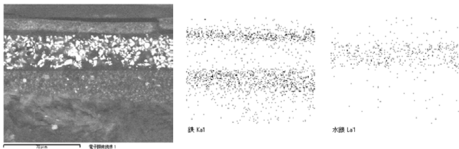
図 37. 漆塗椀 No.7 塗膜断面の SEM-EDX マッピング結果 (07-内赤) (左図：SEM 画像、中図：EDX 鉄のマッピング、右図；EDX 水銀のマッピング)
