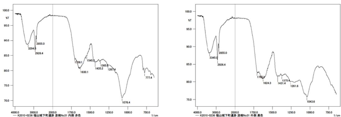
図 154. 漆塗椀 No.31 の ATR-FTIR 測定結果（左図：31-内赤、右図：31-外黒）
