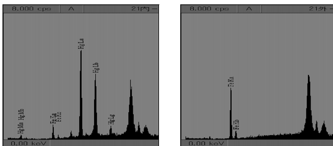
図 105. 漆塗椀 No.21 の XRF 測定結果（左図：21-内赤、右図：21-外黒）
