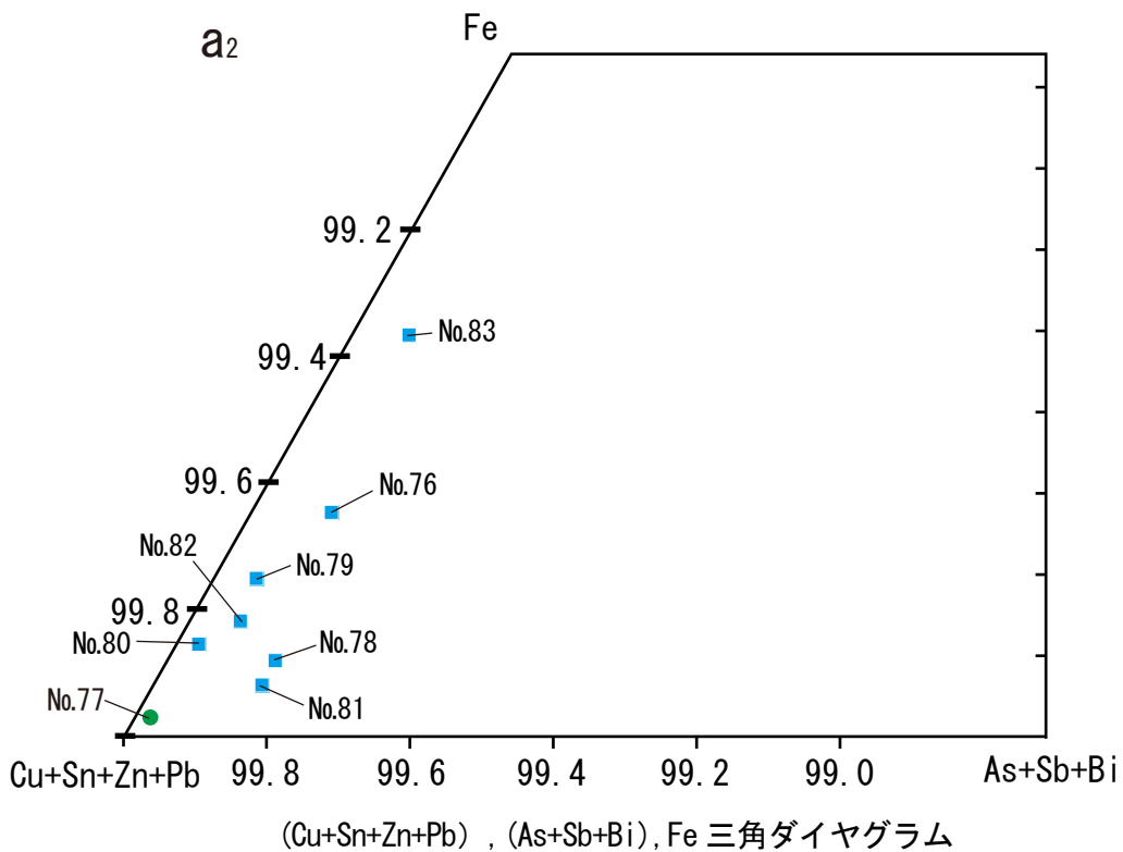
図 34 キセル関係資料 (No. 76 ~ 83) に含有される主成分および微量成分の三角ダイヤグラム No. は表 9 に対応。■ = 真鍮を素材とする試料、● = 銅を素材とする試料。
