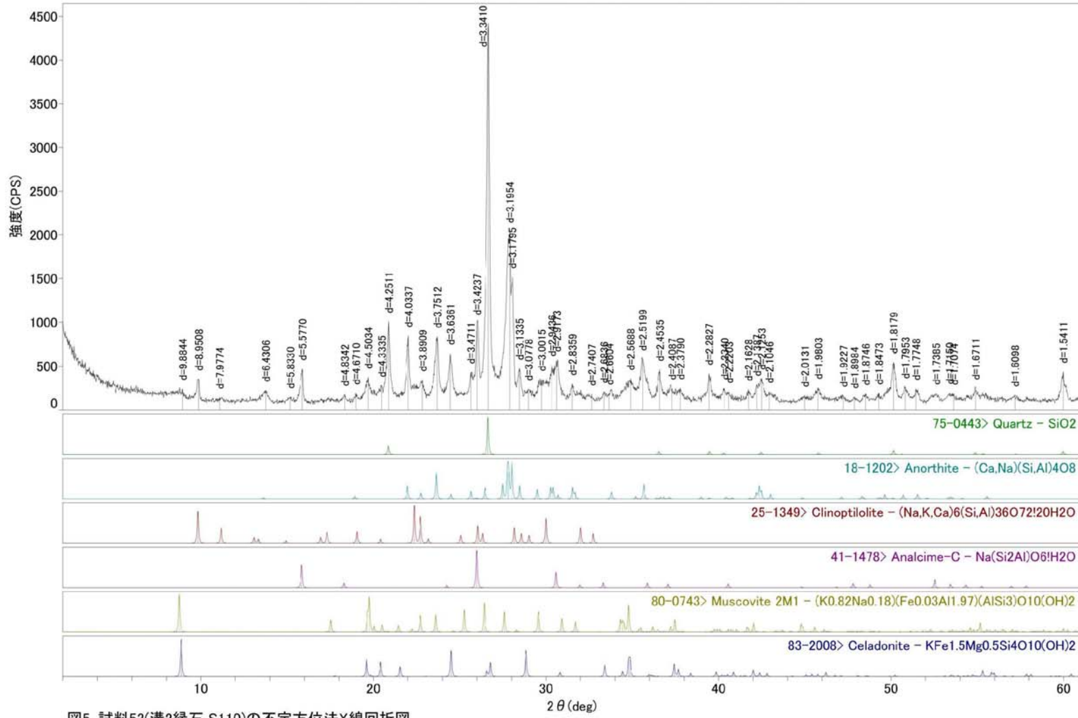
図5. 試料53(溝2緑石 S110)の不定方位法X線回折図
