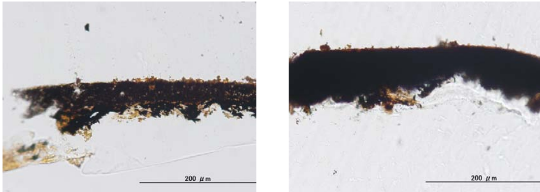
図 91. 漆塗腕 No.18 の塗膜断面透過観察画像 (左図 : 18-内赤、右図 : 18-外赤)
