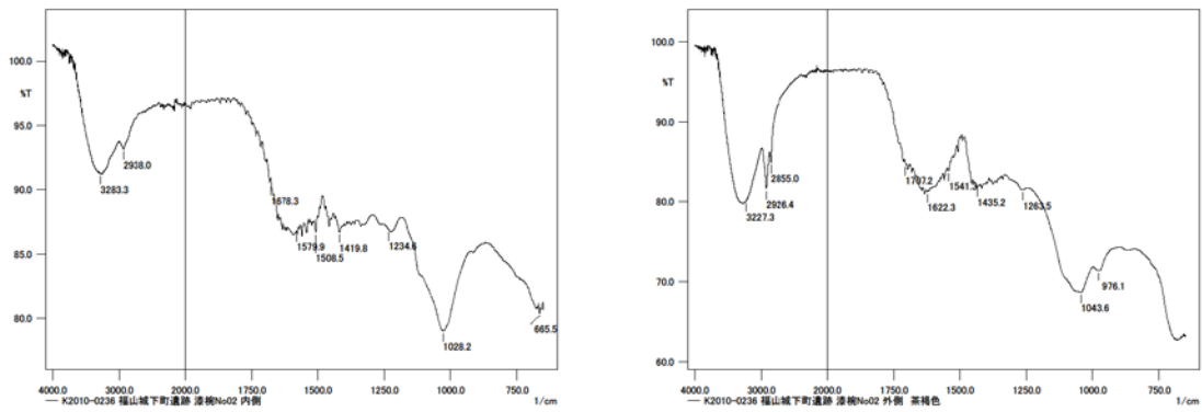
図 7. 漆塗椀 No.2 の ATR-FTIR 測定結果（左図：02-内赤、右図：02-外赤）
