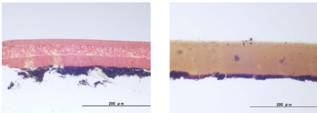
図 36. 漆塗椀 No.7 の塗膜断面落射観察画像 (左図：07-内赤、右図：07-外黒)
