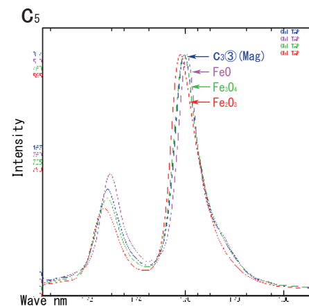
c 3 ③ (Mag) の Fe-L \alpha および Fe-L \beta スペクトル
