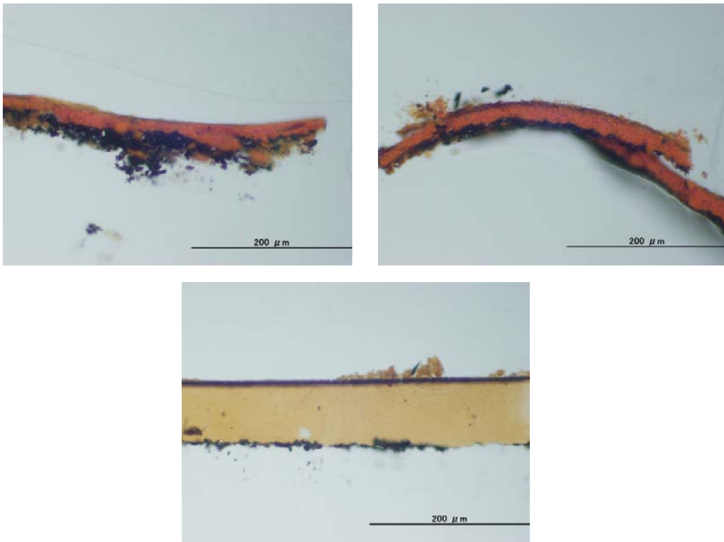
図 177. 漆塗梔 No.35 の塗膜断面落射観察画像 (左図 : 35-内赤、右図 : 35-外赤、下図 : 35-底黒)
