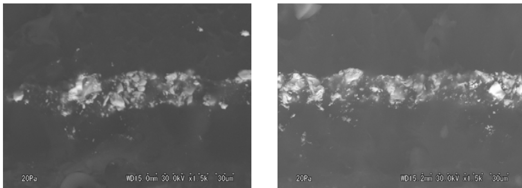
図 202. 漆塗椀 No.4 の塗膜断面 SEM 画像（左図：04-内赤、右図：04-外赤） 漆塗椀 No.4 における朱の粒径は 1.6\sim 7.1\mu\text{m} で、大きさは不揃いであった（図 202）。
