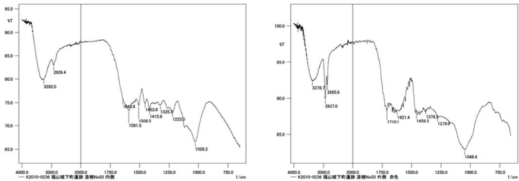
図 12. 漆塗椀 No.3 の ATR-FTIR 測定結果（左図：03-内赤、右図：03-外赤）
