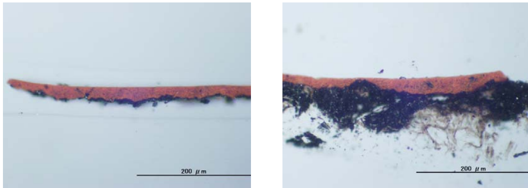
図 15. 漆塗椀 No.3 の塗膜断面落射観察画像 (左図：03-内赤、右図：03-外赤)
