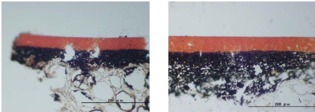
図 172. 漆塗腕 No.34 の塗膜断面落射観察画像 (左図：34-内赤、右図：34-外赤)
