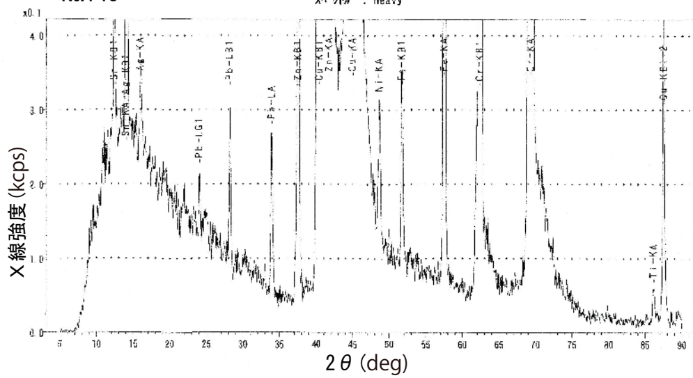
図 26(9) No. 142 および No. 143 の蛍光 X 線定性チャート
