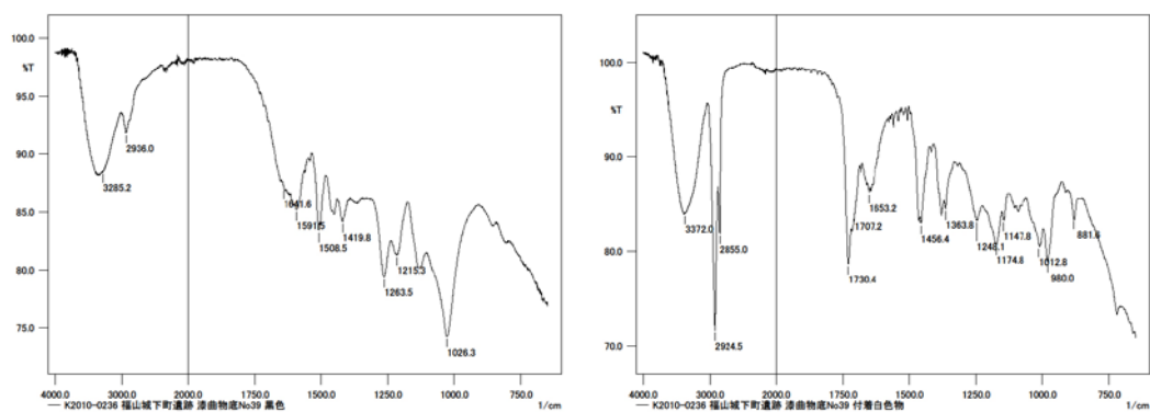
図 195. 漆塗底板 No.39 の ATR-FTIR 測定結果（左：39-黒、右：39-白色付着物）
