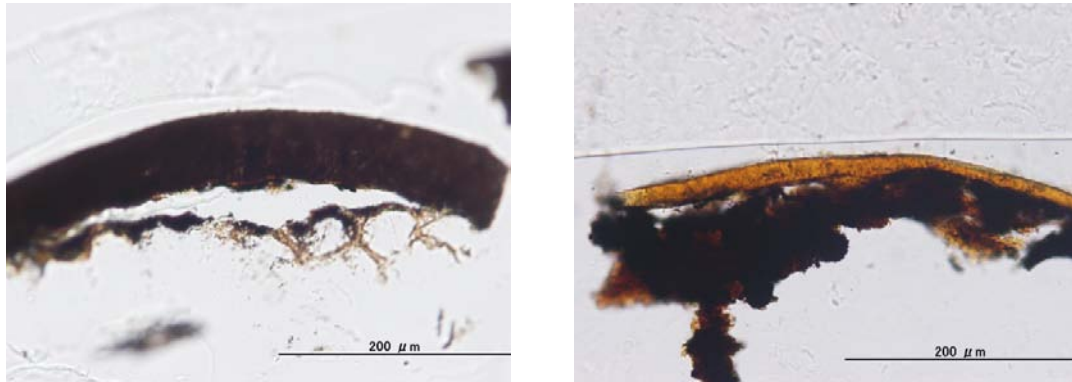
図 86. 漆塗箸 No.17 の塗膜断面透過観察画像（左図：17-赤、右図：17-黒）
