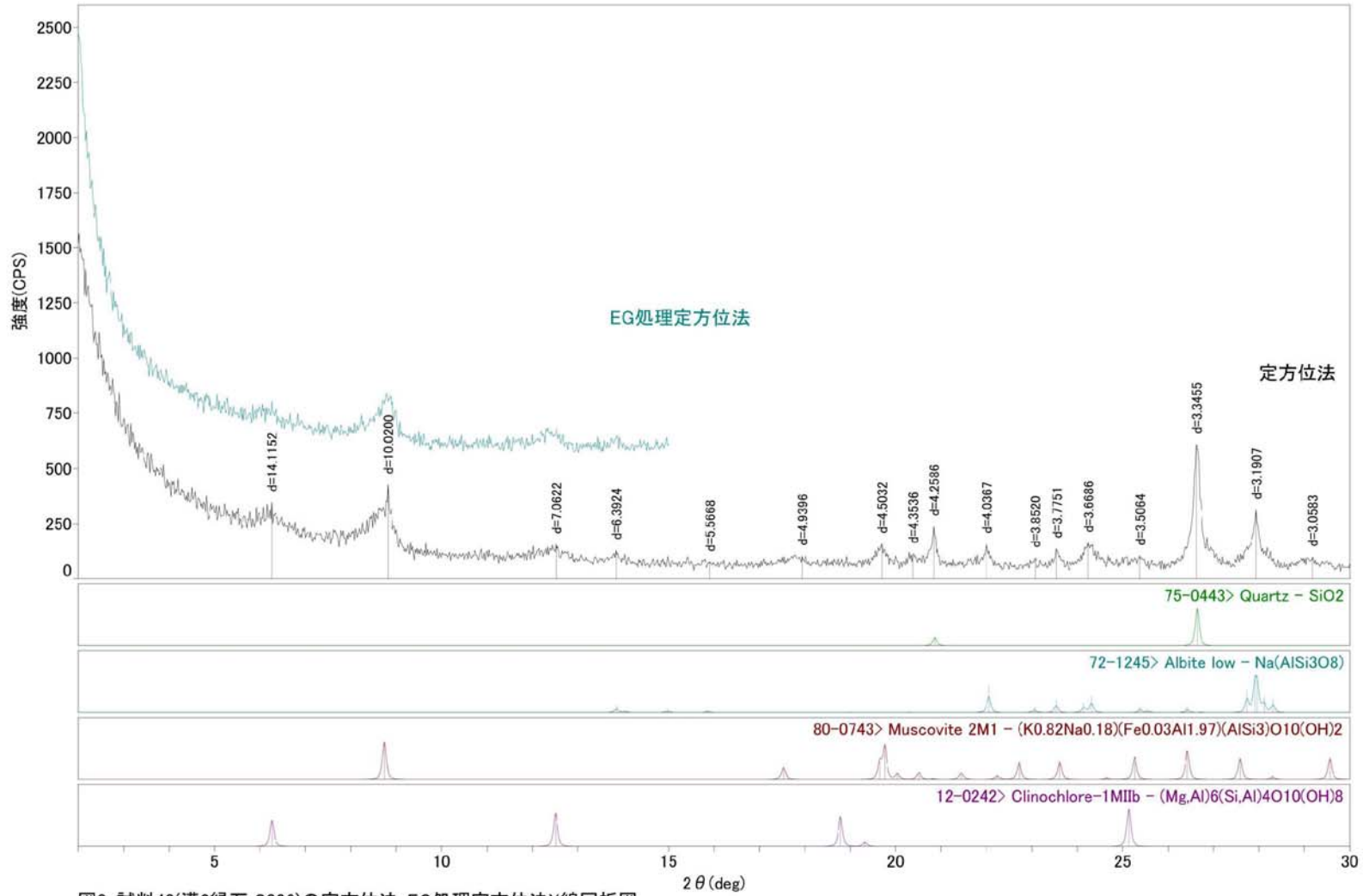
図8. 試料48(溝2緑石 S026)の定方位法・EG処理定方位法X線回折図
