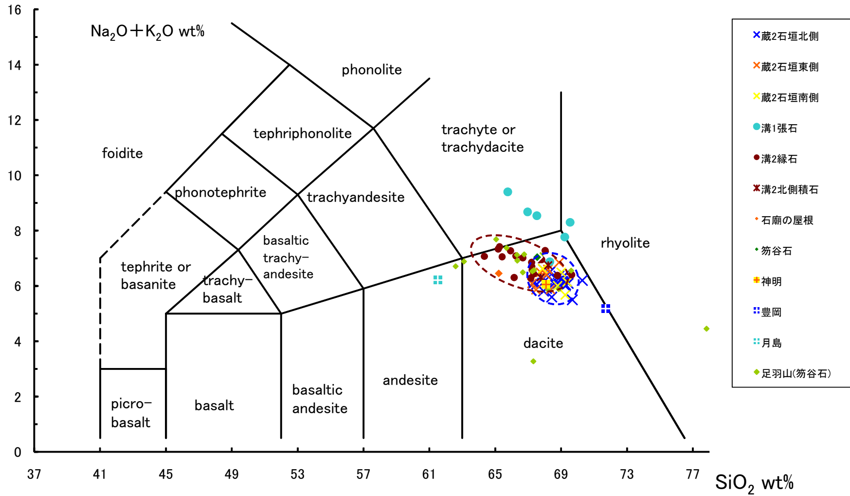
図23 TAS(total alkali-silica)図(Le Maitre, 2002) 青破線は蔵2石垣石材の分布範囲を、茶破線は溝2縁石の主な分布範囲を示す。
