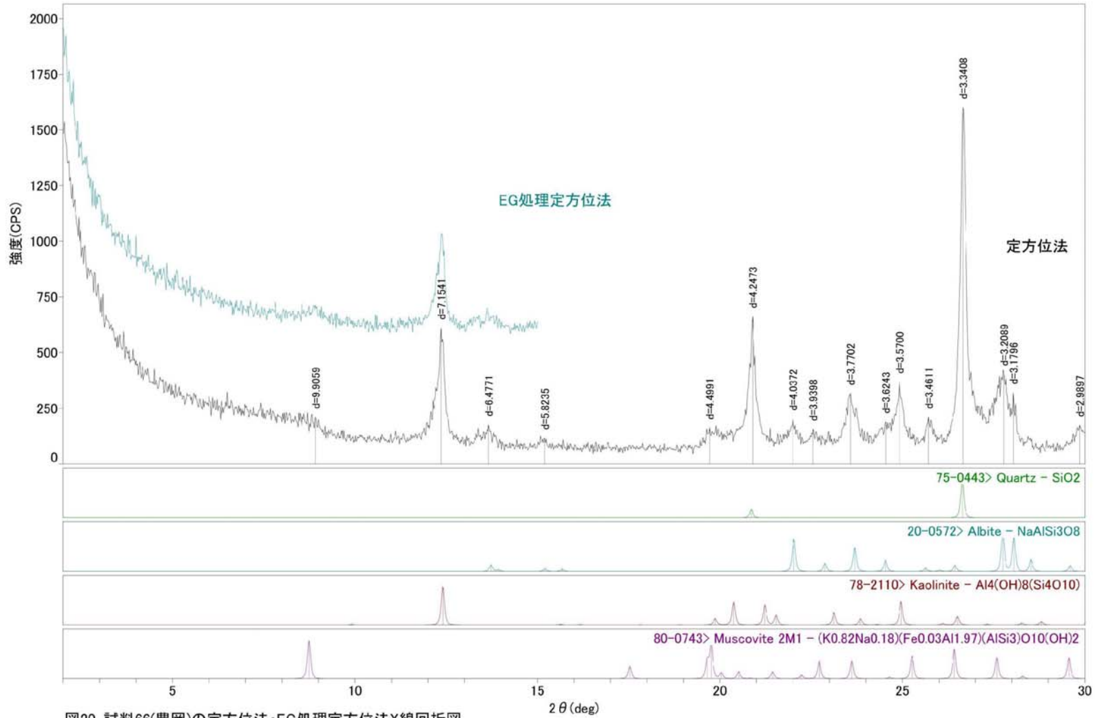
図20. 試料66(豊岡)の定方位法・EG処理定方位法X線回折図
