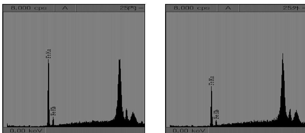
図 125. 漆塗椀 No.25 の XRF 測定結果（左図：25-内赤、右図：25-外黒）
