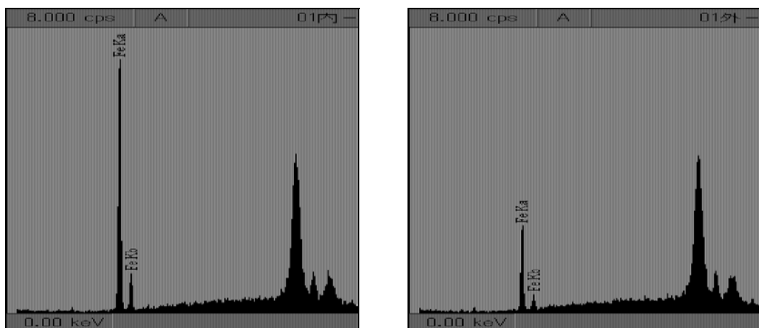
図 3. 漆塗椀 No.1 の XRF 測定結果（左図：01-内赤、右図：01-外黒）
