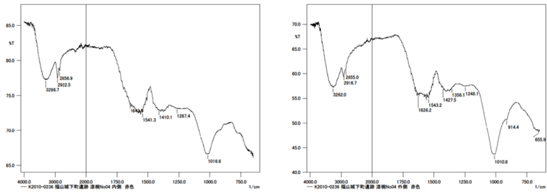
図 17. 漆塗椀 No.4 の ATR-FTIR 測定結果（左図：04-内赤、右図：04-外赤）
