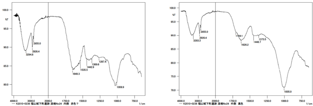
図 119. 漆塗椀 No.24 の ATR-FTIR 測定結果（左図：24-内赤、右図：24-外黒）
