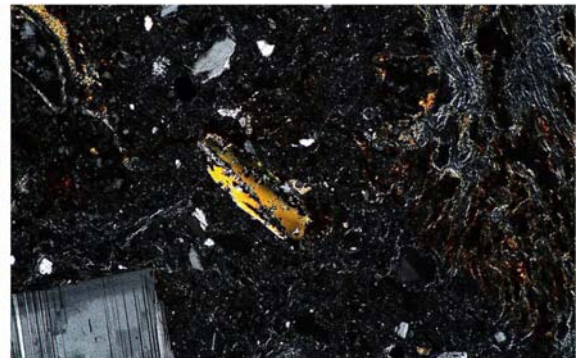
2. グループA 試料29 凝灰岩 蔵2石垣東側 S222 デイサイト質ガラス質凝灰岩
