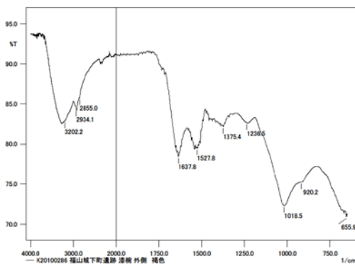
図 26. 漆塗椀 No.5 の ATR-FTIR 測定結果 2 (図 22 右図 : 05-外赤の裏面)
