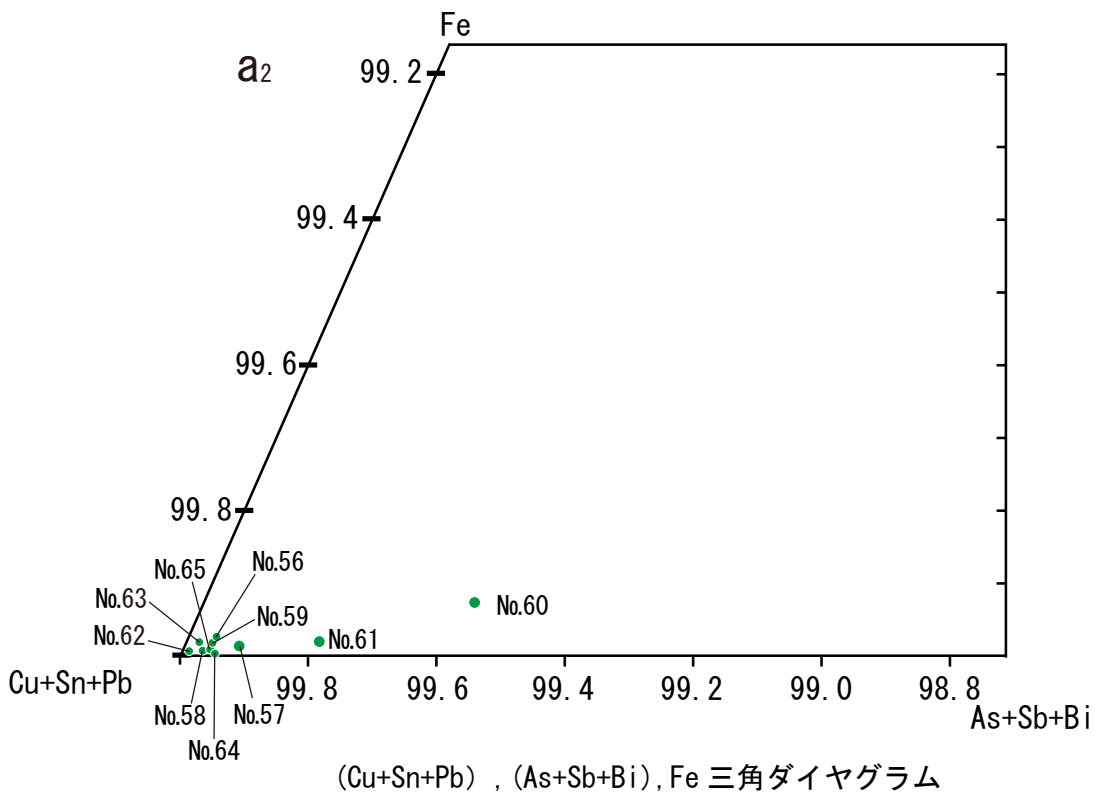
図 28 釘 (No. 56 ~ 65) に含有される主成分および微量成分の三角ダイヤグラム No. は表 9 に対応。
