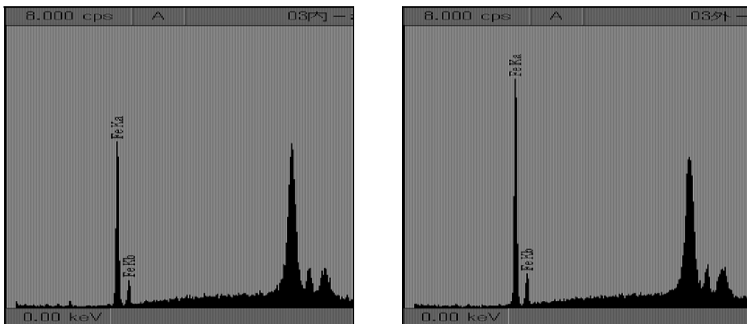
図 13. 漆塗椀 No.3 の XRF 測定結果（左図：03-内赤、右図：03-外赤）
