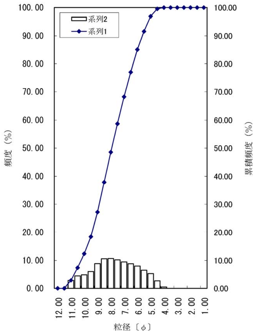
図3 蔵2石垣接合部灰白色粘土の粒度分布
