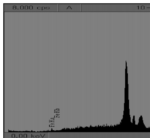
図 50. 漆塗箸 No.10 の XRF 測定結果
