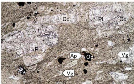
8. 原産地試料 笏谷石 試料64 デイサイト質ガラス質凝灰岩
