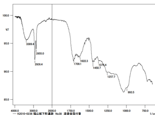
図 189. 漆塗箸 No.38 の ATR-FTIR 測定結果 (38-金黒)
