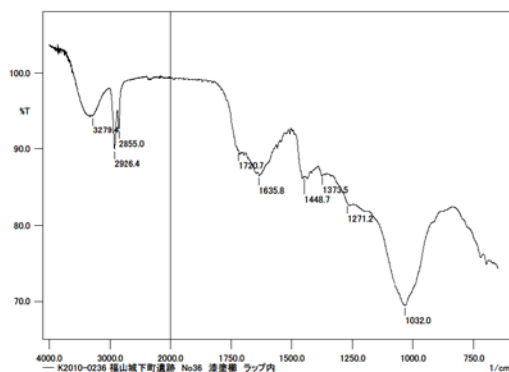
図 179. 漆塗櫛 No.36 の ATR-FTIR 測定結果 図 180. 漆塗櫛 No.36 の XRF 測定結果
