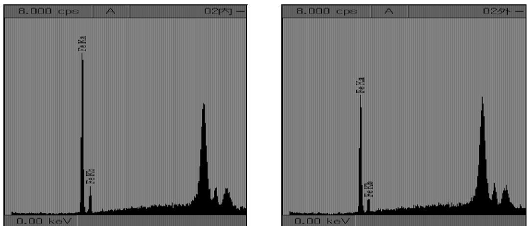
図 8. 漆塗椀 No.2 の XRF 測定結果（左図：02-内赤、右図：02-外赤）
