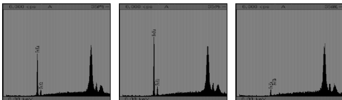
図 175. 漆塗椀 No.35 の XRF 測定結果（左図：35-内赤、中図：35-外赤、右図：35-底黒）
