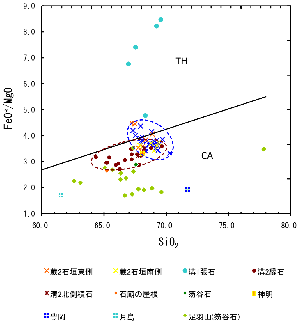
図26 FeO*/MgO-SiO 2 関係図
