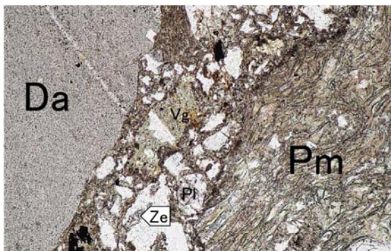
3. グループB 試料53 溝2縁石 S110 デイサイト質火山礫凝灰岩
