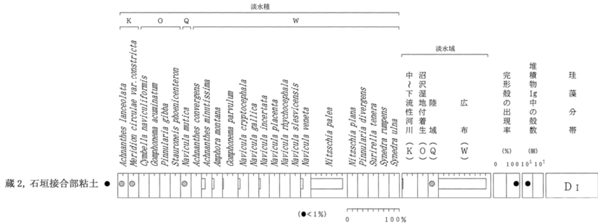
図 2 堆積物中の珪藻化石分布図 (1.0%以上の分類群を表示)
