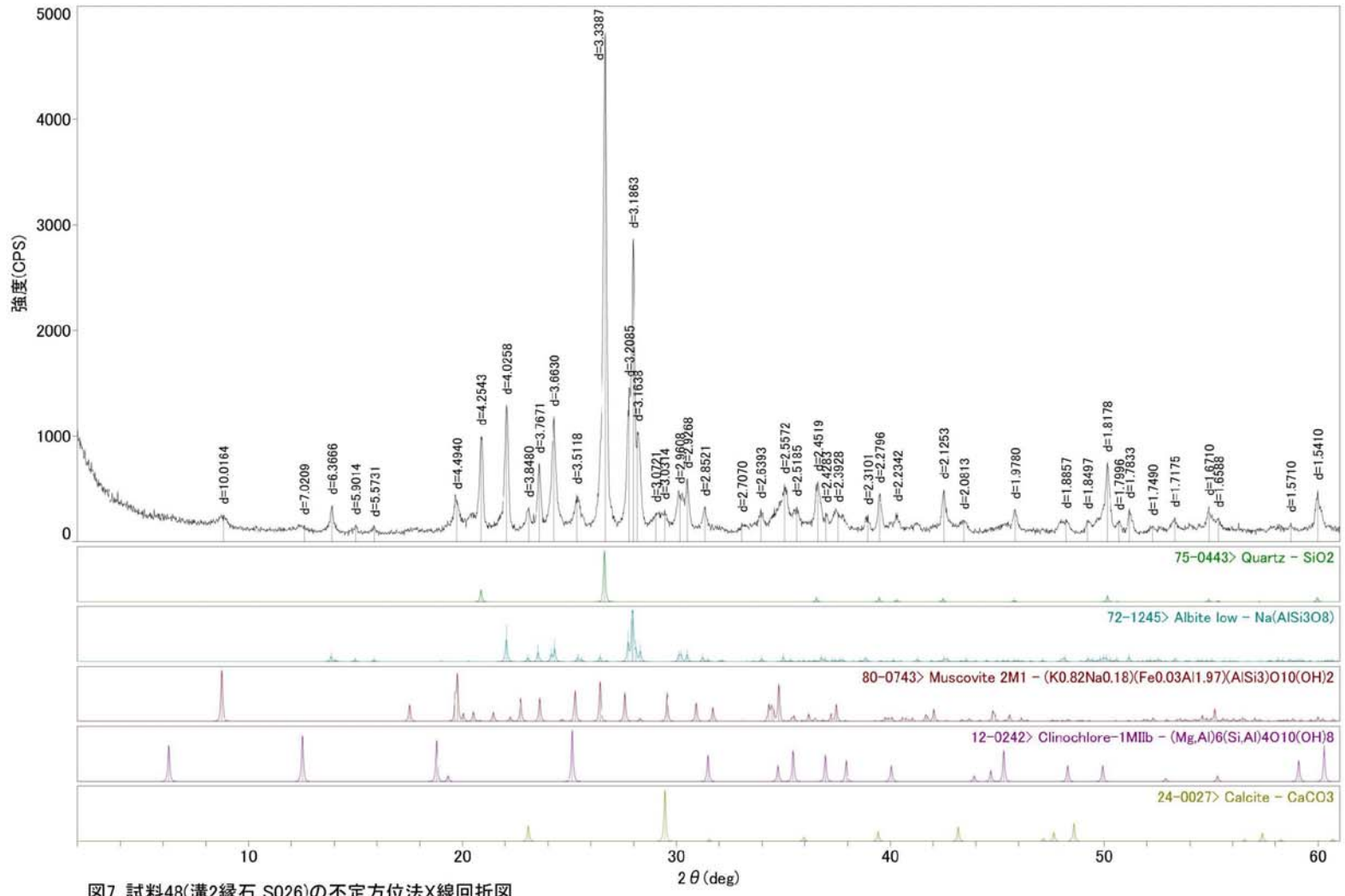
図7. 試料48(溝2緑石 S026)の不定方位法X線回折図
