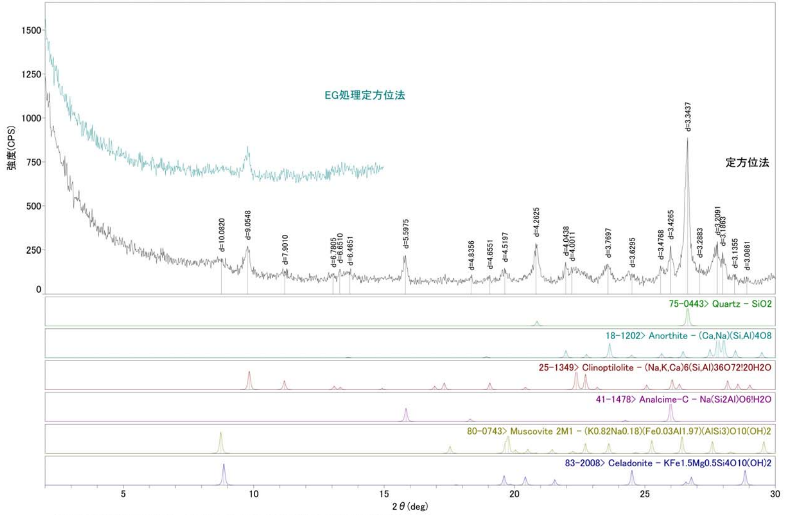
図2. 試料20(藏2石垣北側 S271)の定方位法・EG処理定方位法X線回折図
