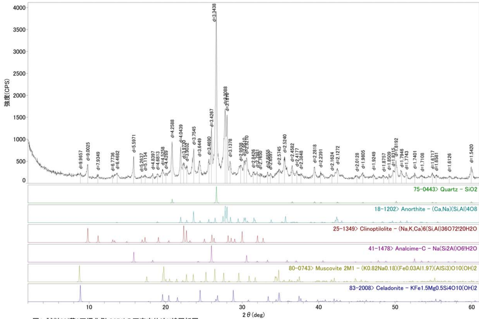
図1. 試料20(藏2石垣北側 S271)の不定方位法X線回折図
