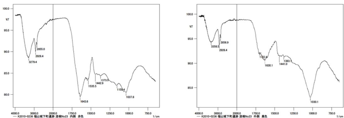
図 114. 漆塗椀 No.23 の ATR-FTIR 測定結果 (左図 : 23-内赤、右図 : 23-外黒)
