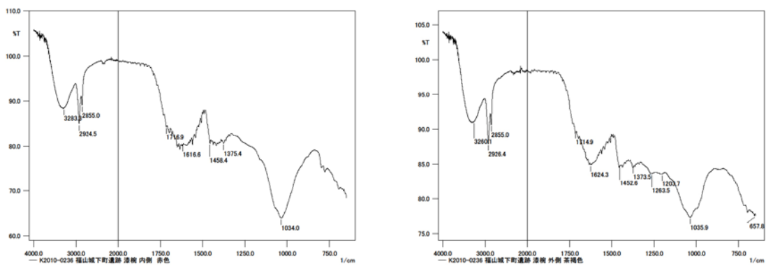
図 2. 漆塗椀 No.1 の ATR-FTIR 測定結果（左図：01-内赤、右図：01-外黒）
