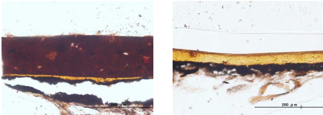
図 146. 漆塗椀 No.29 の塗膜断面透過観察画像 (左図：29-内赤、右図：29-外黒)
