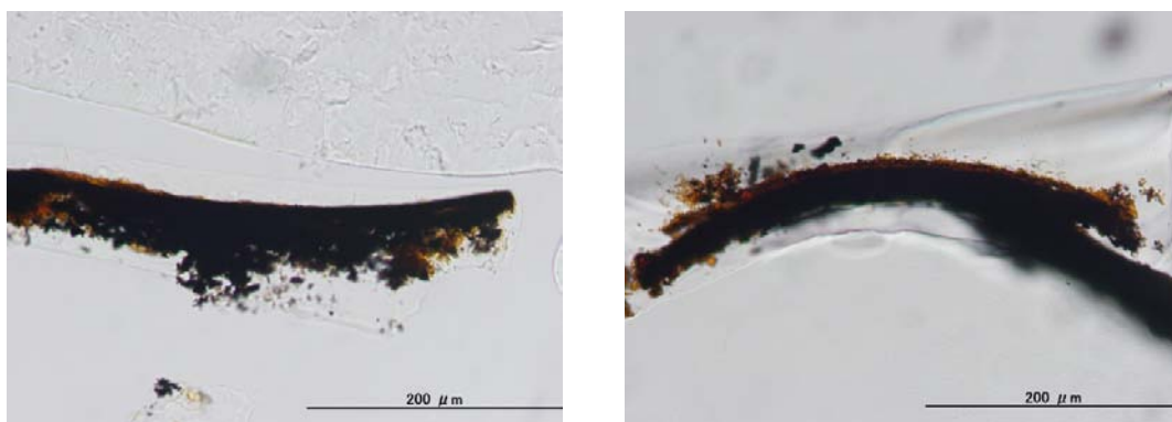
図 176-1. 漆塗椀 No.35 の塗膜断面透過観察画像（左図：35-内赤、右図：35-外赤）
