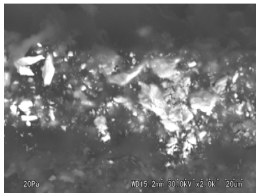
図 207. 漆塗椀 No.21 の塗膜断面 SEM 画像 漆塗椀 No.21 における朱の粒径は 1.2\sim 6.3\mu\text{m} で、大きさは不揃いであった (図 207)。
