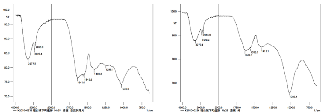
図 124. 漆塗椀 No.25 の ATR-FTIR 測定結果（左図：25-内赤、右図：25-外黒）
