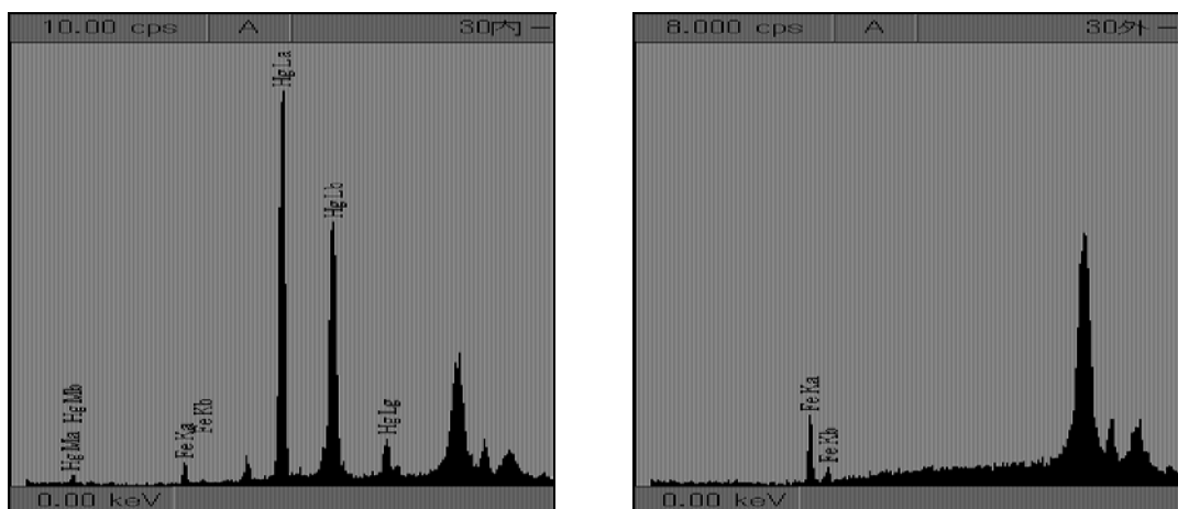
図 150. 漆塗椀 No.30 の XRF 測定結果（左図：30-内赤、右図：30-外黒）
