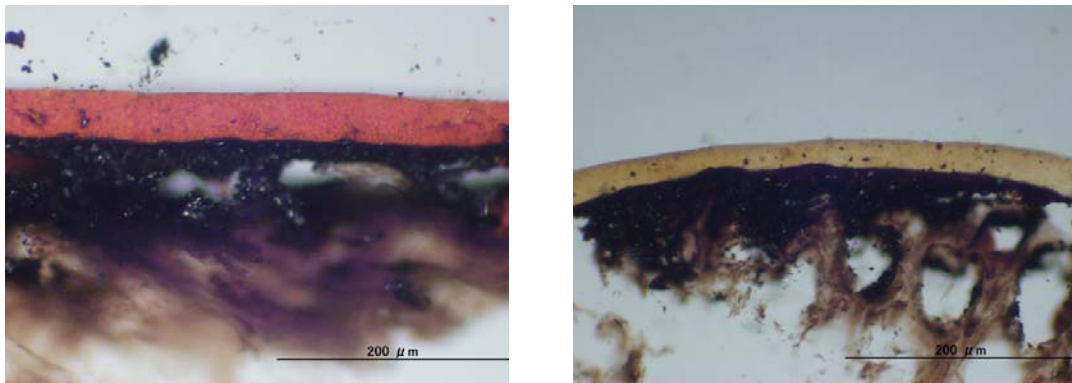
図 117. 漆塗椀 No.23 の塗膜断面落射観察画像 (左図：23-内赤、右図：23-外黒)
