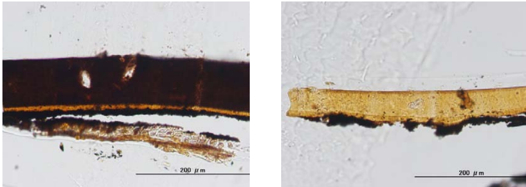
図 156. 漆塗椀 No.31 の塗膜断面透過観察画像 (左図：31-内赤、右図：31-外黒)
