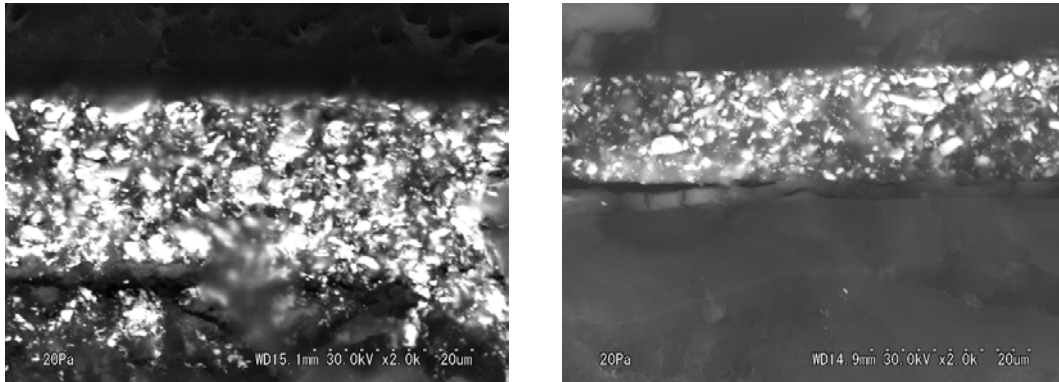
図 205. 漆塗椀 No.16 の塗膜断面 SEM 画像 (左図 : 16-内赤、右図 : 16-外赤) 漆塗椀 No.16 における朱の粒径は 1.0\sim 4.2\mu\text{m} で、大きさは不揃いで、密度は大きい (図 205)。
