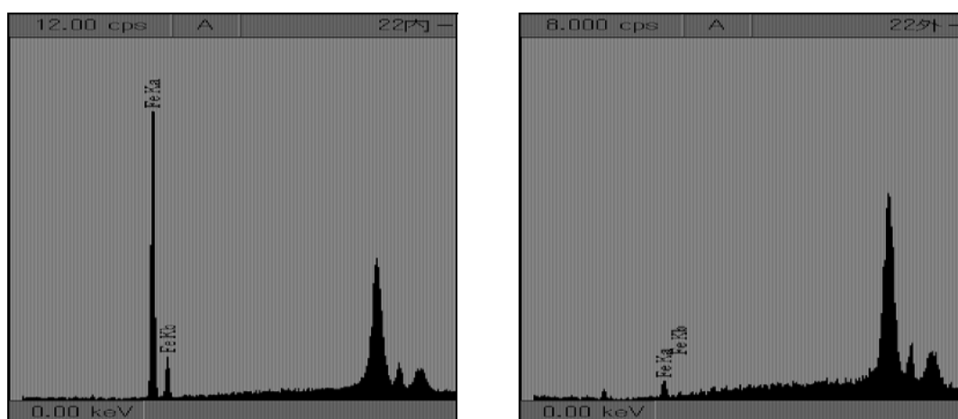
図 110. 漆塗椀 No.22 の XRF 測定結果（左図：22-内赤、右図：22-外黒）
