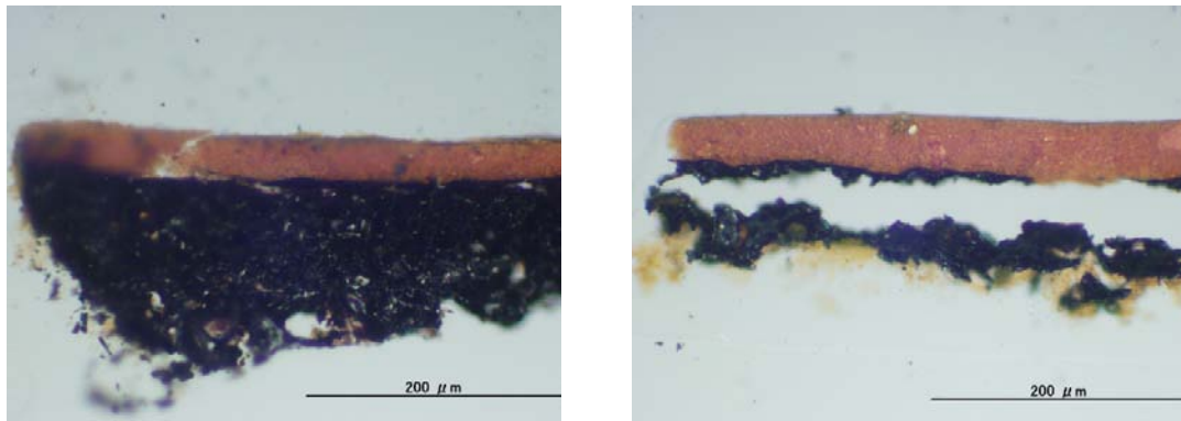
図 25. 漆塗椀 No.5 の塗膜断面落射観察画像 (左図 : 05-内赤、右図 : 05-外赤)
