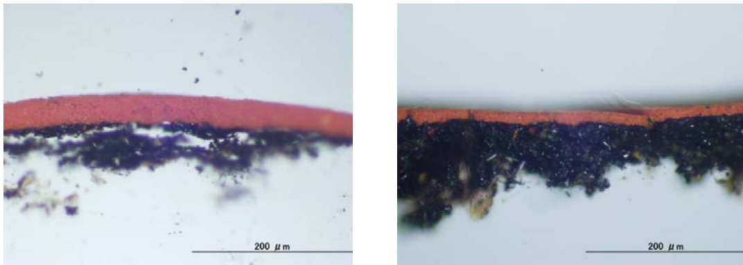
図 97. 漆塗椀 No.19 の塗膜断面落射観察画像 (左図 : 19-内赤、右図 : 19-外赤)
