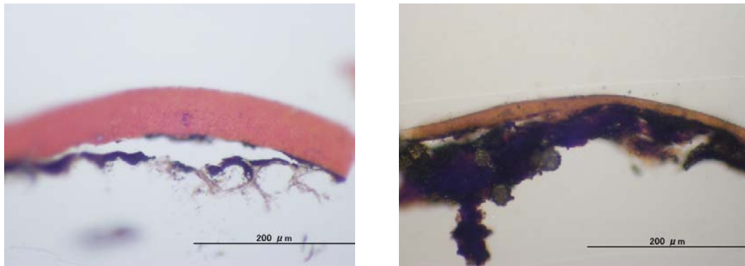
図 87. 漆塗箸 No.17 の塗膜断面落射観察画像（左図：17-赤、右図：17-黒）
