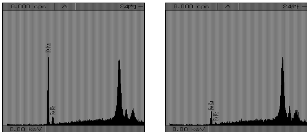
図 120. 漆塗椀 No.24 の XRF 測定結果（左図：24-内赤、右図：24-外黒）
