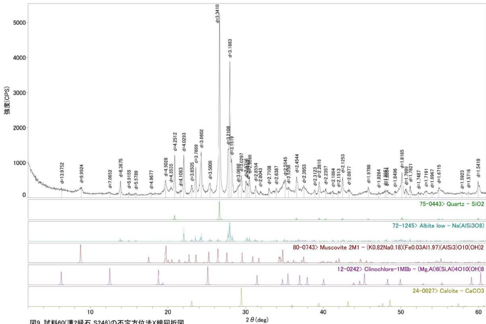
図9. 試料60(溝2緑石 S246)の不定方位法X線回折図
