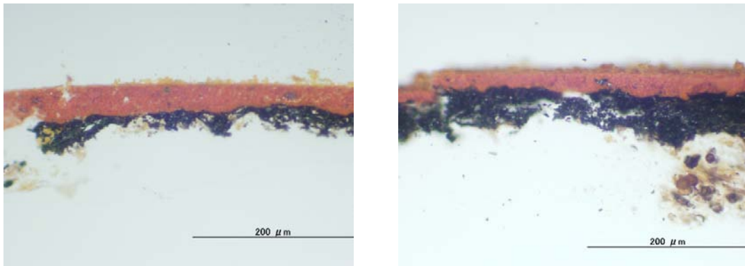
図 92. 漆塗腕 No.18 の塗膜断面落射観察画像 (左図 : 18-内赤、右図 : 18-外赤)
