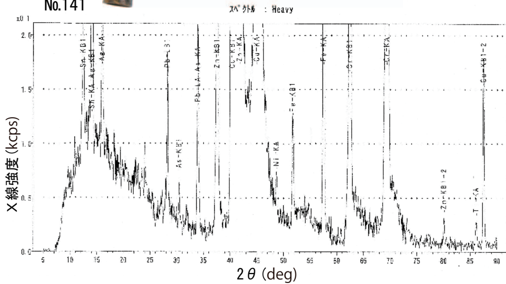
図 26(8) No. 140 および No. 141 の蛍光 X線定性チャート
