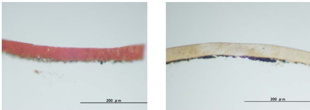
図 137. 漆塗椀 No.27 の塗膜断面落射観察画像 (左図：27-内赤、右図：27-外黒)
