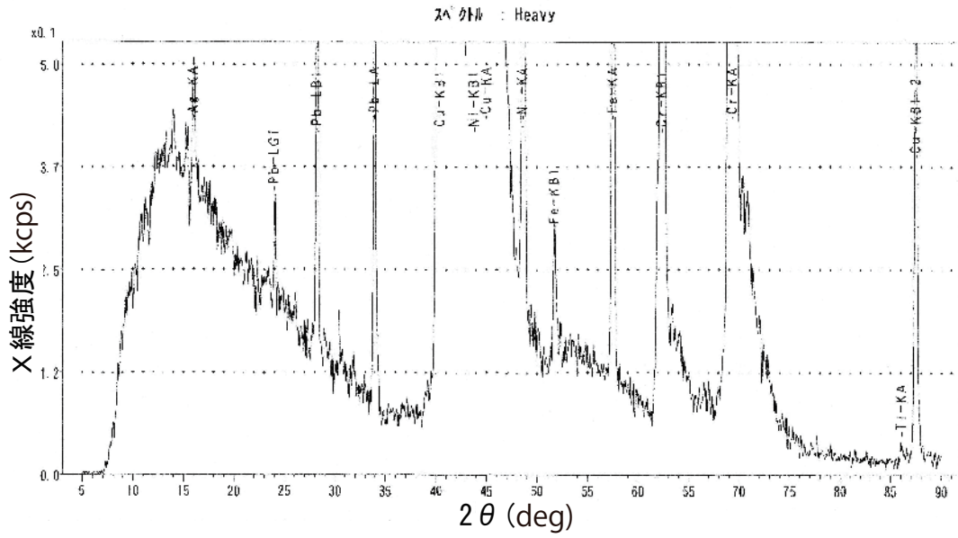
図 26(11) No. 146 の蛍光X線定性チャート
