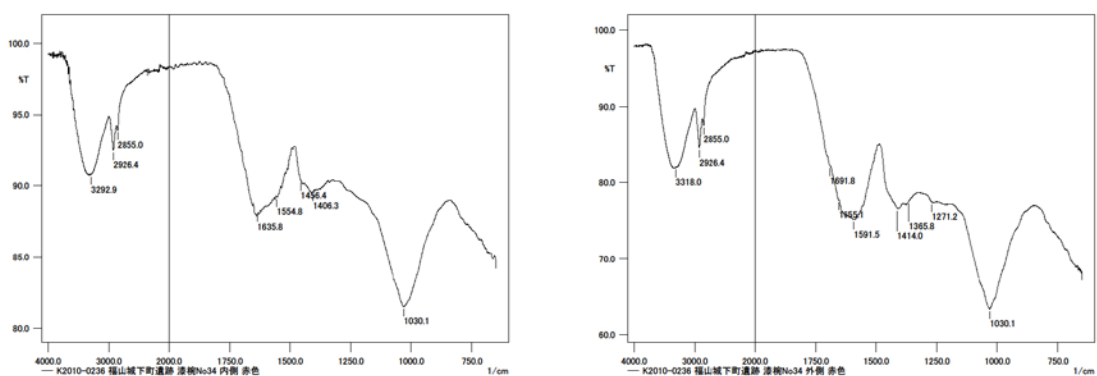
図 169. 漆塗椀 No.34 の ATR-FTIR 測定結果（左図：34-内赤、右図：34-外赤）
