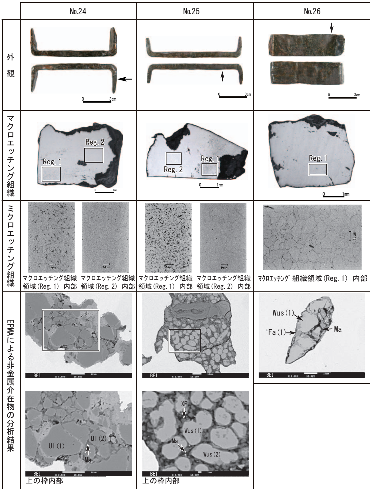
図13 No. 24～26の組織観察結果
