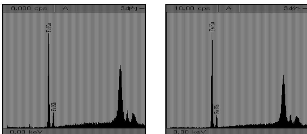
図 170. 漆塗椀 No.34 の XRF 測定結果（左図：34-内赤、右図：34-外赤）
