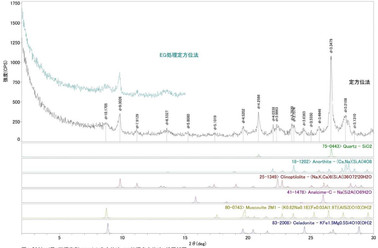
図4. 試料29(藏2石垣東側 S222)の定方位法・EG処理定方位法X線回折図
