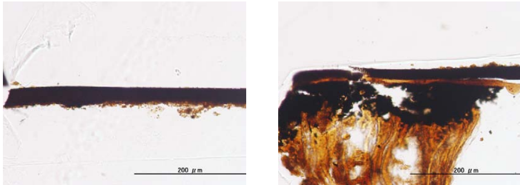
図 81. 漆塗椀 No.16 の塗膜断面透過観察画像 (左図：16-内赤、右図：16-外赤)
