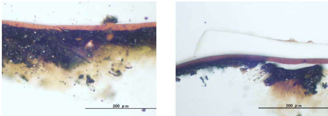
図 162. 漆塗椀 No.32 の塗膜断面落射観察画像 (左図：32-内赤、右図：32-外黒)
