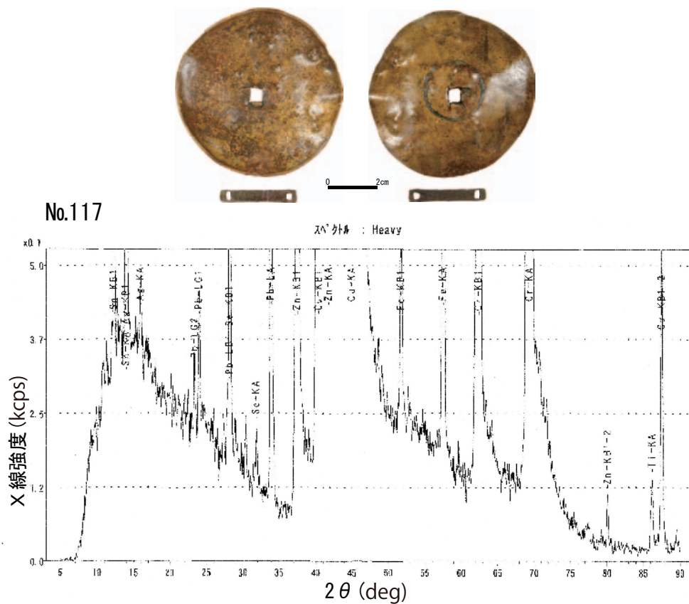
図 26(3) No. 114 および No. 117 の蛍光X線定性チャート
