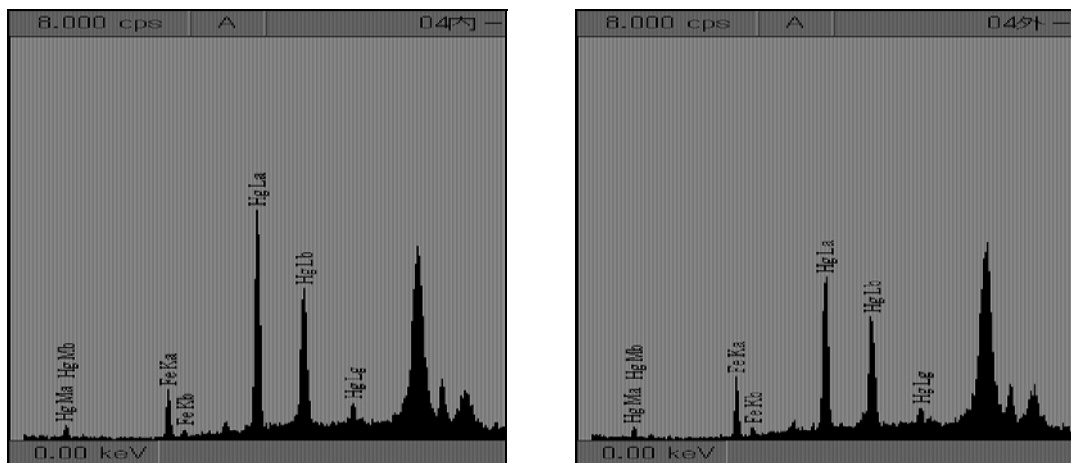
図 18. 漆塗椀 No.4 の XRF 測定結果（左図：04-内赤、右図：04-外赤）
