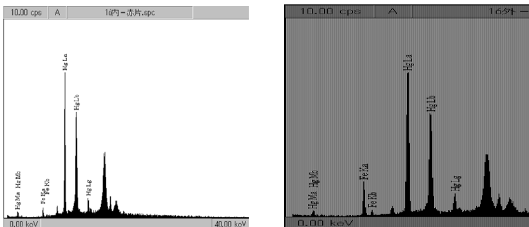
図 80. 漆塗椀 No.16 の XRF 測定結果 (左図：16-内赤、右図：16-外赤)
