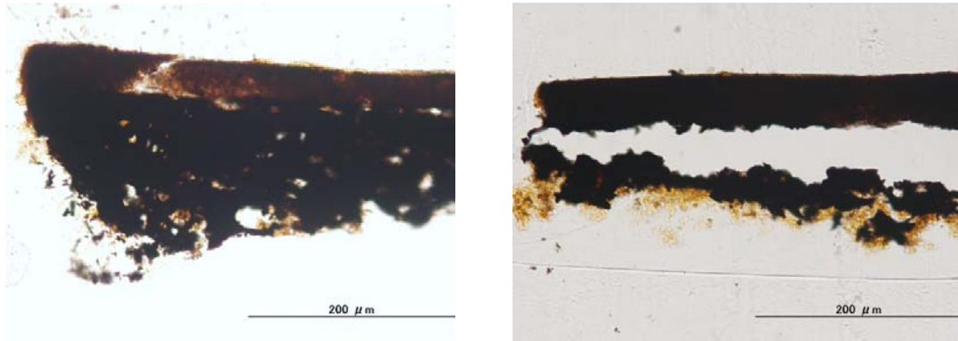
図 24. 漆塗椀 No.5 の塗膜断面透過観察画像 (左図 : 05-内赤、右図 : 05-外赤)
