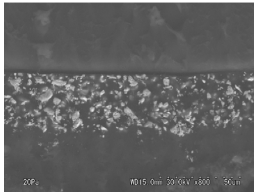
図 206. 漆塗椀 No.20 の塗膜断面 SEM 画像 漆塗椀 No.20 における朱の粒径は 1.7\sim 7.0\mu\text{m} で、大きさは比較的均質であった (図 206)。
