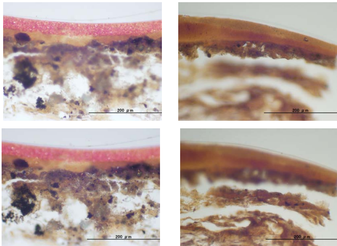
図 102. 漆塗椀 No.20 の塗膜断面落射観察画像 (左図：20-内赤、右図：20-外黒)
