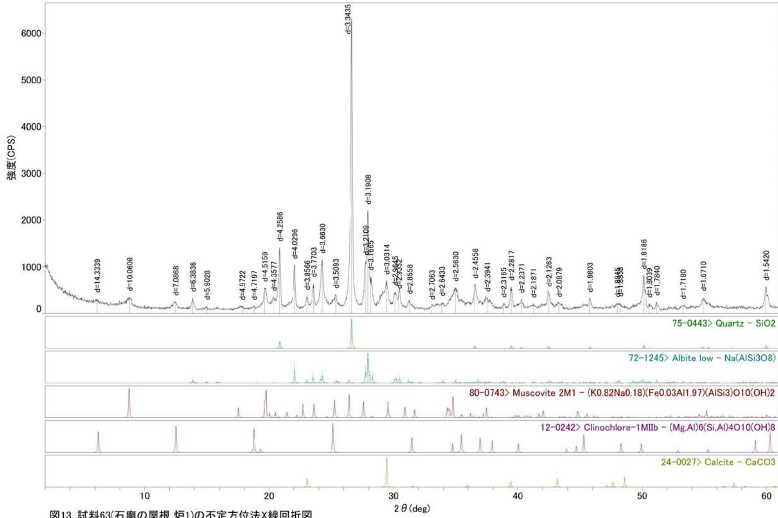
図13. 試料63(石廟の屋根 炉1)の不定方位法X線回折図
