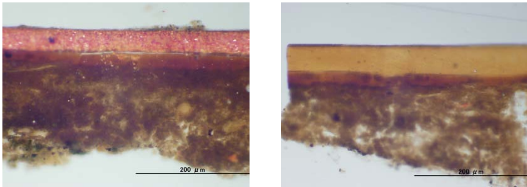
図 152. 漆塗椀 No.30 の塗膜断面落射観察画像 (左図：30-内赤、右図：30-外黒)
