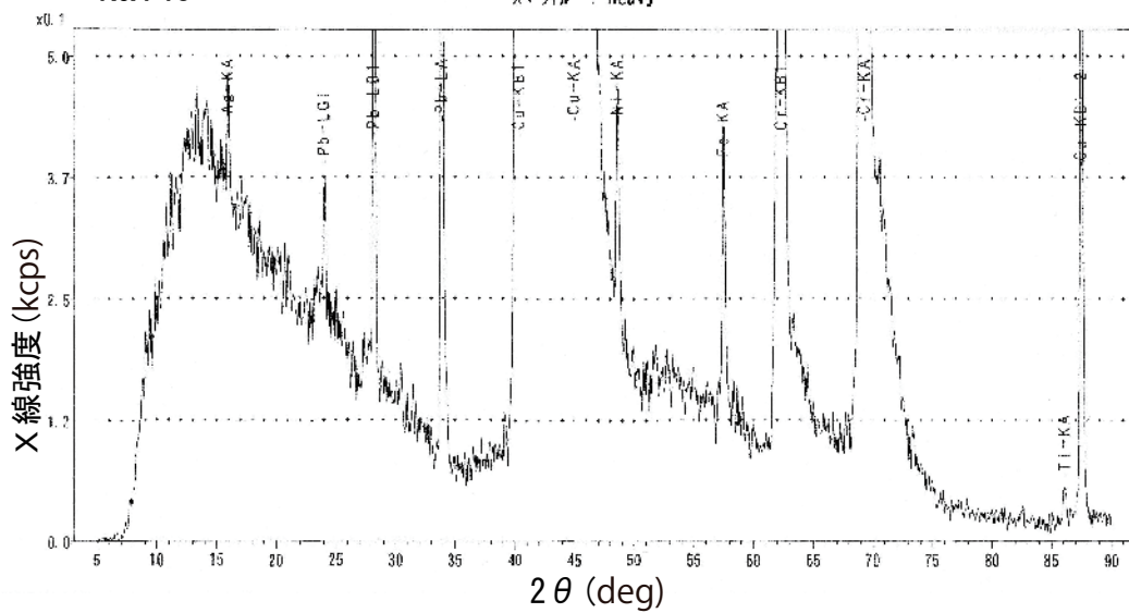
図 26(10) No. 144 および No. 145 の蛍光X線定性チャート
