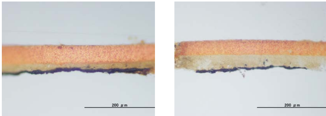
図 142. 漆塗椀 No.28 の塗膜断面落射観察画像 (左図：28-内茶、右図：28-外茶)
