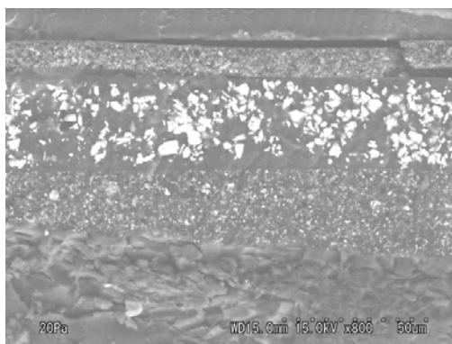
図 203. 漆塗椀 No.7 の塗膜断面 SEM 画像 漆塗椀 No.7 における朱の粒径は 2.4\sim 7.5\mu\text{m} で、大きさは比較的均質であった（図 203）。
