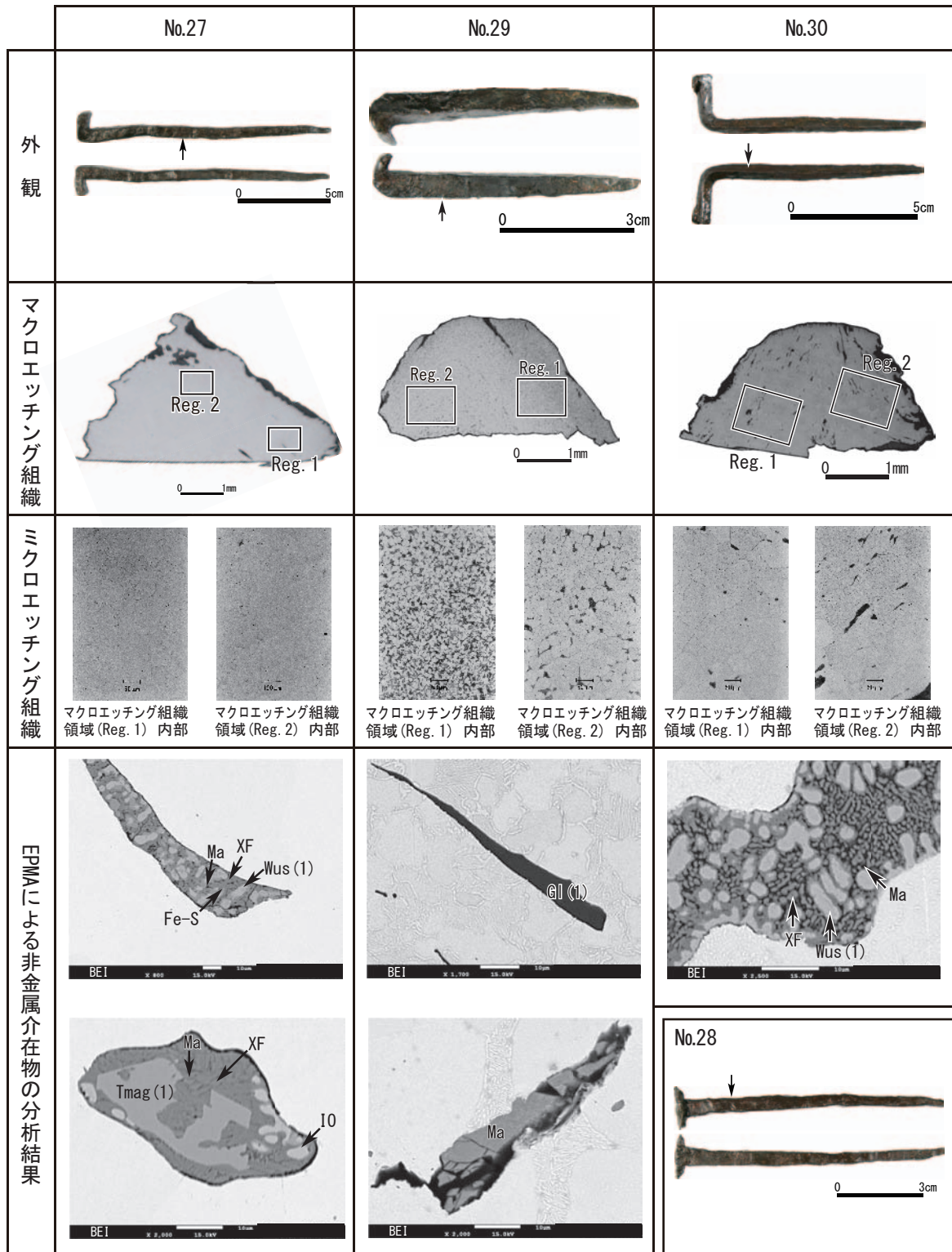
図14 No. 27・29・30の組織観察結果およびNo. 28の外観
