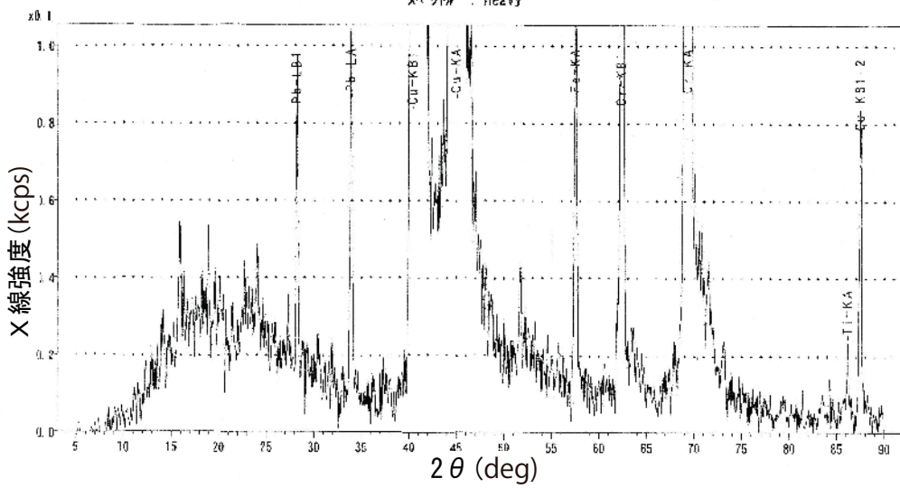
図 26(5) No. 134 および No. 135 の蛍光 X 線定性チャート
