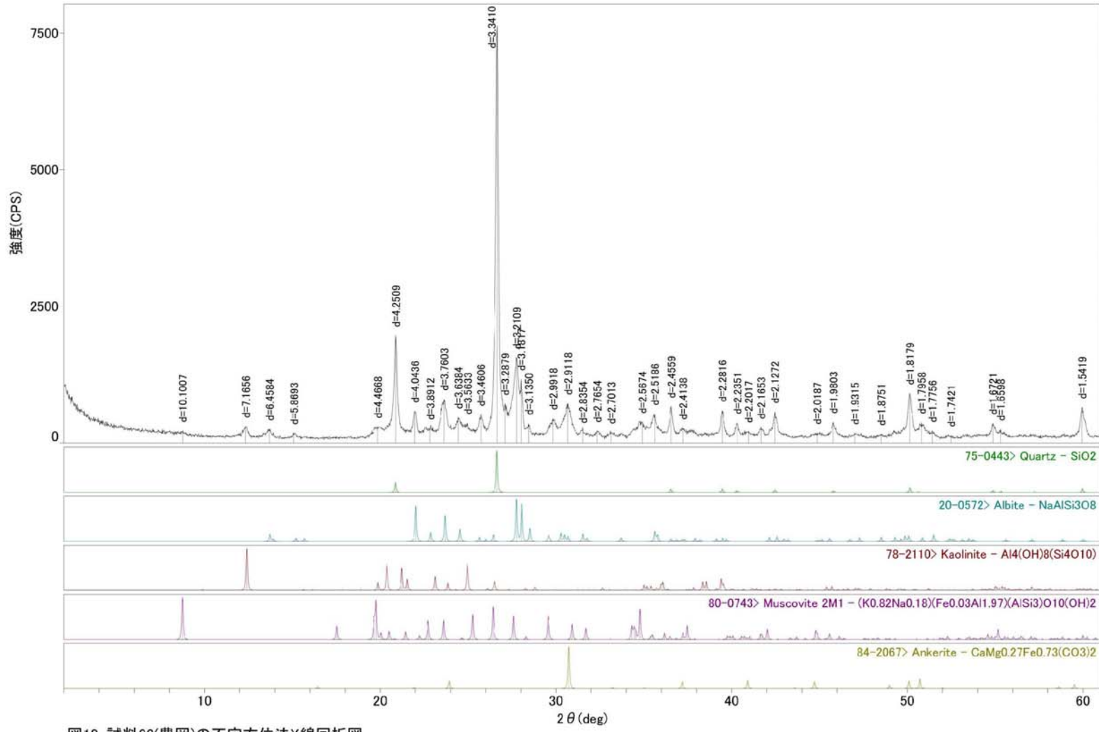
図19. 試料66(豊岡)の不定方位法X線回折図
