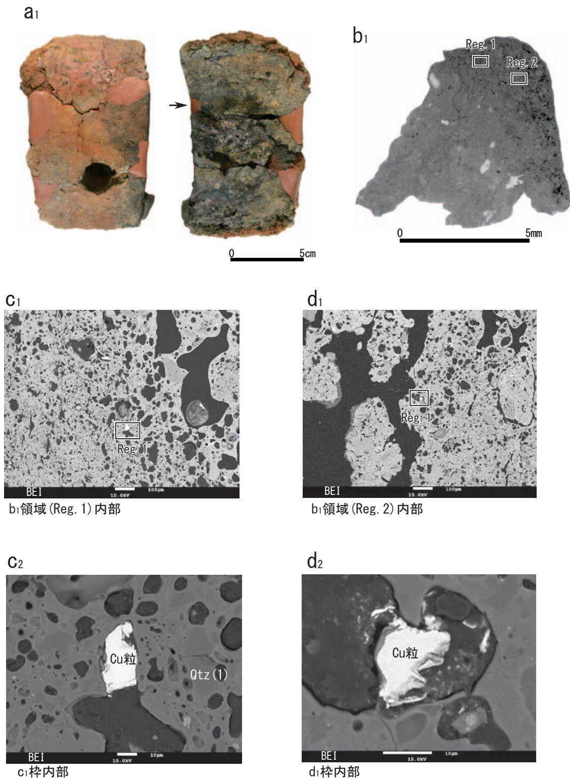
図41 No. 147の組織観察結果
