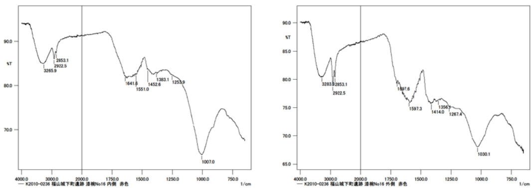
図 79. 漆塗椀 No.16 の ATR-FTIR 測定結果 (左図：16-内赤、右図：16-外赤)
