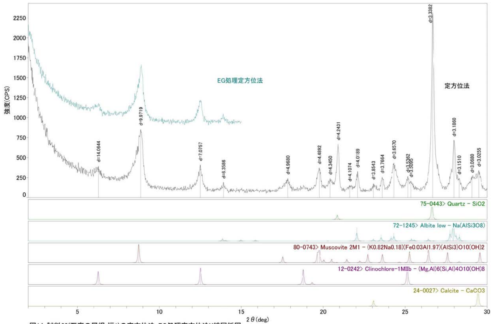
図14. 試料63(石廟の屋根 炉1)の定方位法・EG処理定方位法X線回折図
