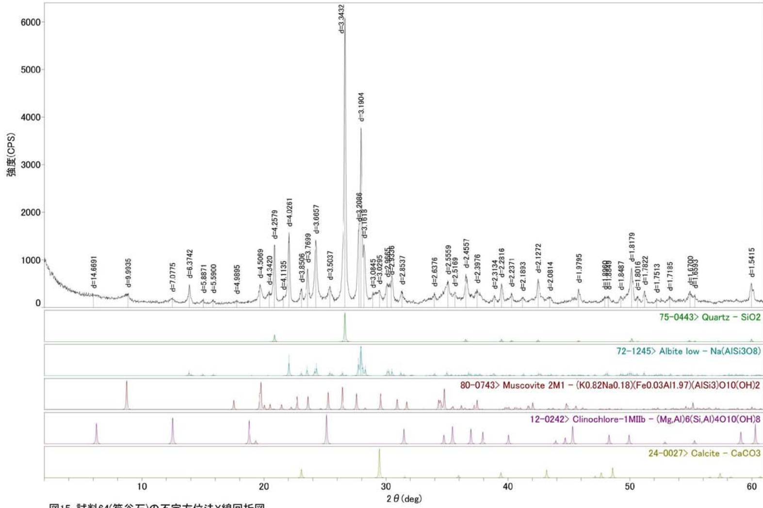
図15. 試料64(笏谷石)の不定方位法X線回折図
