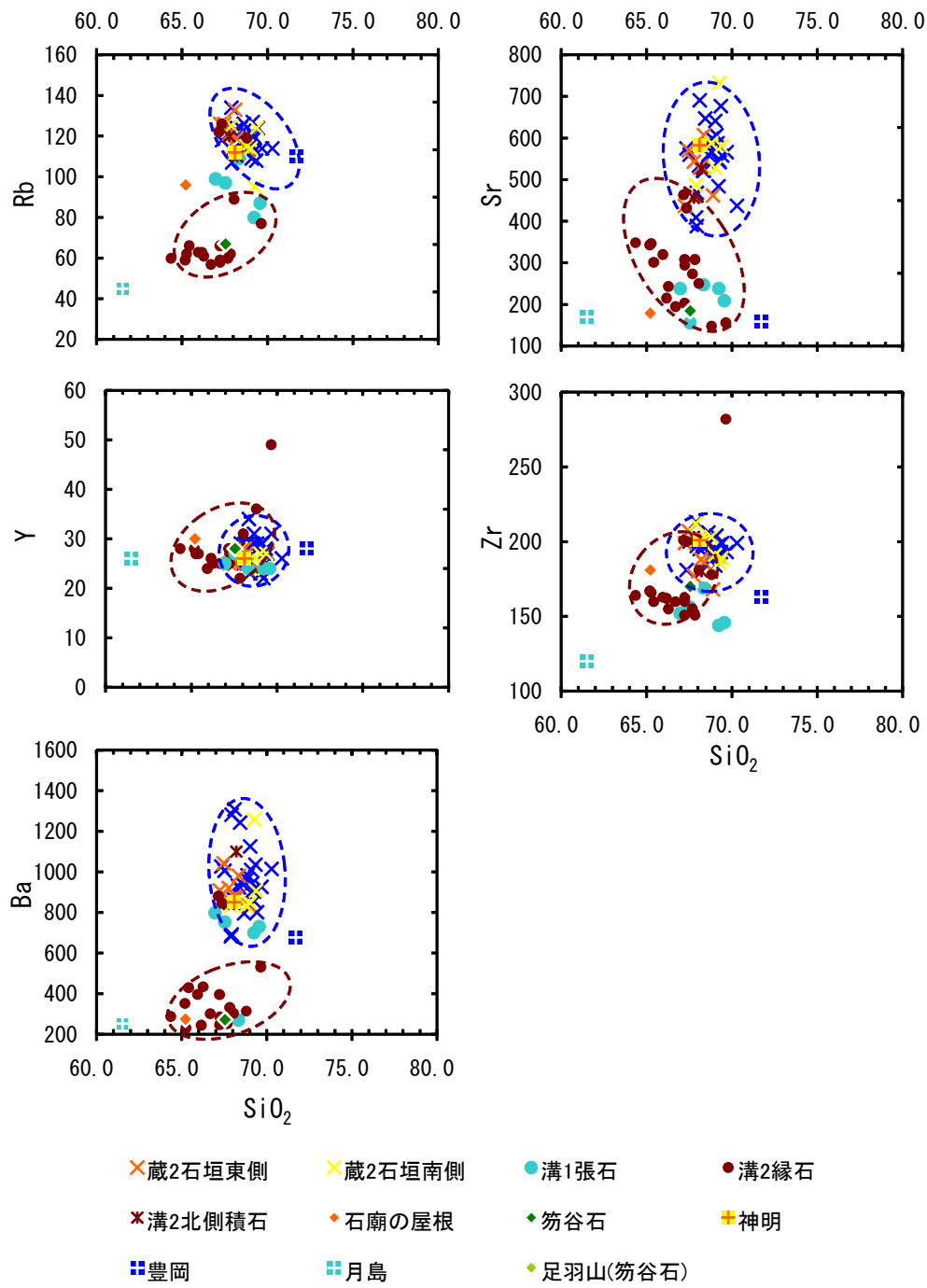
図25 微量成分元素のハーカーク
