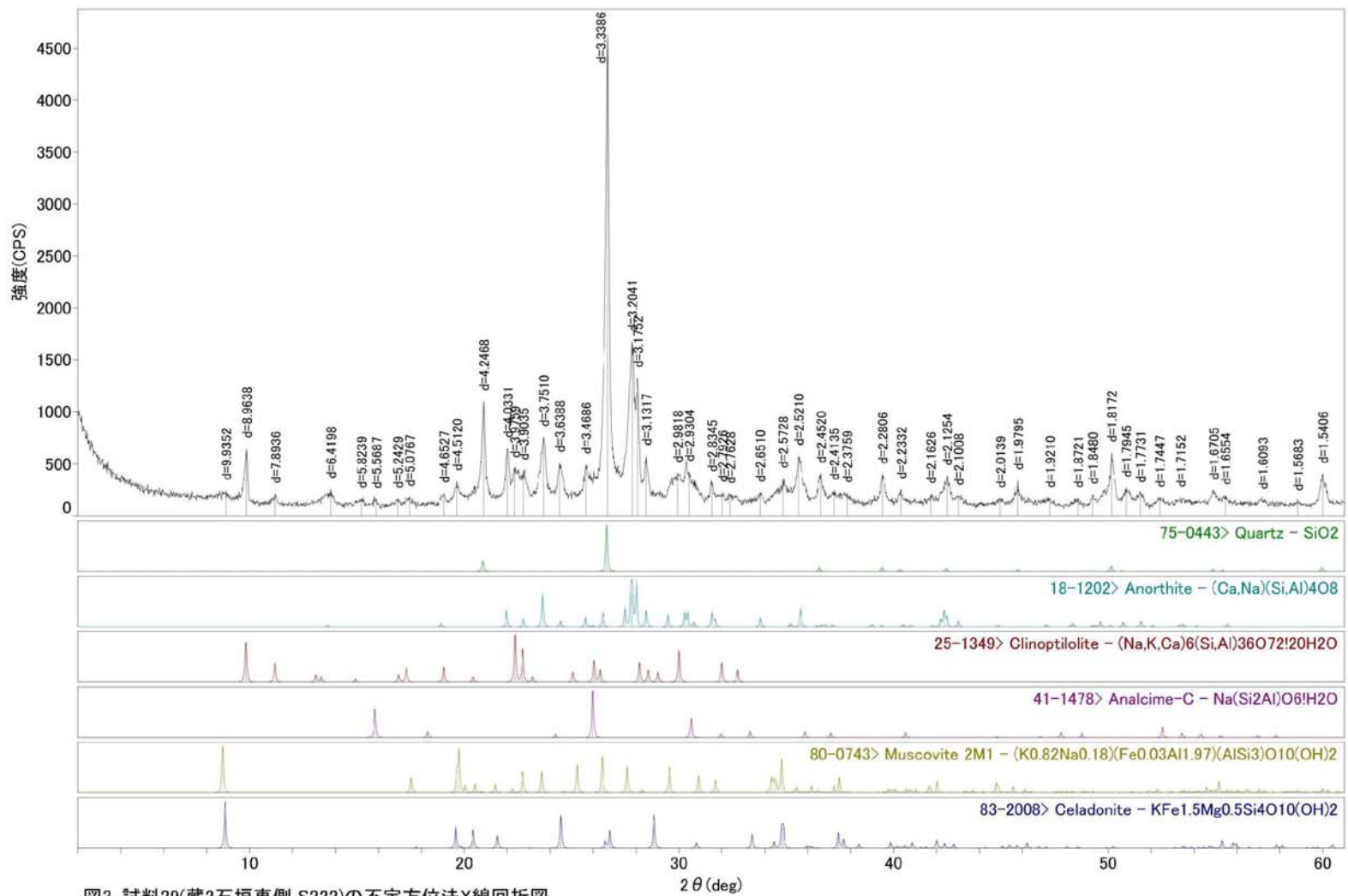
図3. 試料29(藏2石垣東側 S222)の不定方位法X線回折図
