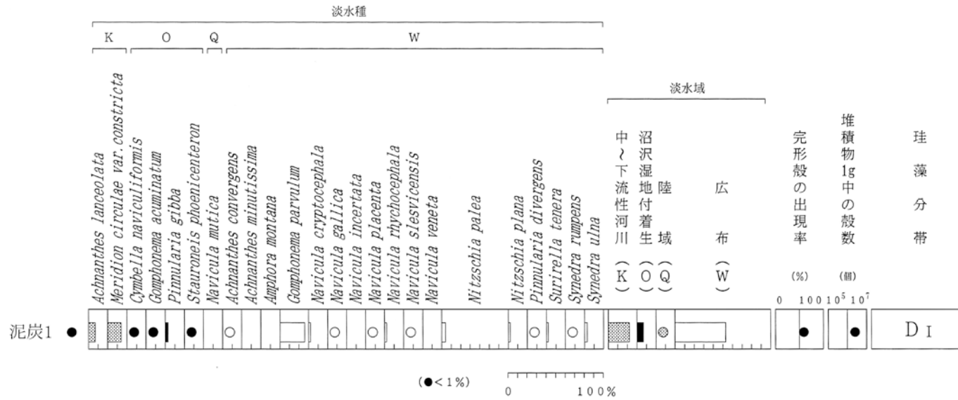
図2 堆積物中の珪藻化石分布図 (1.0%以上の分類群を表示)
