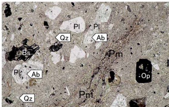
6. グループD 試料42 溝1張石 S253 デイサイト質溶結結晶質凝灰岩
