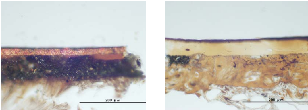
図 107. 漆塗椀 No.21 の塗膜断面落射観察画像 (左図：21-内赤、右図：21-外黒)
