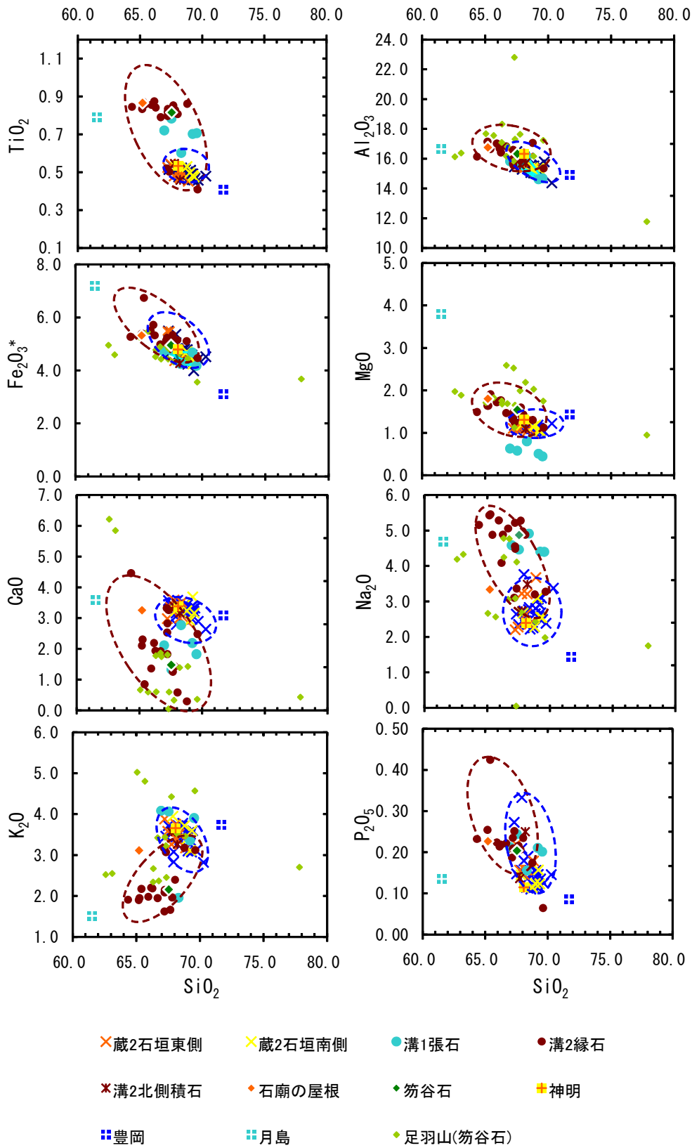
図24 主成分元素のハーカー図
