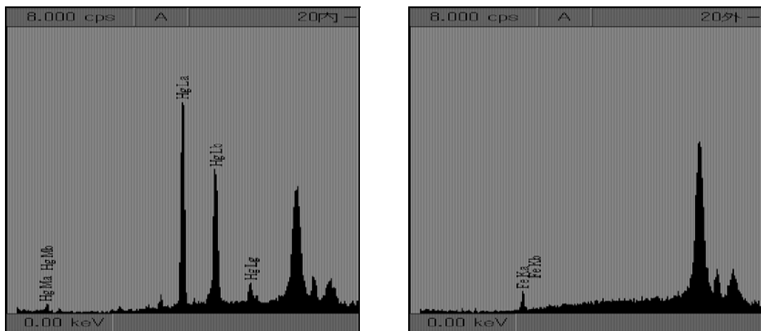
図 100. 漆塗椀 No.20 の XRF 測定結果 (左図 : 20-内赤、右図 : 20-外黒)
