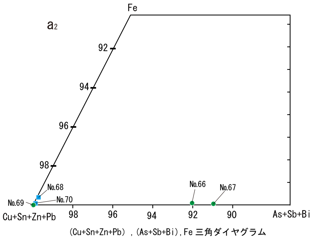
図 30 装身具 (No. 66 ~ 70) に含有される主成分および微量成分の三角ダイヤグラム No. は表 9 に対応。■ = 真鍮を素材とする試料、● = Cu または Cu-Pb 合金を素材とする試料。
