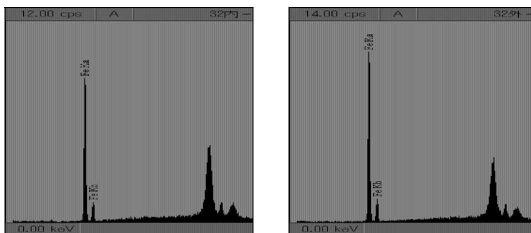
図 160. 漆塗椀 No.32 の XRF 測定結果（左図：32-内赤、右図：32-外黒）
