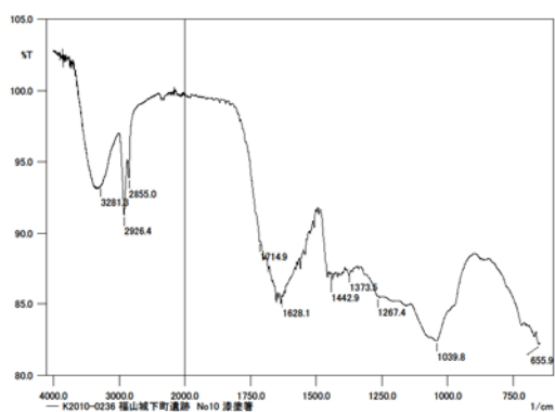
図 49. 漆塗箸 No.10 の ATR-FTIR 測定結果
