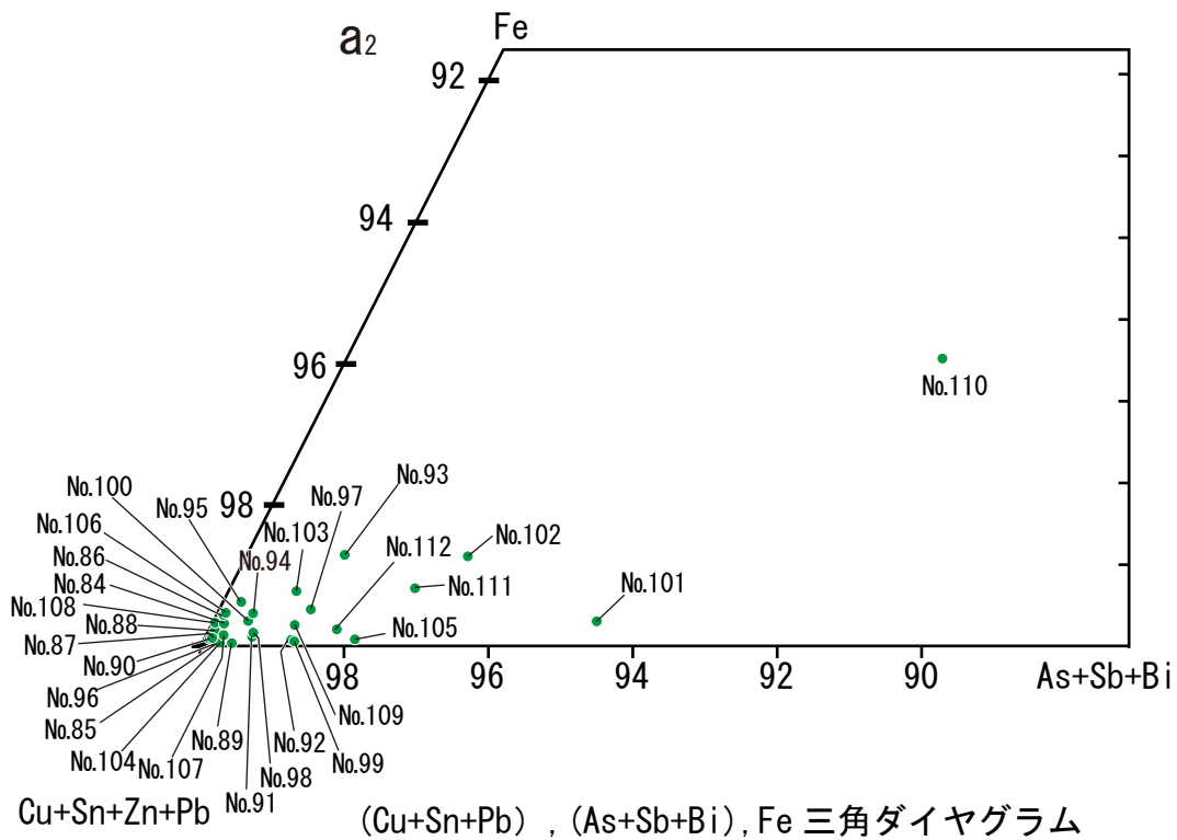
図 36 錢貨 (No. 84 ~ 112) に含有される主成分および微量成分の三角ダイヤグラム No. は表 9 に対応。■ = 真鍮を素材とする試料、● = Cu、Cu-Pb、または青銅を素材とする試料。
