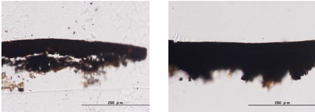
図 96. 漆塗椀 No.19 の塗膜断面透過観察画像 (左図 : 19-内赤、右図 : 19-外赤)
