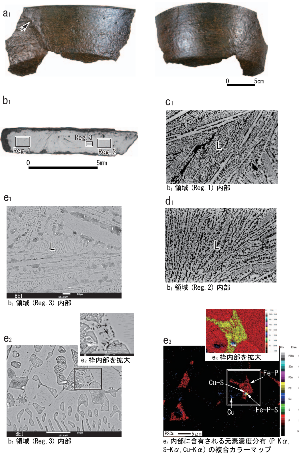
図2 No. 2の組織観察結果
