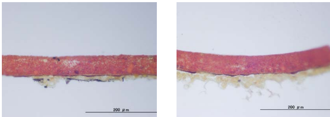
図 72. 漆塗箱物 No.14 の塗膜断面落射観察画像 (左図：14-表赤、右図：14-裏赤)
