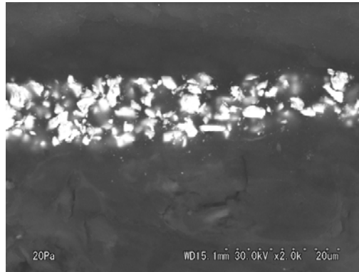
図 208. 漆塗部材 No.26 の塗膜断面 SEM 画像
