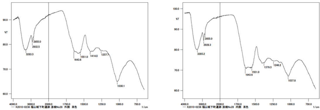
図 139. 漆塗椀 No.28 の ATR-FTIR 測定結果（左図：28-内茶、右図：28-外茶）
