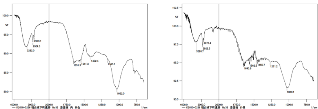
図 164. 漆塗椀 No.33 の ATR-FTIR 測定結果（左図：33-内赤、右図：33-外黒）
