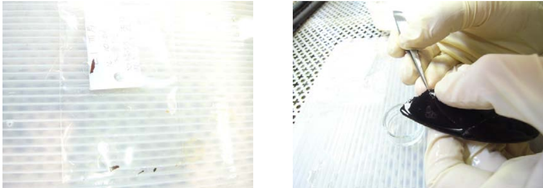
図 148. 漆塗椀 No.30 の塗膜採取箇所（左図：30-内赤、右図：30-外黒）
