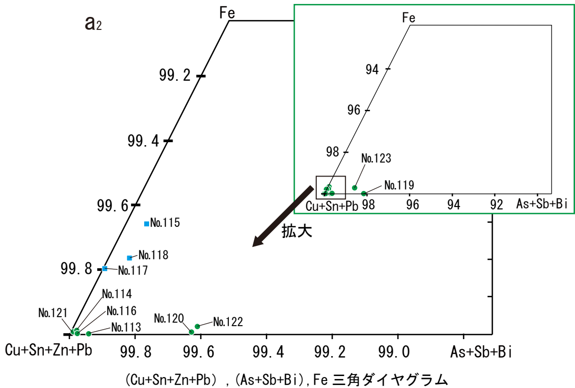
図 38 不定銅製品 (No. 113 ~ 123) に含有される主成分および微量成分の三角ダイヤグラム
