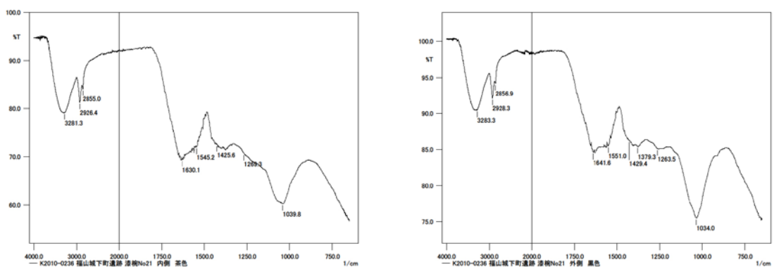
図 104. 漆塗椀 No.21 の ATR-FTIR 測定結果（左図：21-内赤、右図：21-外黒）
