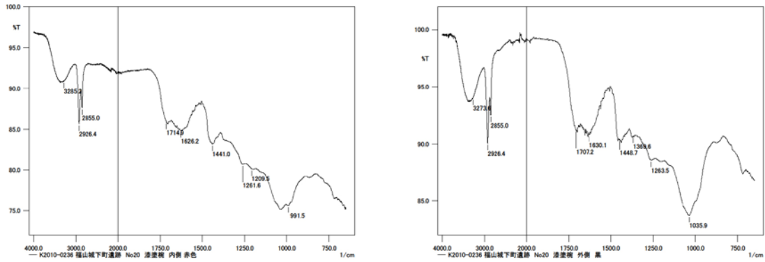
図 99. 漆塗椀 No.20 の ATR-FTIR 測定結果 (左図 : 20-内赤、右図 : 20-外黒)
