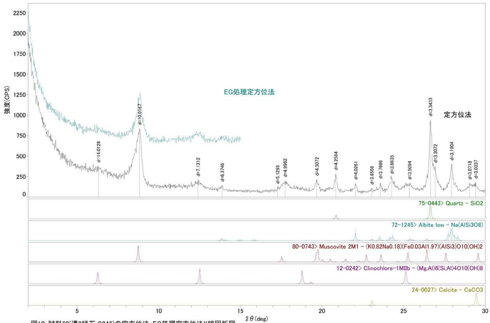
図10. 試料60(溝2緑石 S246)の定方位法・EG処理定方位法X線回折図
