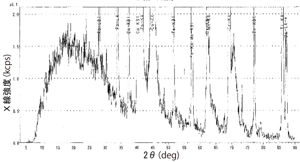
図 26(1) No. 66 および No. 69 の蛍光 X 線定性チャート
