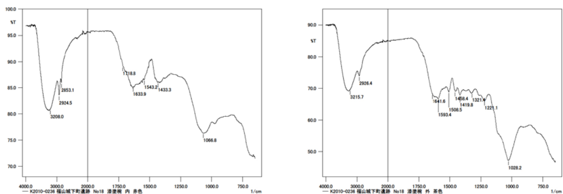
図 89. 漆塗椀 No.18 の ATR-FTIR 測定結果（左図：18-内赤、右図：18-外赤）
