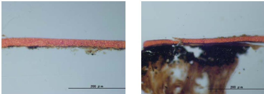
図 82. 漆塗椀 No.16 の塗膜断面落射観察画像 (左図：16-内赤、右図：16-外赤)
