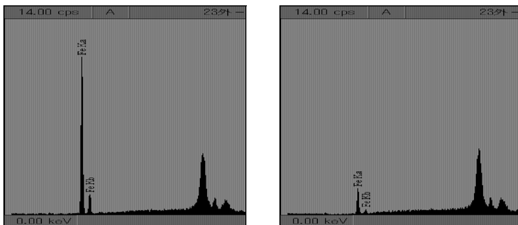
図 115. 漆塗椀 No.23 の XRF 測定結果 (左図 : 23-内赤、右図 : 23-外黒)
