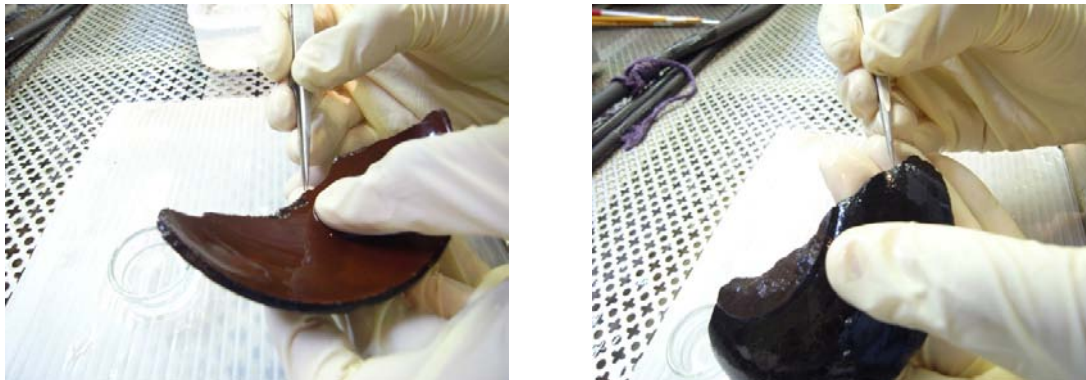
図 153. 漆塗椀 No.31 の塗膜採取箇所（左図：31-内赤、右図：31-外黒）
