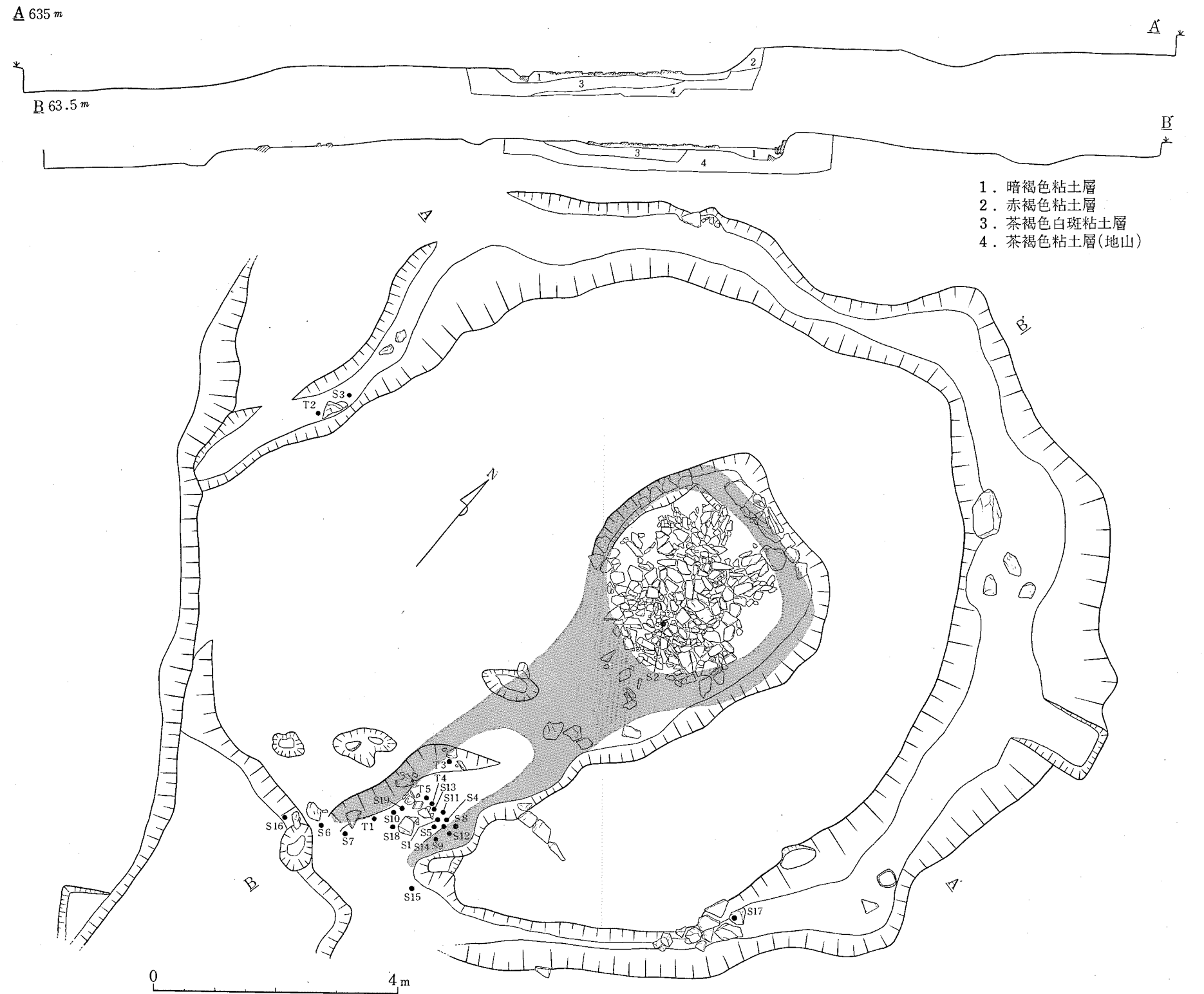
Fig. 24 鱈口古墳実測図(縮尺1/80)
