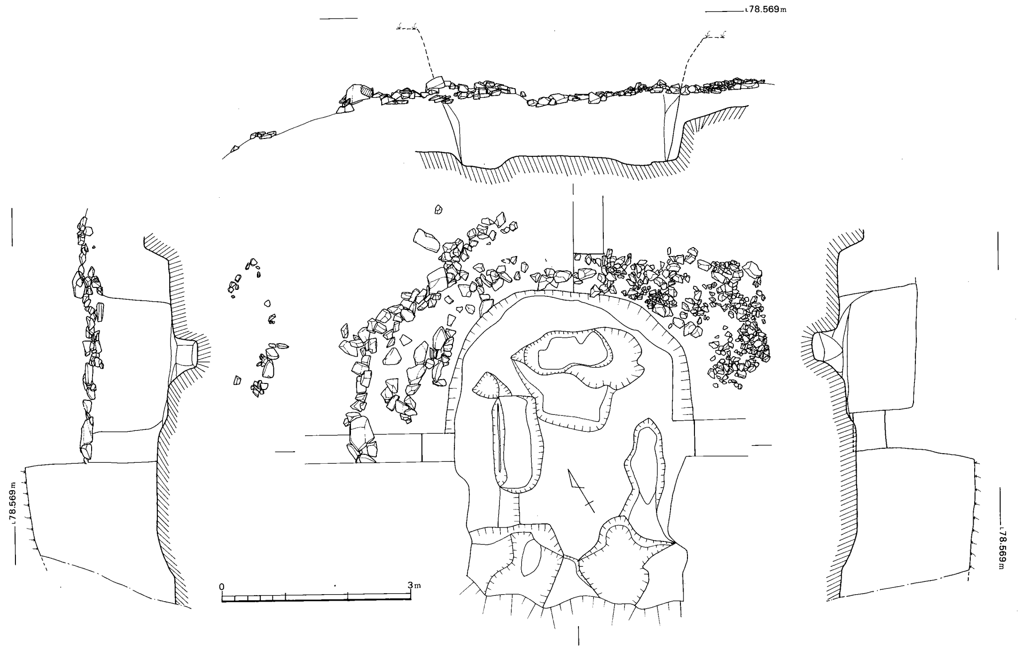
Fig. 7 扇祇 1 号墳石室実測図 (縮尺 1/60)
