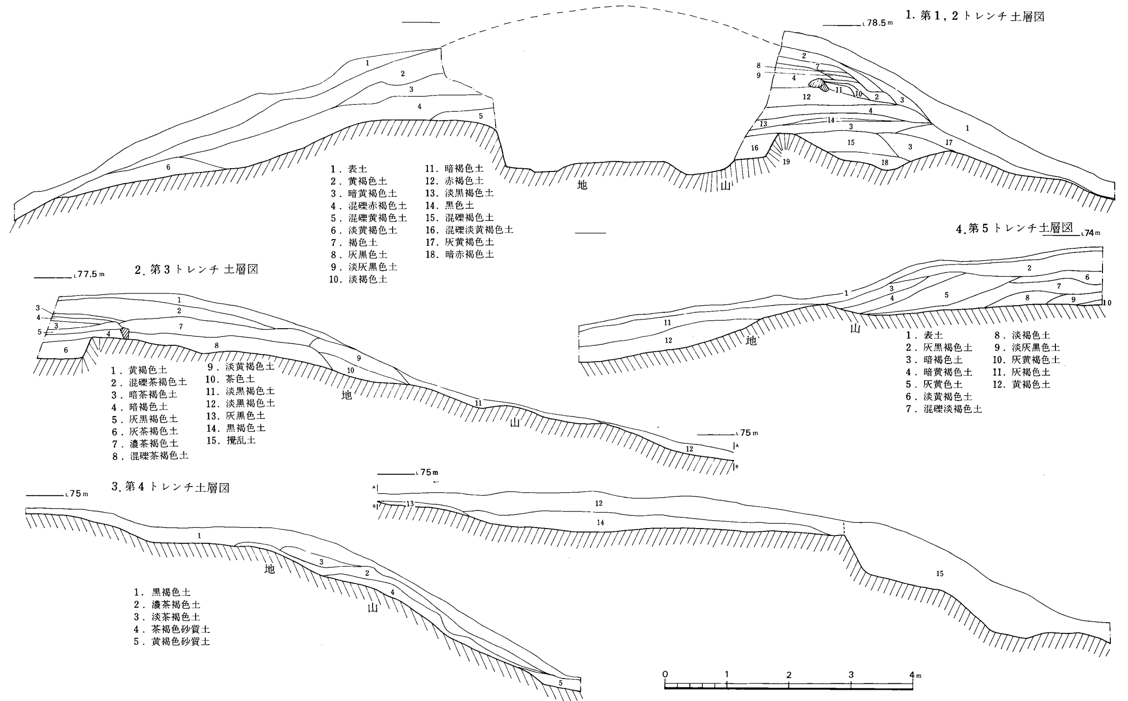
Fig. 6 扇祇1号墳土層図 (縮尺1/60)
