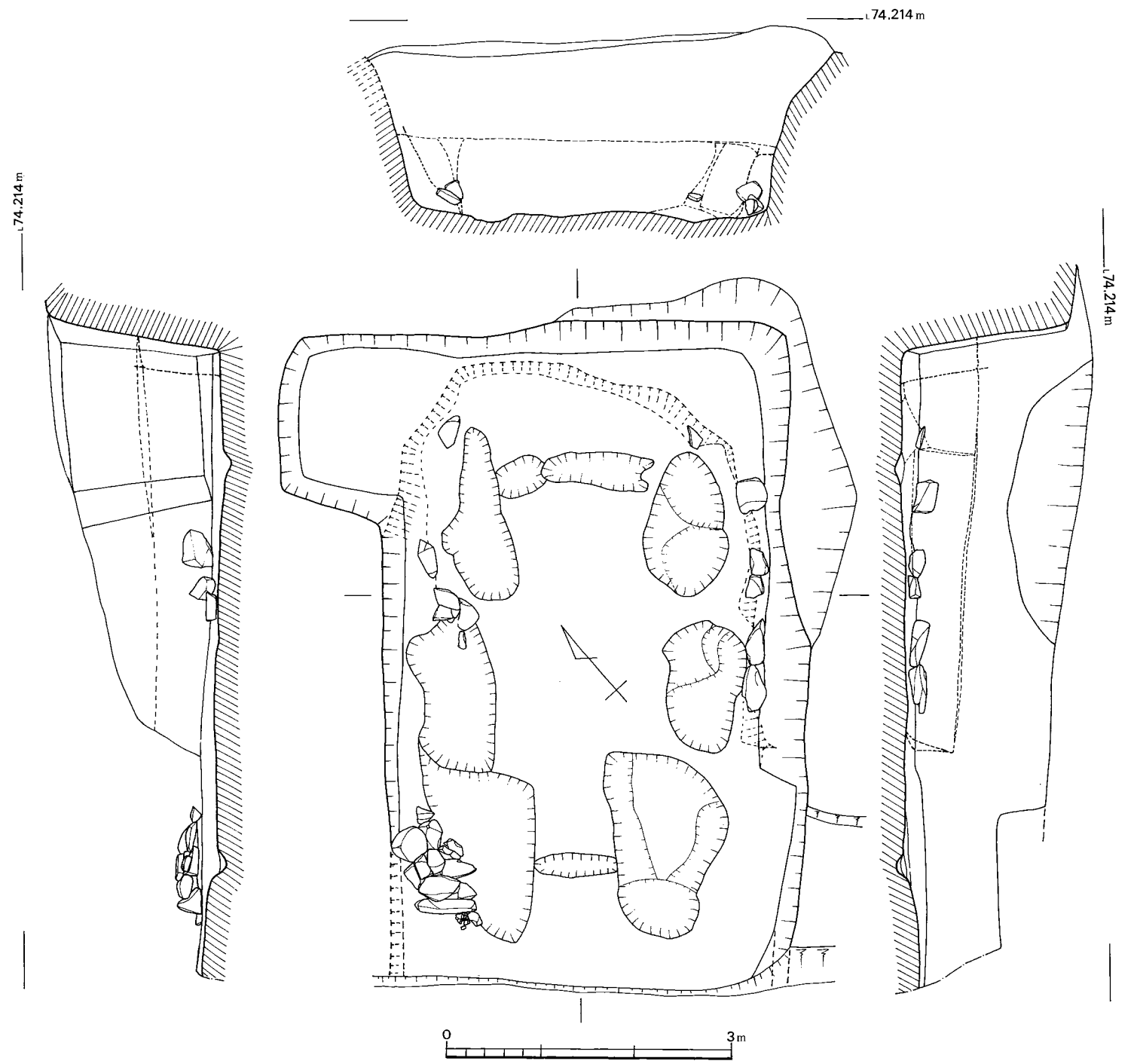
Fig. 14 扇祇 2 号墳石室実測図 (縮尺1/60)
