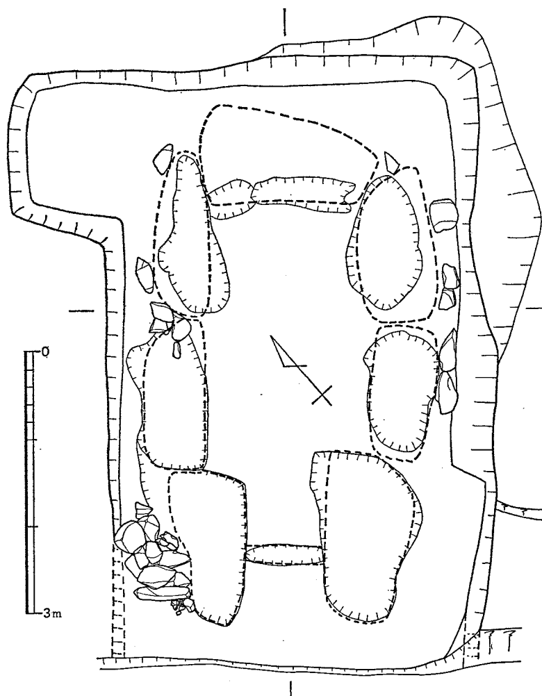
Fig. 15 扇祇2号墳石室復元図 (縮尺1/60)
