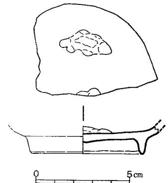
Fig. 36 青磁実測図 (縮尺1/2)
