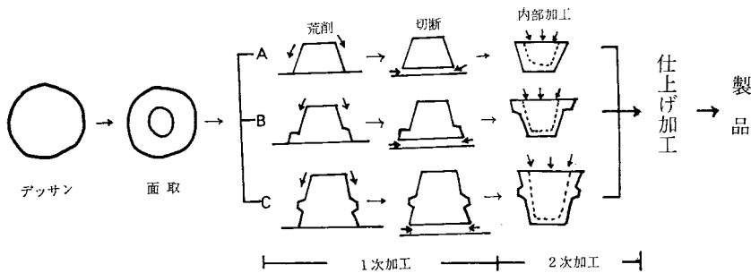
Fig. 44 長崎県西彼杵郡雪ノ浦遺跡石鍋製造模式図
