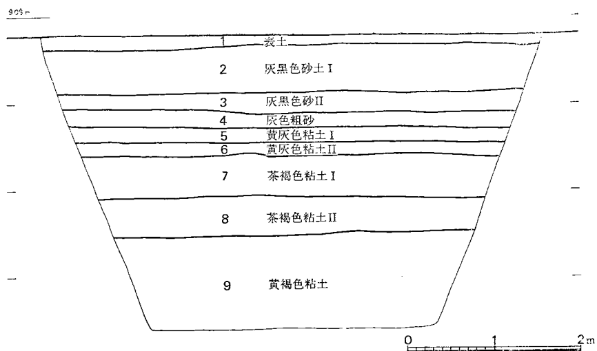
Fig. 21 第2トレンチ土層図 (縮尺1/10)
