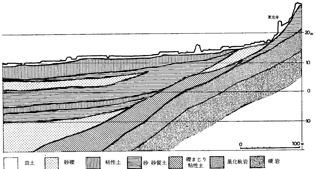
左. Fig. 20-1 筑後川付近ボーリングによる土層図 (縮尺1/4000)
