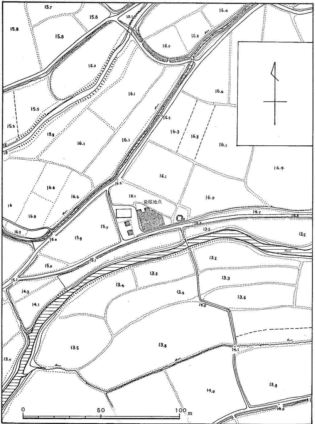
Fig. 30 大地田遺跡地形図 (縮尺1/1500)
