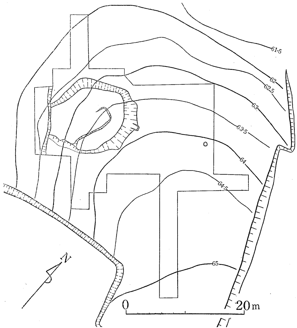
Fig. 23 鱈口古墳地形図 (縮尺 1/400)
