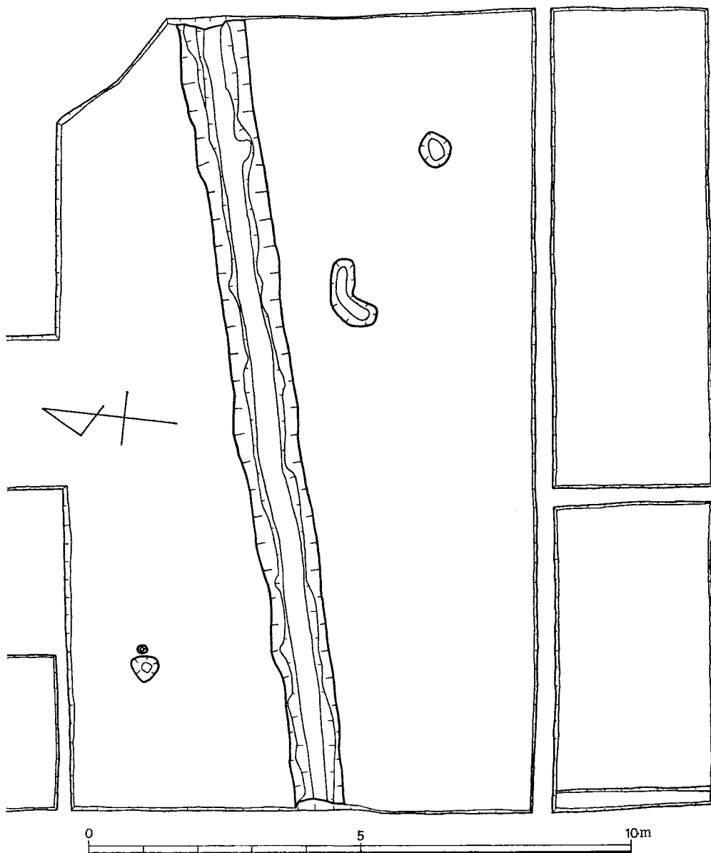
Fig. 33 調査地域平面図 (縮尺1/100)
