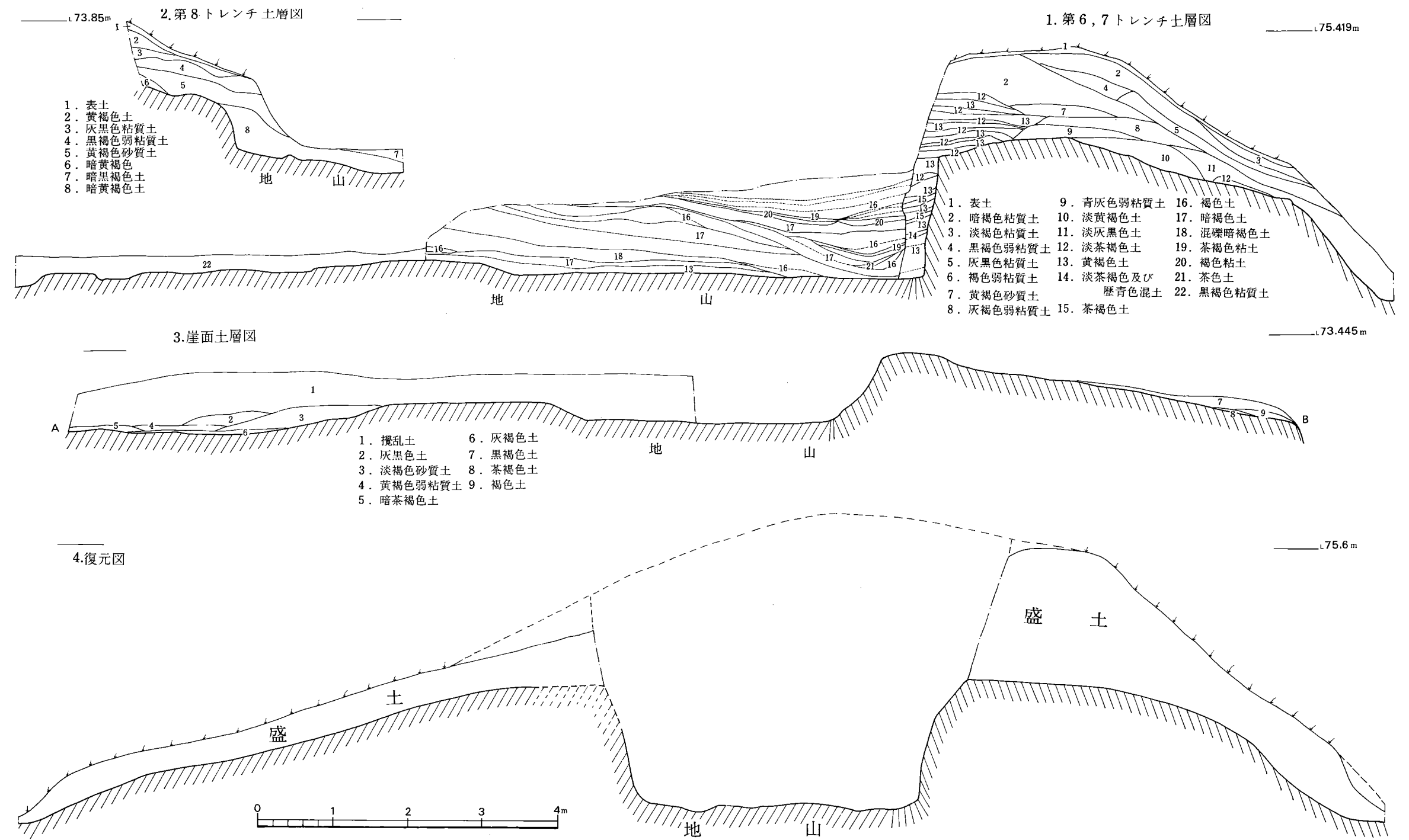
Fig. 13 扇祇2号墳土層図(縮尺1/60)
