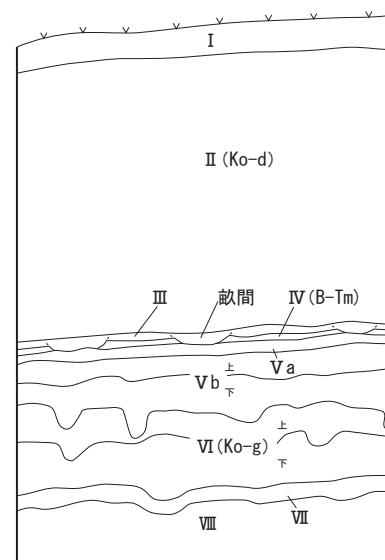
図 I - 4 土層模式図
