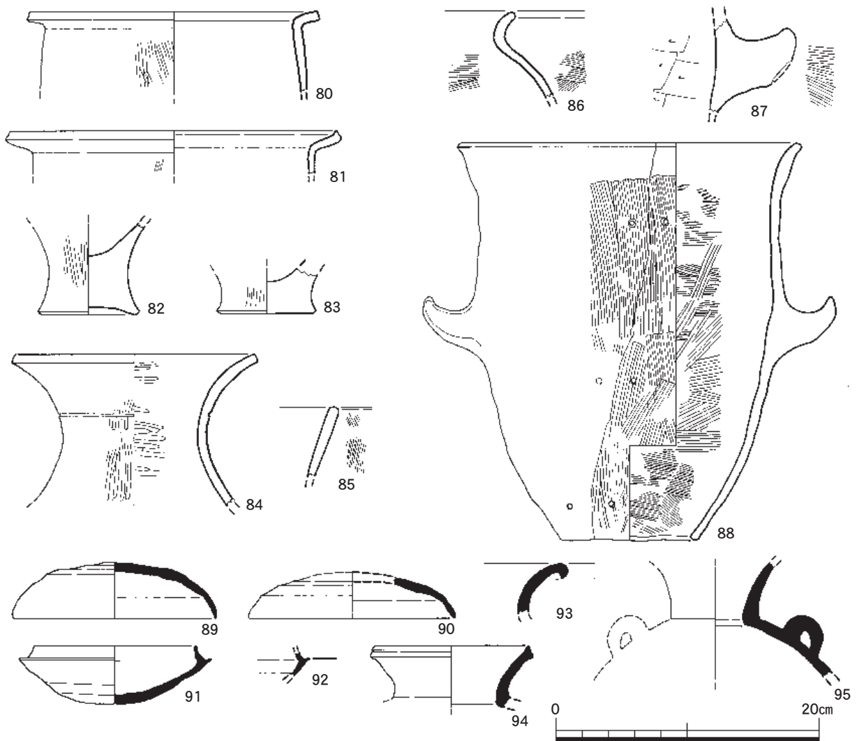
第15図 集石遺構出土遺物実測図（縮尺1/4）
