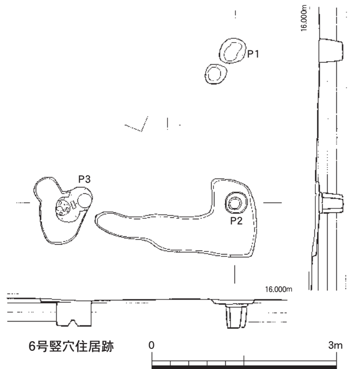
第6図 竪穴住居跡実測図2 (縮尺1/60)
