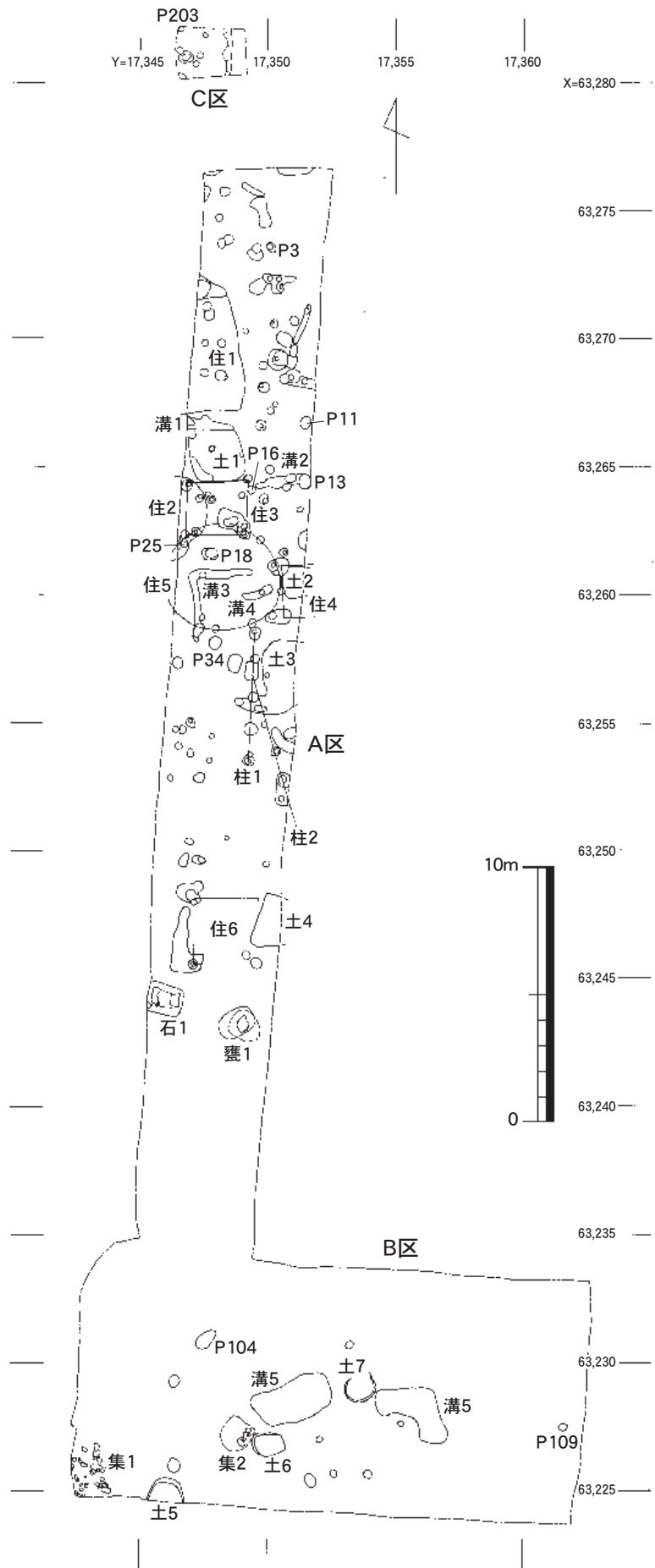
第3図 三口遺跡5次調査全体図 (縮尺1/250)
