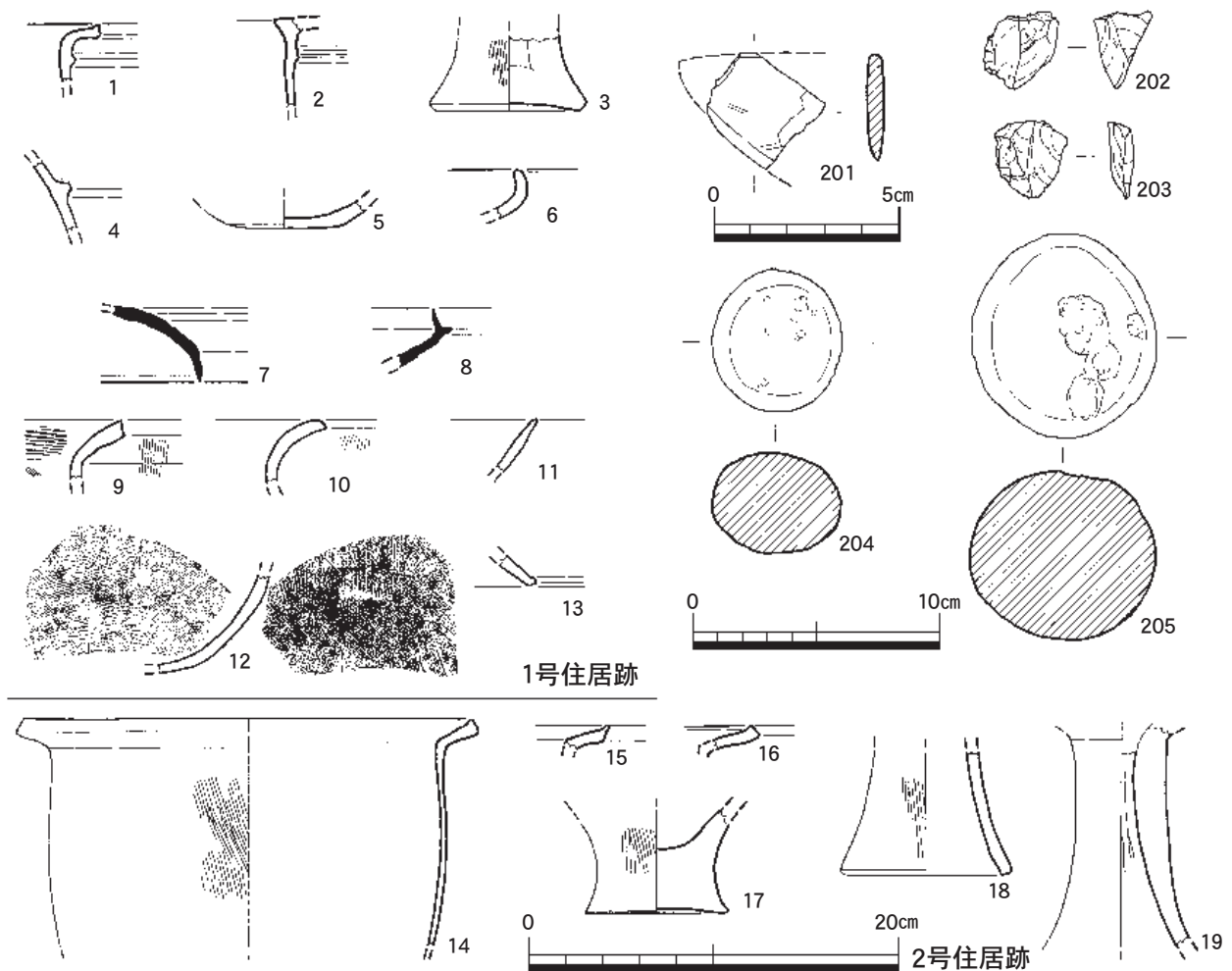
第5図 竪穴住居跡出土遺物実測図1（縮尺1/4（1～19）、縮尺1/2（201～203）、縮尺1/3（204・205））
