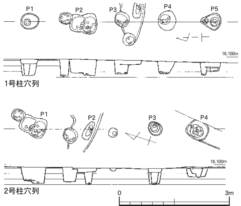
第8図 柱穴列実測図(縮尺1/60)
