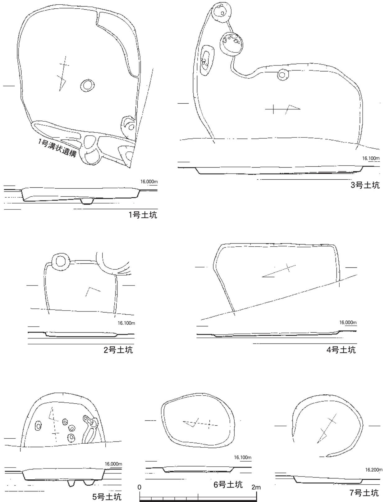
第12図 土坑実測図（縮尺1/40）
