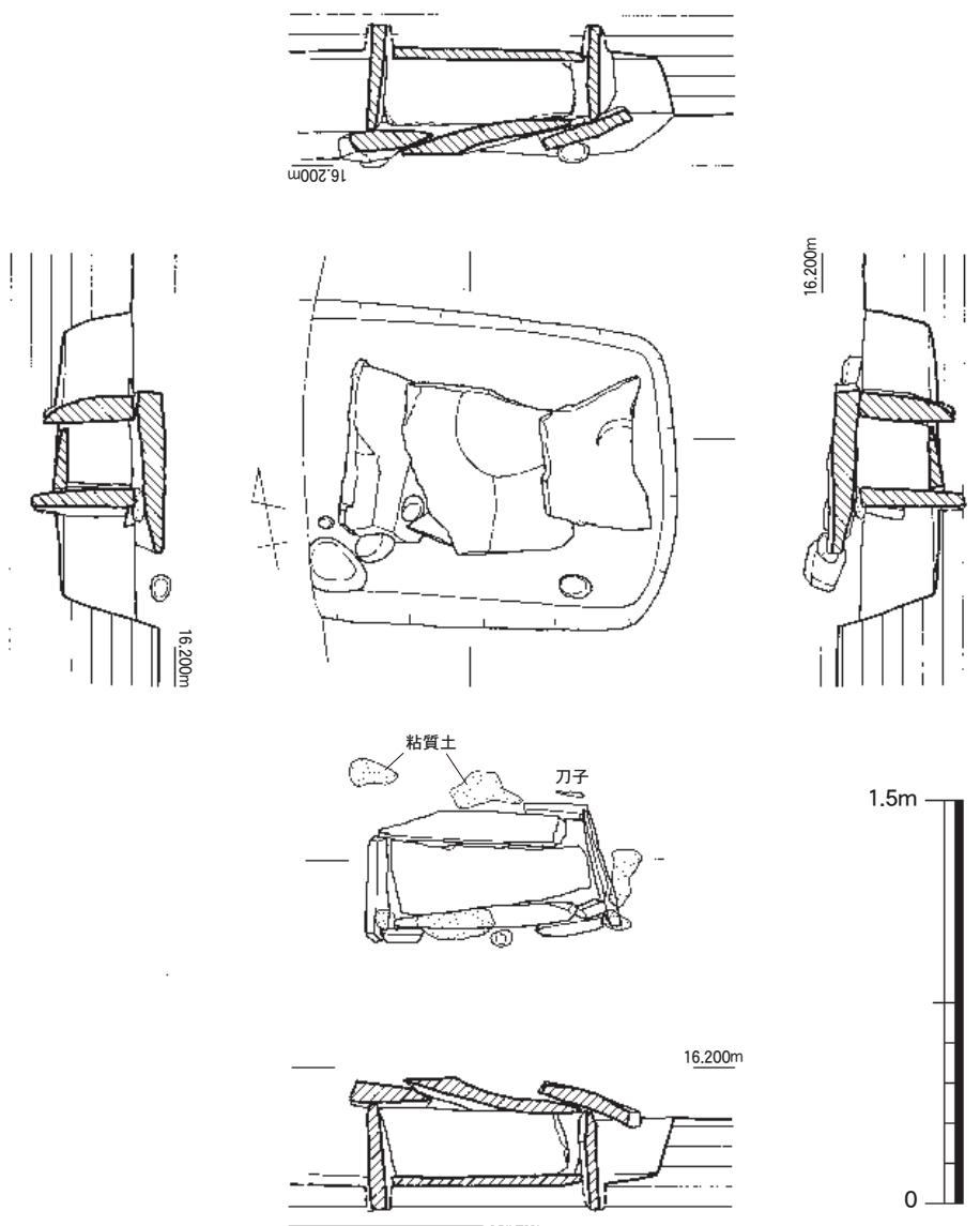
第9図 1号石棺墓実測図（縮尺1/30）
