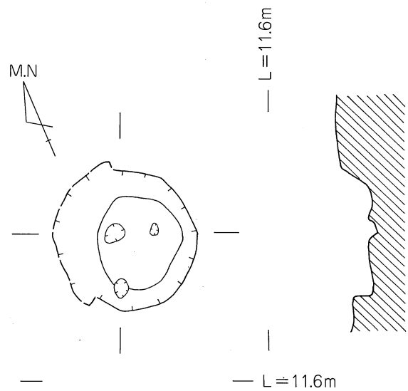
第107图 F区 SC 2 实测图
