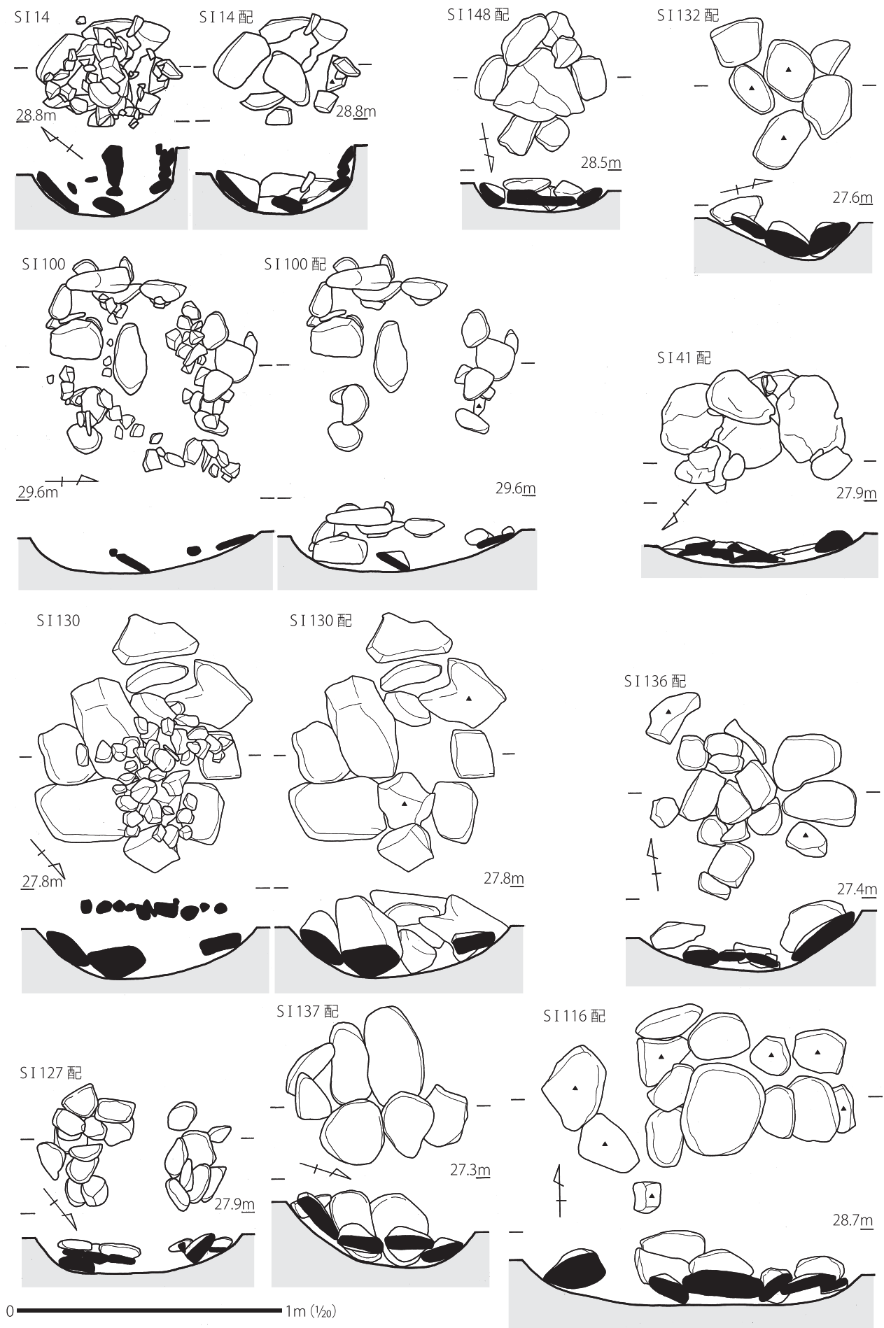
第38図 森ノ上遺跡集石遺構実測図 (15)
