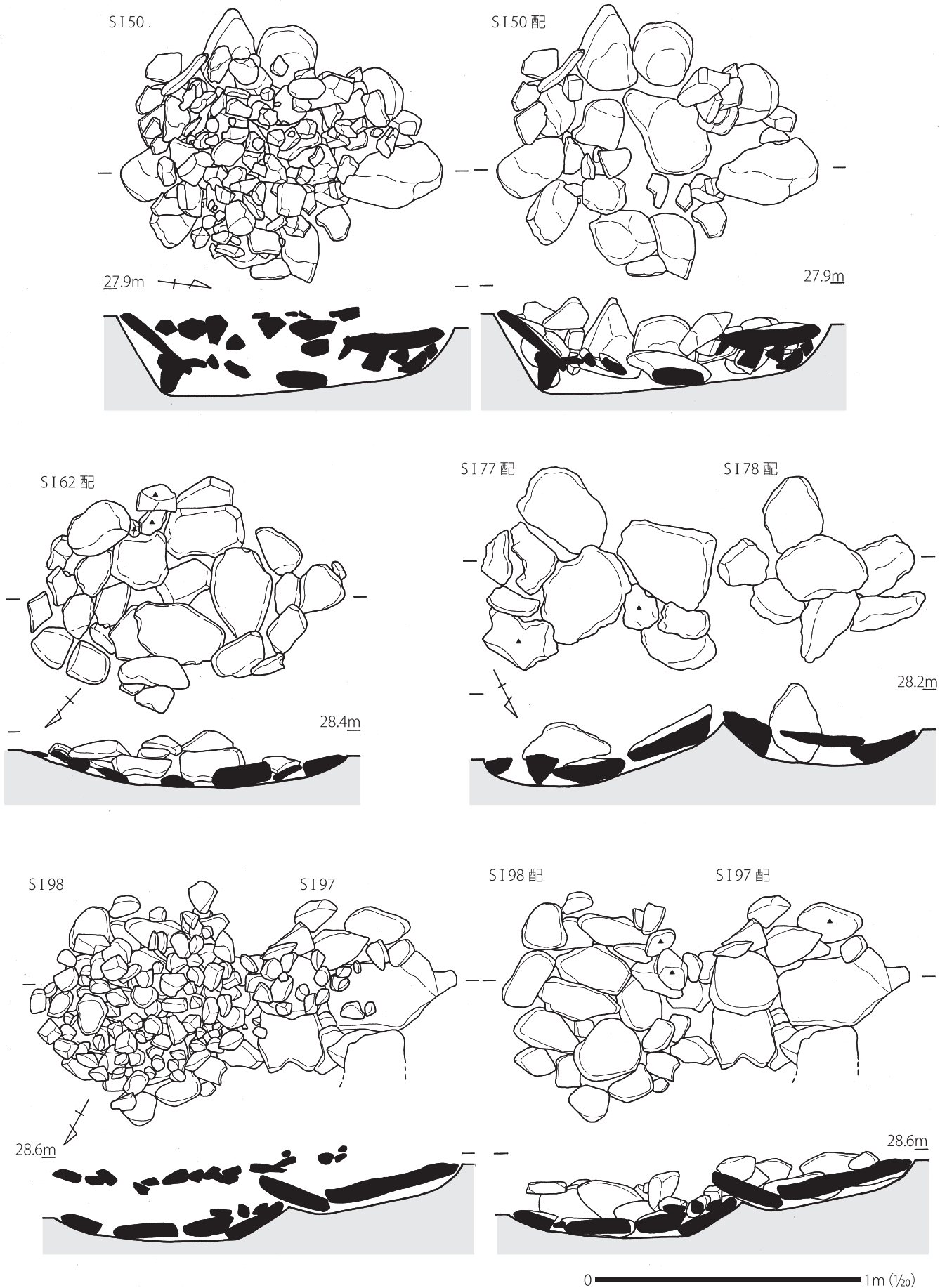
第34図 森ノ上遺跡集石遺構実測図 (11)
