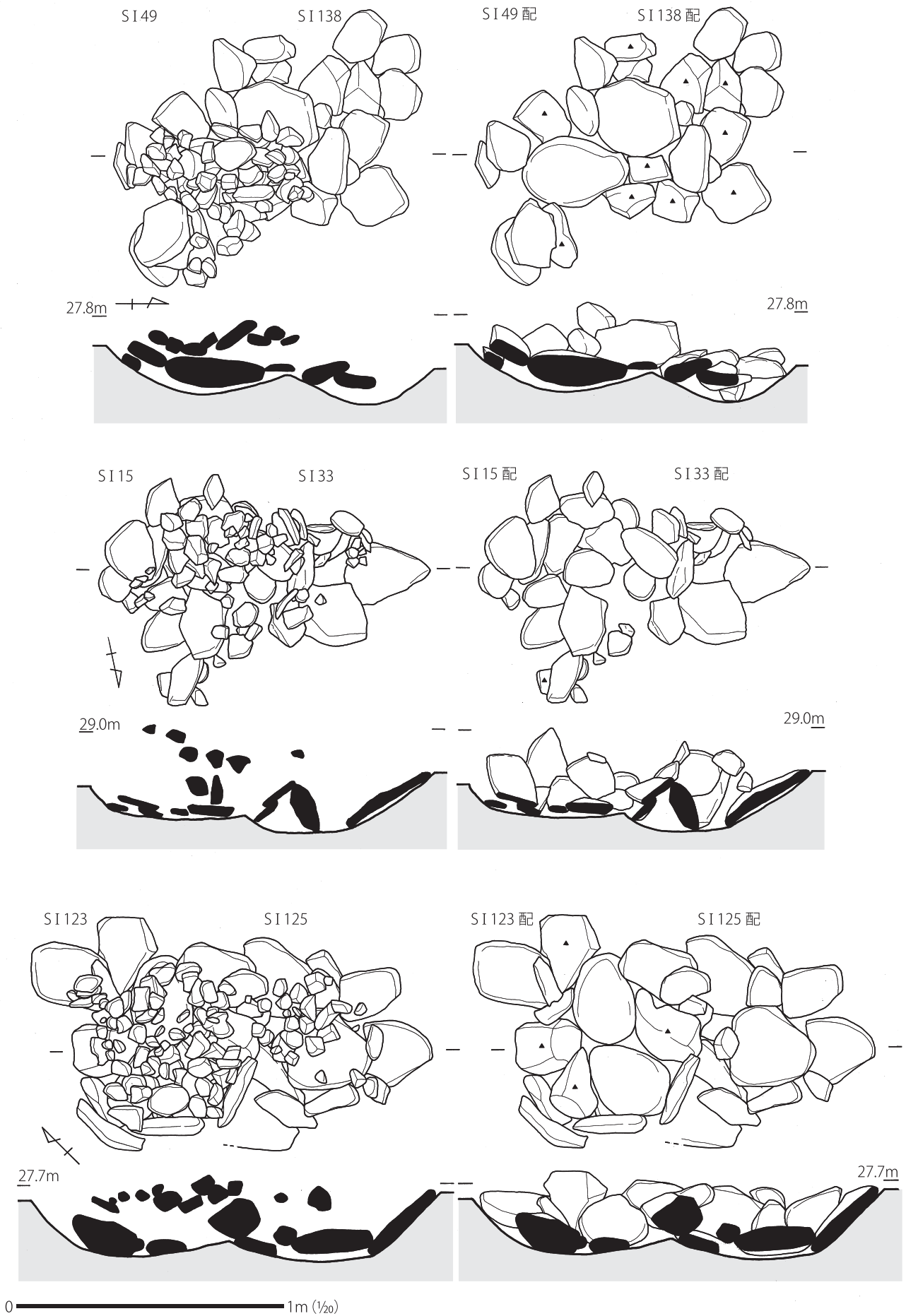
第35図 森ノ上遺跡集石遺構実測図 (12)
