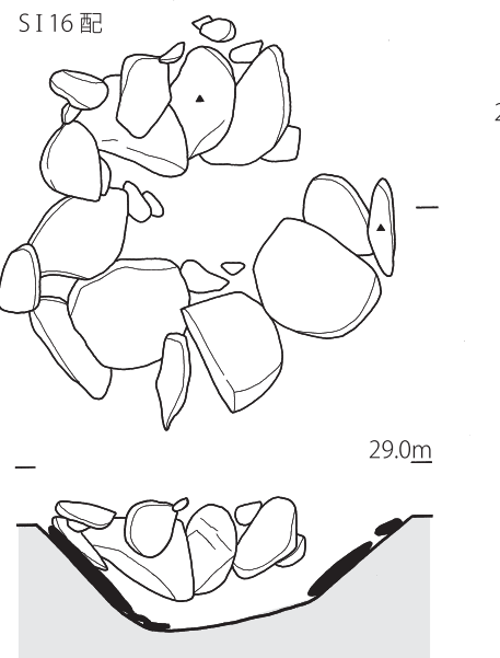
第36図 森ノ上遺跡集石遺構実測図 (13)
