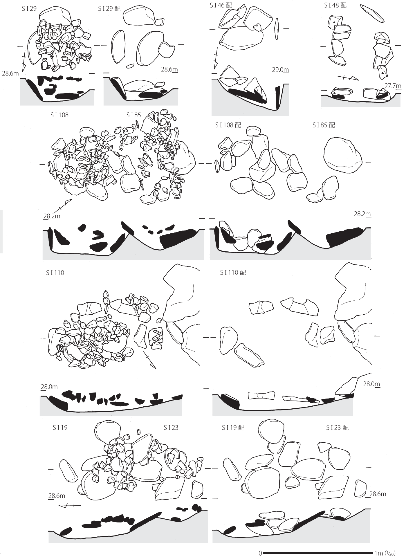
第41図 森ノ上遺跡集石遺構実測図 (18)
