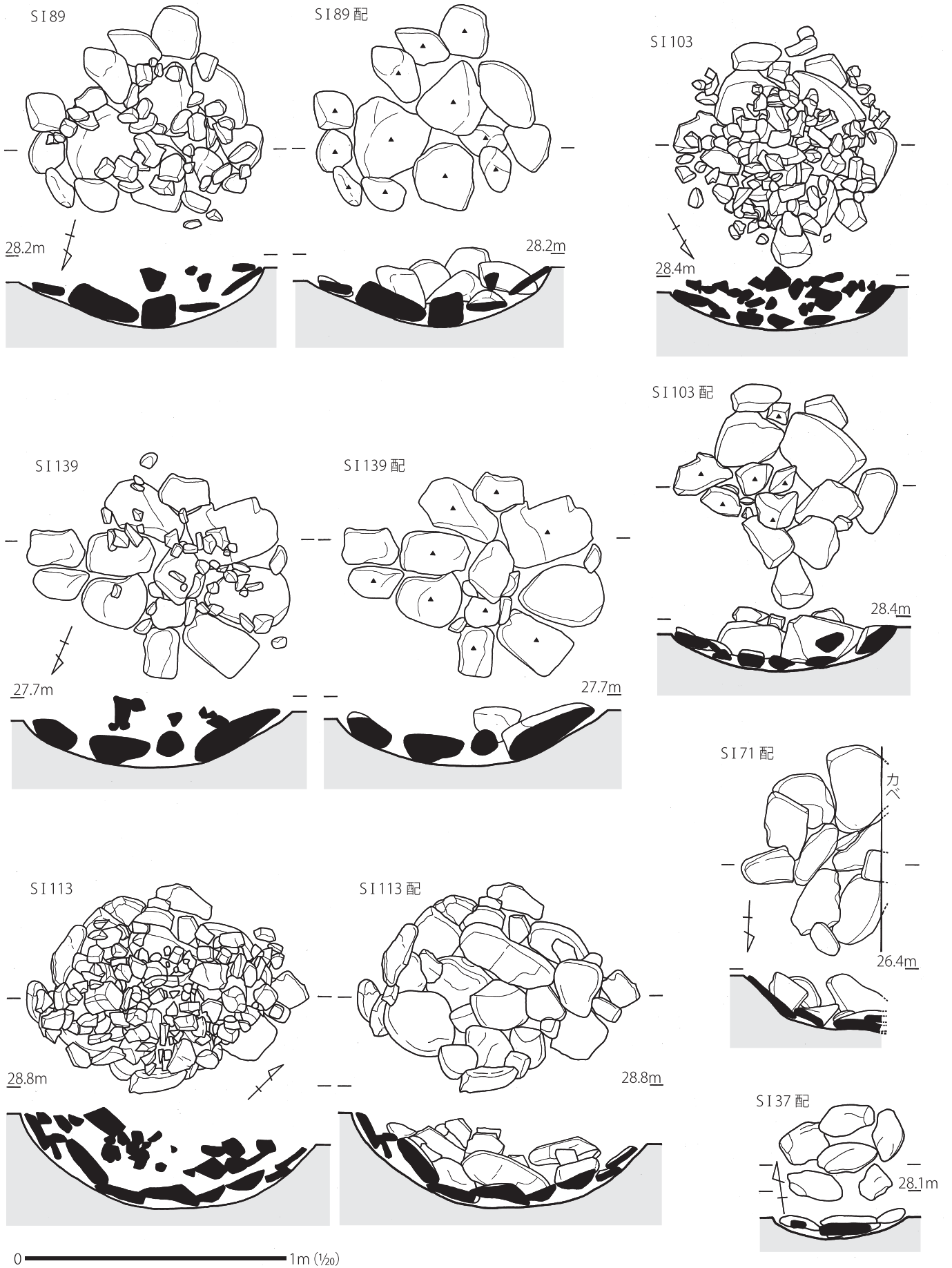
第33図 森ノ上遺跡集石遺構実測図 (10)
