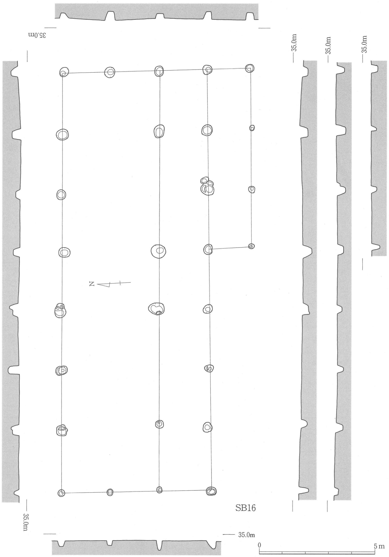
第94図 古代～中世掘立柱建物実測図⑩ (1/100)
