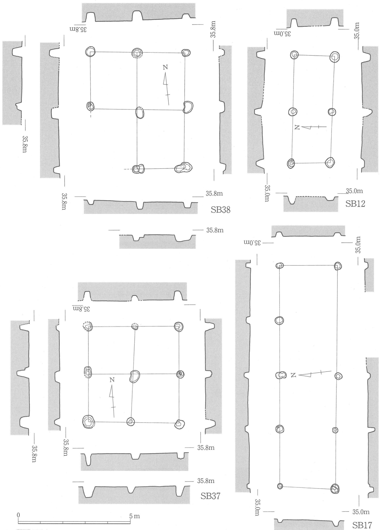
第91図 古代～中世掘立柱建物実測図⑦ (1/100)
