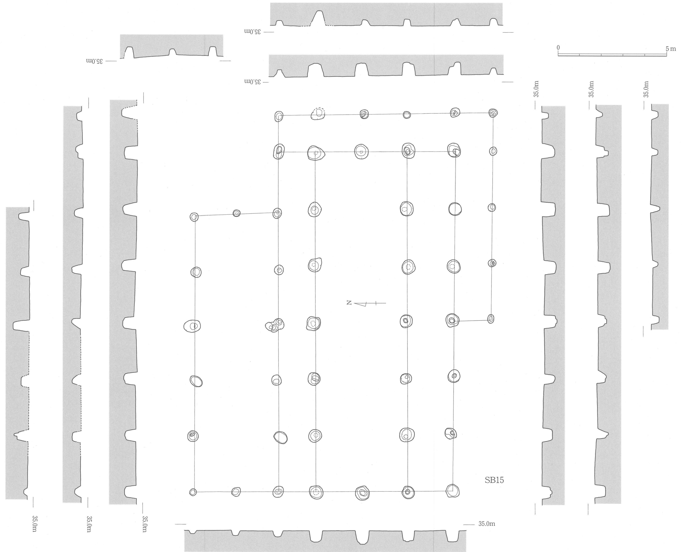
第93图 古代~中世掘立柱建物実測图⑨ (1/100)
