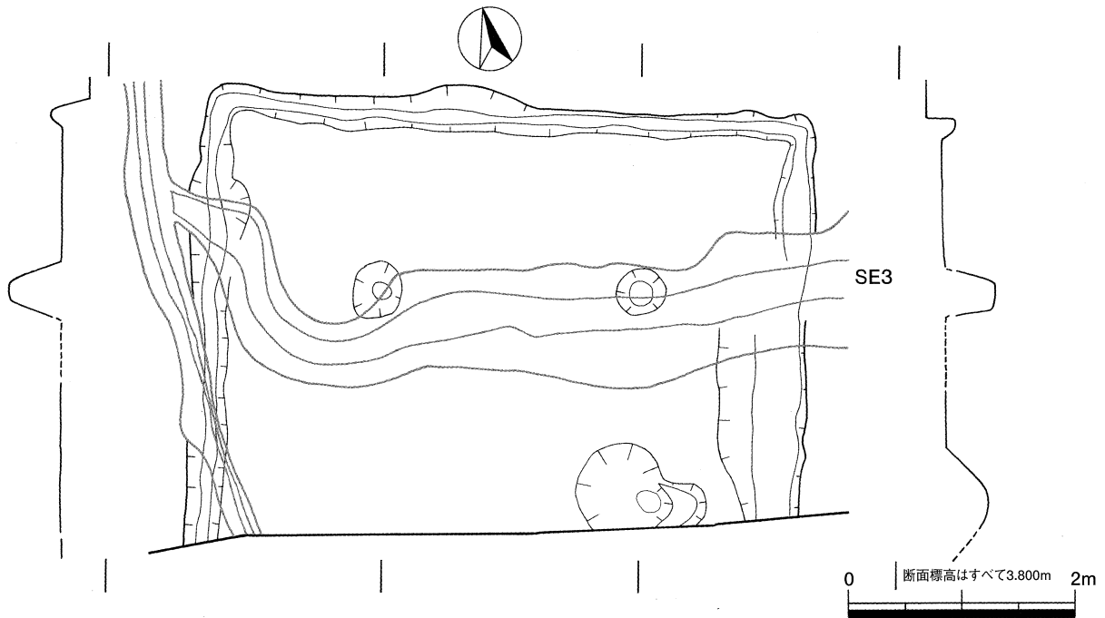
第14図 5号住居実測図
