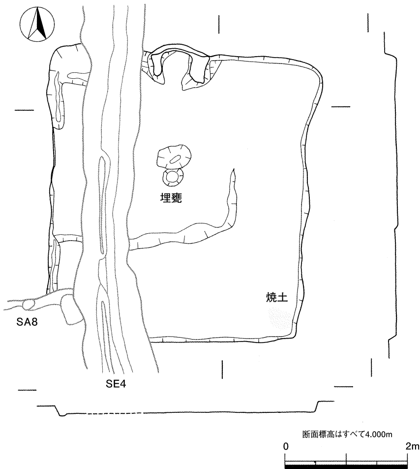
第16図 7号住居実測図
