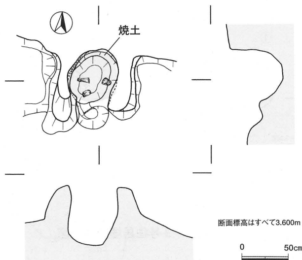
第12図 4号住居竈実測図
