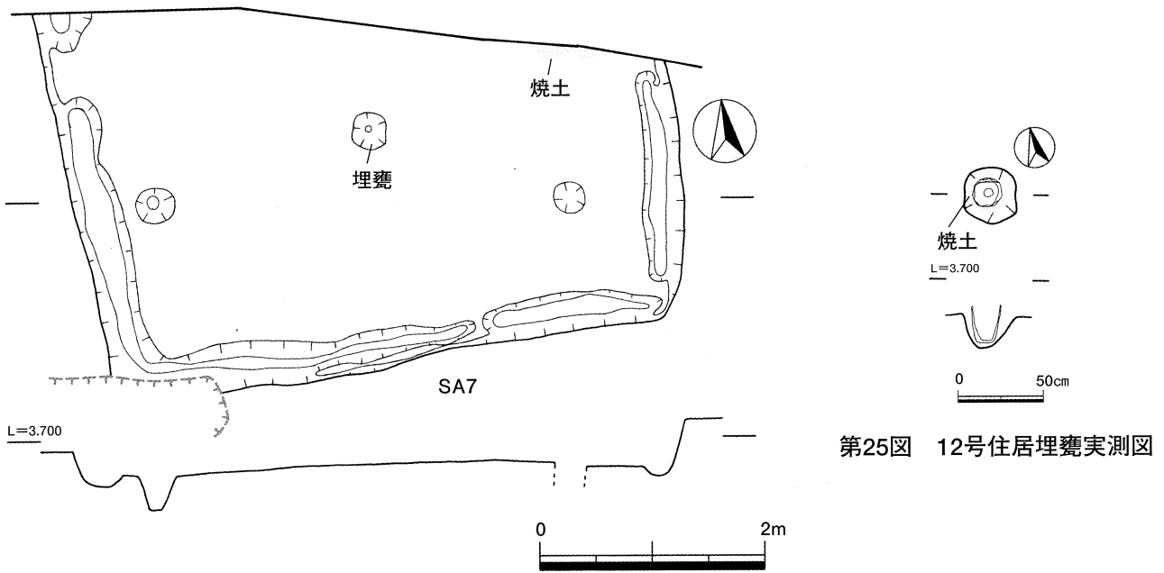
第24図 12号住居実測図
