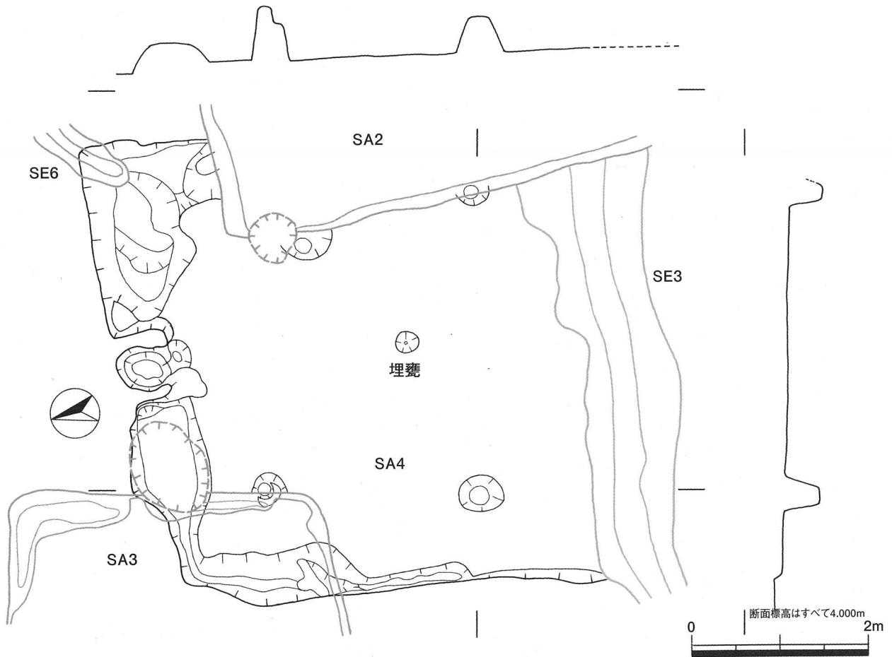
第11図 4号住居実測図
