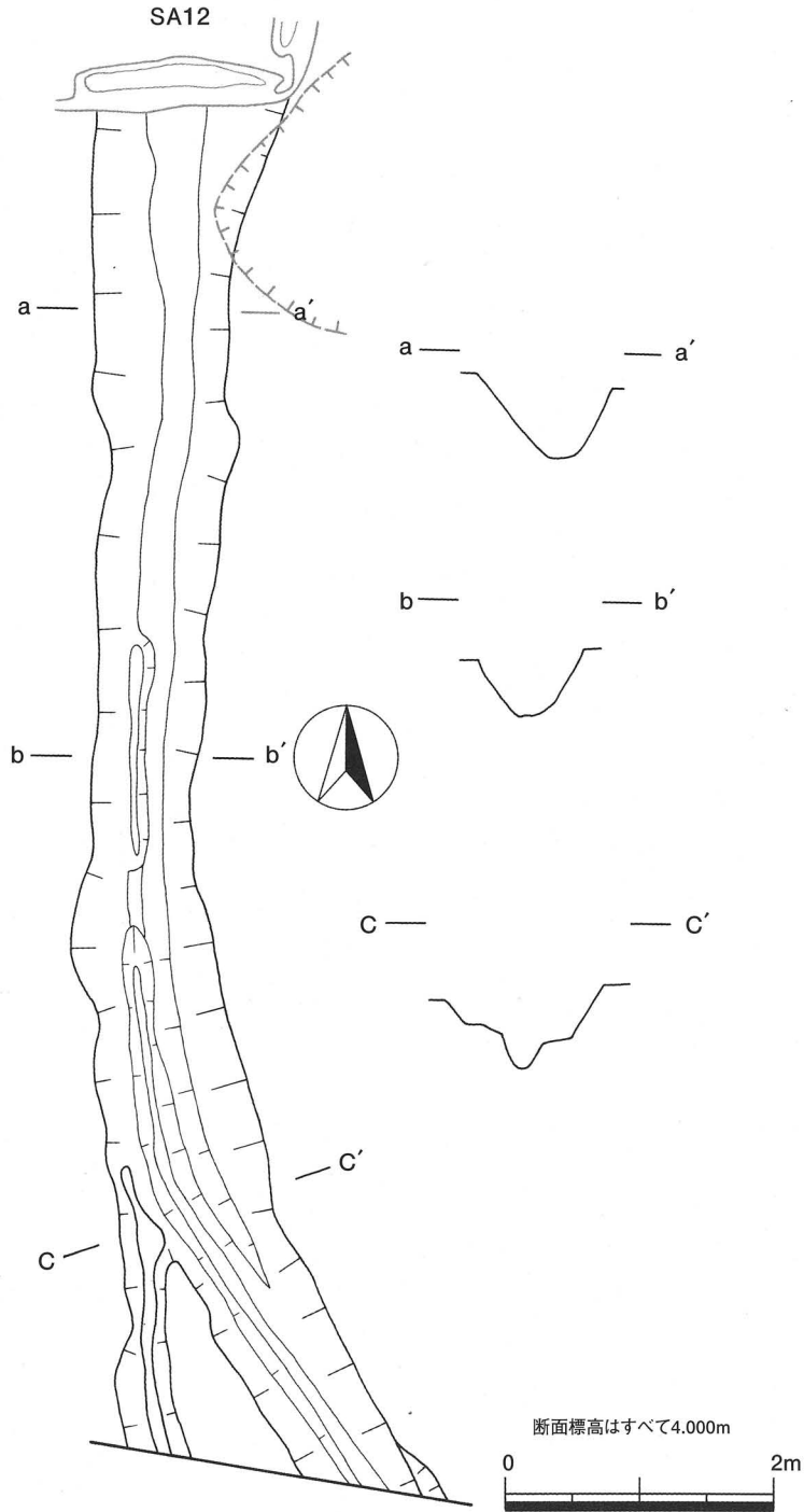
第37図 4号溝状遺構実測図
