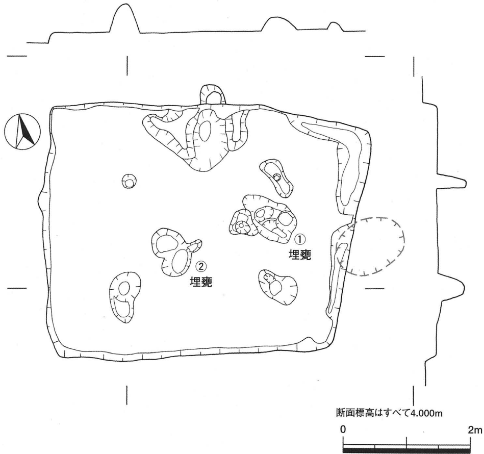
第8図 3号住居実測図
