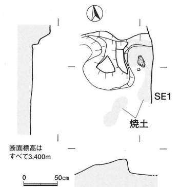
第6図 2号住居竈実測図
