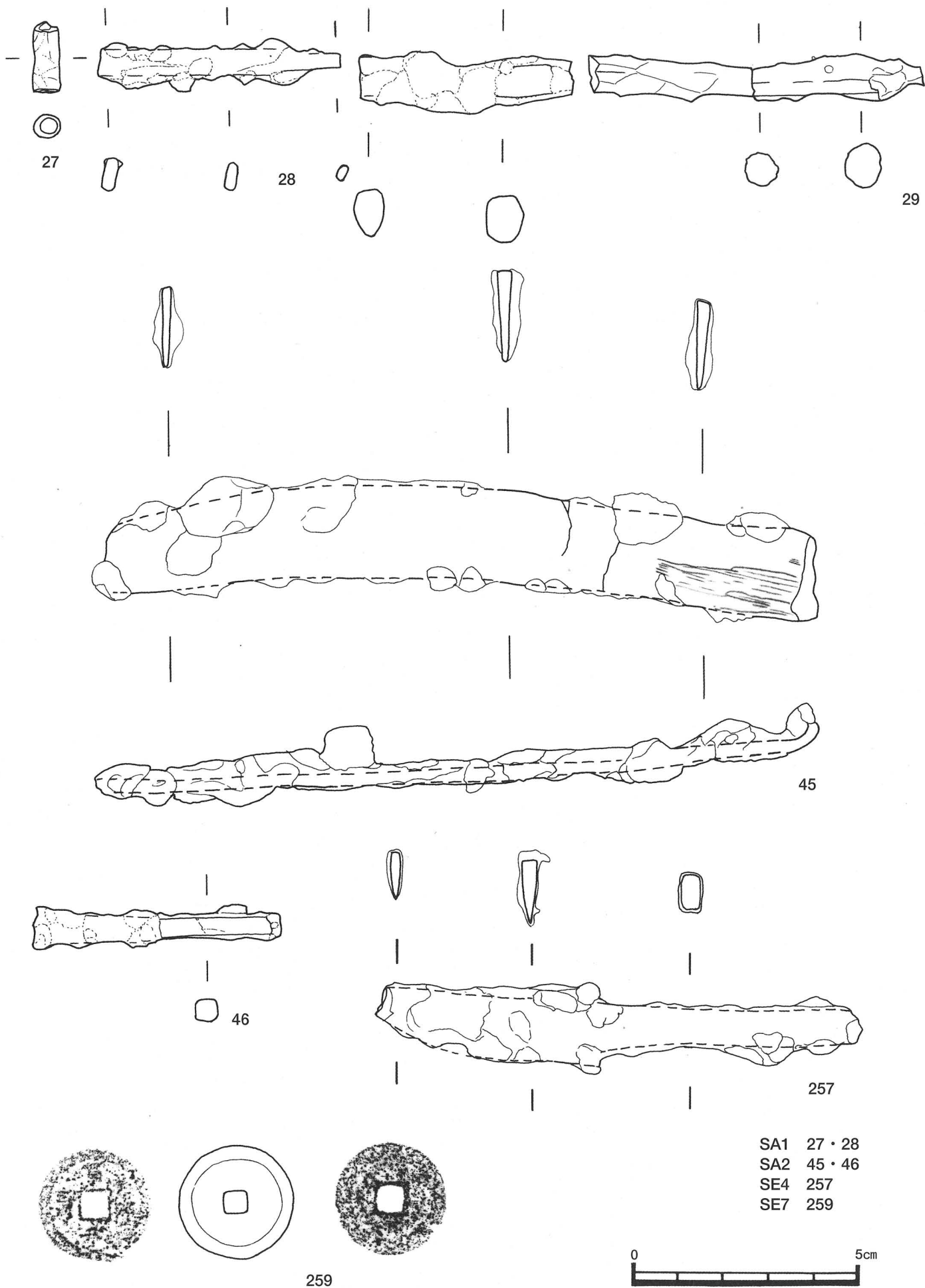
第47図 出土金属製品実測図
