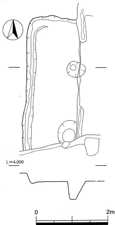
第26図 13号住居実測図
