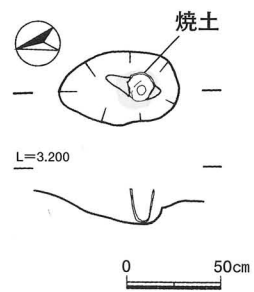
第7図 2号住居埋甕実測図
