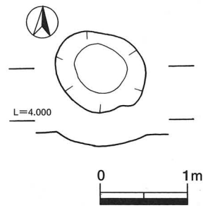
第34図 2号土坑実測図
