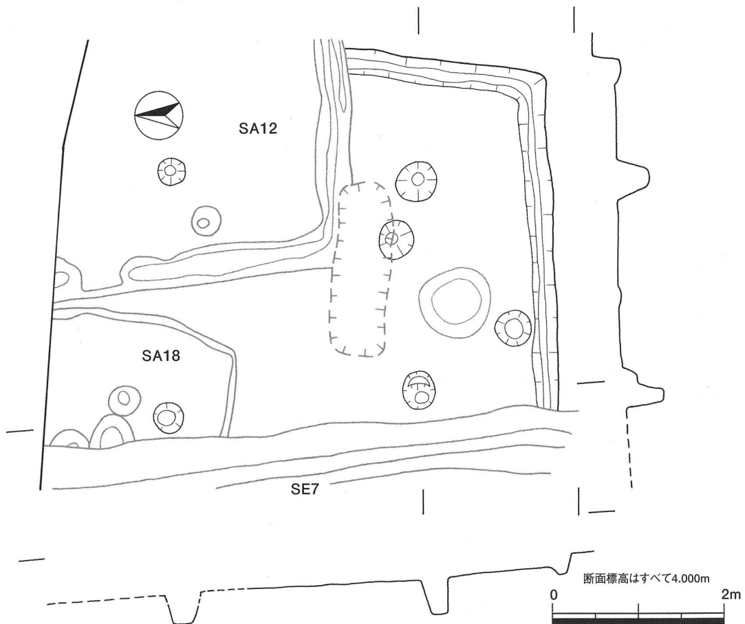
第31図 17号住居実測図
