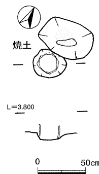
第18図 7号住居埋甕実測図
