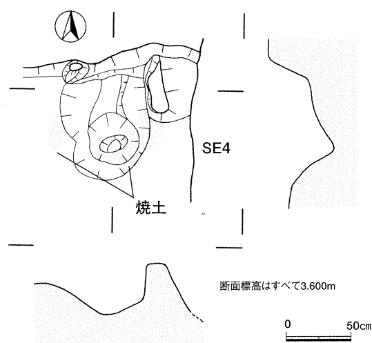
第20図 8号住居竈実測図
