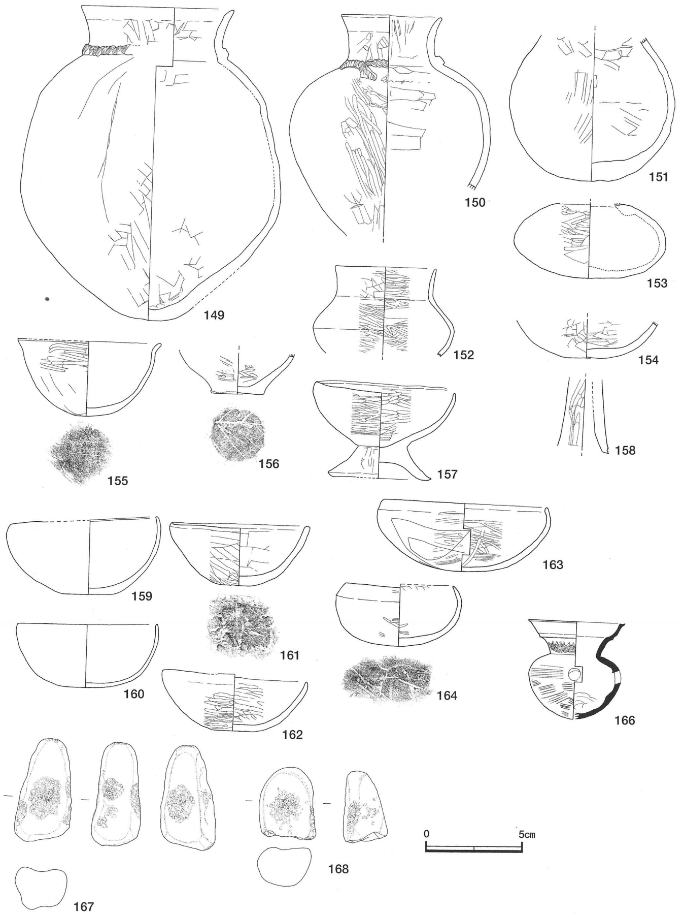
第44图 10号住居出土遺物実測図(2)
