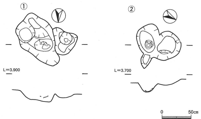
第10図 3号住居埋甕実測図
