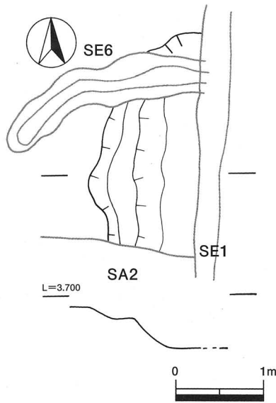
第33図 1号土坑実測図
