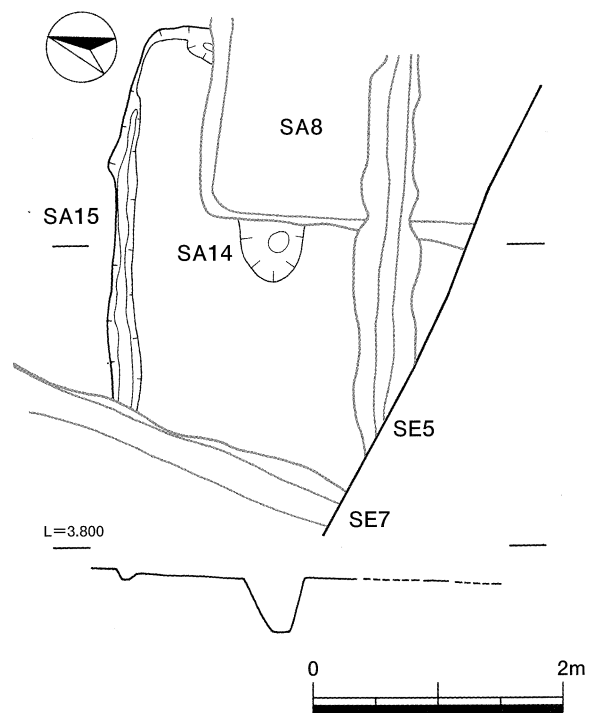
第27図 14号住居実測図
