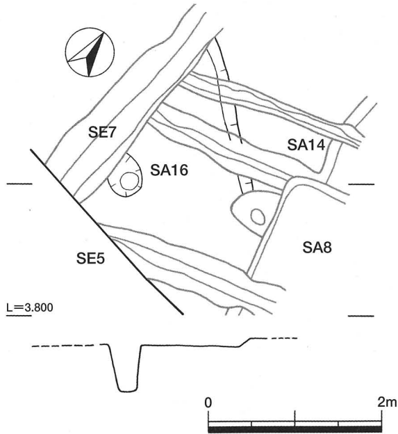
第30図 16号住居実測図
