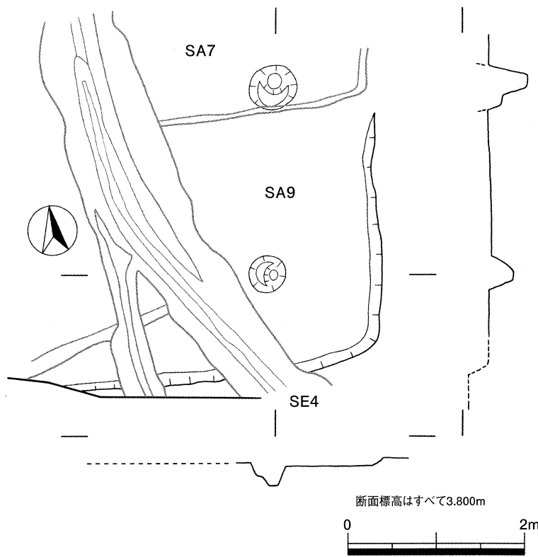
第21図 9号住居実測図
