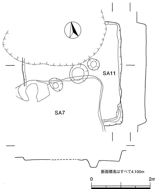
第23図 11号住居実測図
