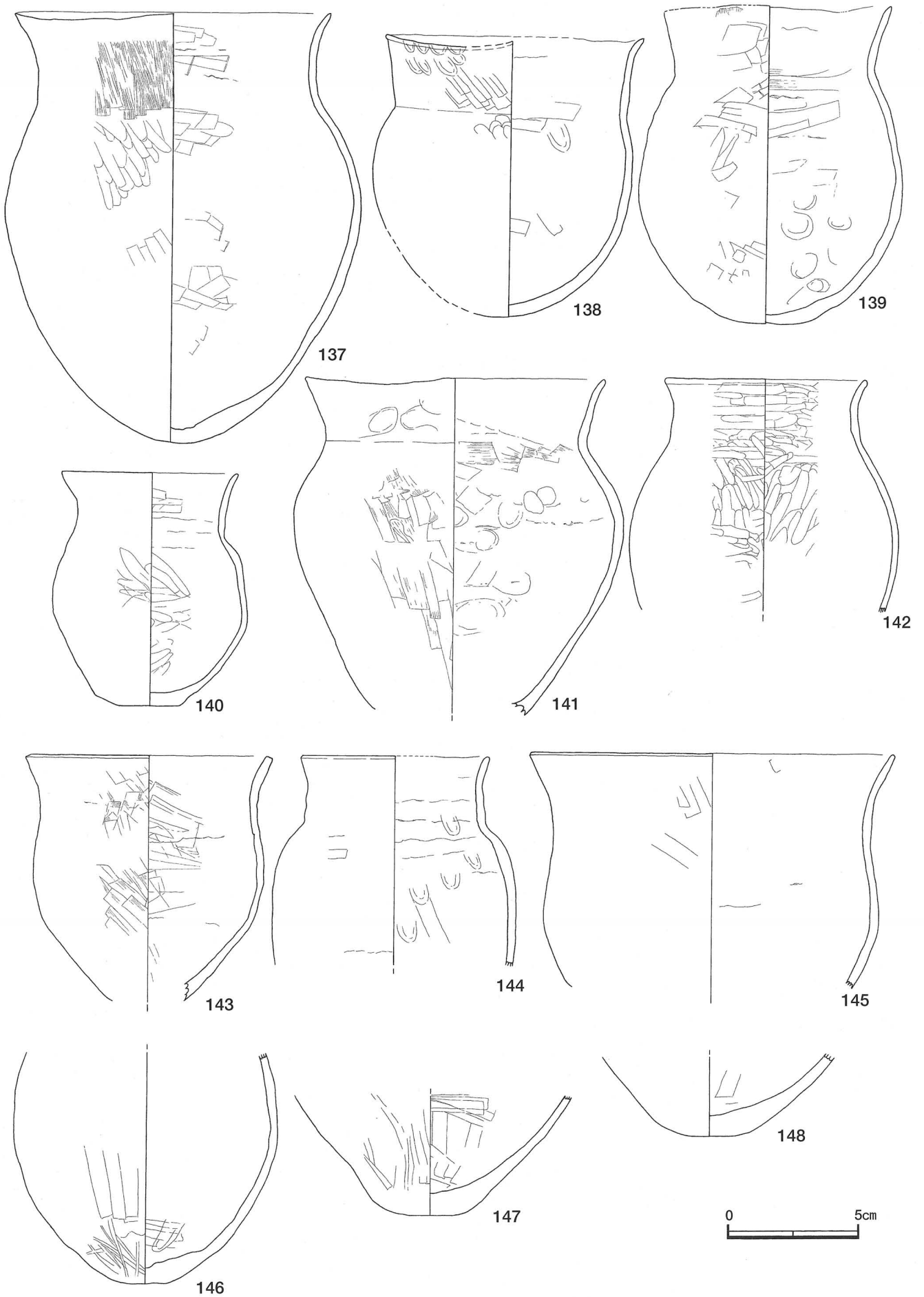
第43図 10号住居出土遺物実測図(1)
