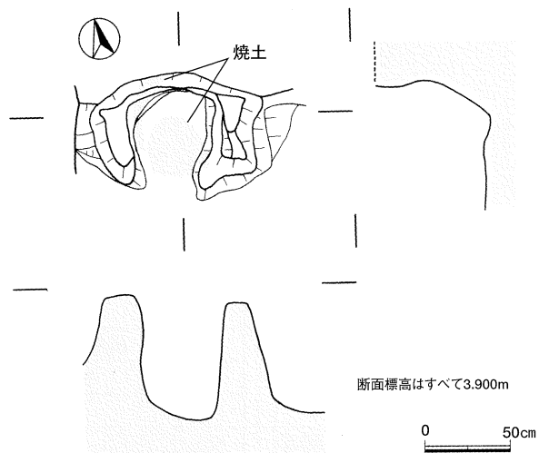
第17図 7号住居竈実測図
