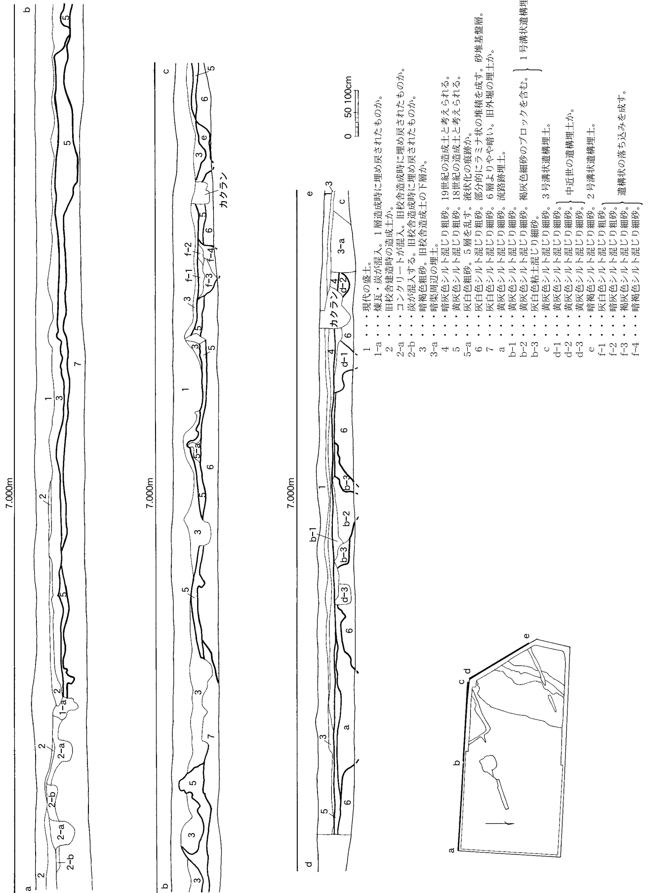
第4図 高鍋城三ノ丸跡 土層図 (1:80)
