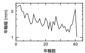
図2 高鍋城三ノ丸出土材(サンプルA)の年輪幅変動
