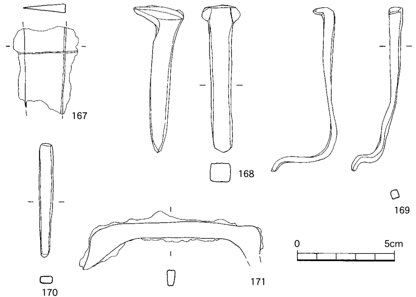
第42図 包含層出土の遺物【鉄製品】 (1:2)
