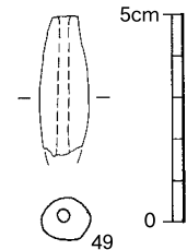
第23図 2号溝状遺構出土遺物【土錘】(1:2)
