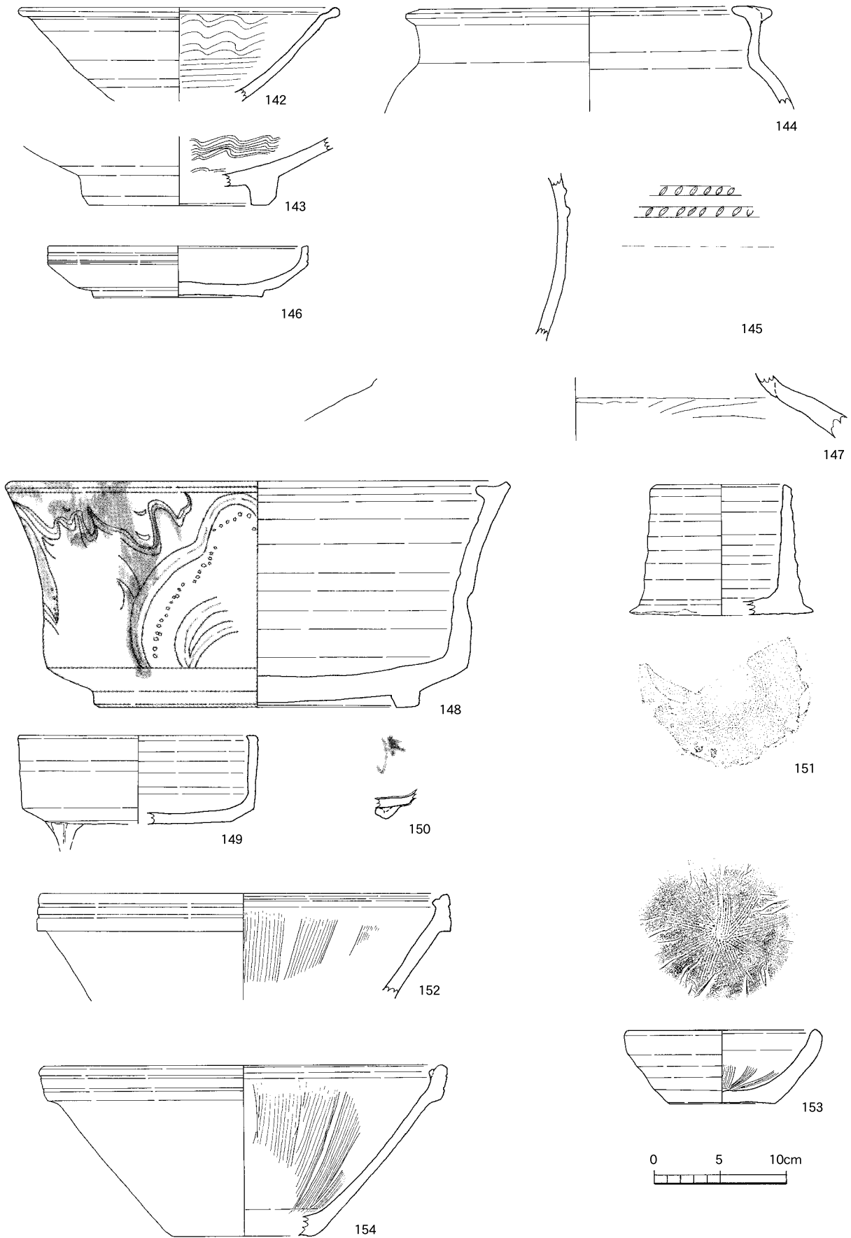
第39図 包含層出土の遺物【陶磁器類③】（1：4）
