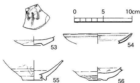
第26図 3号溝状遺構出土遺物【陶磁器類】(1:4)
