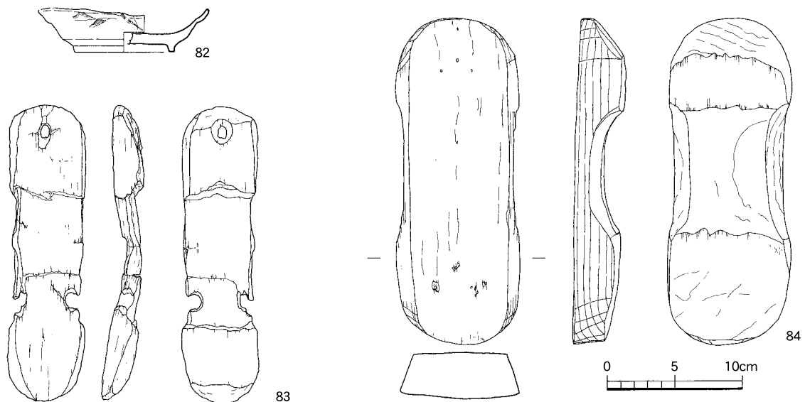
第33図 土坑出土遺物【漆器・下駄】（1：4）
