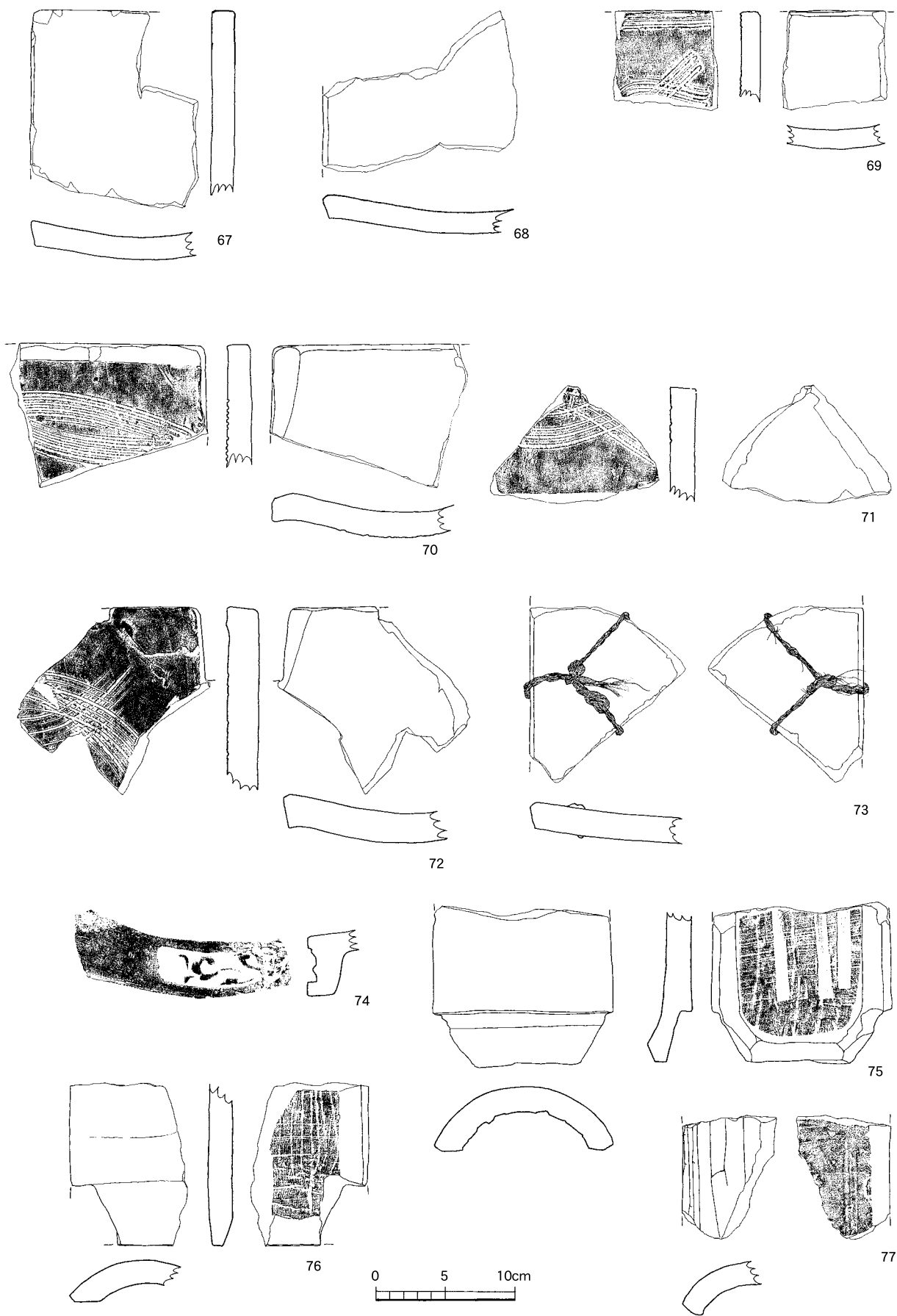
第31図 土坑出土遺物【平瓦・軒平瓦・丸瓦】（1：4）
