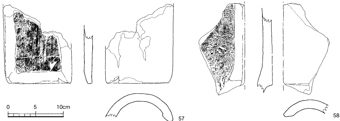
第27図 3号溝状遺構出土遺物【瓦】(1:4)
