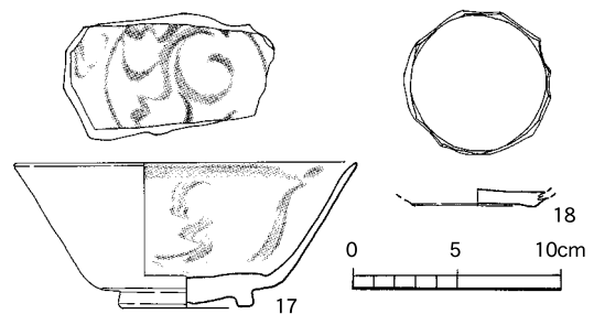
第10図 流路跡出土遺物【輸入陶磁器類】（1：4）
