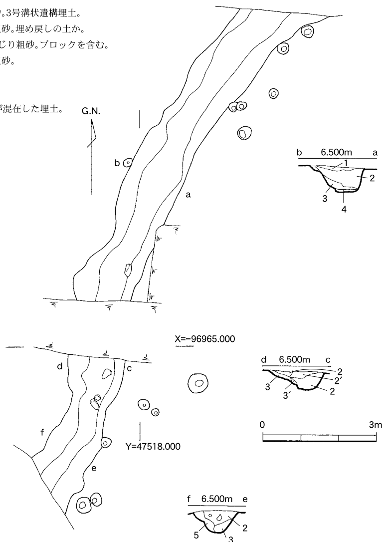
第13図 1号溝状遺構実測図（1：100）
