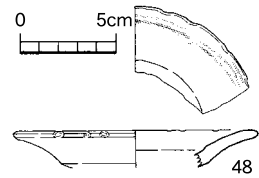
第22図 2号溝状遺構出土遺物【青磁】(1:4)
