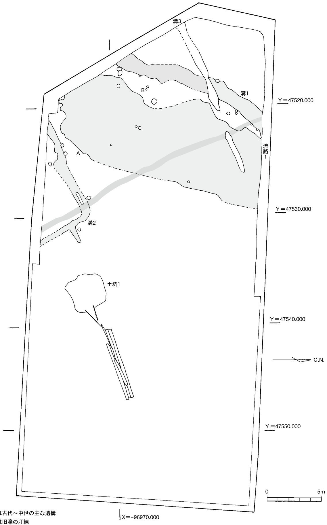
第3図 高鍋城三ノ丸跡 遺構分布図 (1 : 200)
