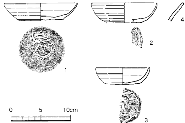
第6図 流路跡出土遺物【土師器坏類】（1：4）
