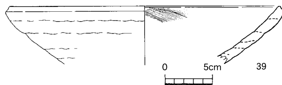
第17図 1号溝状遺構出土遺物【瓦質焼成土器】(1:4)
