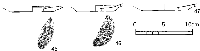
第21図 2号溝状遺構出土遺物【土師器】（1：4）
