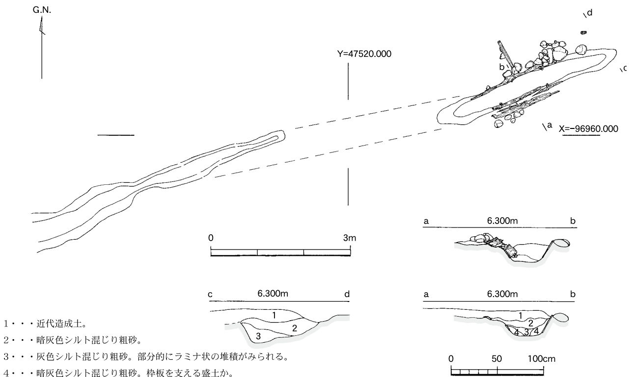
第24図 3号溝状遺構実測図(平面図1:80 土層断面・立面図1:40)
