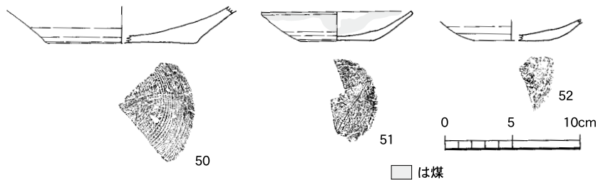
第25図 3号溝状遺構出土遺物【土師器】(1:4)
