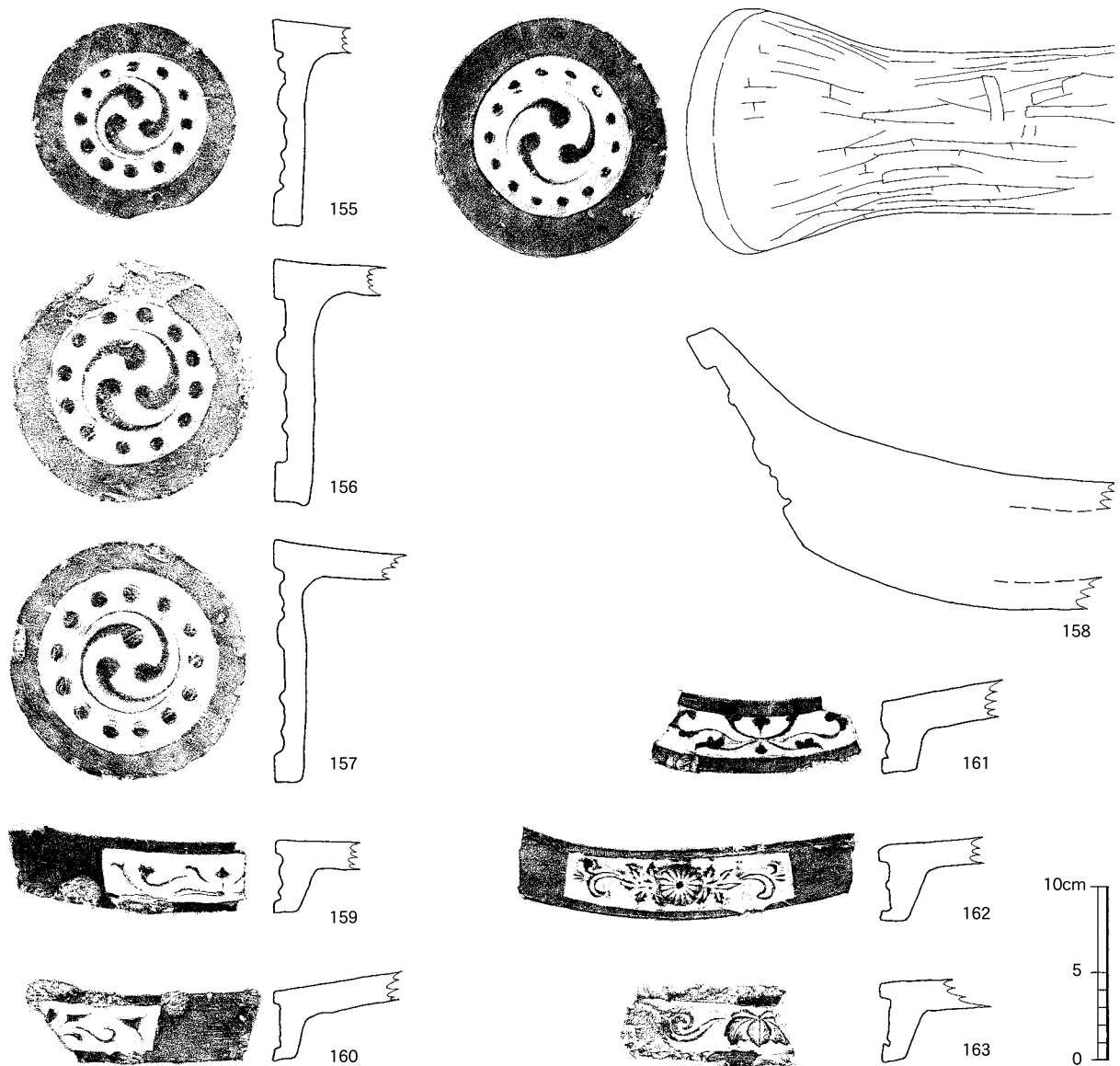
第40図 包含層出土の遺物【瓦】 (1:4)
