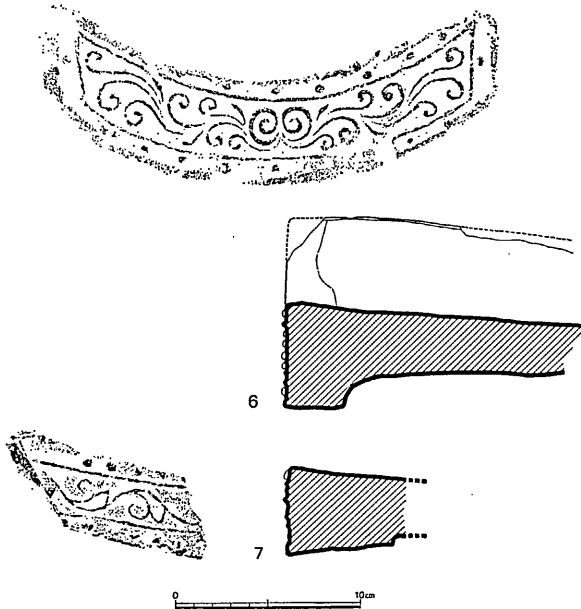
第13図 軒平瓦拓影・実測図(Ⅰ)
