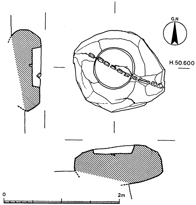
第7図 塔心礎実測図
