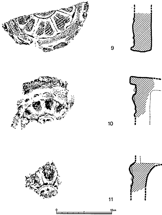
第12図 軒丸瓦拓影・実測図(Ⅲ)
