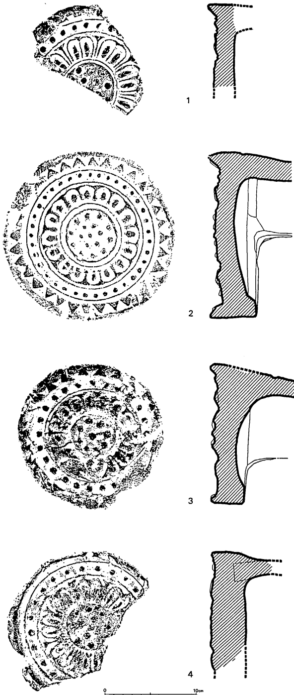
第10図 軒丸瓦拓影・実測図 (I)
