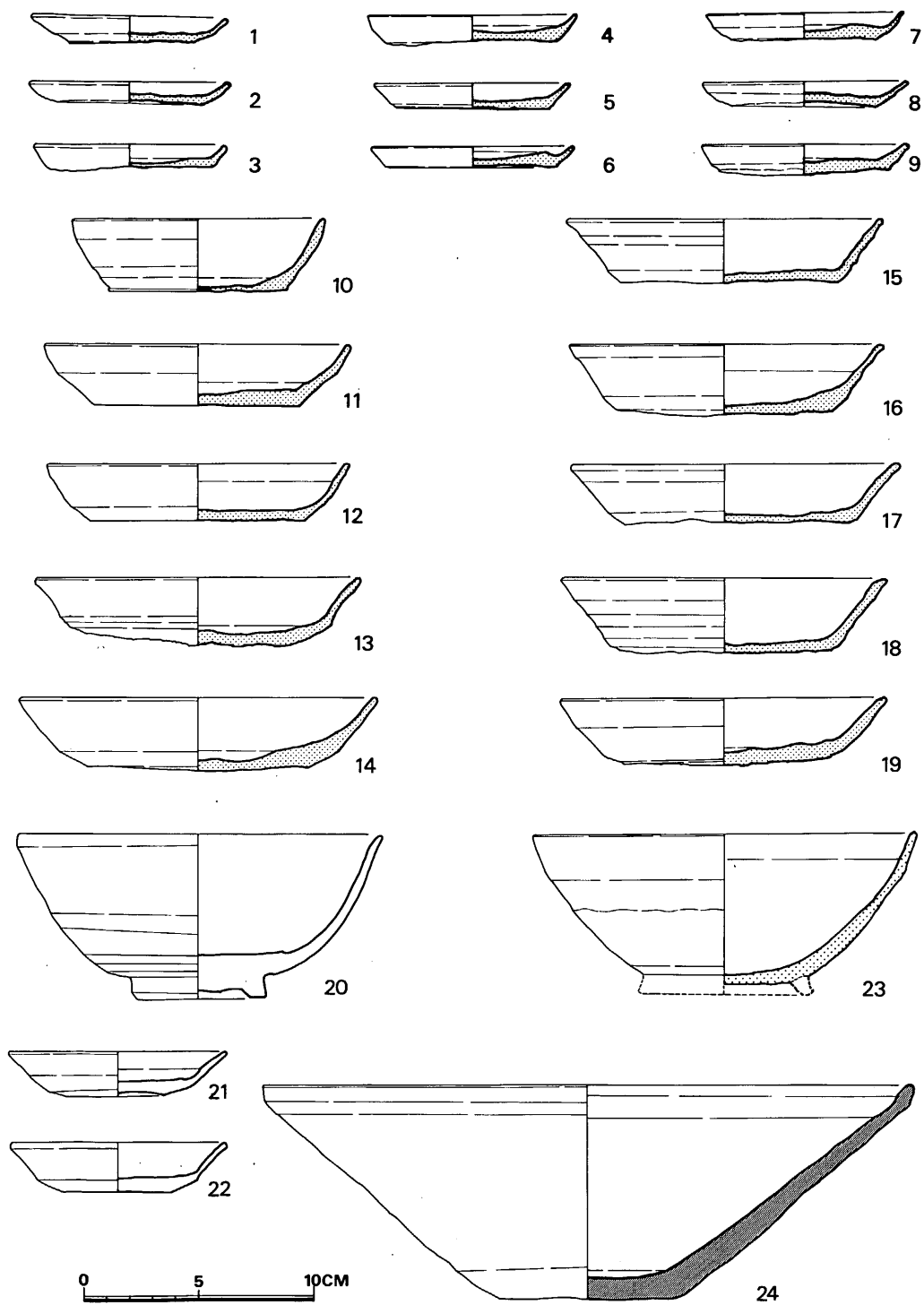
第7図 第33次発掘調査出土土器実測図
