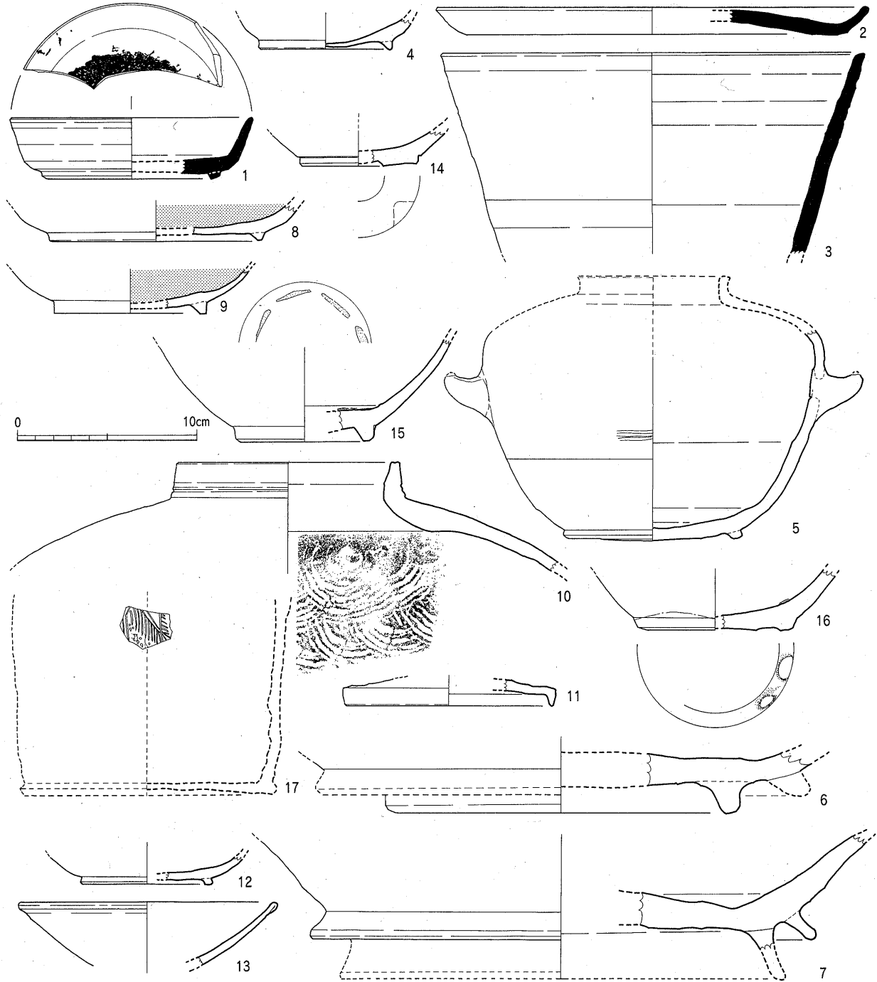
Fig.51 黄灰色土出土土器実測図 (1/3)
