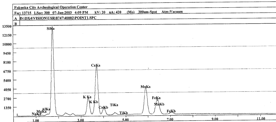
Fig.56 鴻臚館出土ガラス(緑色)K-1の分析結果
