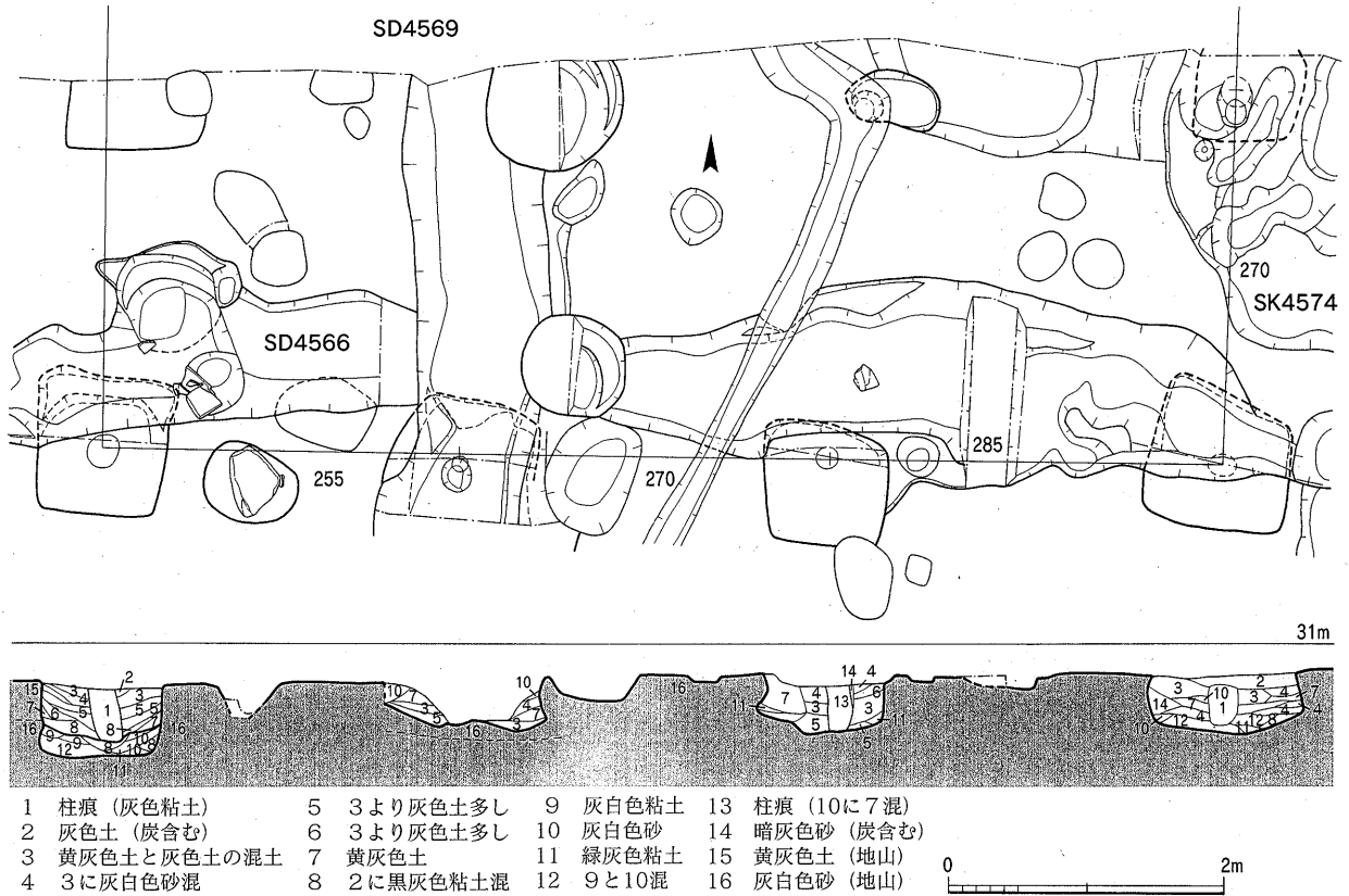
Fig.20 SB4561実測図 (1/60)
