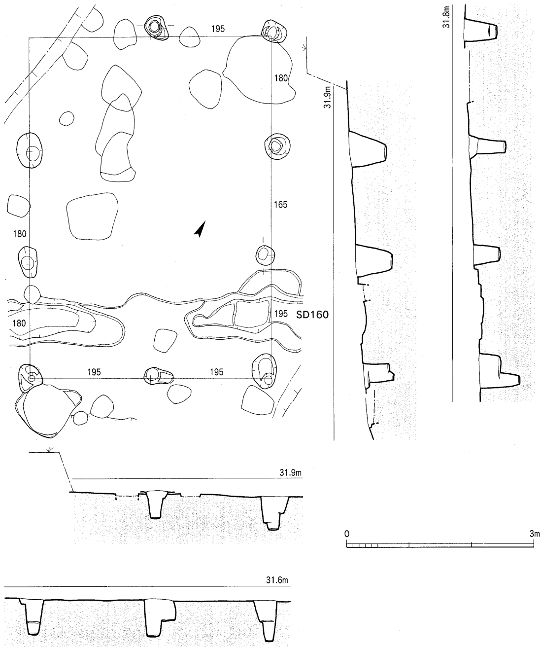
Fig.71 SB144実測図 (1/60)
