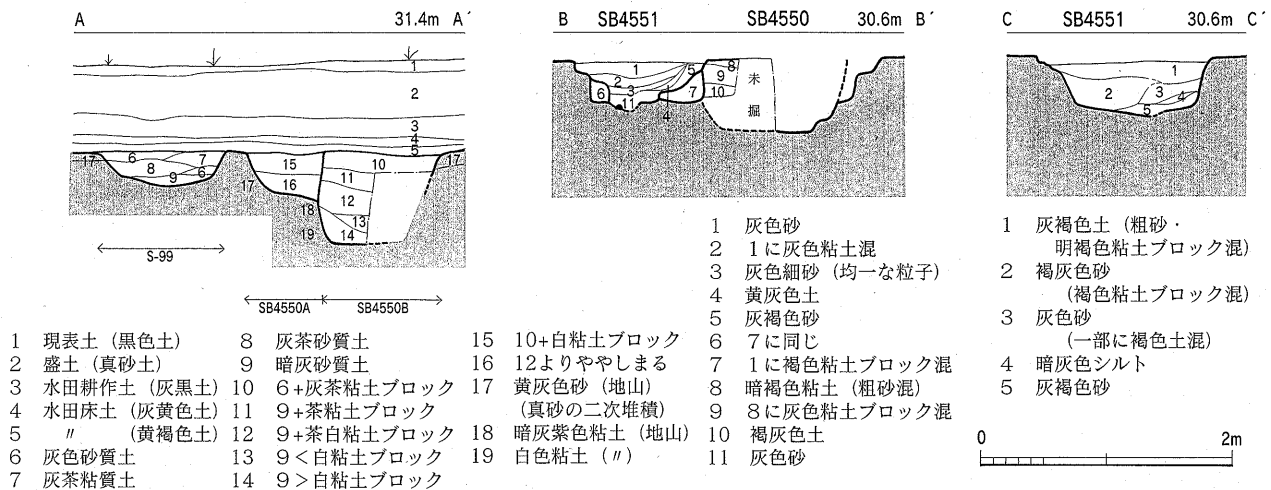
Fig. 7 SB4550・4551柱穴断面実測図 (1/60)
