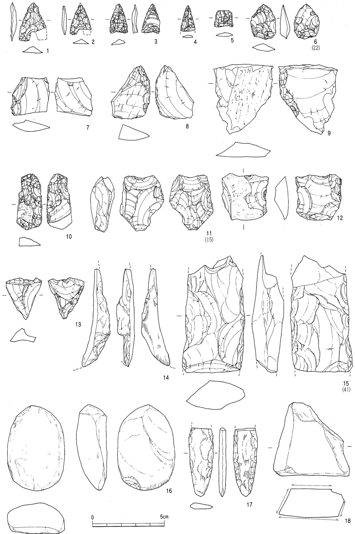
Fig.94 縄文時代以降の石器実測図 (2/3)
