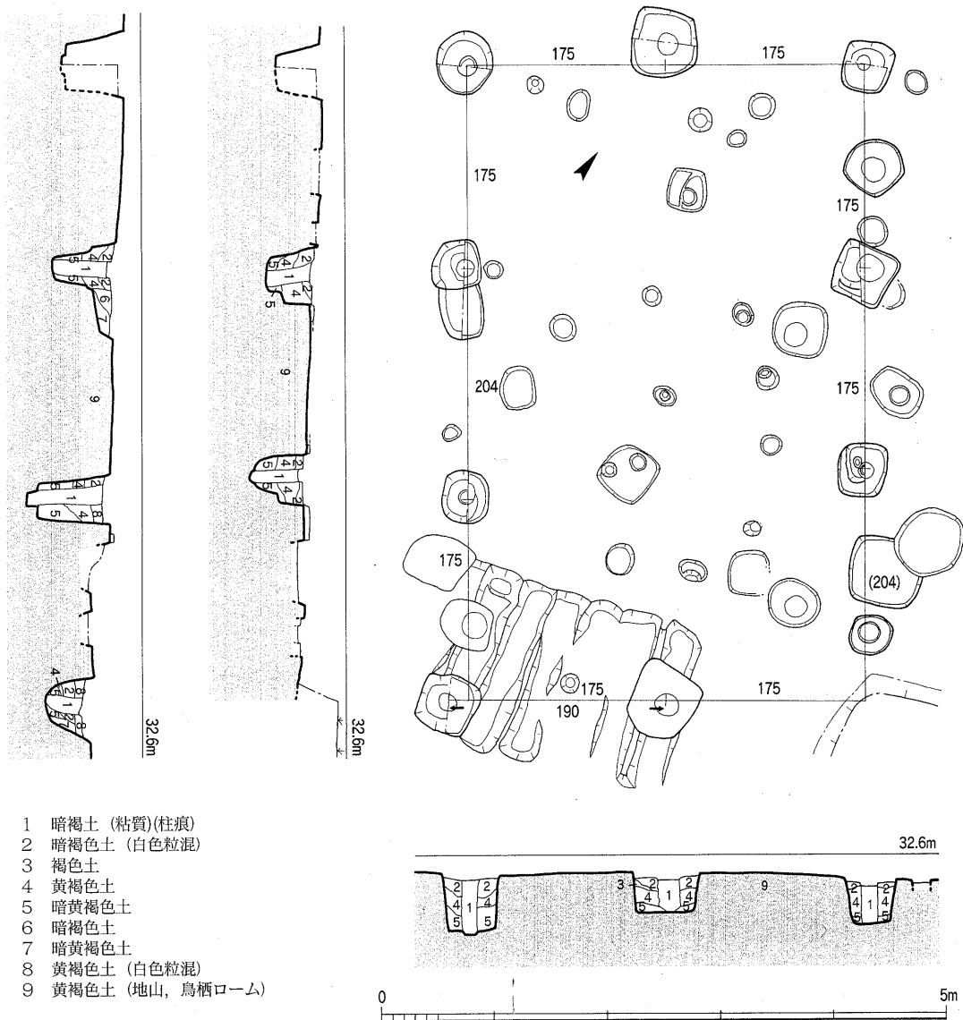
Fig.67 SB141実測図 (1/60)
