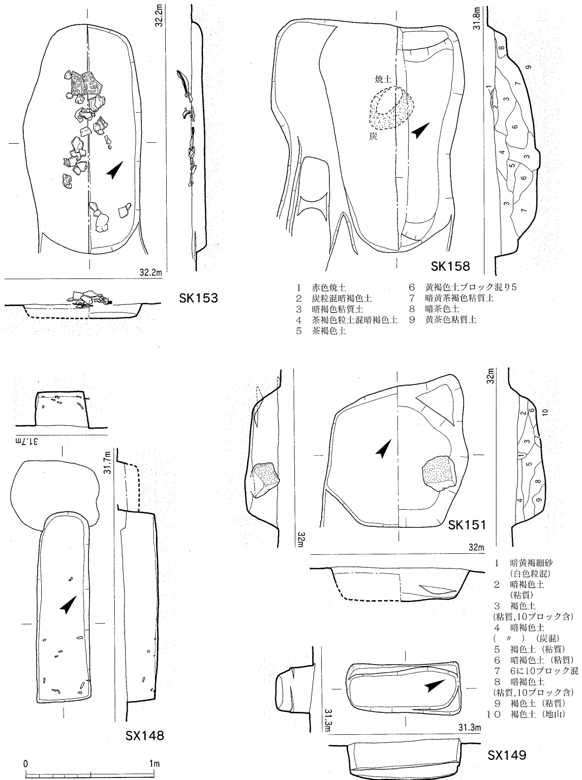
Fig.75 SK151~158, SX148・149実測図 (1/30)
