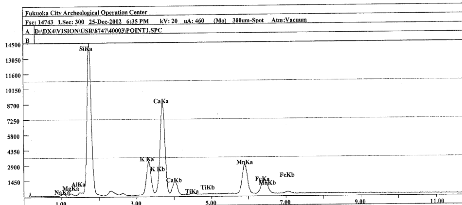
Fig.57 鴻臚館出土ガラス(透明)K-2の分析結果
