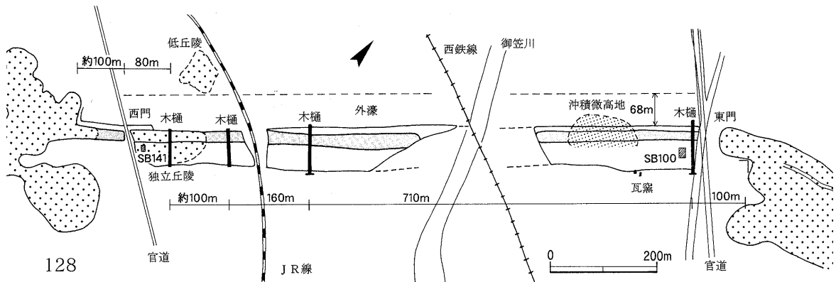
Fig.96 水城全体概念図 (1/10,000)
