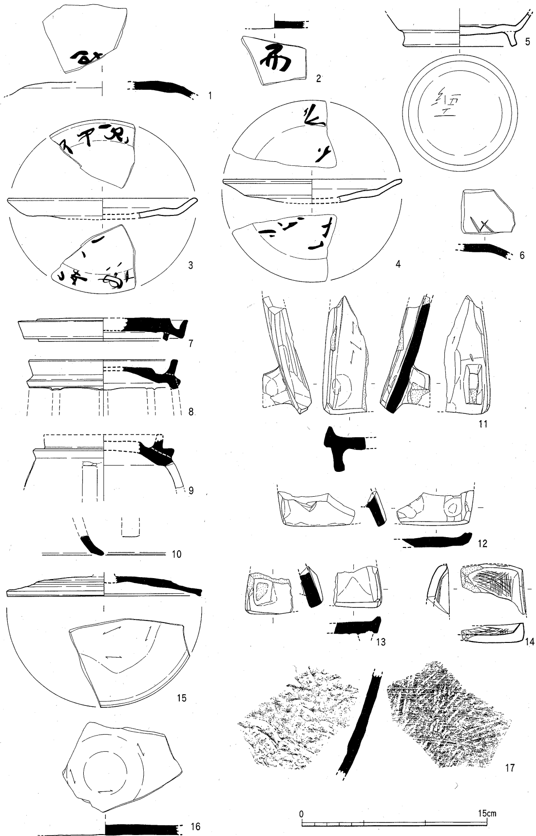
Fig.52 墨書土器・碗等実測図 (1/3)
