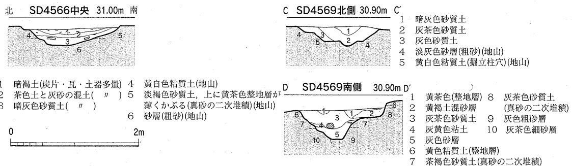
Fig.22 SD4566・4569土層断面実測図 (1/60)
