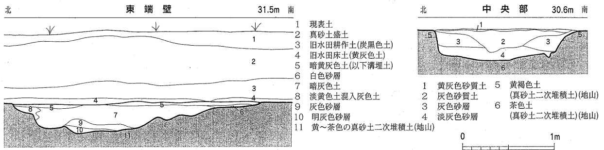
Fig.12 SD4542土層実測図 (1/40)
