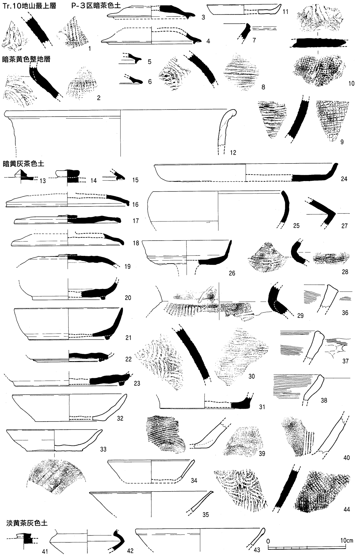
Fig.84 各整地層出土土器実測図 (1/3)
