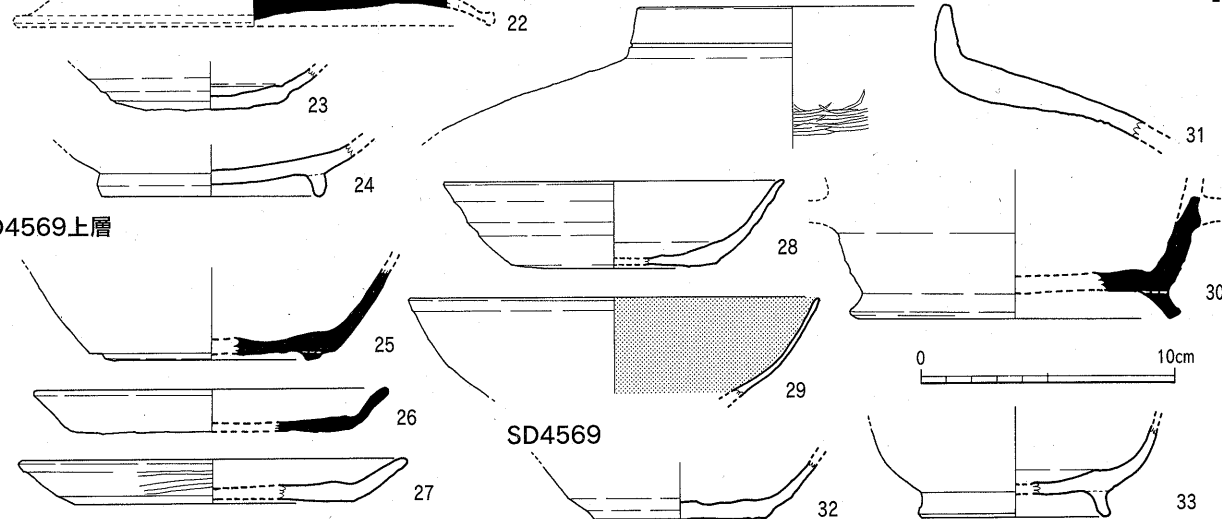
Fig.45 SD4567~4569出土土器実測図 (1/3)
