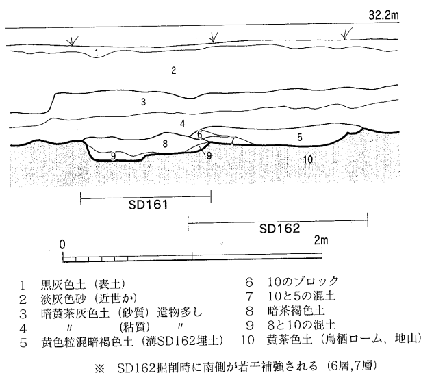
Fig.79 SD161・162土層断面実測図 (1/40)
