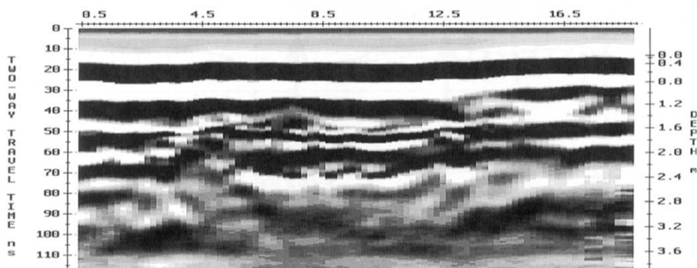
Fig.113 C1異常部の地中レーダープロフィール
