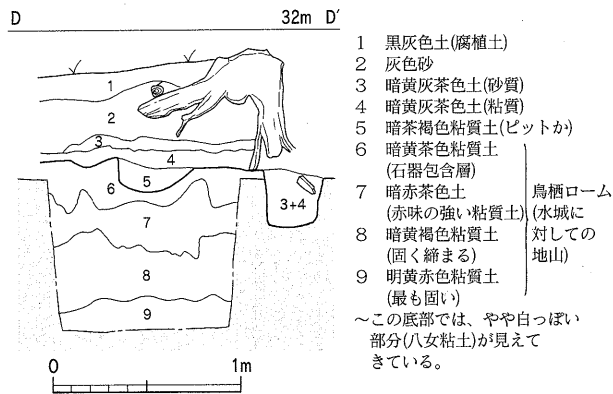
Fig.88 深掘り部土層実測図 (1/40)
