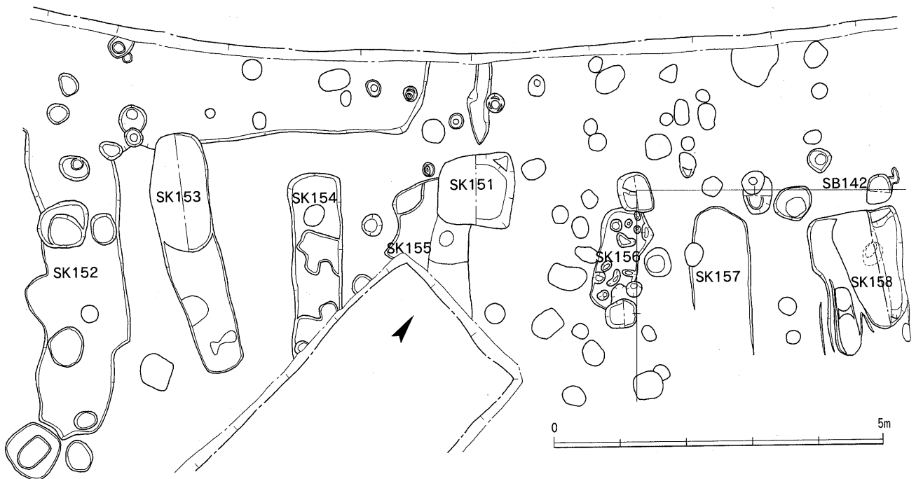
Fig.77 並列土壇群 (SK152~158) 実測図 (1/80)
