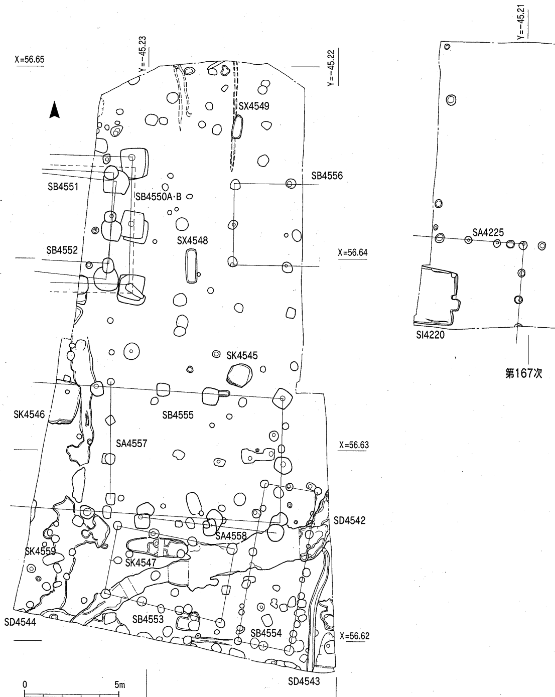
Fig. 5 第186次調査遺構全体図 (1/200)
