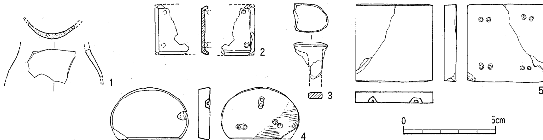
Fig.27 ガラス・銅製品・銚帯実測図 (1/2)
