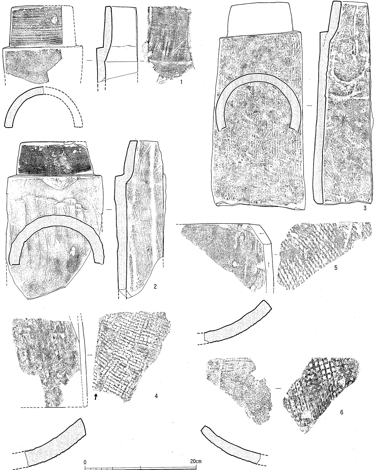
Fig.31 第187次調査出土丸・平瓦拓影 (1/4)
