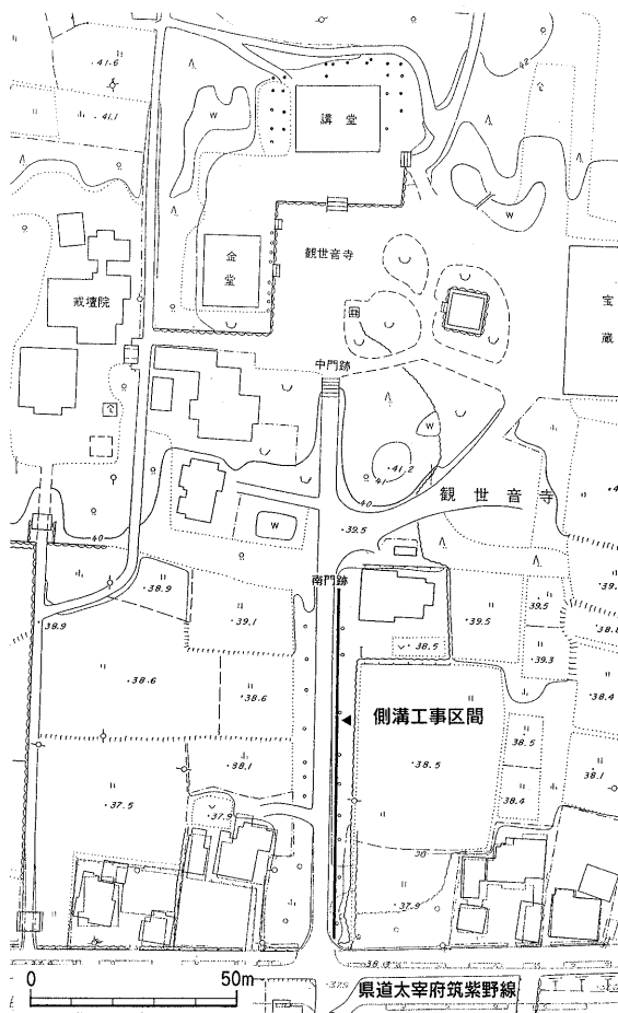
Fig.58 観世音寺側溝工事立会位置図 (1/2,000)
