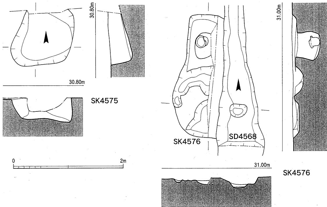
Fig.25 SK4575・4576実測図 (1/40)
