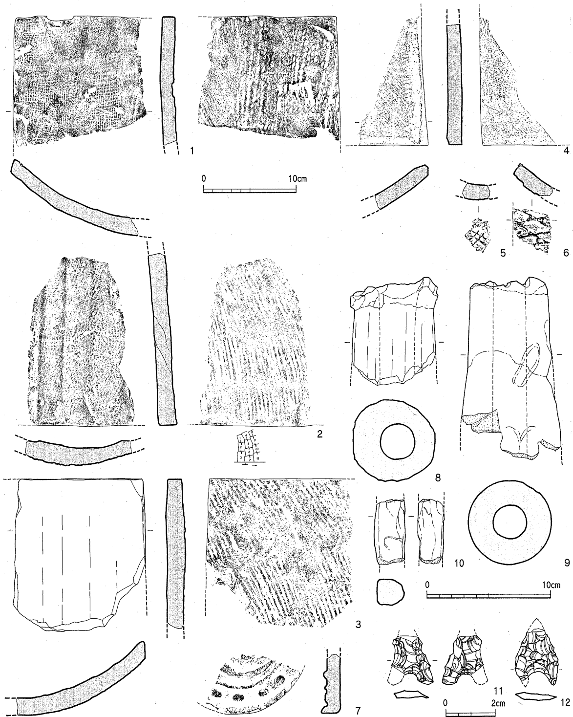
Fig.15 各遺構出土土瓦等実測図 (瓦：1/4, 土製品：1/3, 石鏃：2/3)
