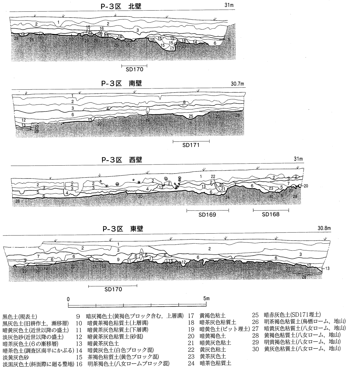
Fig.66 P-3区調査区各壁土層実測図 (1/80)
