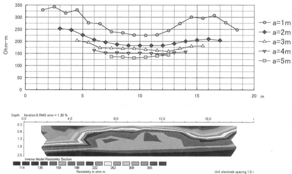
Fig.115 C1異常部付近のウェンナー法による見掛け比抵抗曲線(上図)と2次元インバージョンにより計算した比抵抗断面図(下図)
