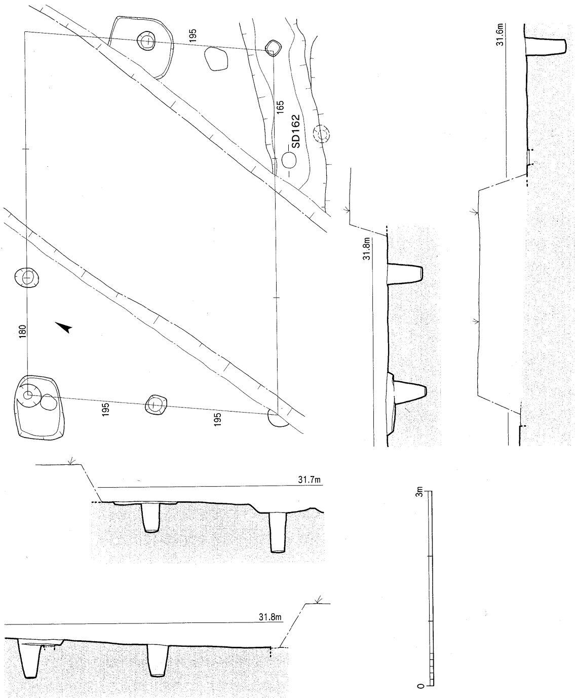
Fig.72 SB145実測図 (1/60)
