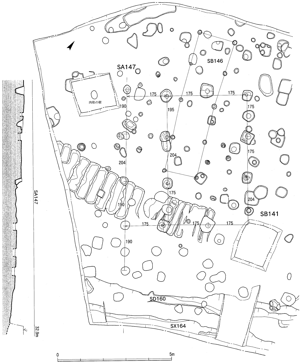
Fig.74 SB141とSA147との関係実測図 (1/80)
