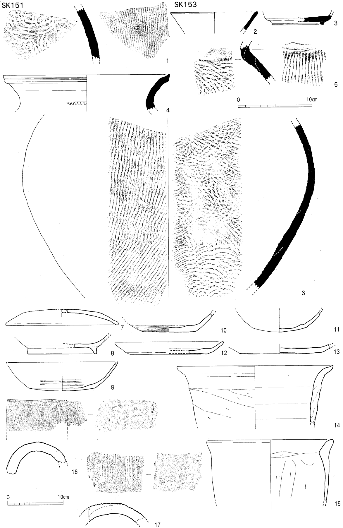
Fig.76 SK151・153出土遺物実測図 (1/3, 瓦: 1/4)
