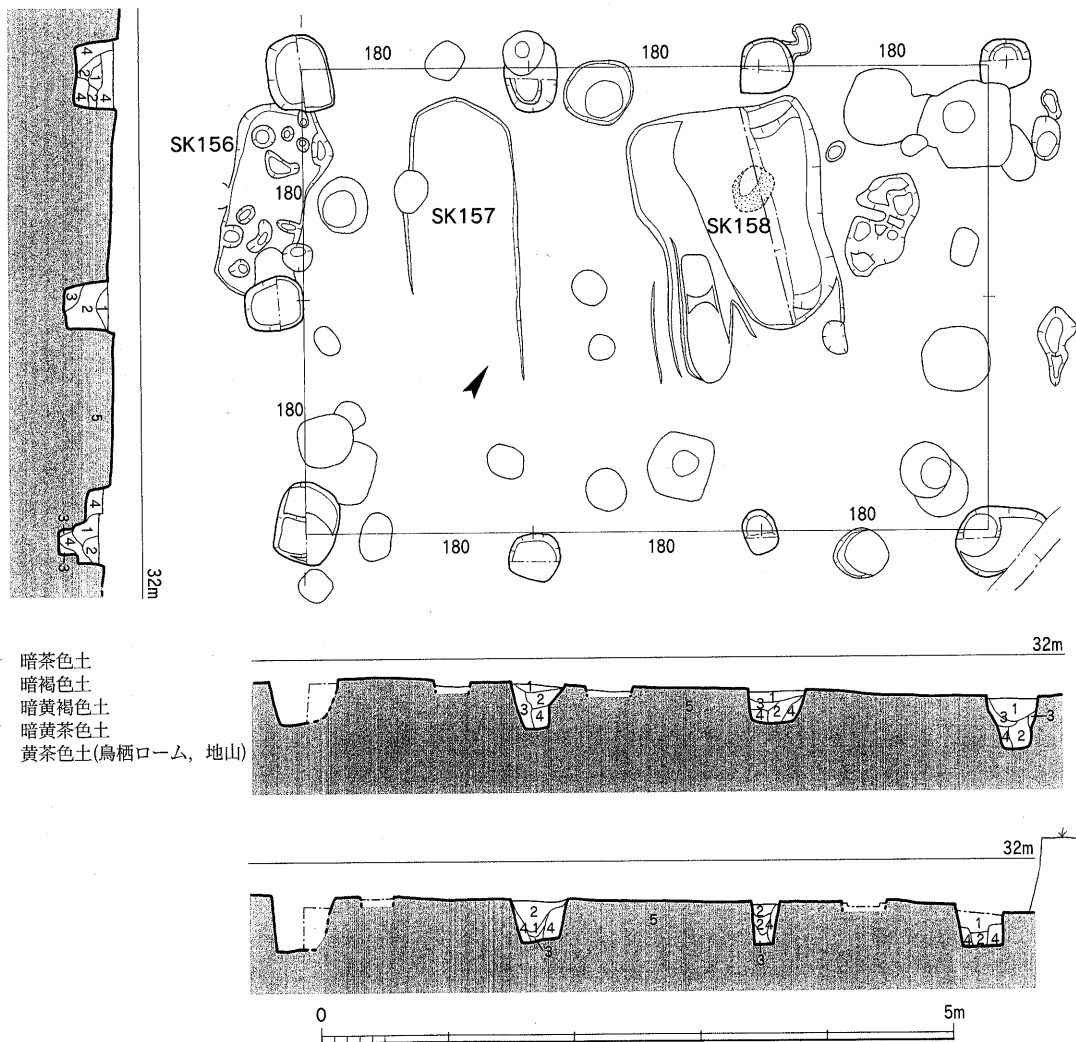
Fig.68 SB142実測図 (1/60)
