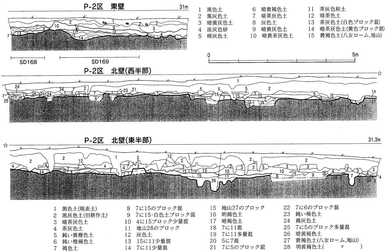
Fig.65 P-2区調査区東・北壁土層実測図 (1/80)
