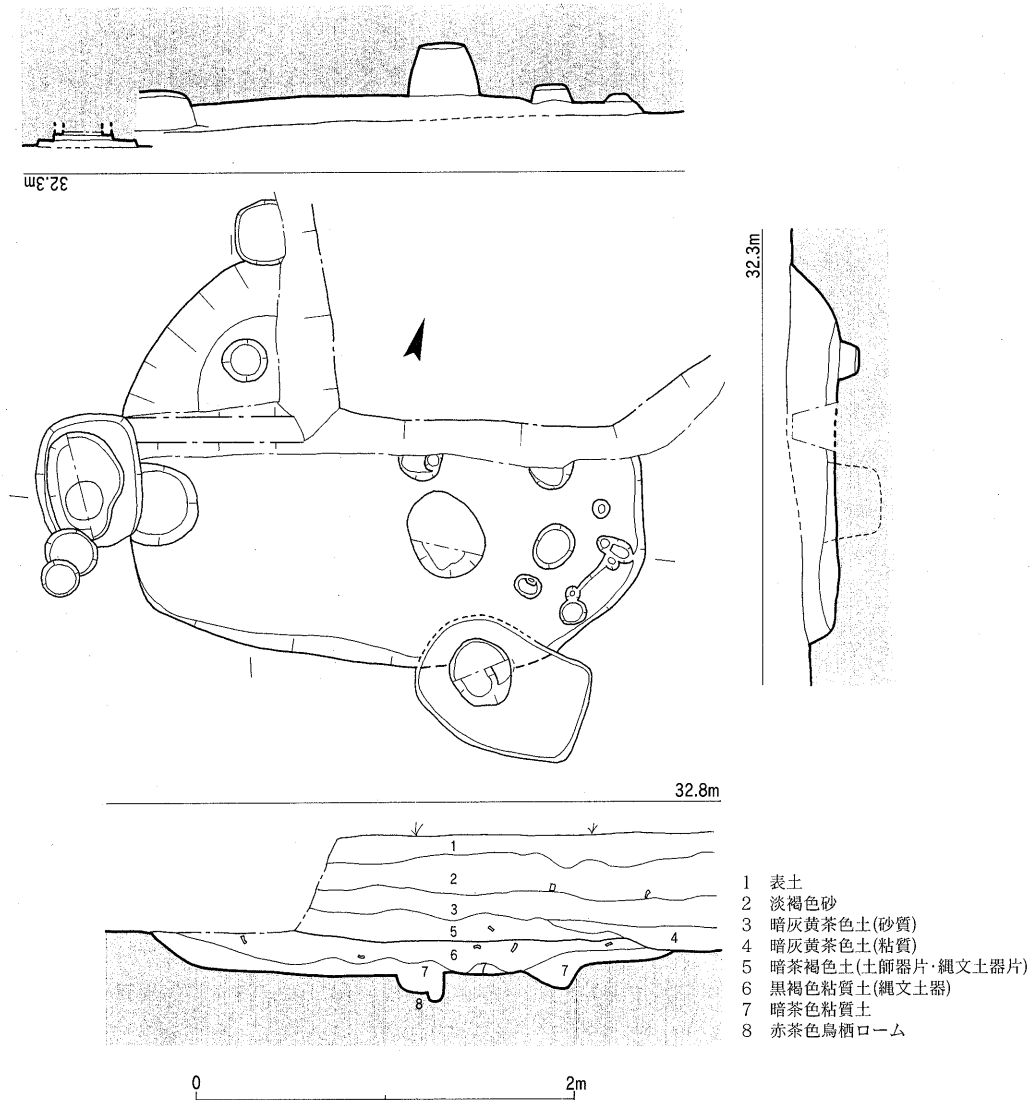
Fig.92 縄文期竪穴住居跡(SI159)実測図 (1/40)
