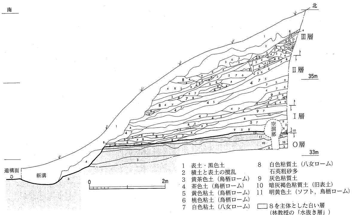
Fig.82 土塁南半 (トレンチ10) 積土状況実測図 (1/60)
