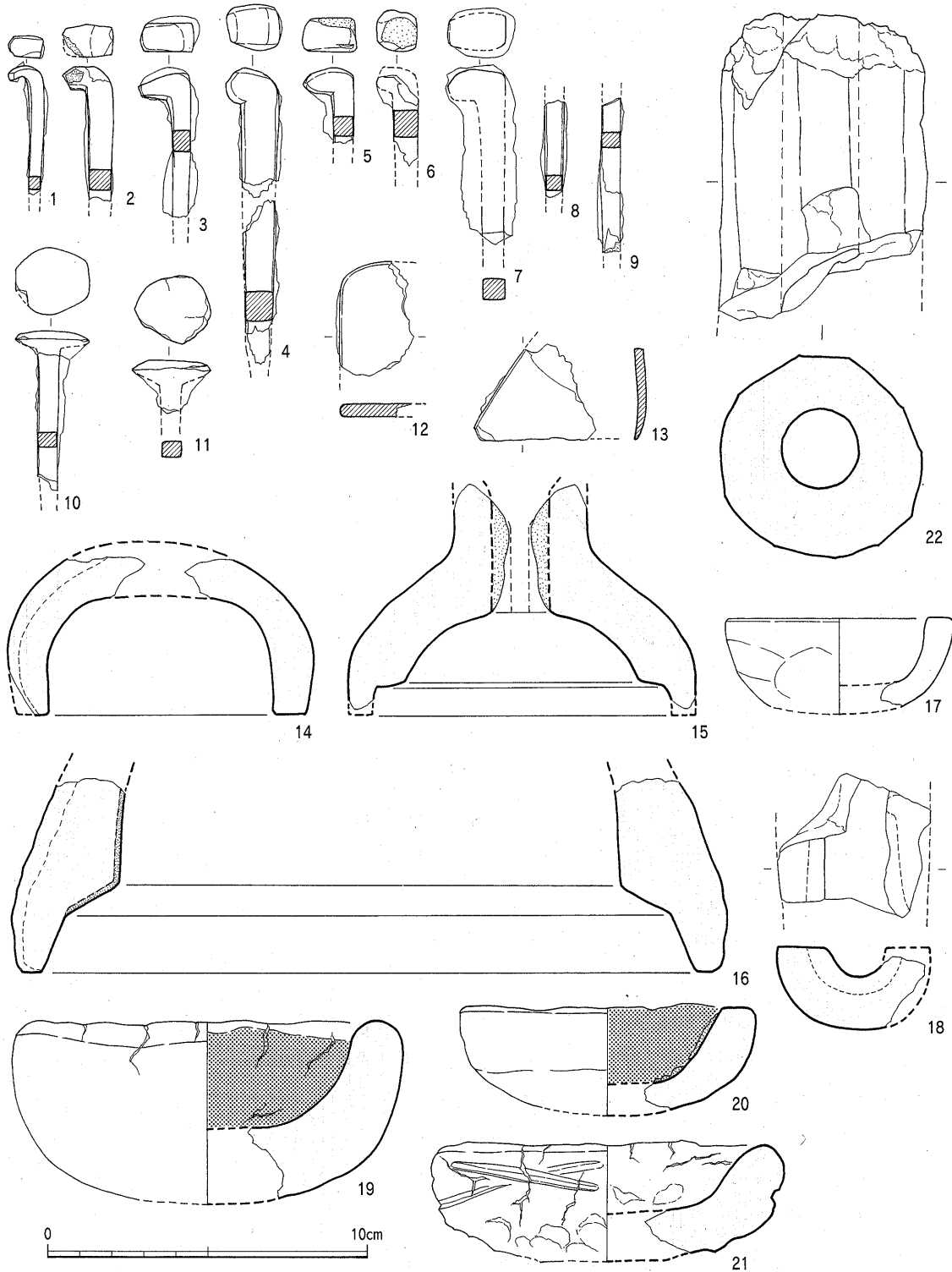
Fig.28 鉄器・鑄型等実測図 (1/2)
