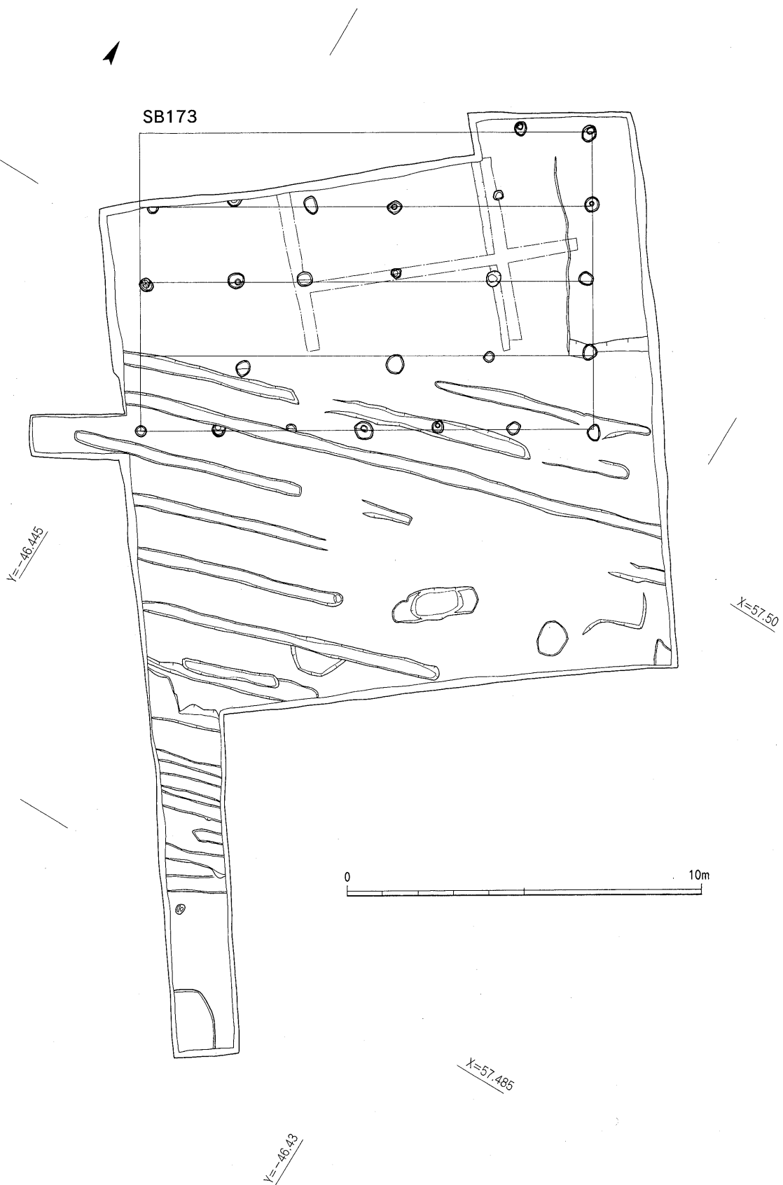
Fig.100 B区遺構配置図 (1/150)
