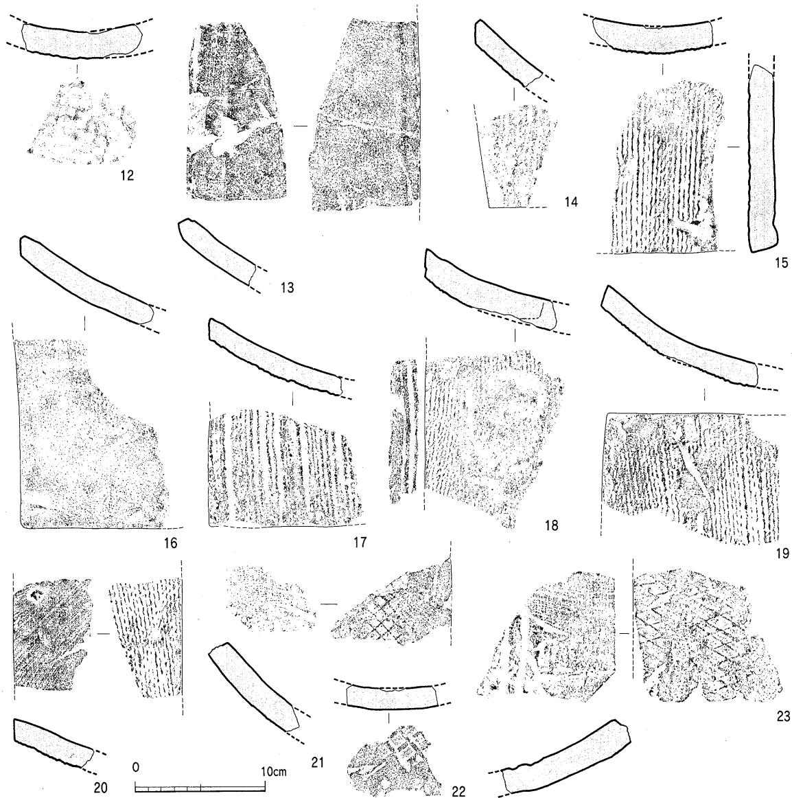
Fig.87 水城跡第33次出土平瓦実測図 (1/4)
