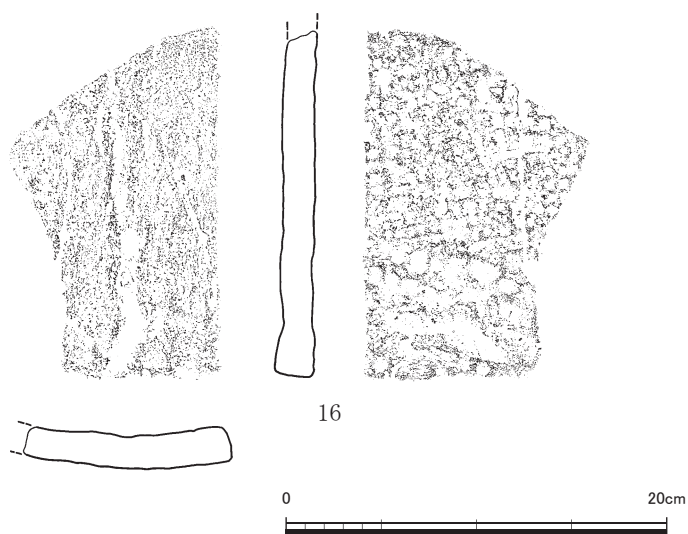
第 16 图 平瓦实测图⑦ (1/4)
