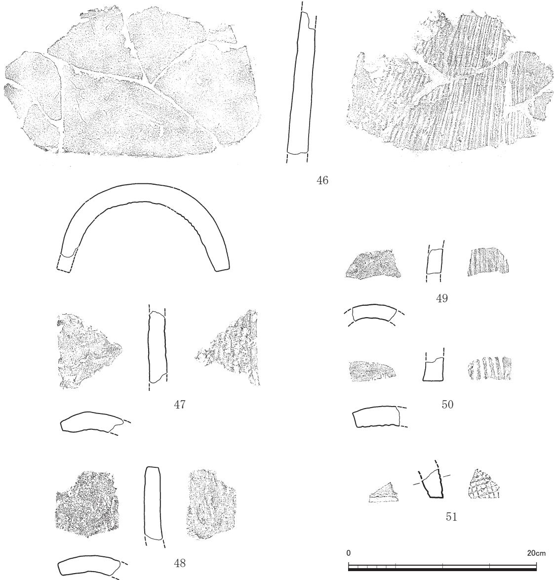
第22図 丸瓦実測図 (1/4)
