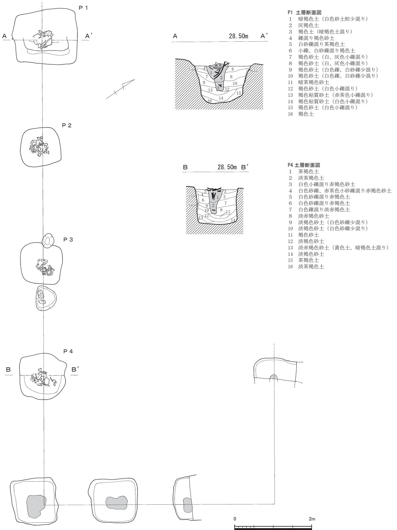
第4図 1号掘立柱建物跡実測図 (1/60)
