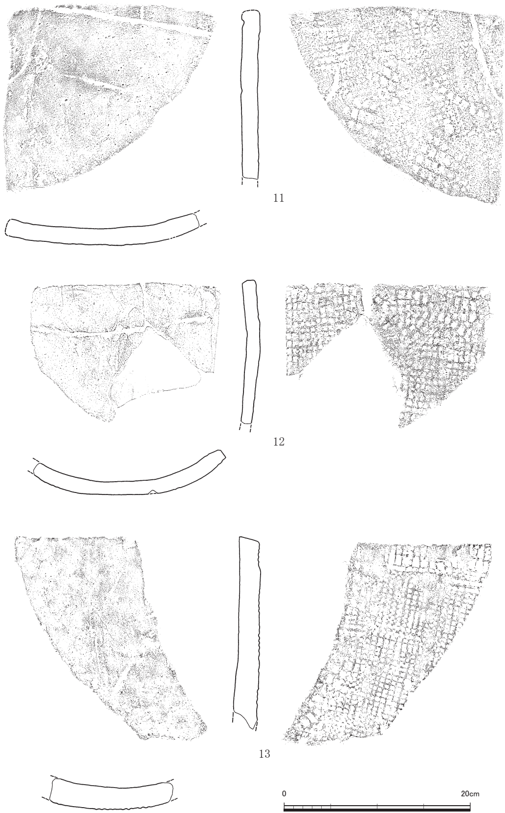
第15图 平瓦实测图⑥ (1/4)
