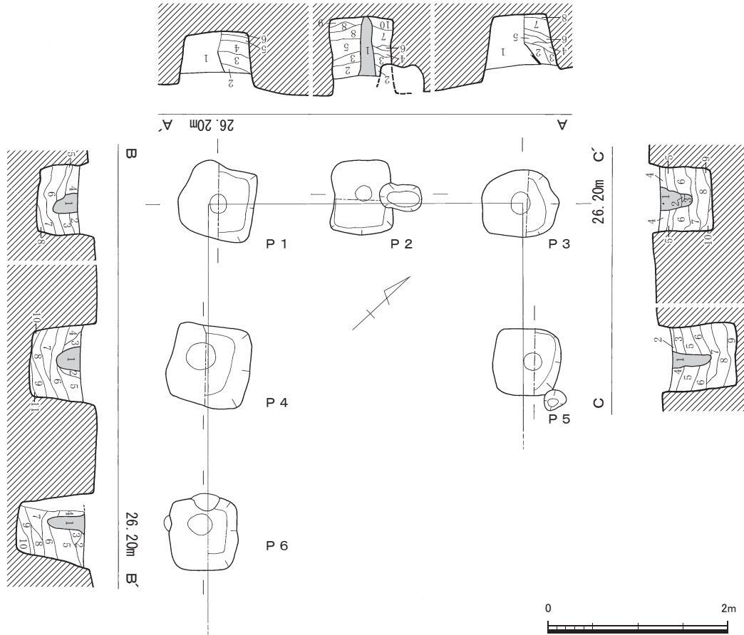
第5図 2号掘立柱建物跡実測図 (1/60)
