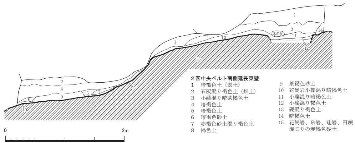
第7図 土層断面実測図② (1/40)
