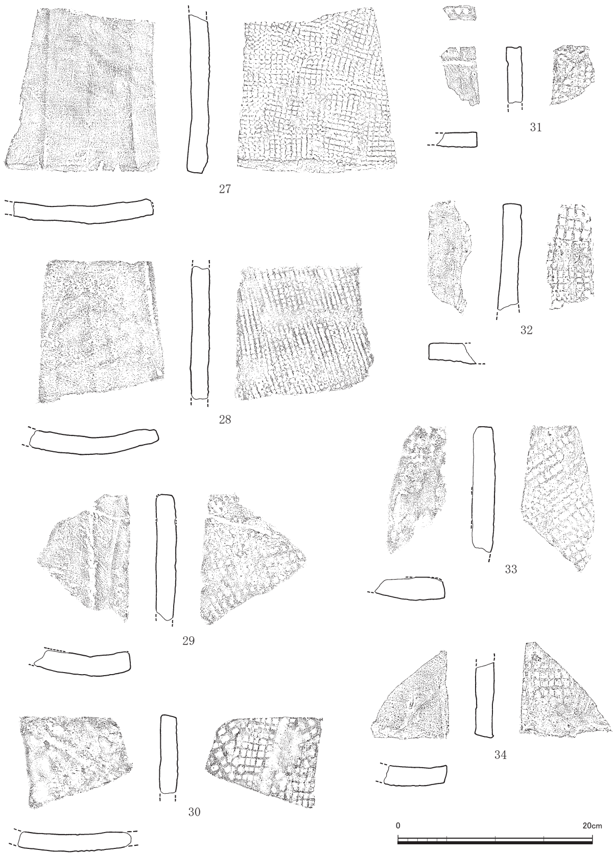
第19图 平瓦实测图⑩ (1/4)
