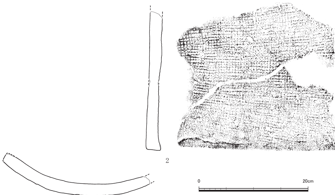
第11図 平瓦実測図② (1/4)
