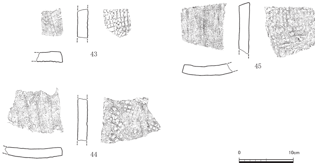
第 21 図 平瓦実測図⑫ (1/4)
