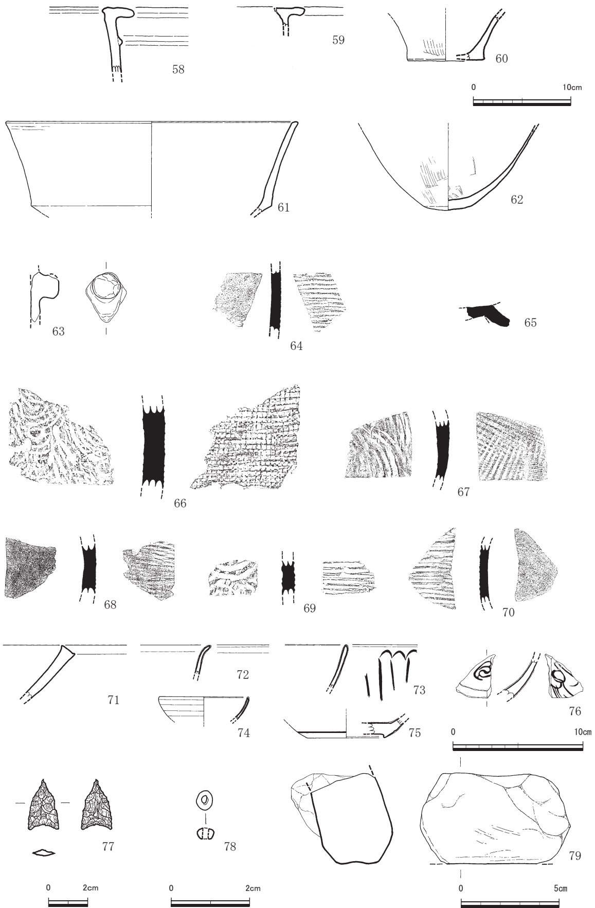
第 25 図 土器・陶磁器・石器・ガラス小玉・土製品実測図 (1/1・1/2・1/3・1/4)
