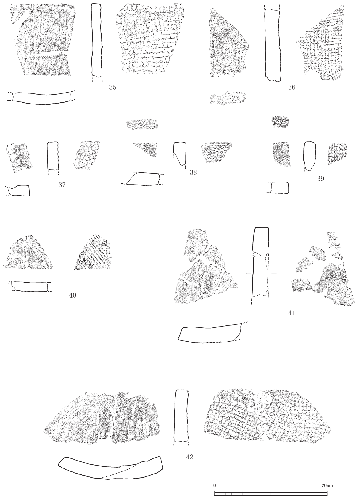
第 20 图 平瓦实测图① (1/4)
