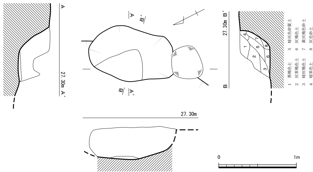
第11図 1号土坑実測図 (1/30)
