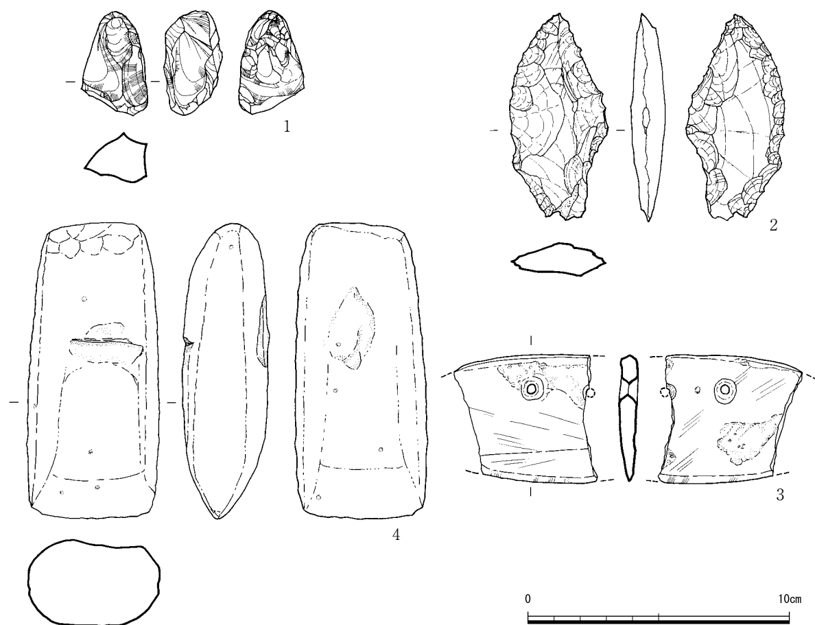
第9図 石器実測図 (1/2)
