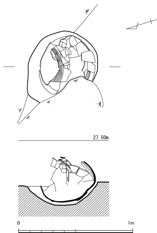
第6図 1号甕棺墓実測図（1/20）
