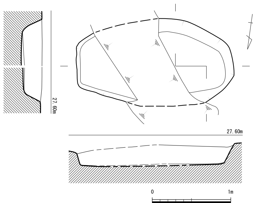
第4図 1号土坑実測図 (1/30)
