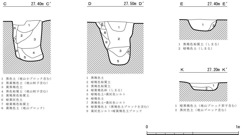
第12図 溝断面土層図① (1/20)
