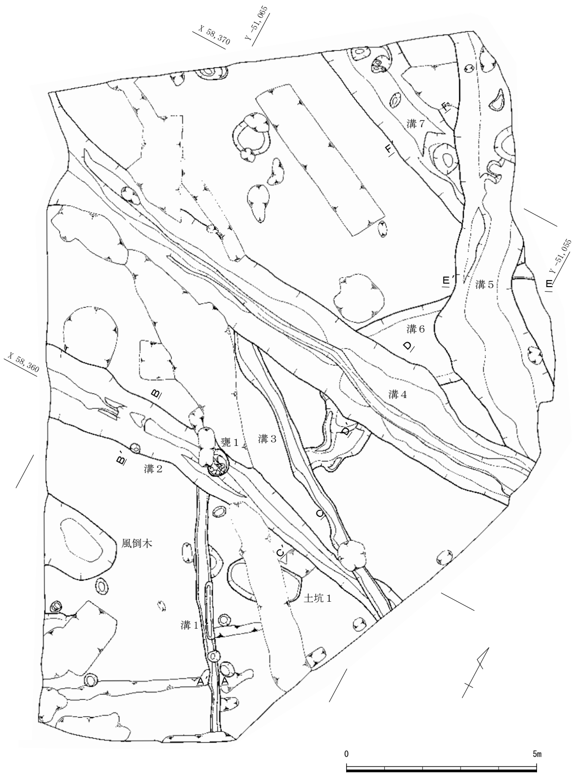
第3図 宮の下遺跡5次調査遺構配置図 (1/100)
