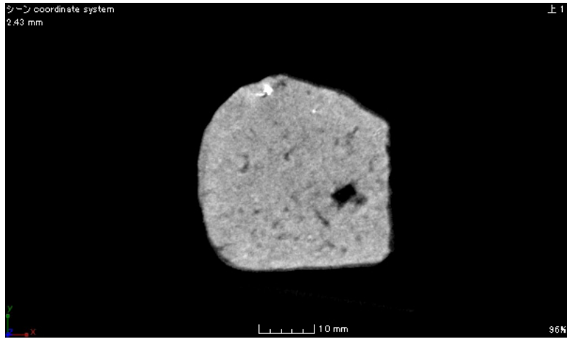
土製鑄型9号 断面 b-b'
