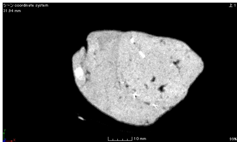
土製鑄型 11 号 断面 b-b'
