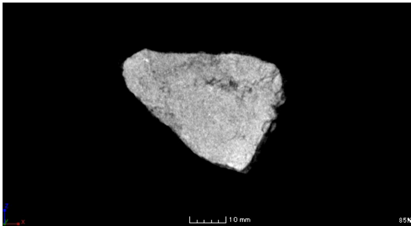
土製鑄型 14号 断面
