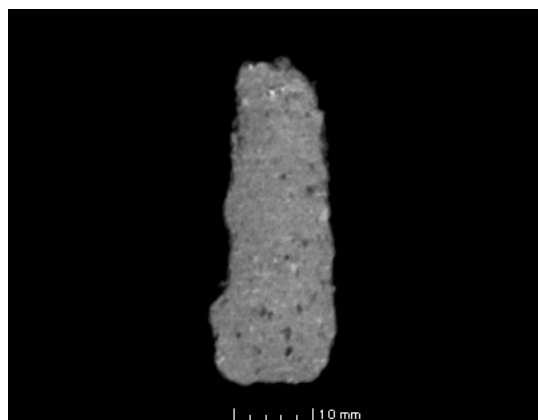
土製鑄型 20号 断面 b-b'
