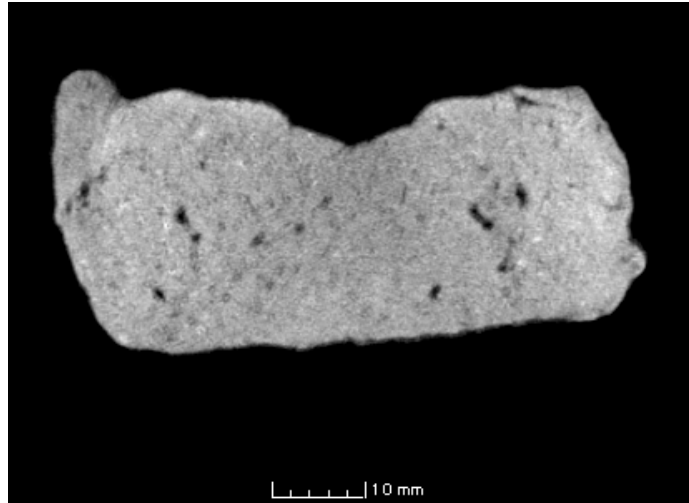
土製鑄型 5号 断面 a-a'
