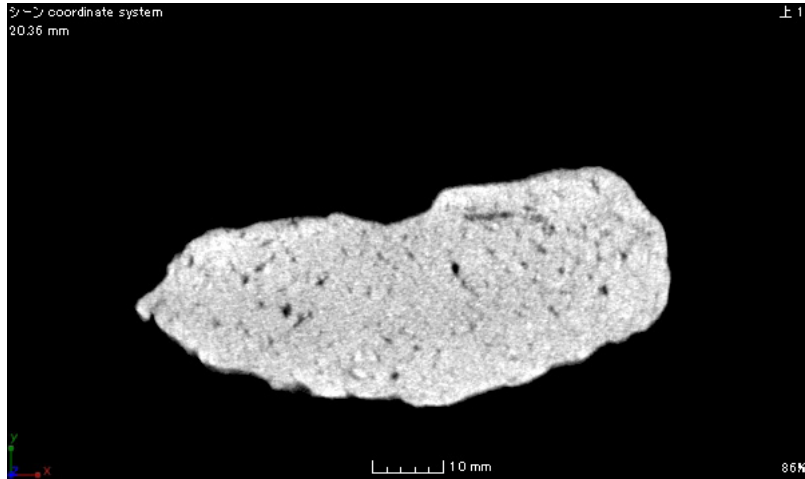
土製鋳型 24 号 断面 a-a'
