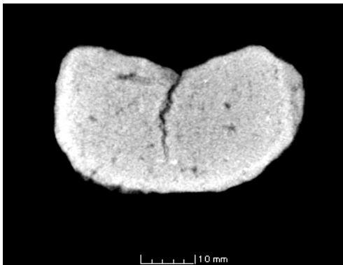
土製鑄型 6号 断面 d-d'
