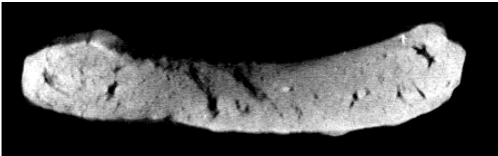
土製鑄型 7号 断面 d-d'
