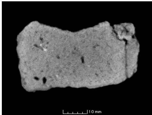
土製鑄型 4号 断面 c-c'
