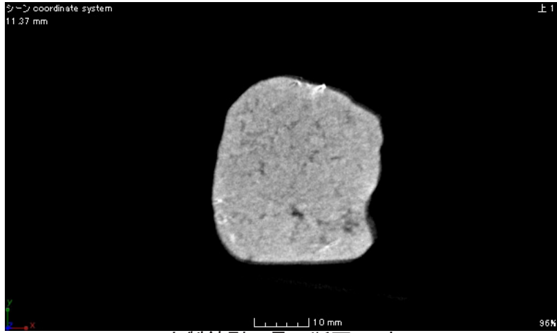
土製鑄型9号 断面 a-a'
