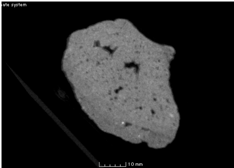
土製鑄型 2号 断面 a-a'
