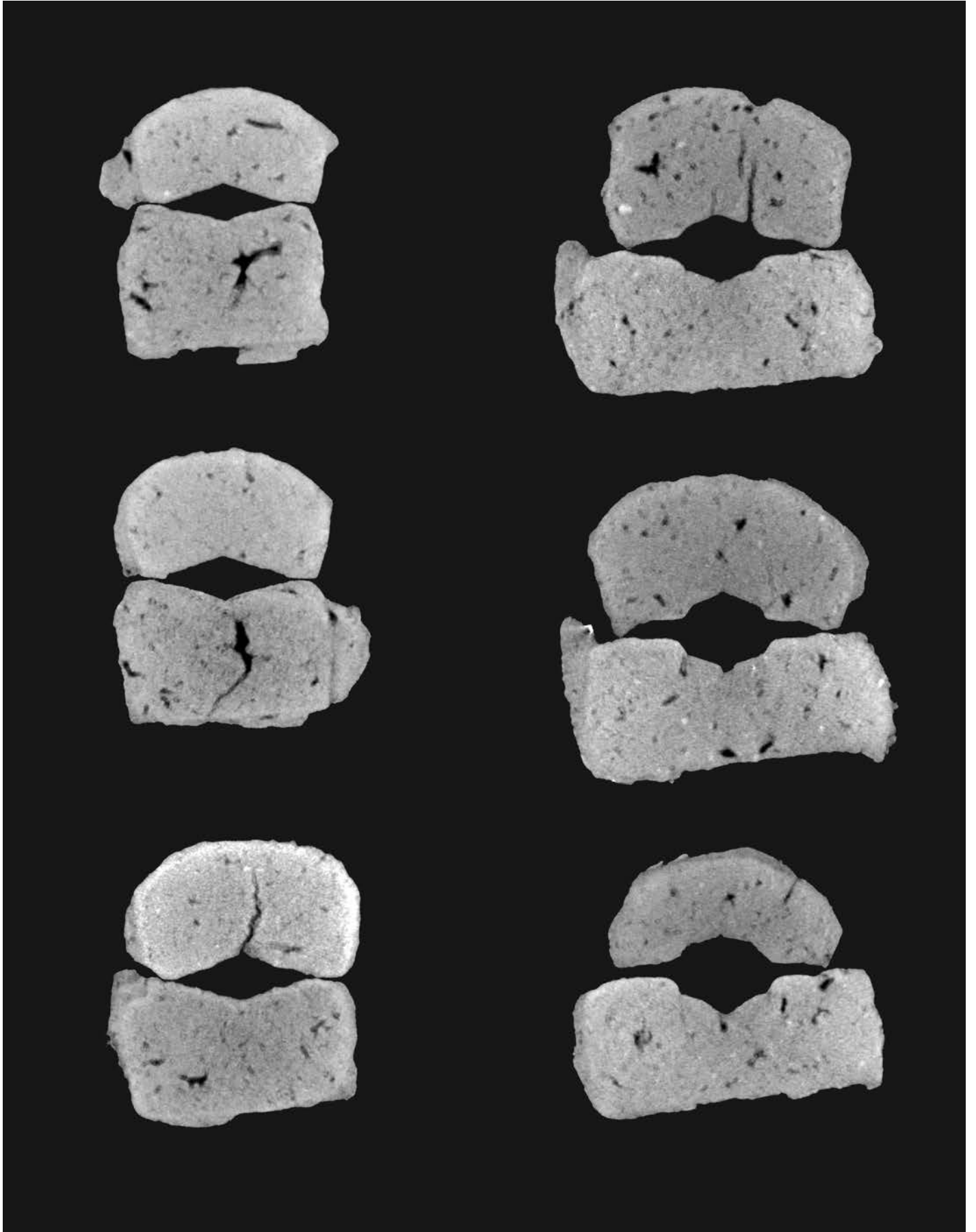
土製鑄型4、5、6号（合わせ鑄型、武器形）断面
