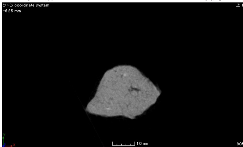
土製鑄型 18号 断面
