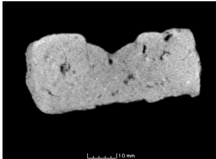
土製鑄型 5号 断面 c-c'
