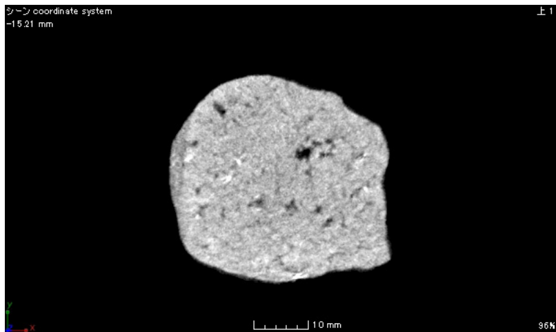
土製鑄型9号 断面 c-c'
