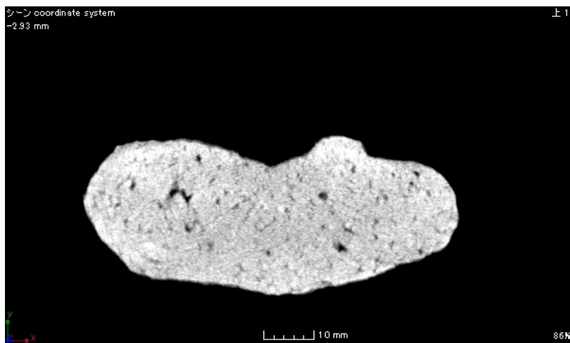
土製鋳型 24 号 断面 b-b'
