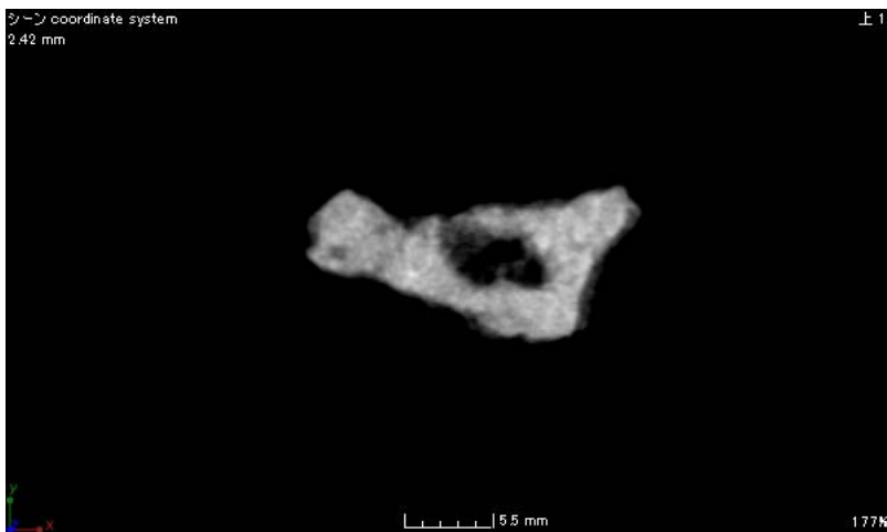
土製鑄型 15号 断面
