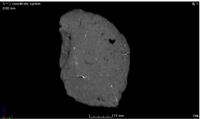
土製鑄型 17号 断面 b-b'
