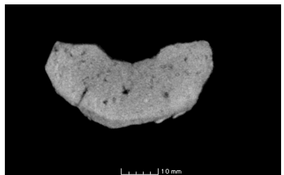
土製鑄型 6号 断面 i-i'
