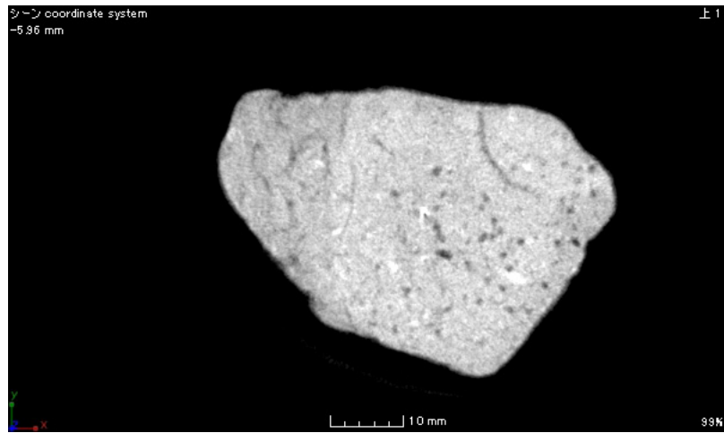
土製鑄型 11 号 断面 a-a'
