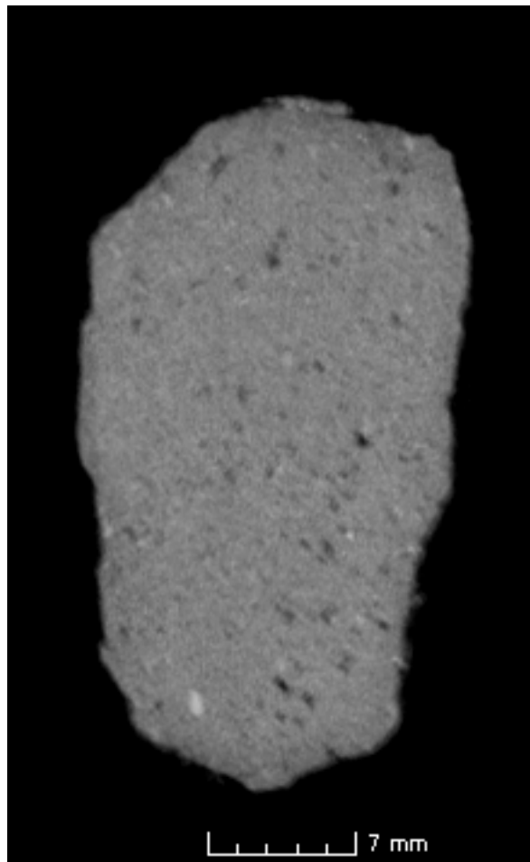
土製鑄型 3号 断面 c-c'
