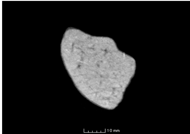
土製鑄型 1号 断面 b-b'
