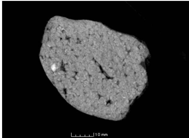
土製鑄型 1号 断面 a-a'
