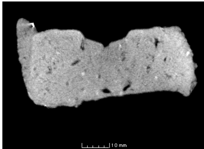
土製鑄型 5号 断面 b-b'
