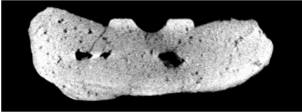
土製鑄型 8号 断面 b-b'
