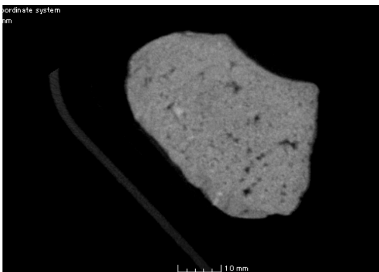
土製鑄型 2号 断面 c-c'
