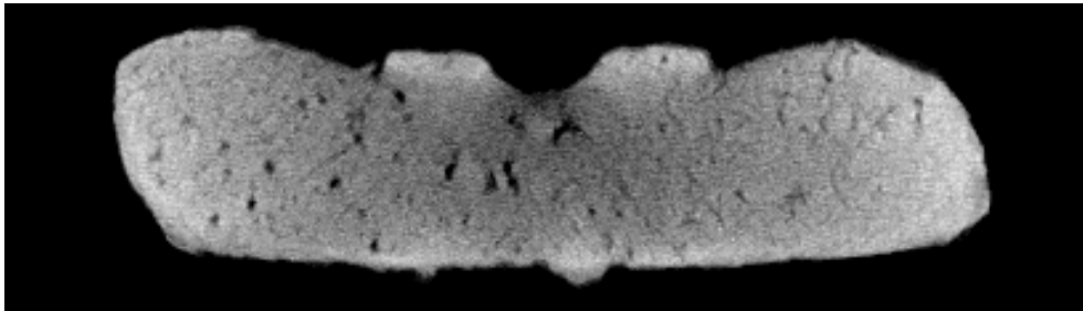
土製鑄型 8号 断面 c-c'
