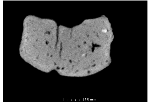
土製鑄型 6号 断面 g-g'
