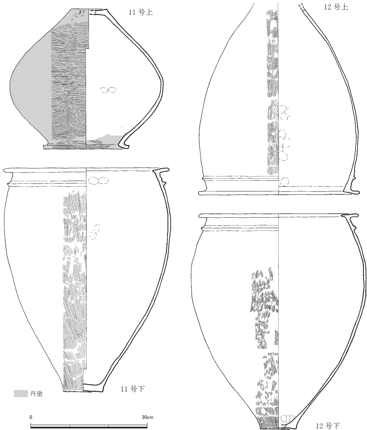
第57図 甕棺実測図⑤ (1/6)
