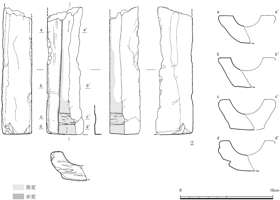
第 18 图 1号竖穴建物跡出土石製鑄型実測图① (1/2)
