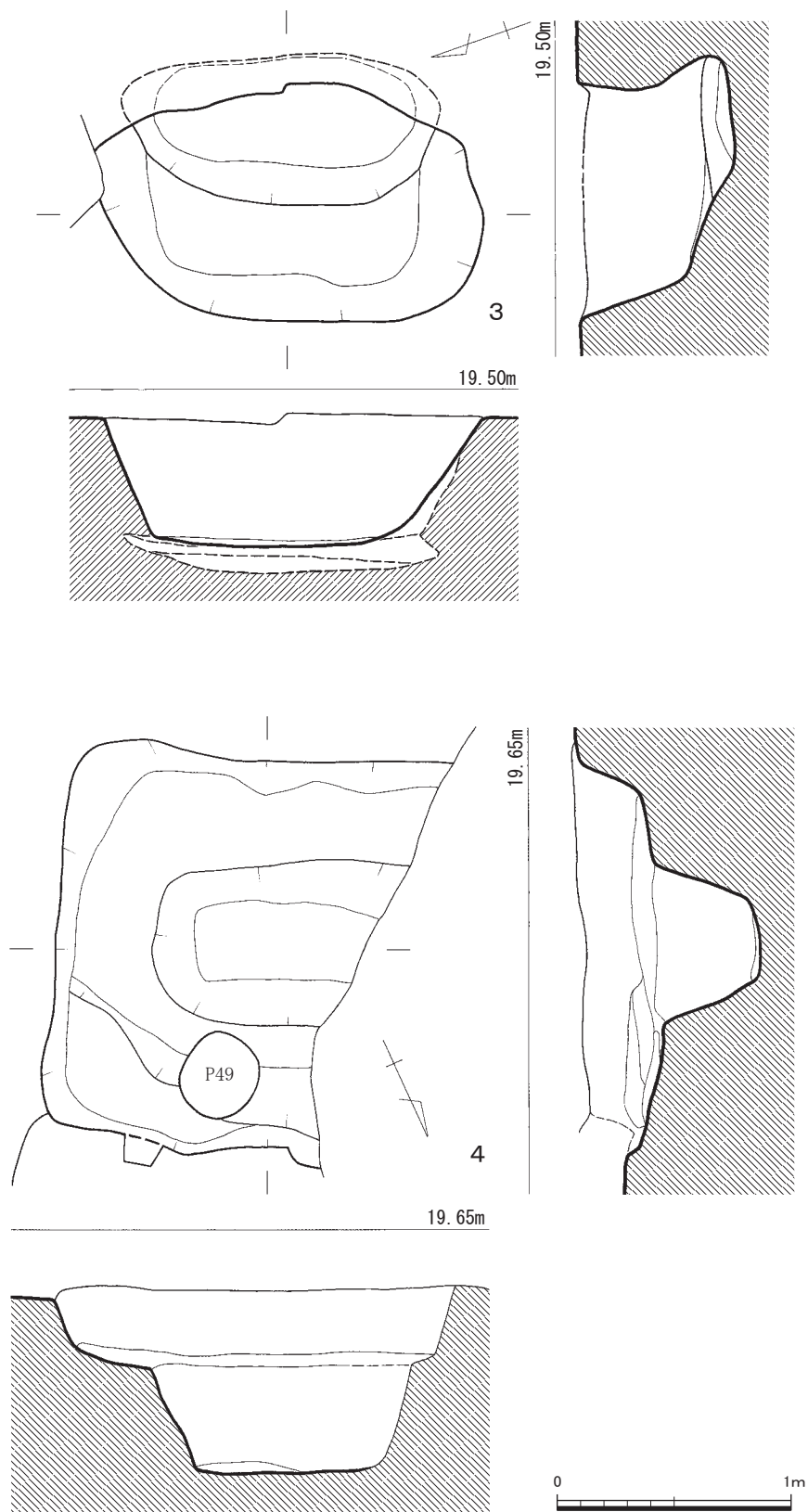
第 34 图 3·4 号土坑墓实测图 (1/30)
