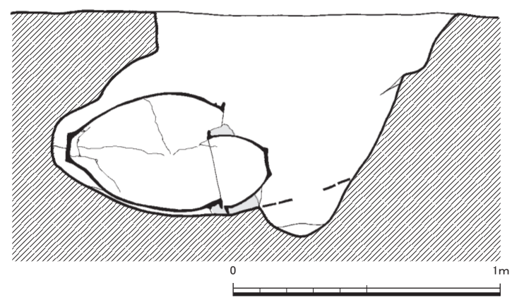
第 49 図 甕棺墓実測図⑮ (1/20)
