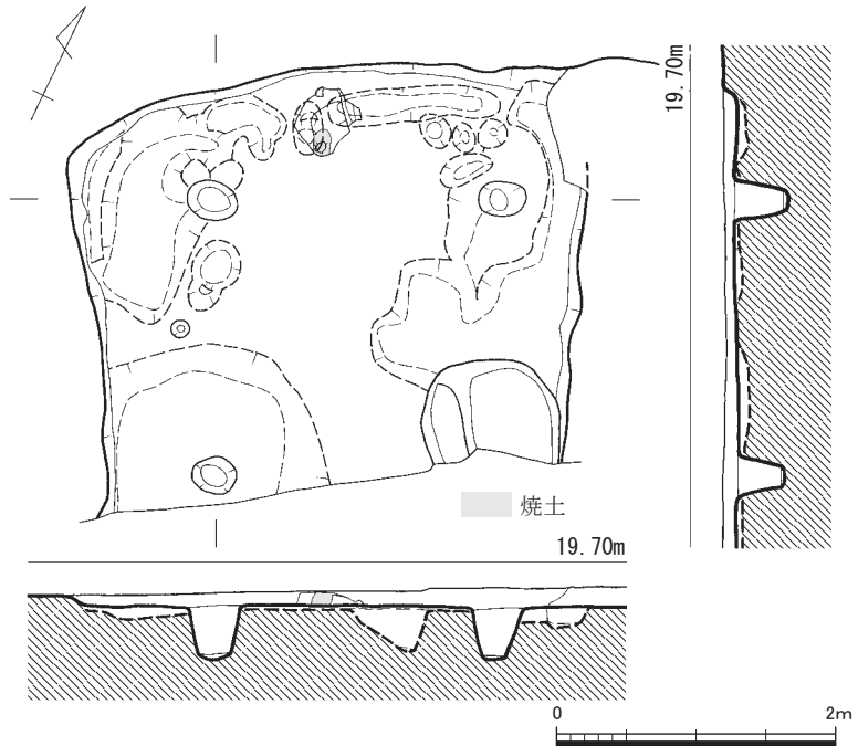
第 71 図 2 号竪穴建物跡実測図 (1/60)
