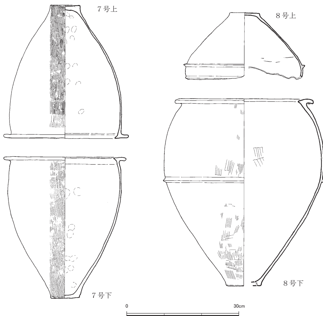
第 55 図 甕棺実測図③ (1/6)
