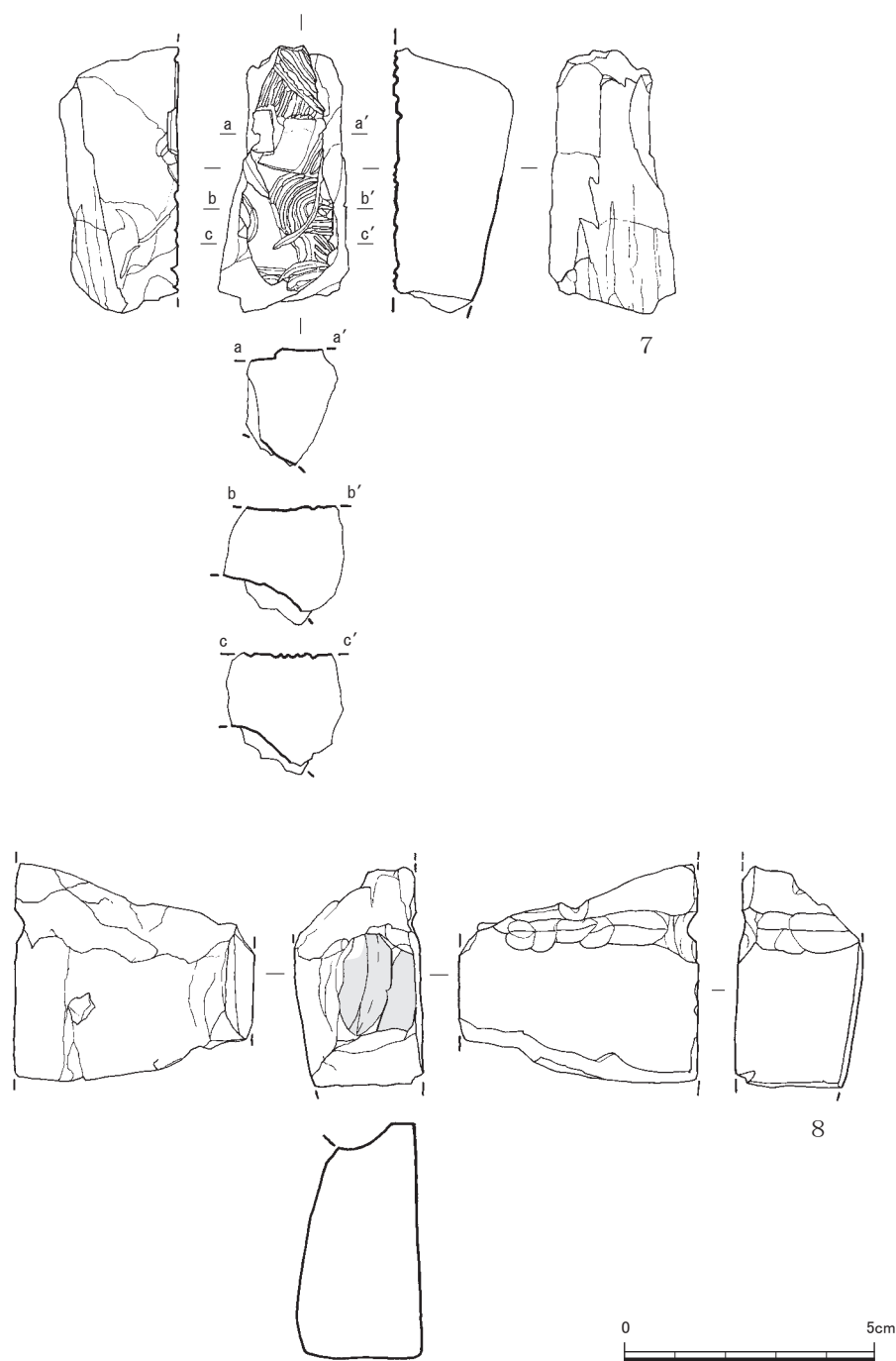
第21図 34号甕棺墓・2号掘立柱建物跡出土石製鑄型実測図(2/3)
