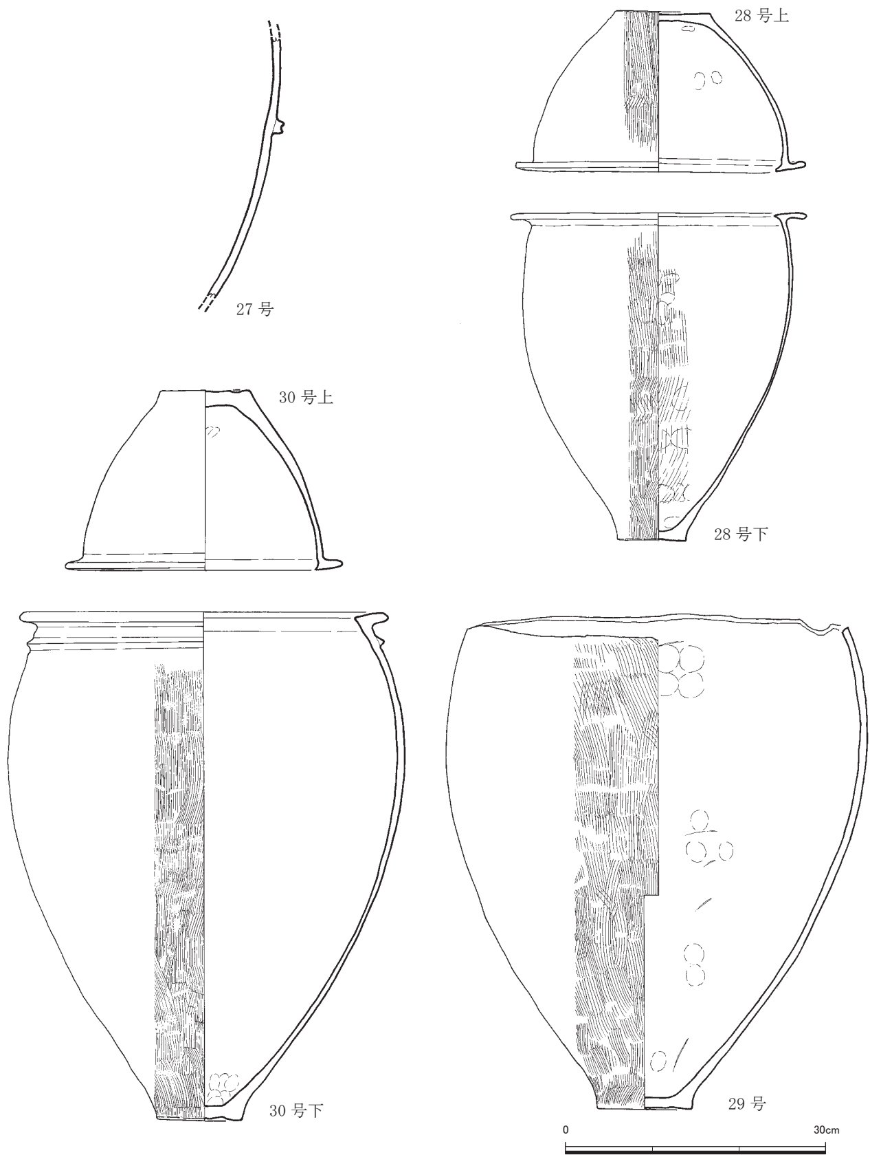
第64图 甕棺実測图⑫ (1/6)
