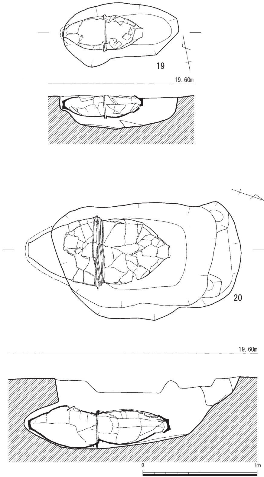
第44图 甕棺墓実測图⑩ (1/20)
