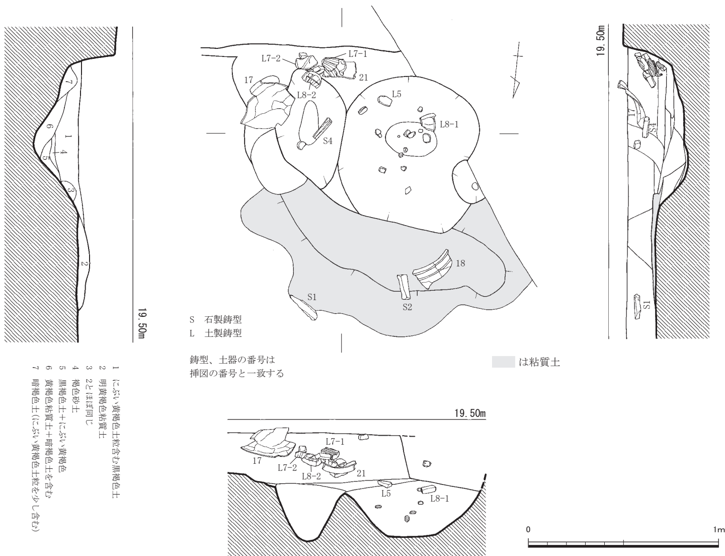
第5図 1号竪穴建物跡屋内土坑・鋳型出土状況実測図(1/20)
