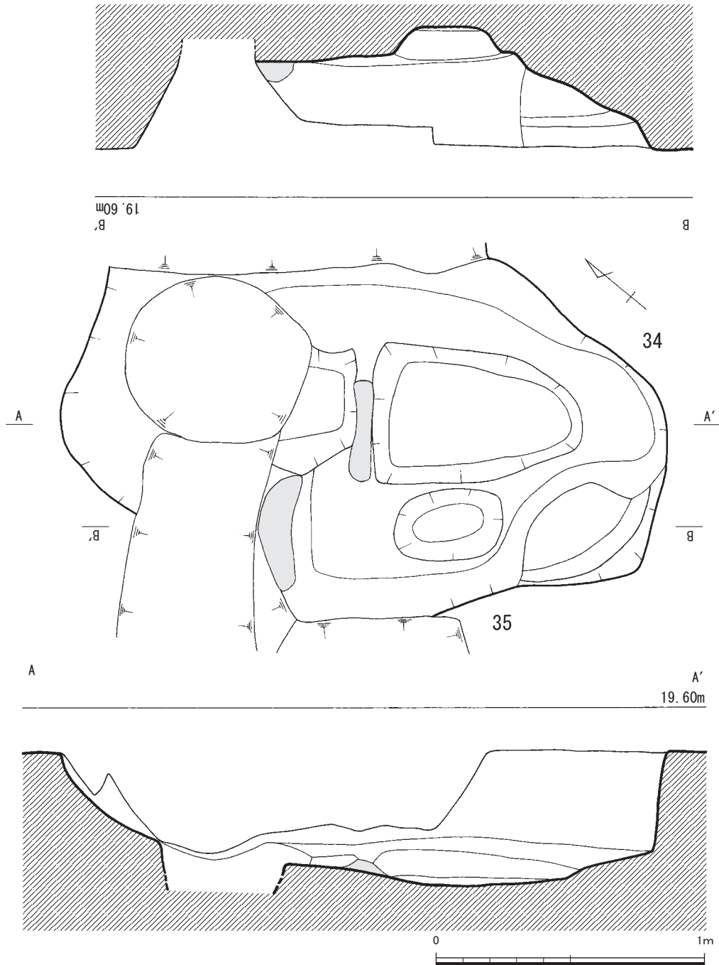
第51図 甕棺墓実測図① (1/20)
