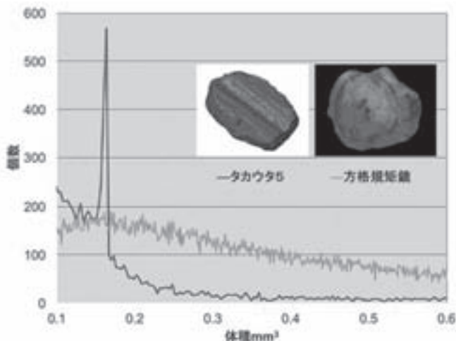
図8 須玖タカウタ遺跡土製鑄型と中国鏡鑄型の空隙分布
