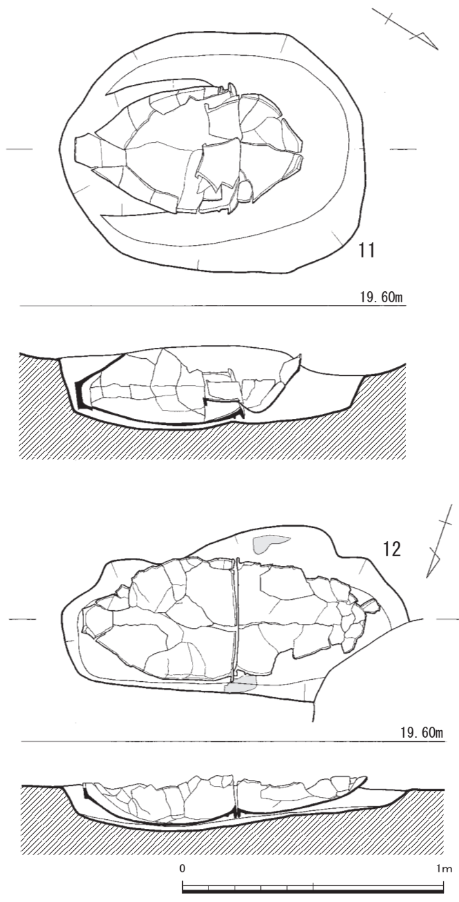
第40図 甕棺墓実測図⑥ (1/20)
