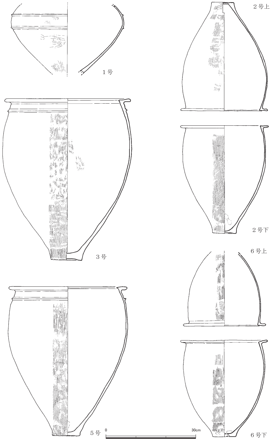
第 53 图 甕棺実測图① (1/6)
