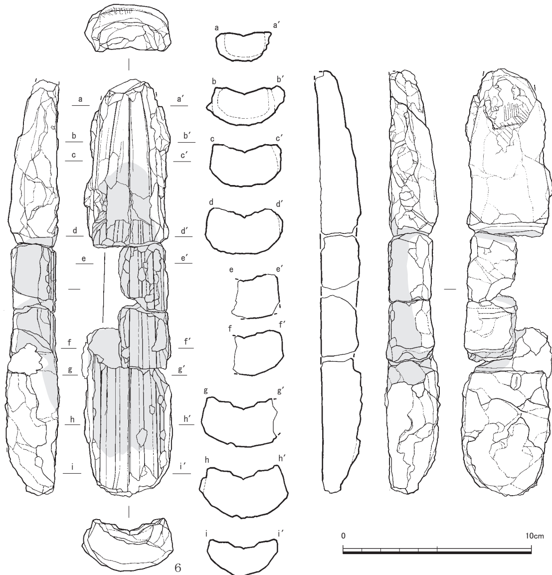
第24図 1号竪穴建物跡出土土製鑄型実測図③ (1/2)
