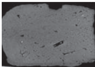
図3 土製鋳型の断面像
