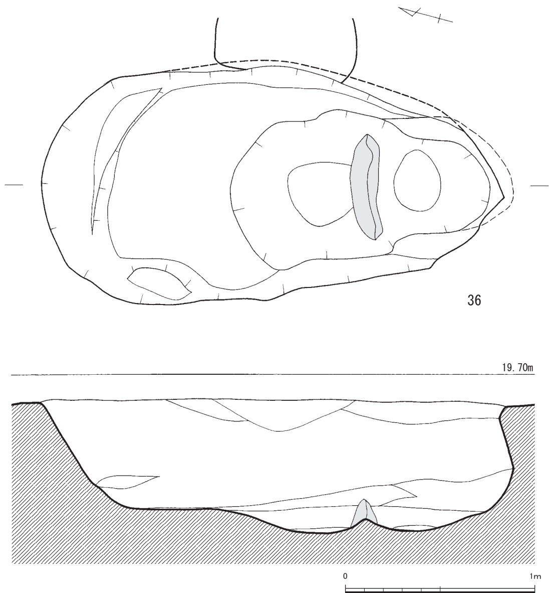
第 52 図 甕棺墓実測図⑩ (1/20)
