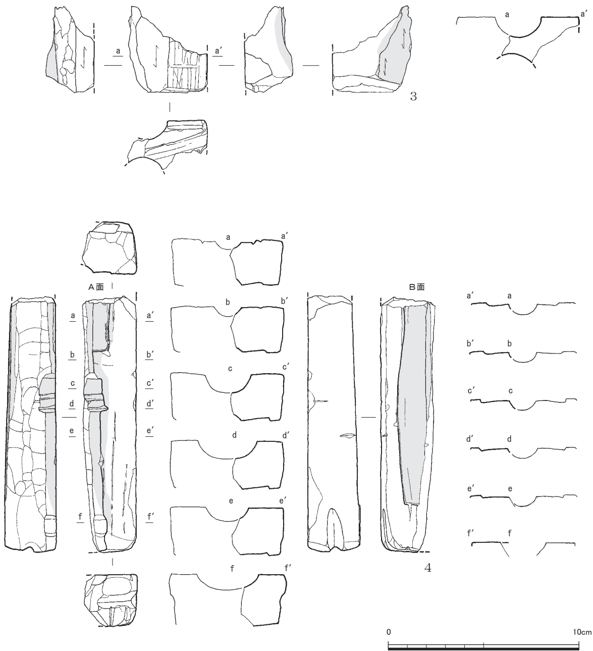
第19図 1号竪穴建物跡出土石製鑄型実測図② (1/2)
