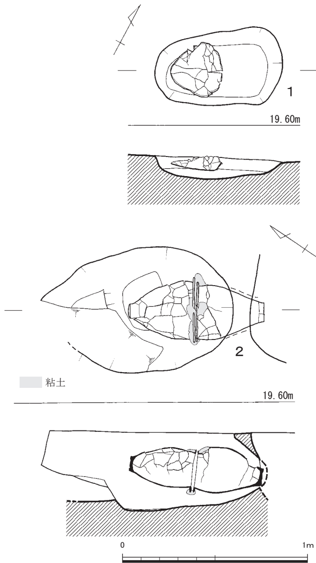
第35図 甕棺墓実測図① (1/20)
