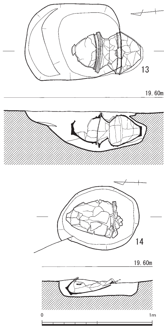
第41図 甕棺墓実測図⑦(1/20)
