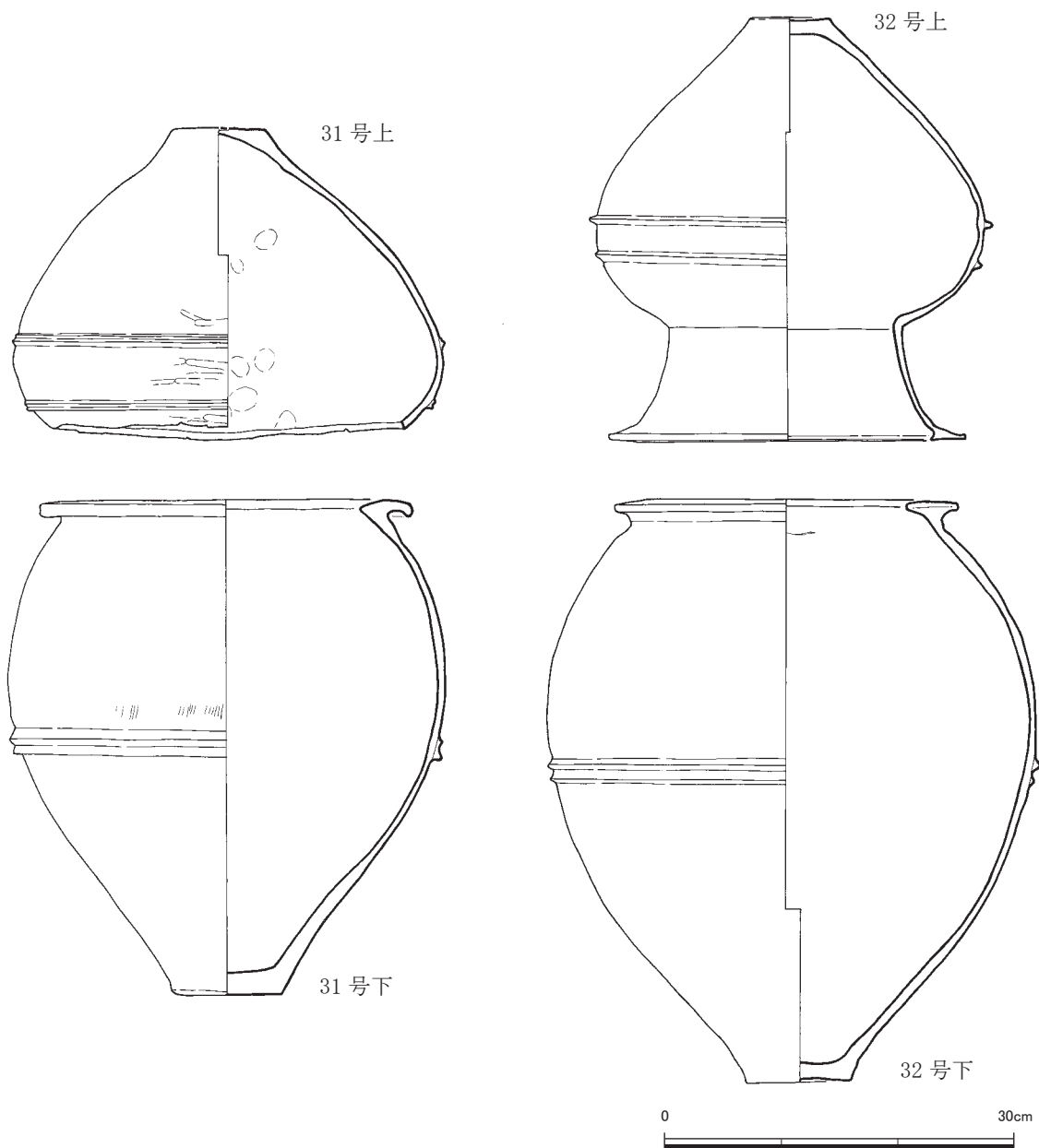
第 65 図 甕棺実測図⑬ (1/6)
