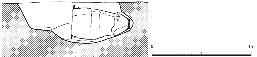
第46图 甕棺墓実測图⑫ (1/20)
