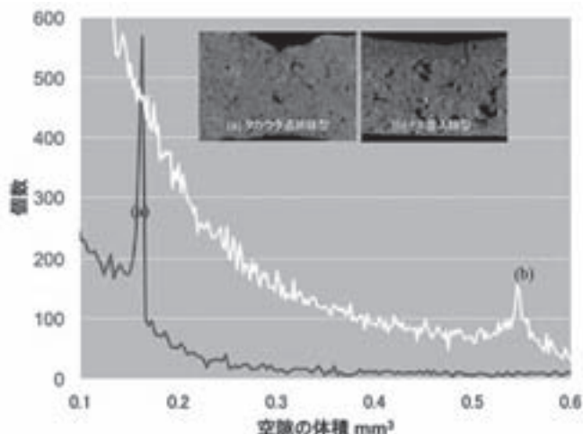
図6 須玖タカウタ遺跡土製鑄型と粃殻混入鑄型の空隙分布
