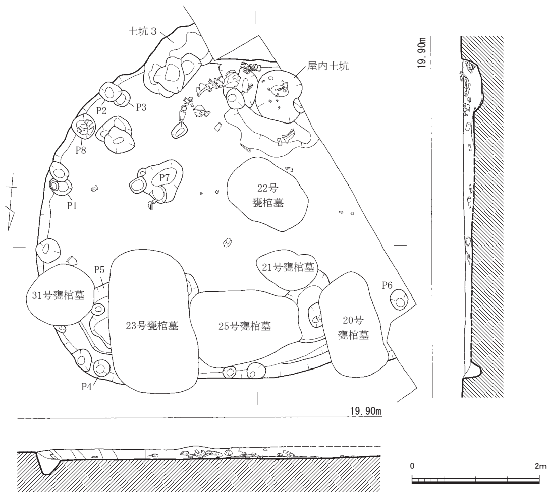
第4図 1号竪穴建物跡実測図 (1/60)
