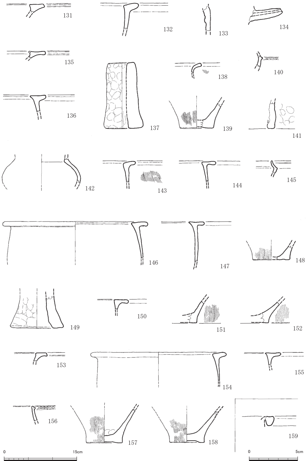
第 68 图 20 ~ 23 · 25 · 29 · 35 · 36 号甕棺墓出土土器实测图 (1/4 · 1/2)
