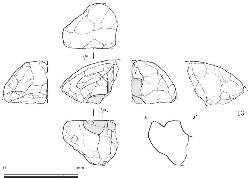
第 28 図 1 号竪穴建物跡出土土製鋳型実測図⑦ (2/3)
