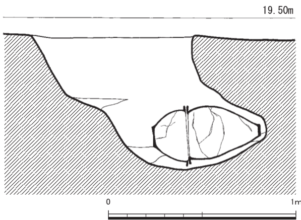
第48図 甕棺墓実測図⑭ (1/20)
