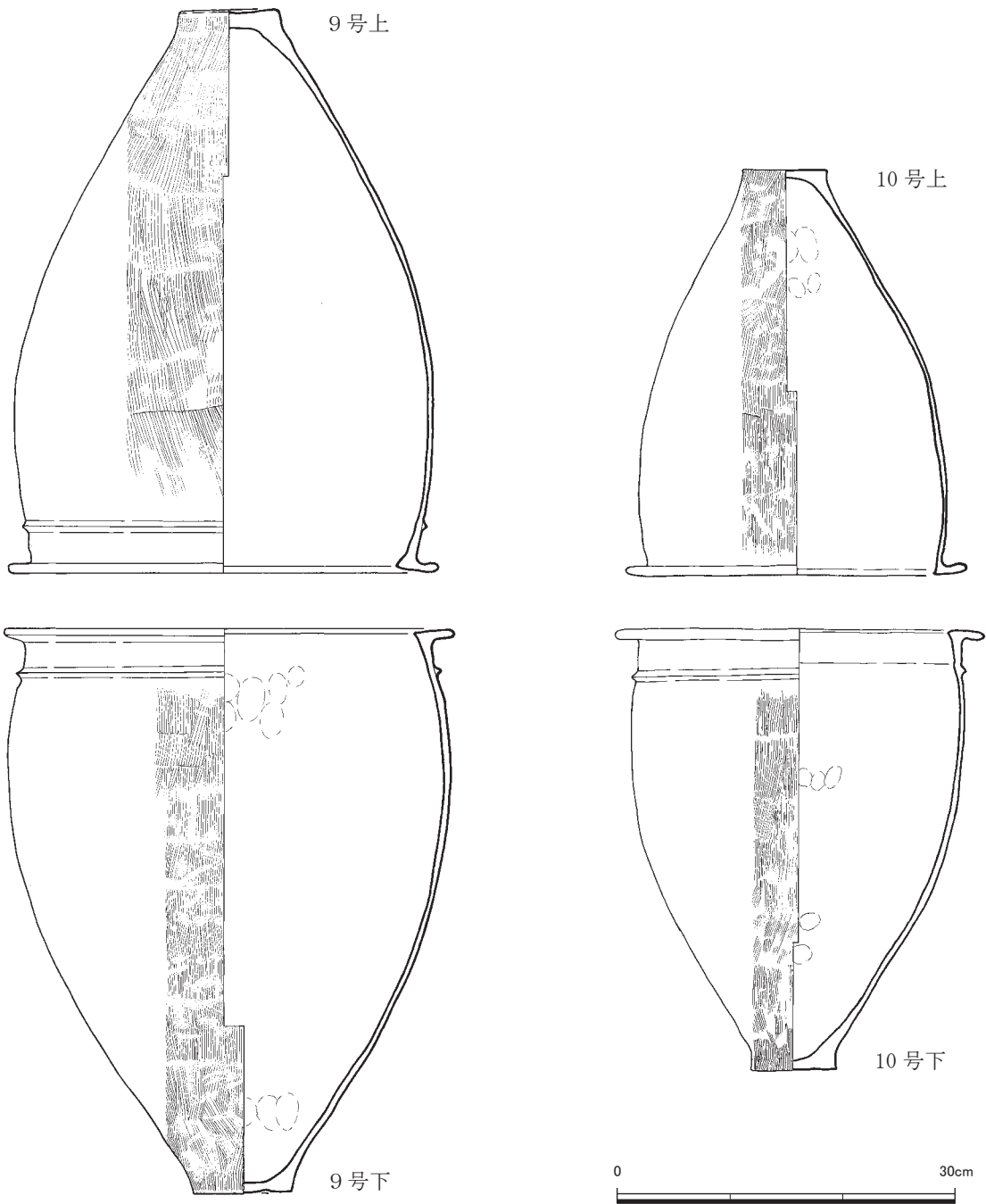
第56図 甕棺実測図④ (1/6)
