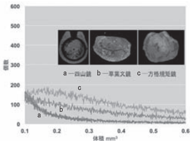
図7 漢代中国鏡鑄型の空隙分布
