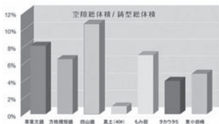
図9 各種土製鑄型の空隙率の比較
