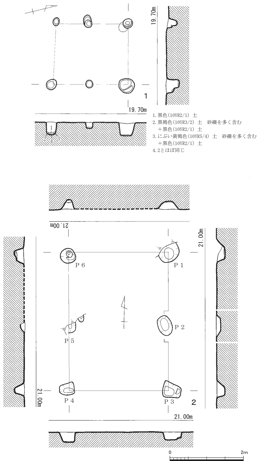
第6図 1・2号掘立柱建物跡実測図 (1/60)
