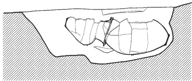
第50图 甕棺墓実測图⑩ (1/20)
