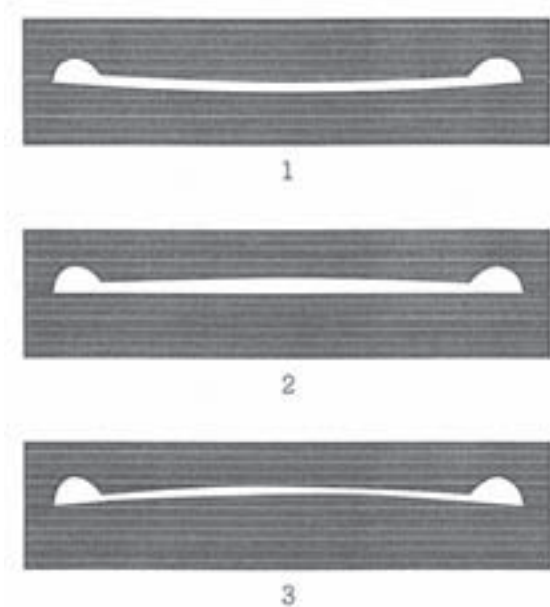
図1 多鈕鏡の鏡面形態と鑄型 （趙鎮先 2014 による）
