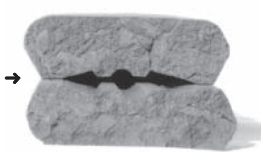
【図版6】側面の開先削り取り
