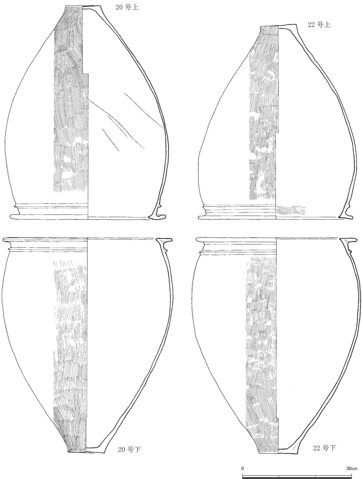
第 61 图 甕棺実測图⑨ (1/6)
