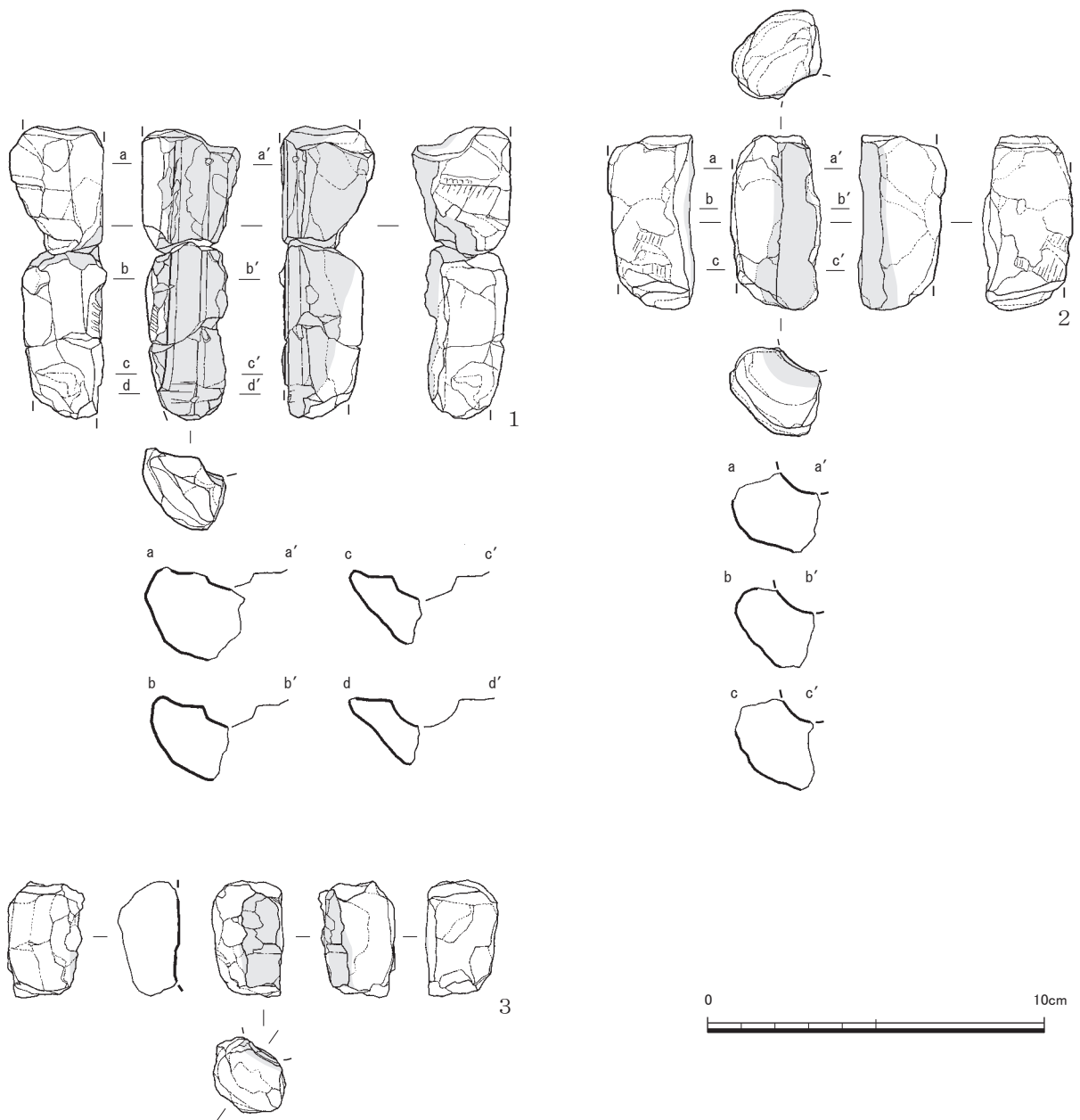
第22図 1号竪穴建物跡出土土製鑄型実測図①(1/2)
