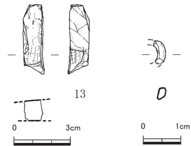
第70図 石器・ガラス小玉実測図 （1/2・1/1）
