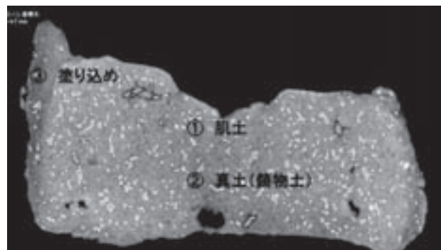
図5 土製鋳型の断面構造
