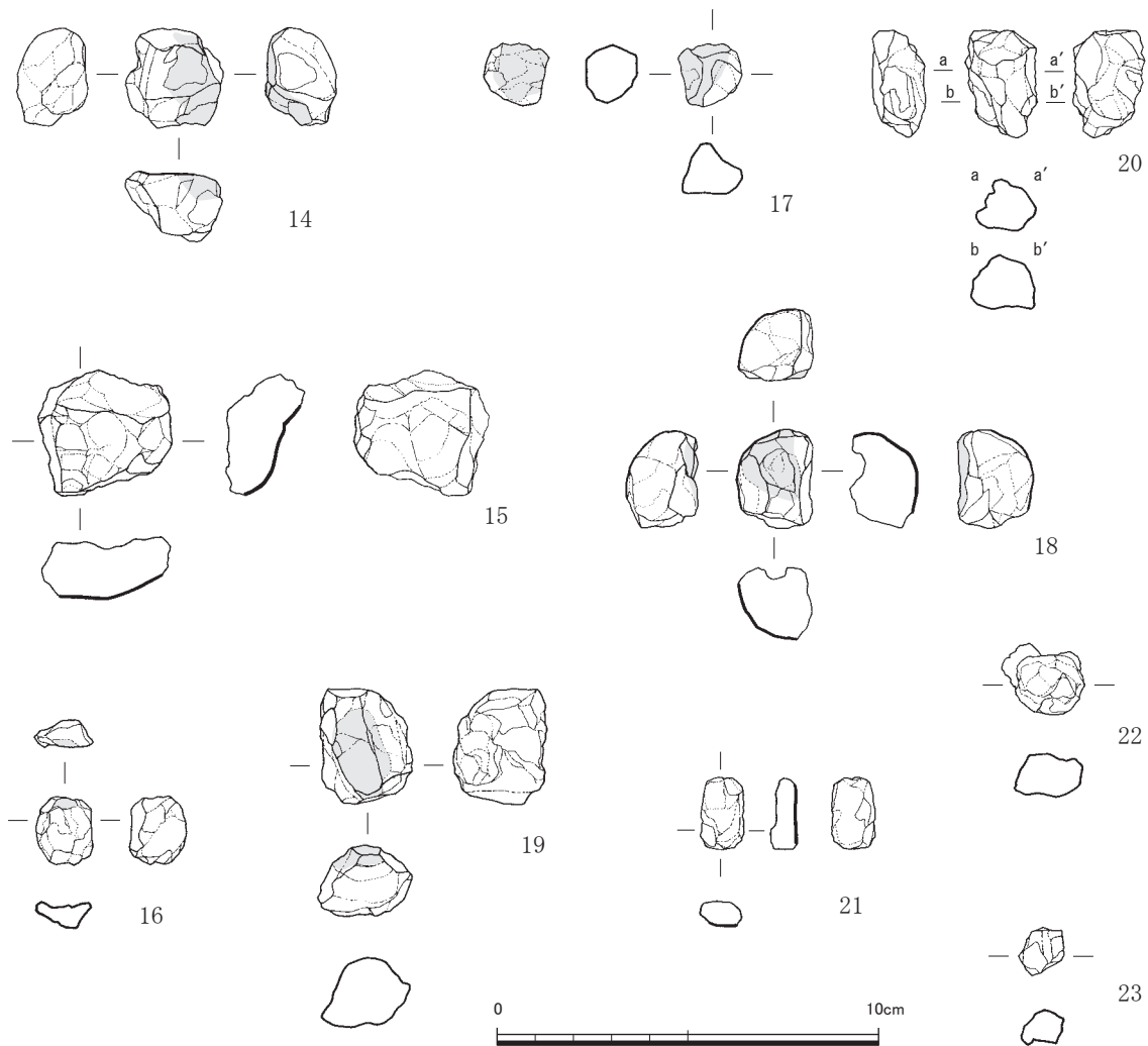
第29図 1号竪穴建物跡出土土製鑄型実測図⑧ (1/2)
