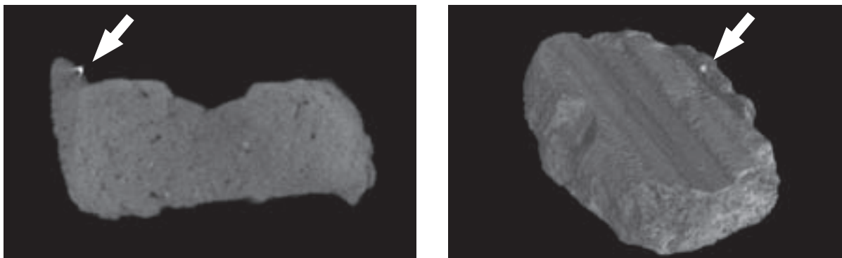
図1 鋳型（5号）の断層像（左）と三次元像（右）
