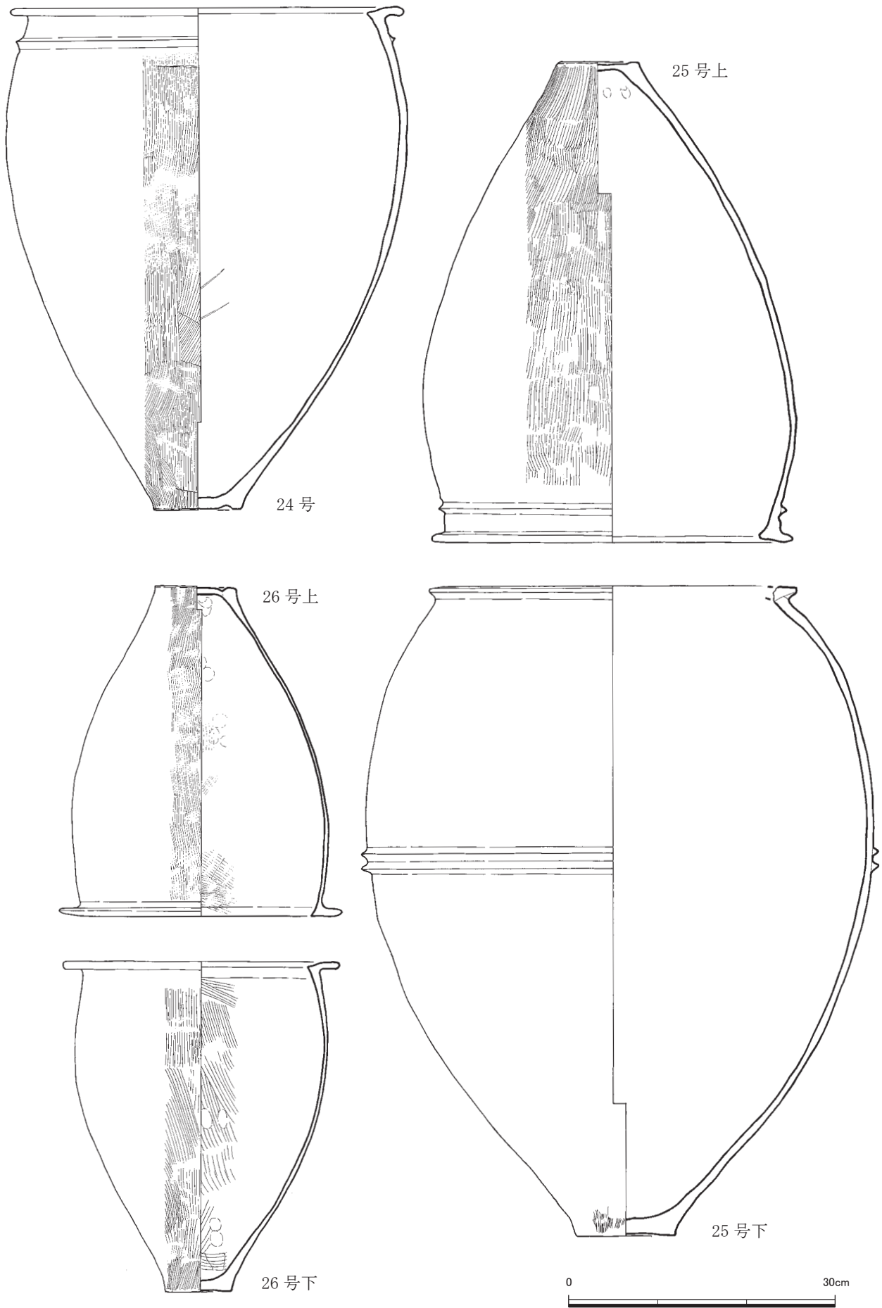
第 63 图 甕棺実測図⑪ (1/6)
