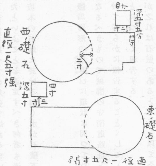
圖違相の式形の石礎の右左の門手水
