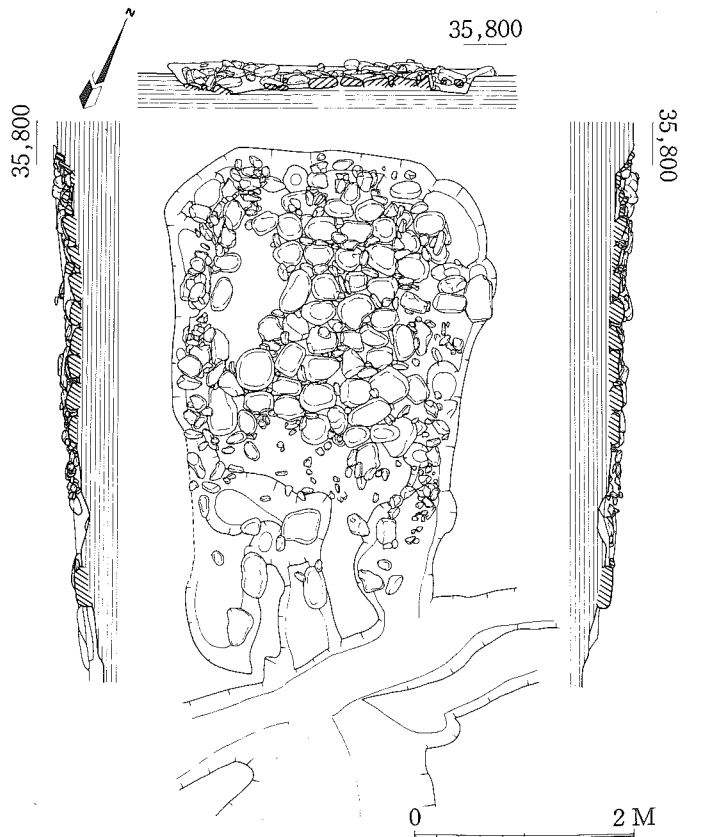
図4 6号墳主体部実測図 (S=1/60)
