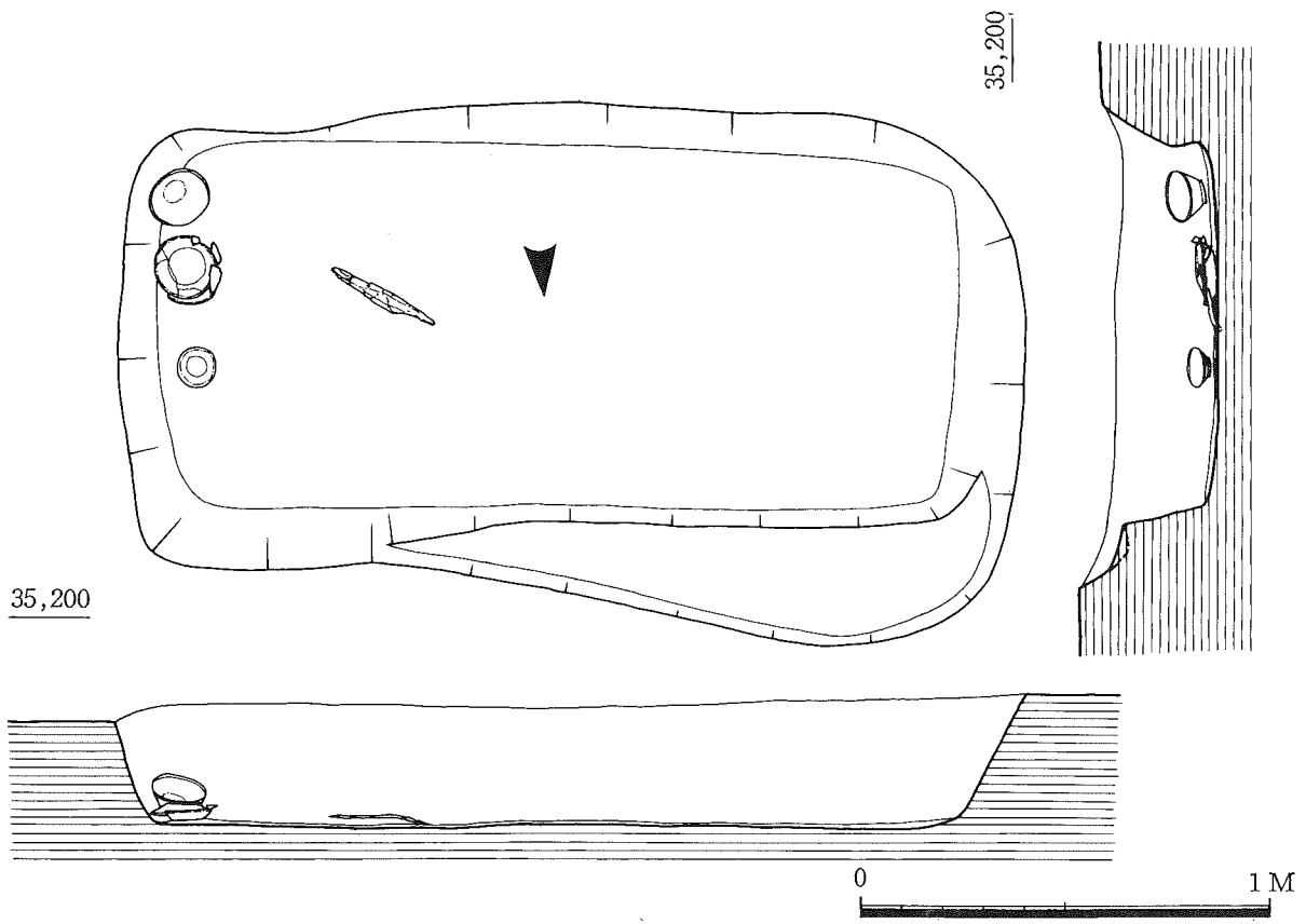
图6 2号土墳墓实测图 (S=1/20)
