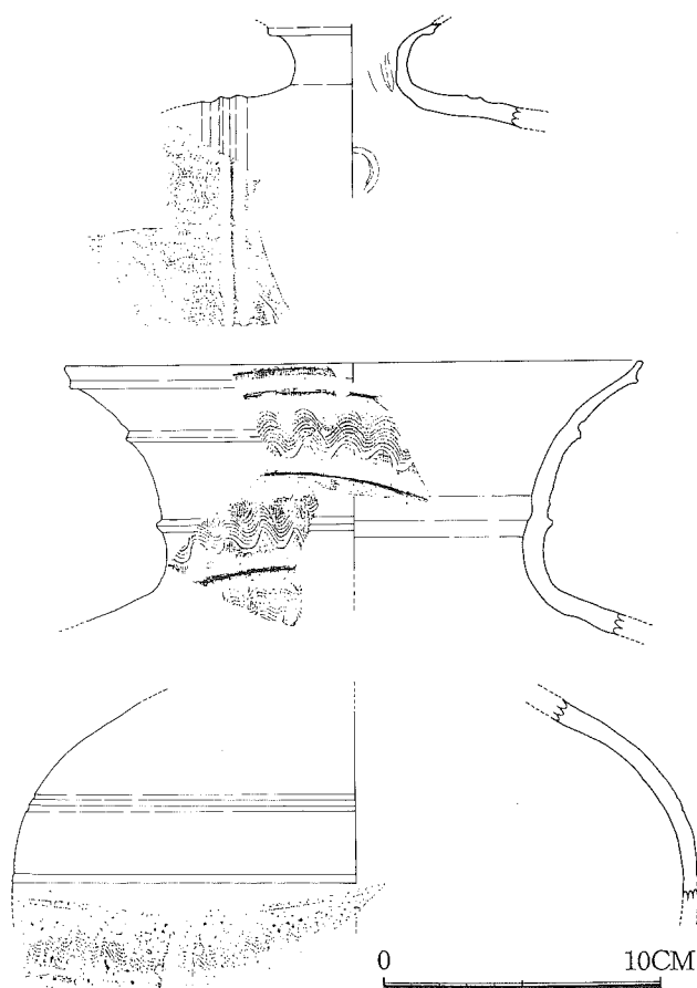
図9 1号墳周溝内出土土器実測図 (S=1/3)
