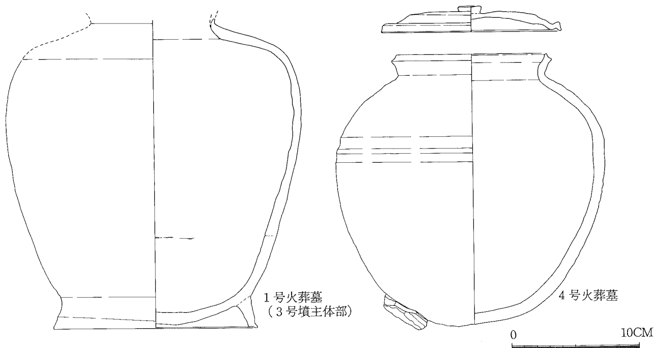
図11 1, 4号蔵骨器実測図 (S = 1 / 3)
