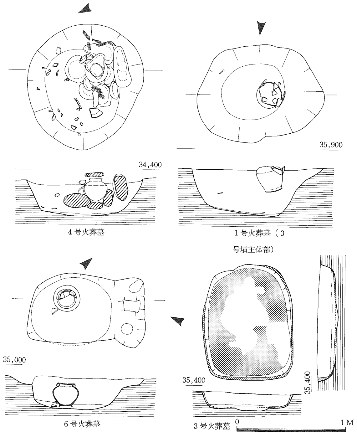
図7 火葬実測図 (S=1/20)
