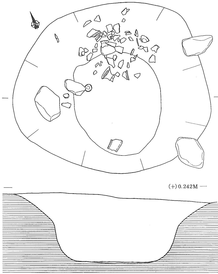
第16図 SK17 平・断面図(1 / 20)
