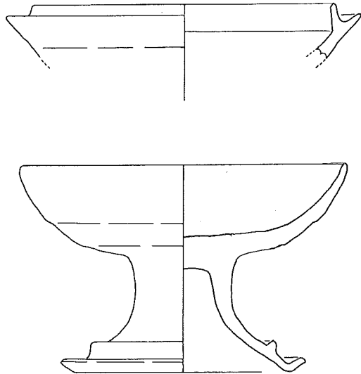
第4図 SB2 出土土器実測図 (1/2)
