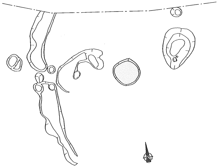
第13図 SB8 平面図 (1/30)
