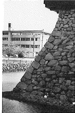
本丸石垣 縫い隅勾配の状況
