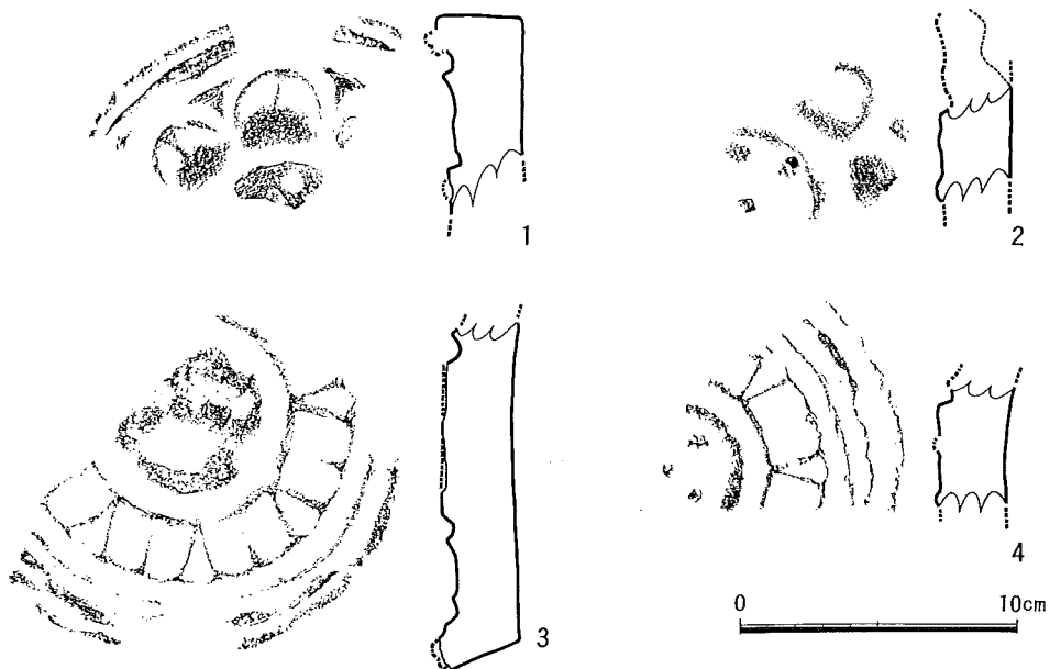
図8 相原廃寺B地区出土軒丸瓦実測図 (S=1/3)
