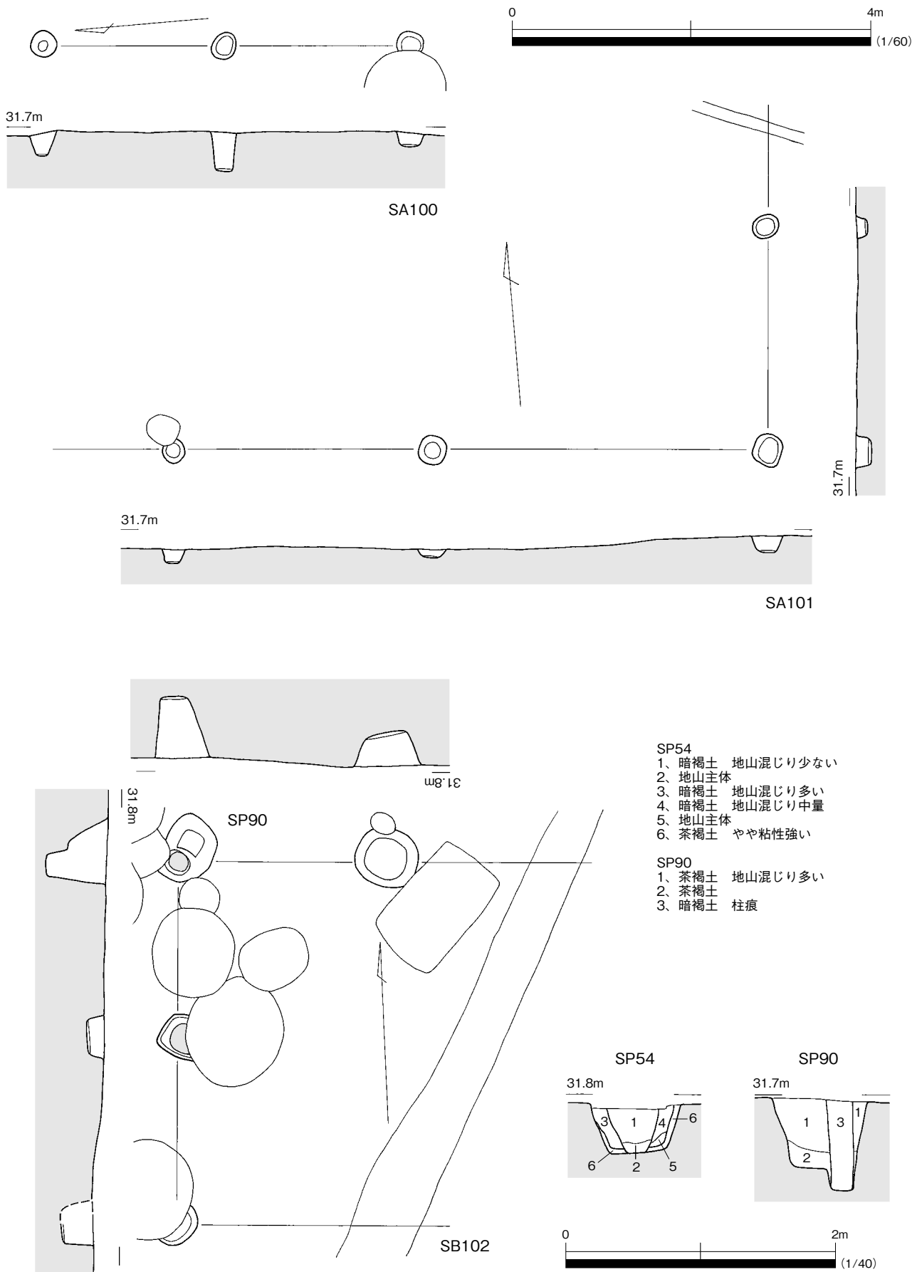
Fig.25 建物・柵列の可能性のある柱穴列①(1/40・1/60)
