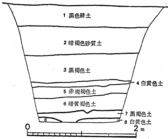
第8図 D-7 区西壁土層図
