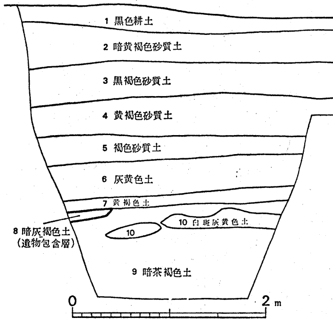
第6図 C-5区北壁土層図
