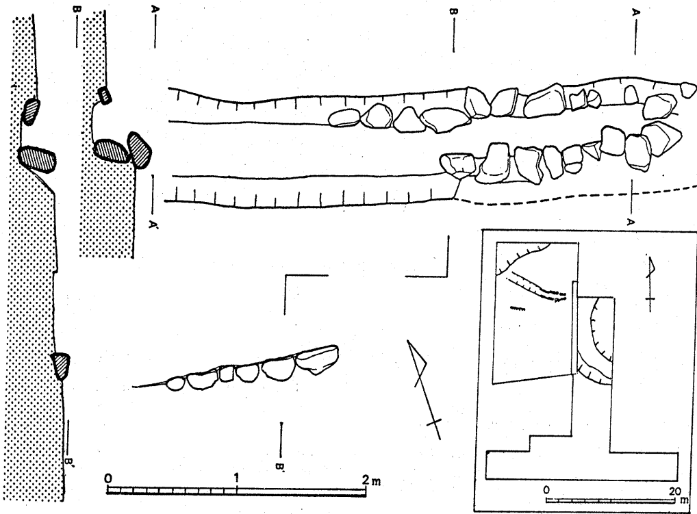
第4図 Aトレンチ遺構実測図
