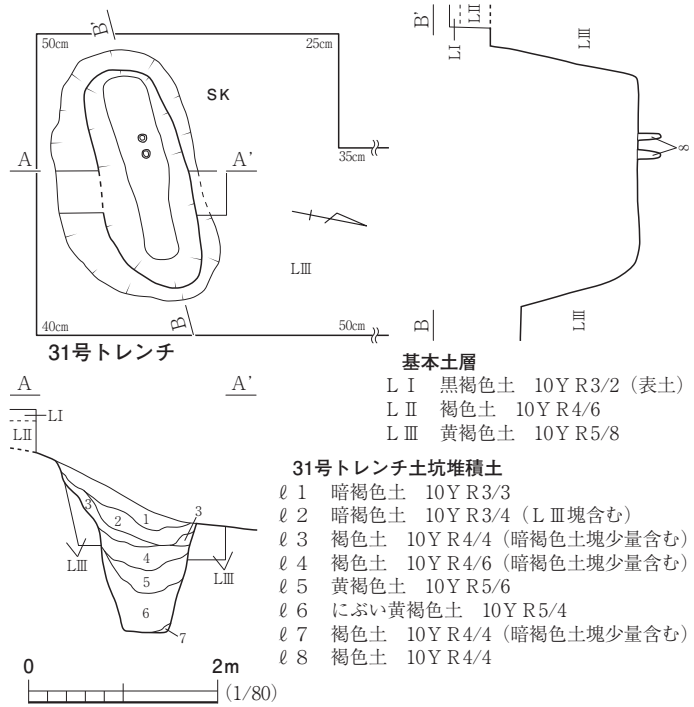
図18 SM-B⑮検出遺構
