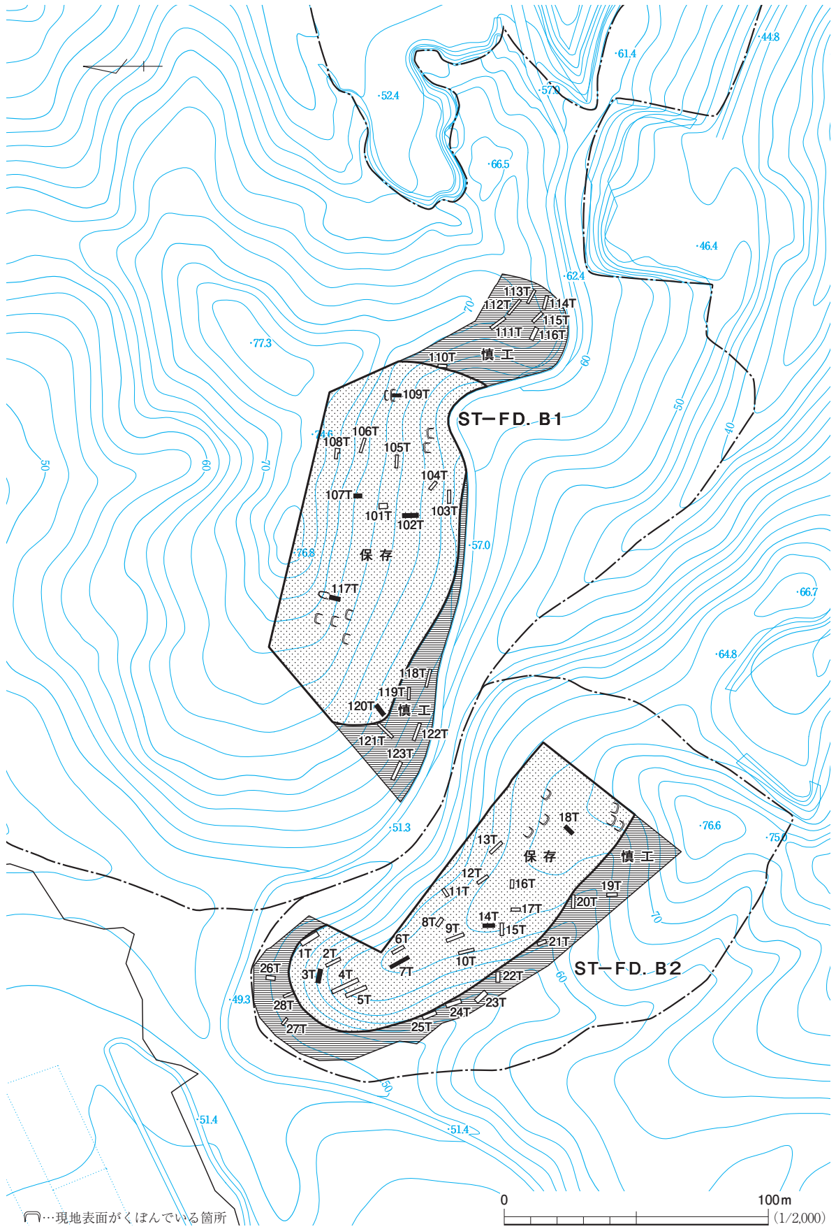
図31 ST-FD. B1・ST-FD. B2トレンチ配置図
