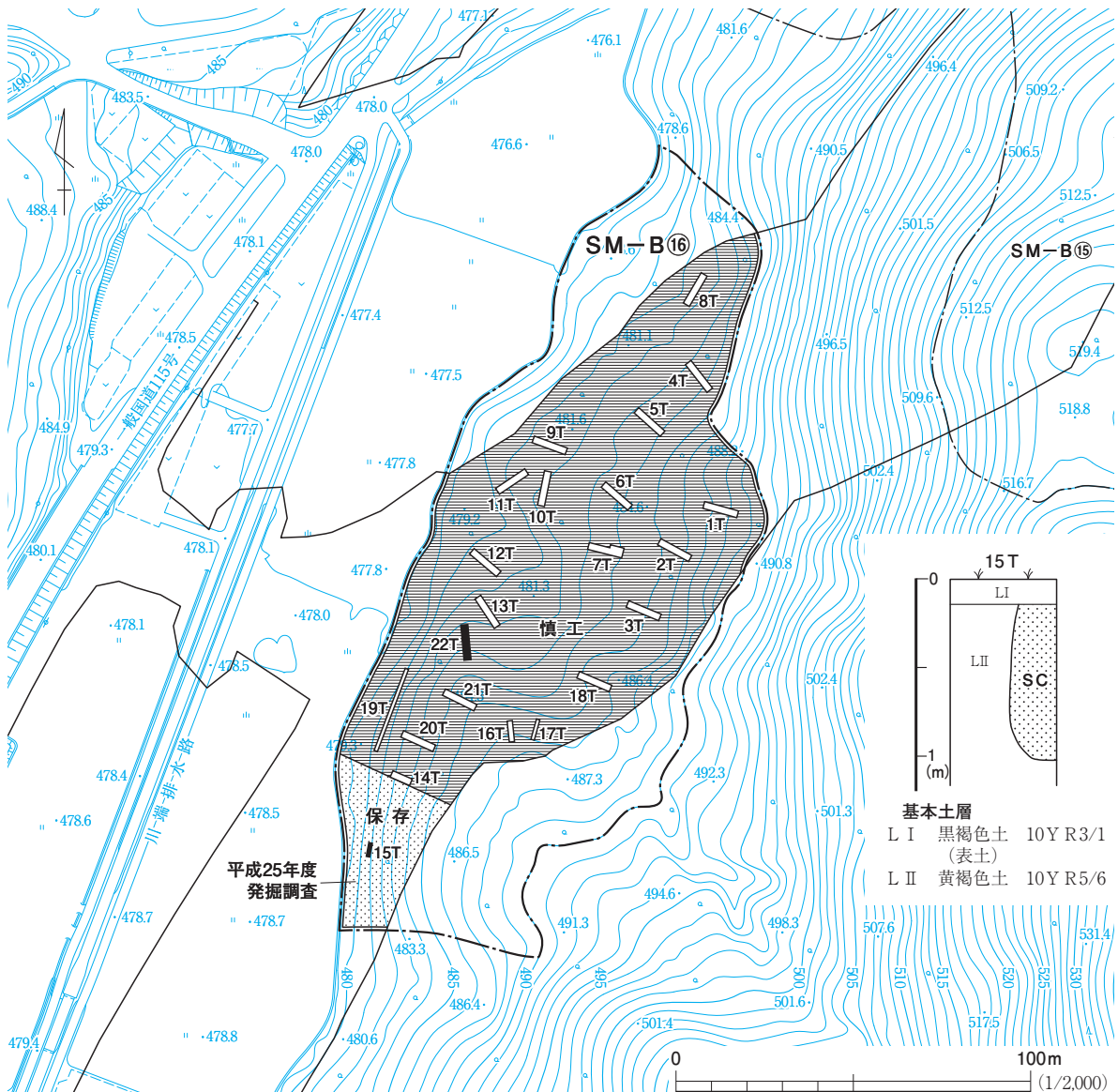
図19 SM-B⑩トレンチ配置図・土層柱状図
