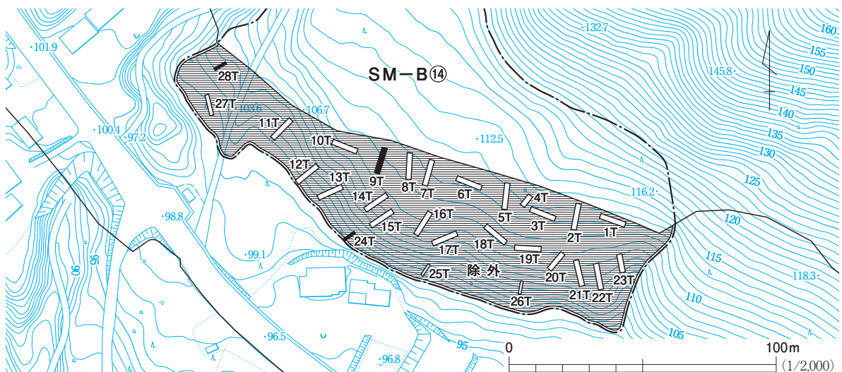
図16 SM-B⑭トレンチ配置図
