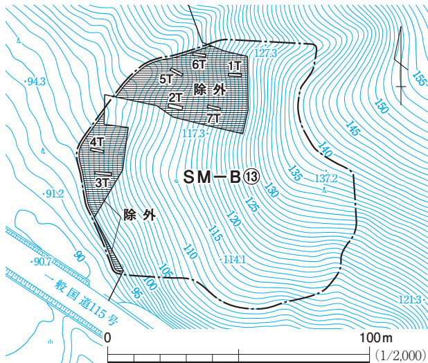
図15 SM-B⑬トレンチ配置図
