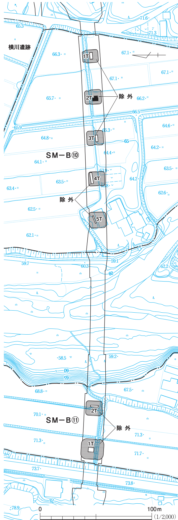
図14 SM-B⑩・B⑪トレンチ配置図
