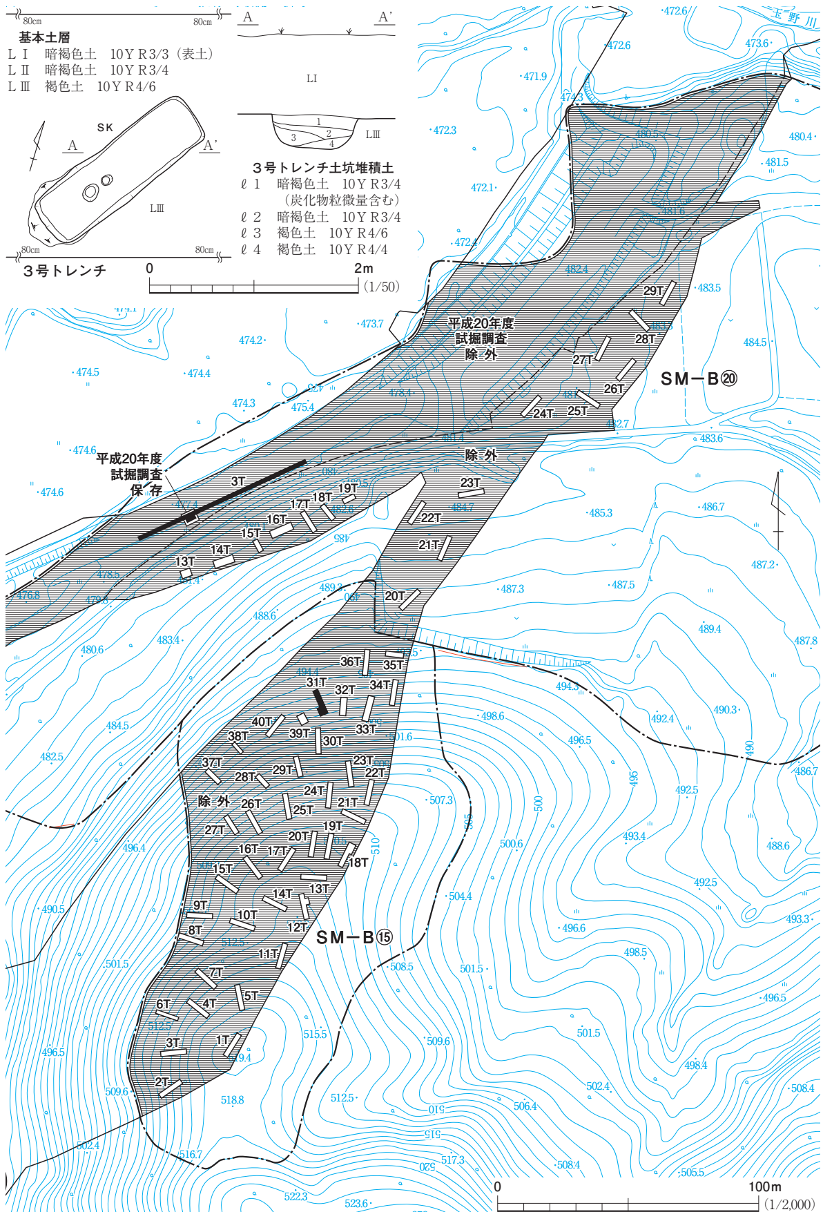
図17 SM-B⑳トレンチ配置図・検出遺構, SM-B⑮トレンチ配置図
