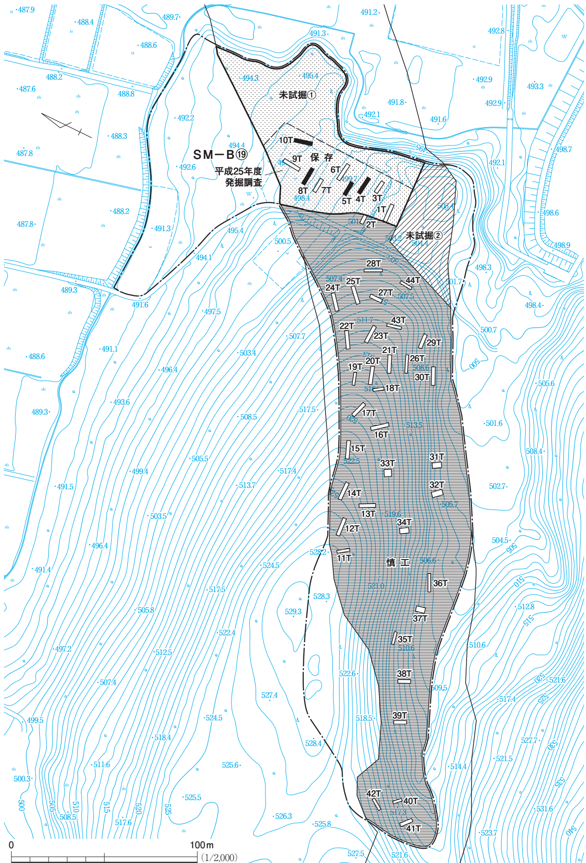
図21 SM-B(19)トレンチ配置図
