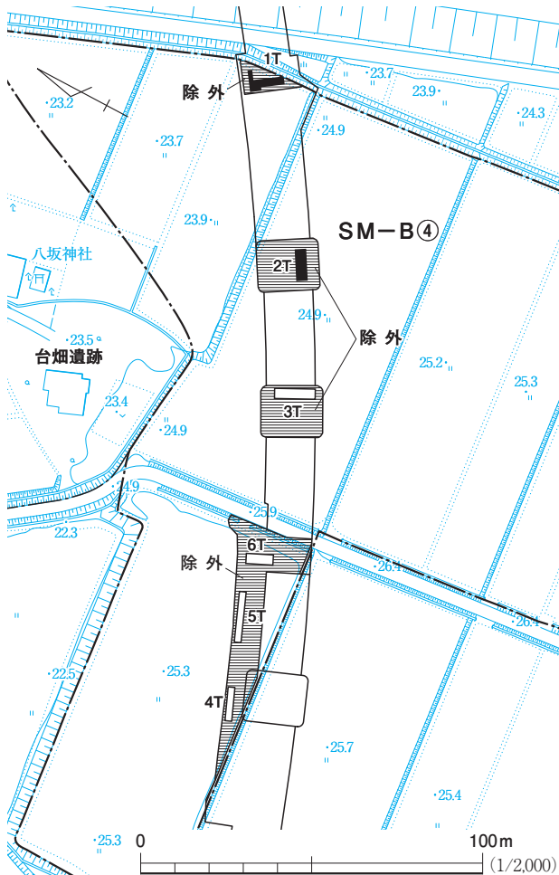
図11 SM-B④トレンチ配置図
