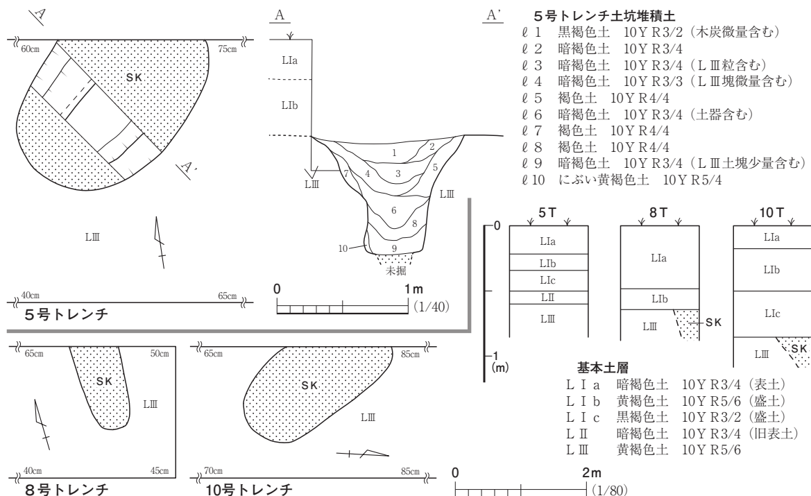
図22 SM-B⑱検出遺構・土層柱状図
