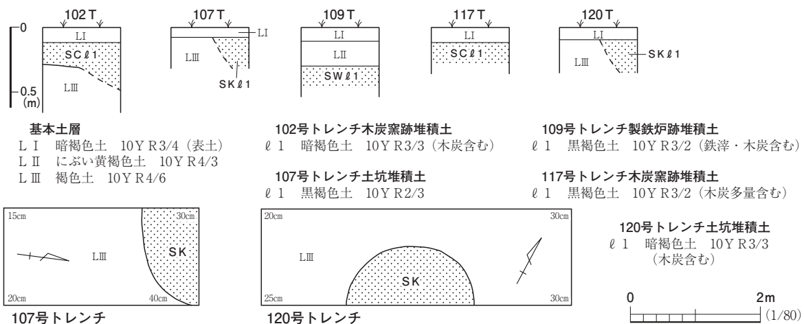
図32 S T-F D. B 1 検出遺構・土層柱状図
