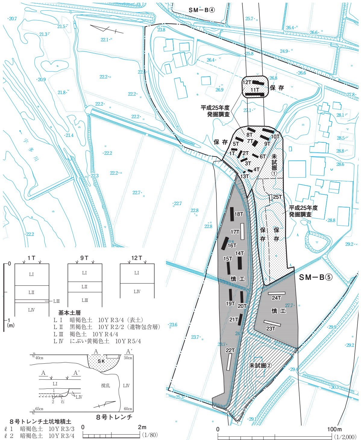
図12 SM-B⑤トレンチ配置図・検出遺構・土層柱状図
