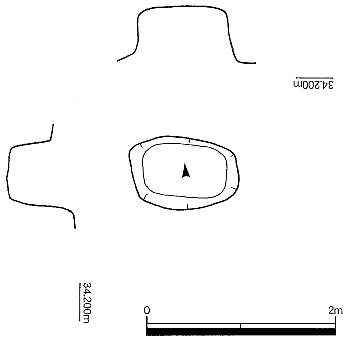
第5図 土坑図 (S=1/40)
