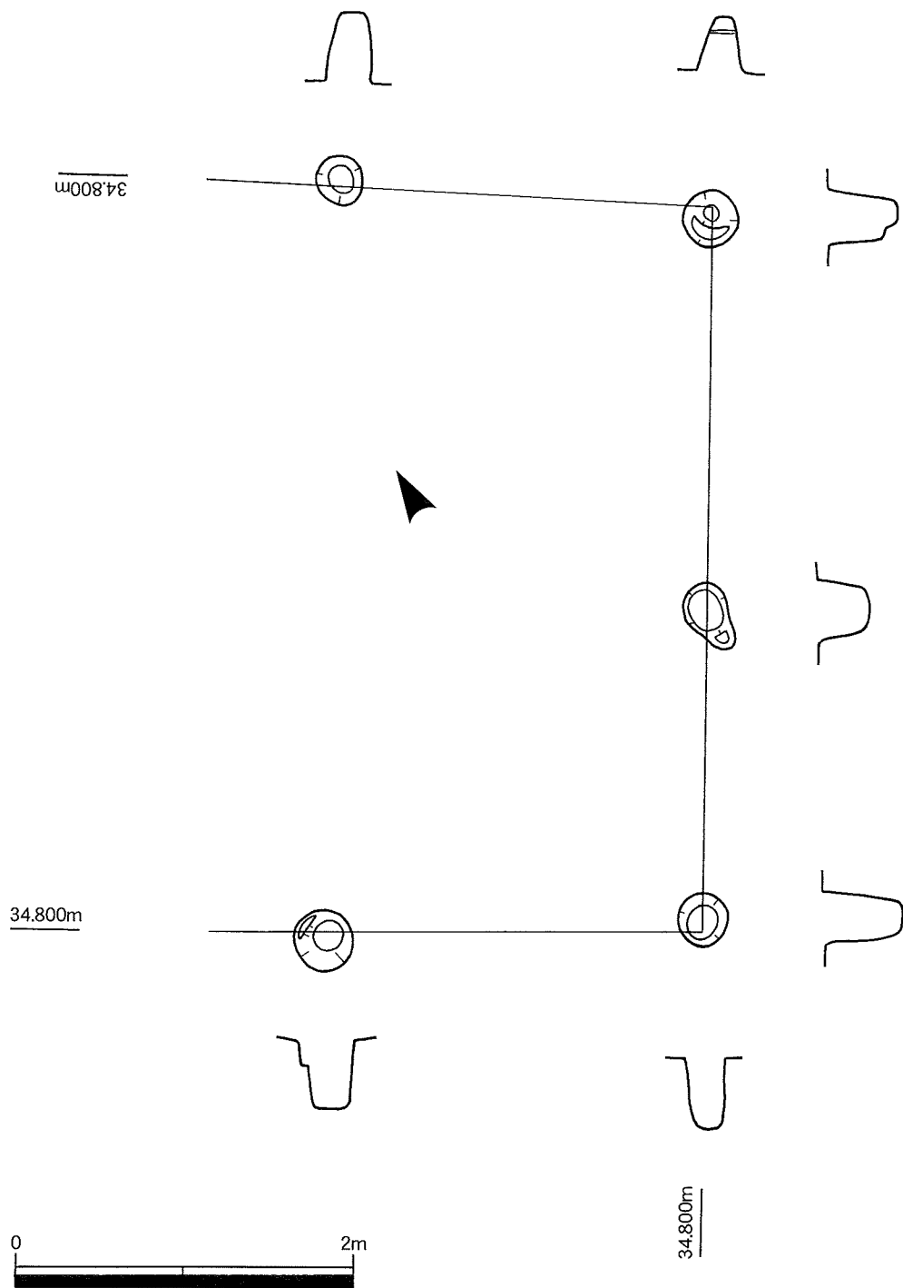
第6図 掘立柱建物図 (S=1/40)
