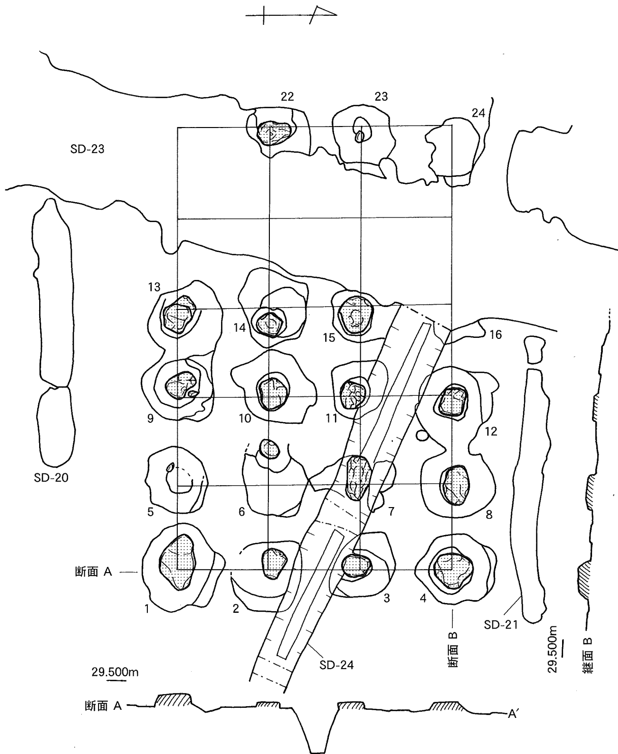
第5図 SB-13平面図・断面図 (S=1/100)
