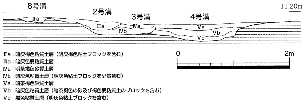
第7図 2号～4号・8号溝土層断面図 (縮尺1/40)
