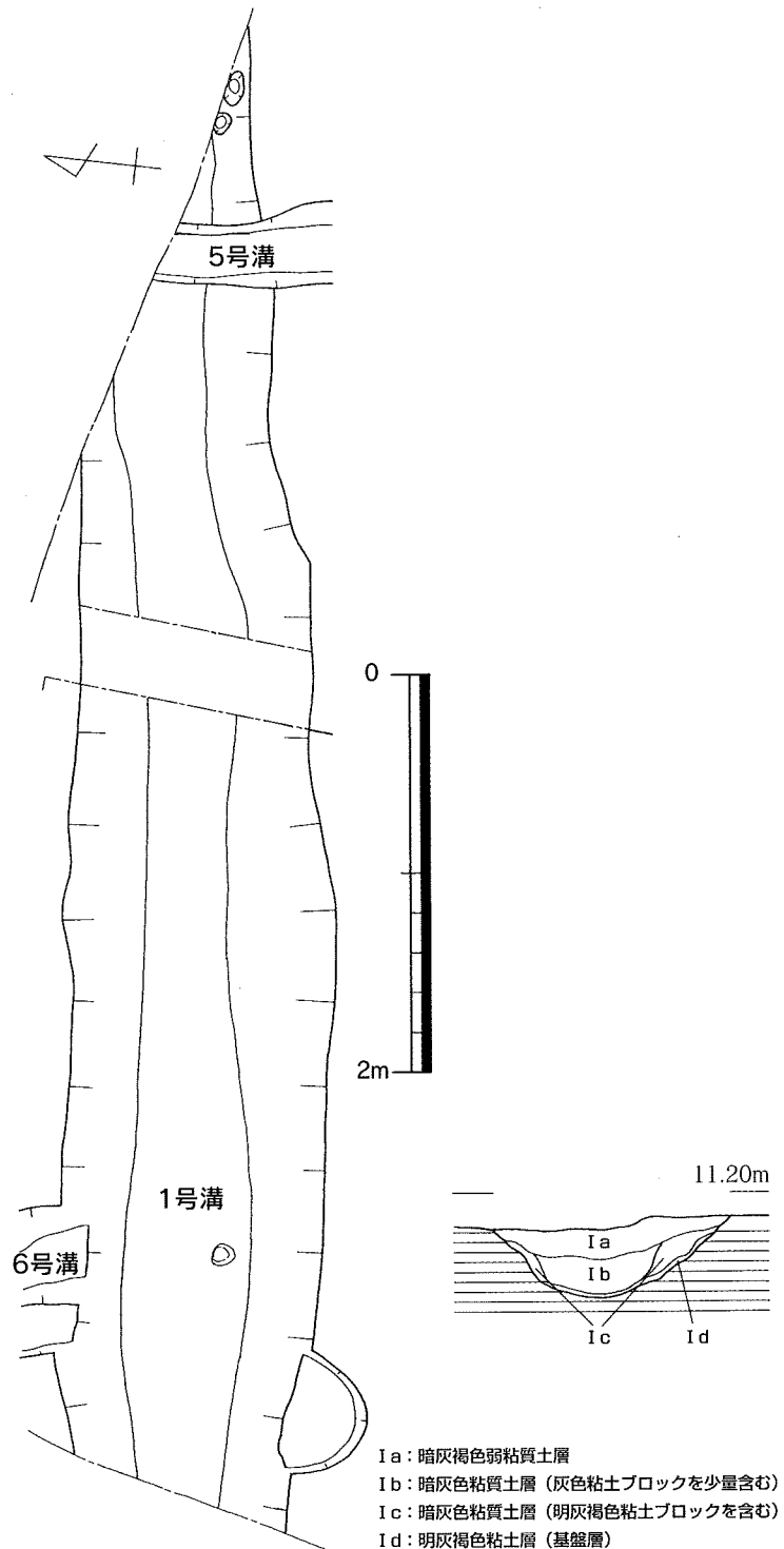
第5図 1号溝実測図（縮尺1/40）
