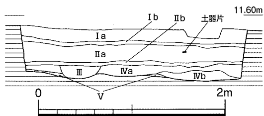
第13図 北区南壁土層断面図(縮尺1/40)
