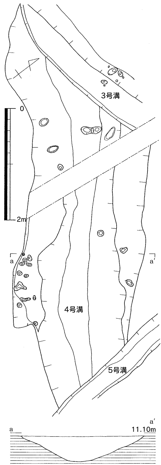
第9図 4号溝実測図 (縮尺1/40)
