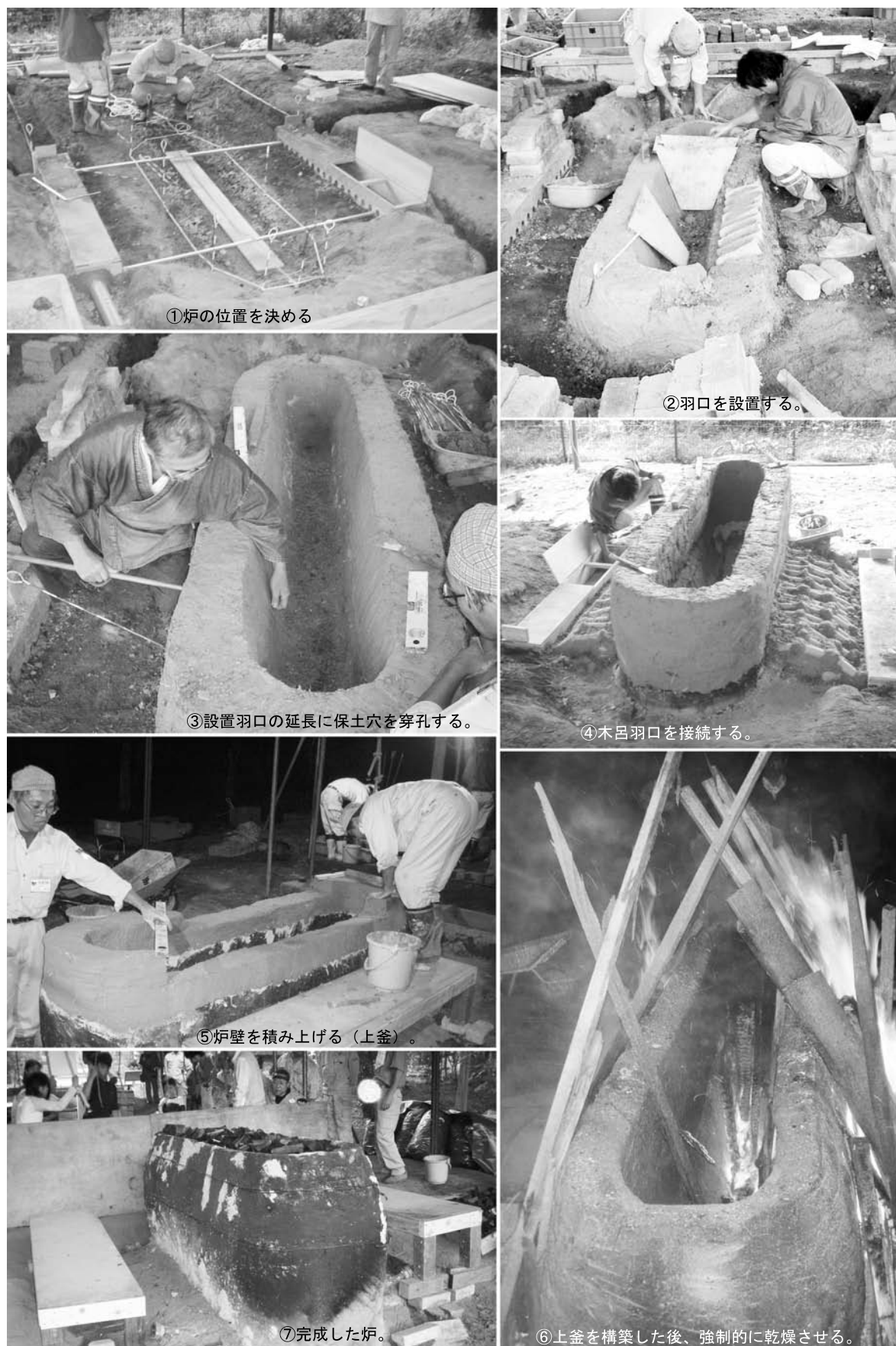
写真5 プレ操業炉構築
