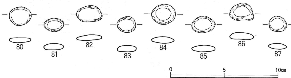
第14図 出土遺物実測図⑤
