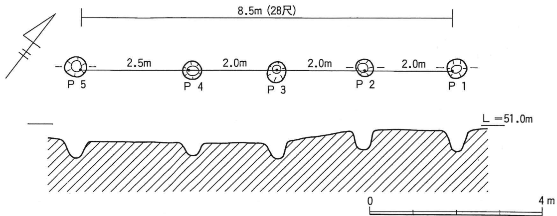
第8図 検出遺構実測図① (杭列)
