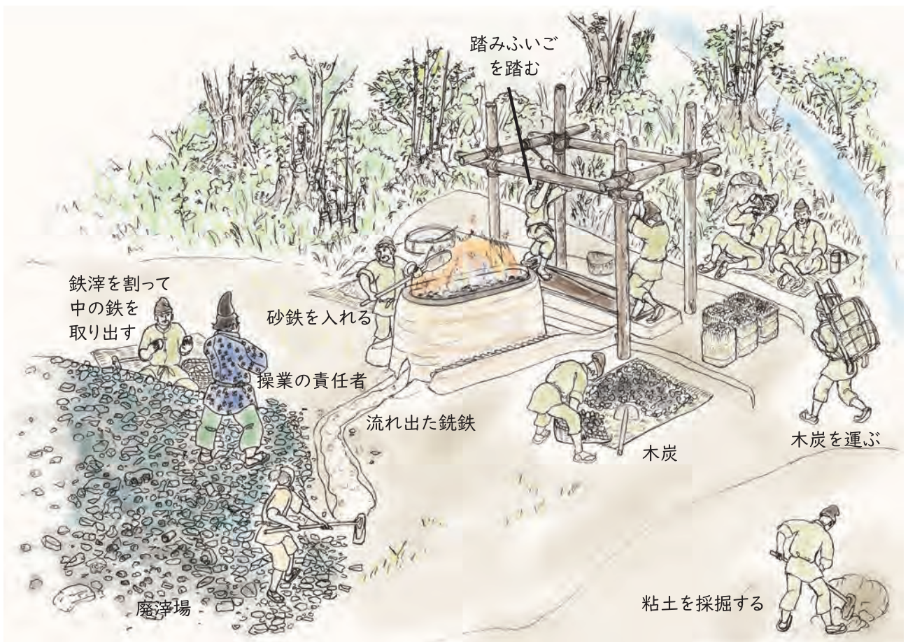
箱形炉の操業の様子（9世紀中葉頃）
