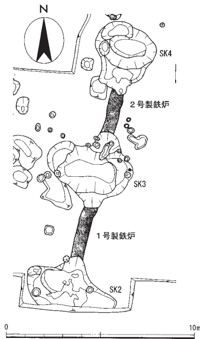
平津池ノ下遺跡 1号・2号製鉄炉 (平津池ノ下型 1/200)
