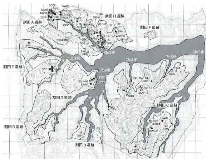
図7 割田地区製鉄遺跡群
