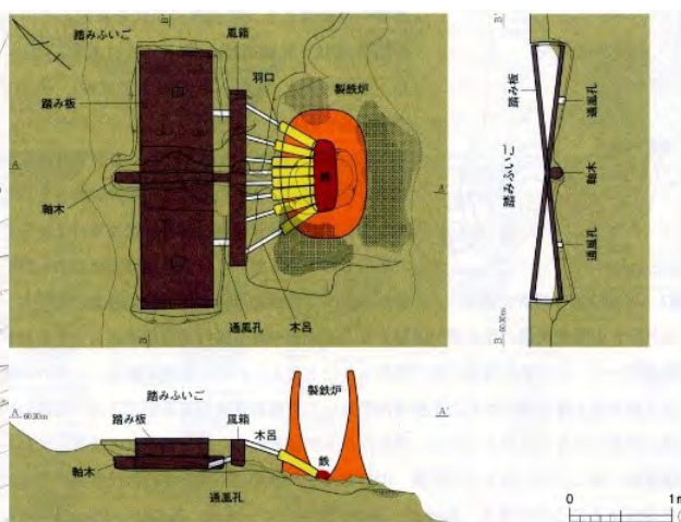
図14 南狼沢A遺跡1号製鉄遺構復元図
