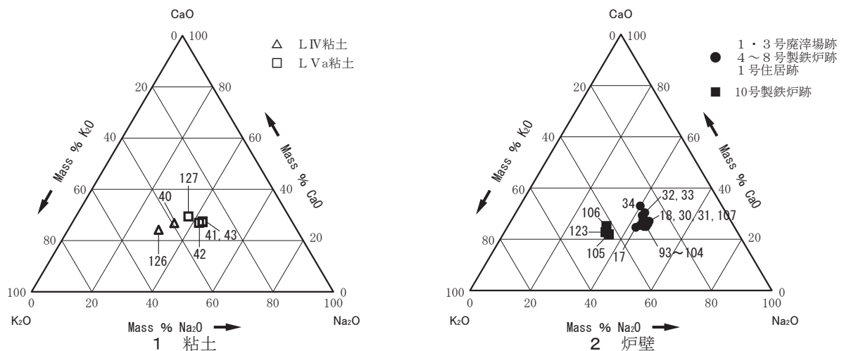
図6 横大道製鉄遺跡の炉壁胎土分類(板谷2010)
