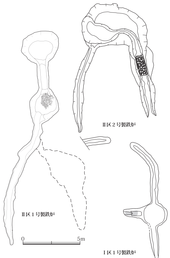
図6 峯山遺跡の箱形炉
