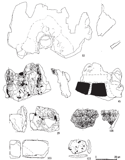
図8 鍛冶屋敷遺跡出土炉壁
