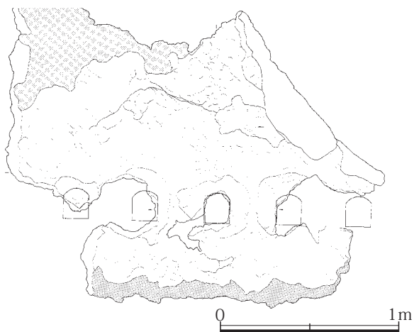
図8 峯山遺跡I区1号製鉄炉出土炉壁
