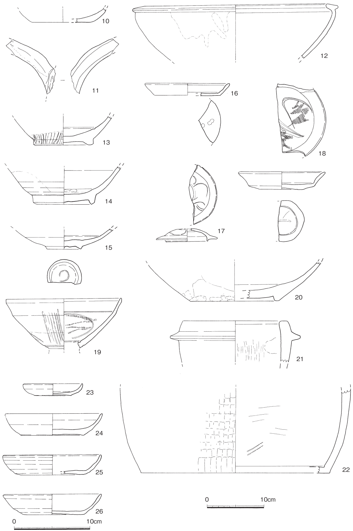
第8図 SK13・27出土遺物 (21・22は1/4、その他は1/3)
