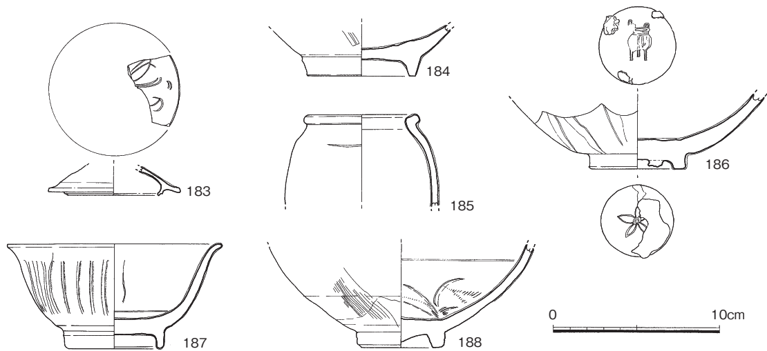
第26図 第2層包含層出土遺物実測図(2)(1/3)
