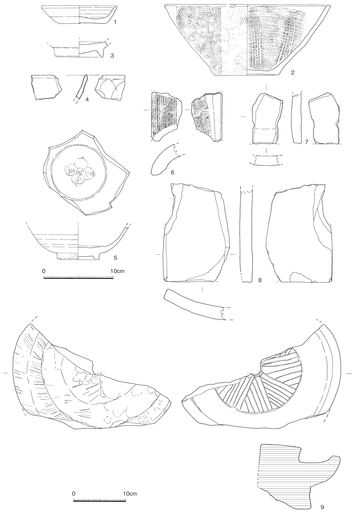
第7図 SK10出土遺物 (2・6～9は1/4、その他は1/3)
