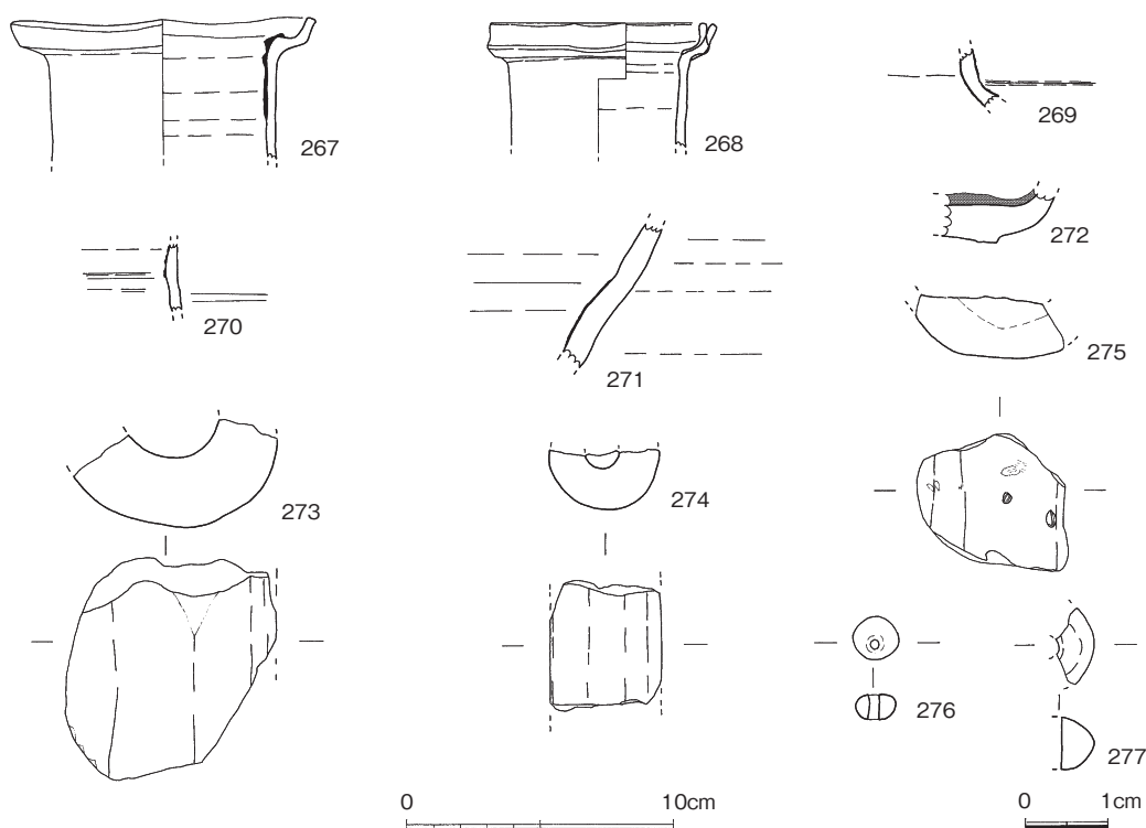
第42図 ガラス製作関連遺物・ガラス製品・鑄造関連遺物実測図 (1/1、1/3)
