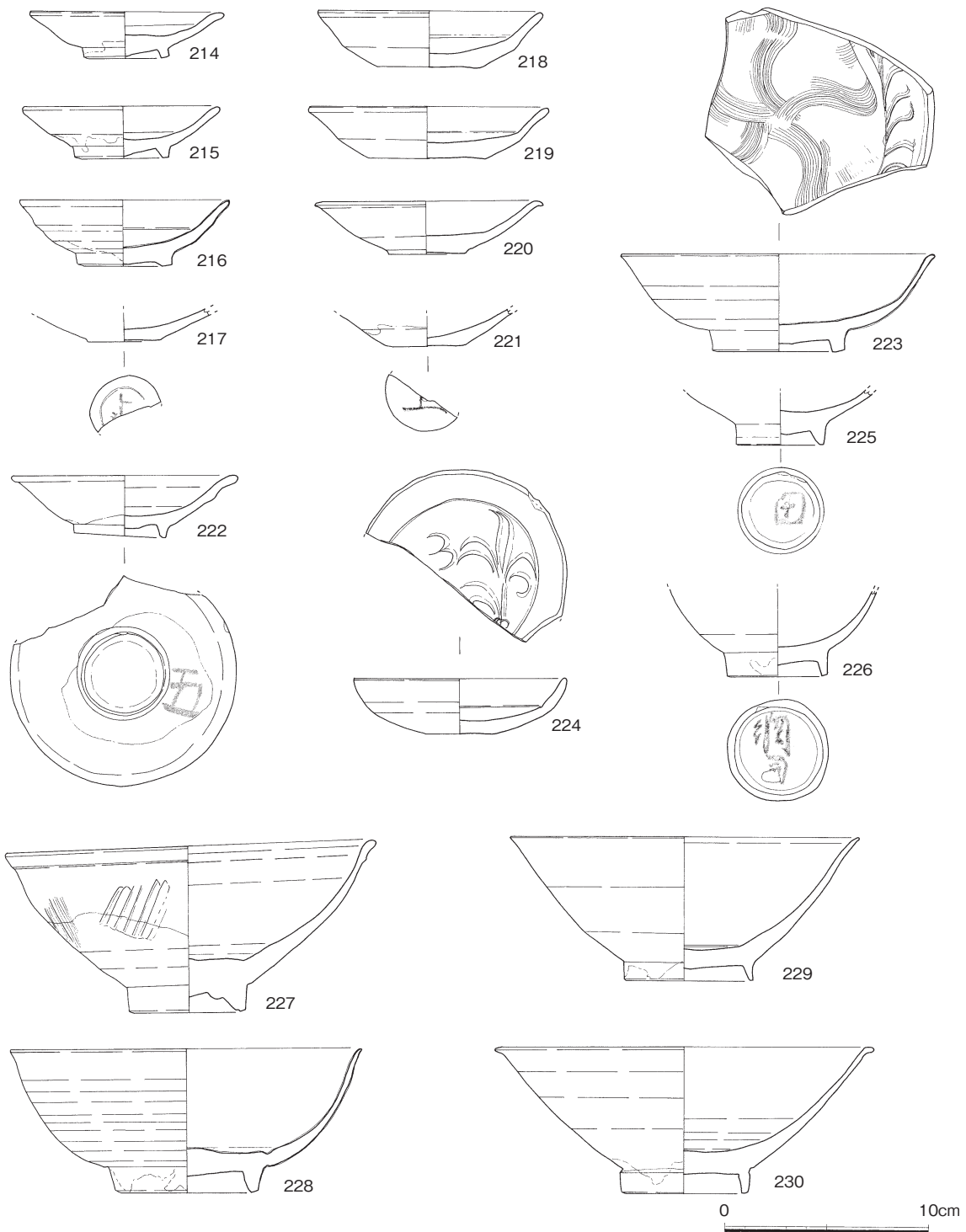
第31図 SD74出土遺物実測図(3)(1/3)
