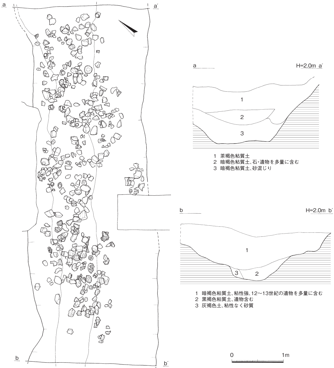
第28図 SD74実測図 (1/40)
