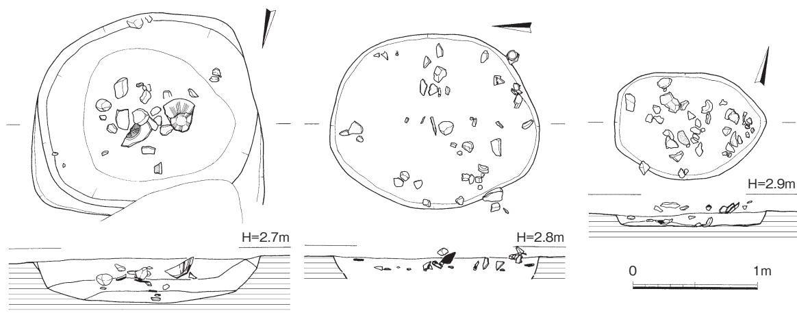
第6図 SK10・13・27実測図(1/40)
