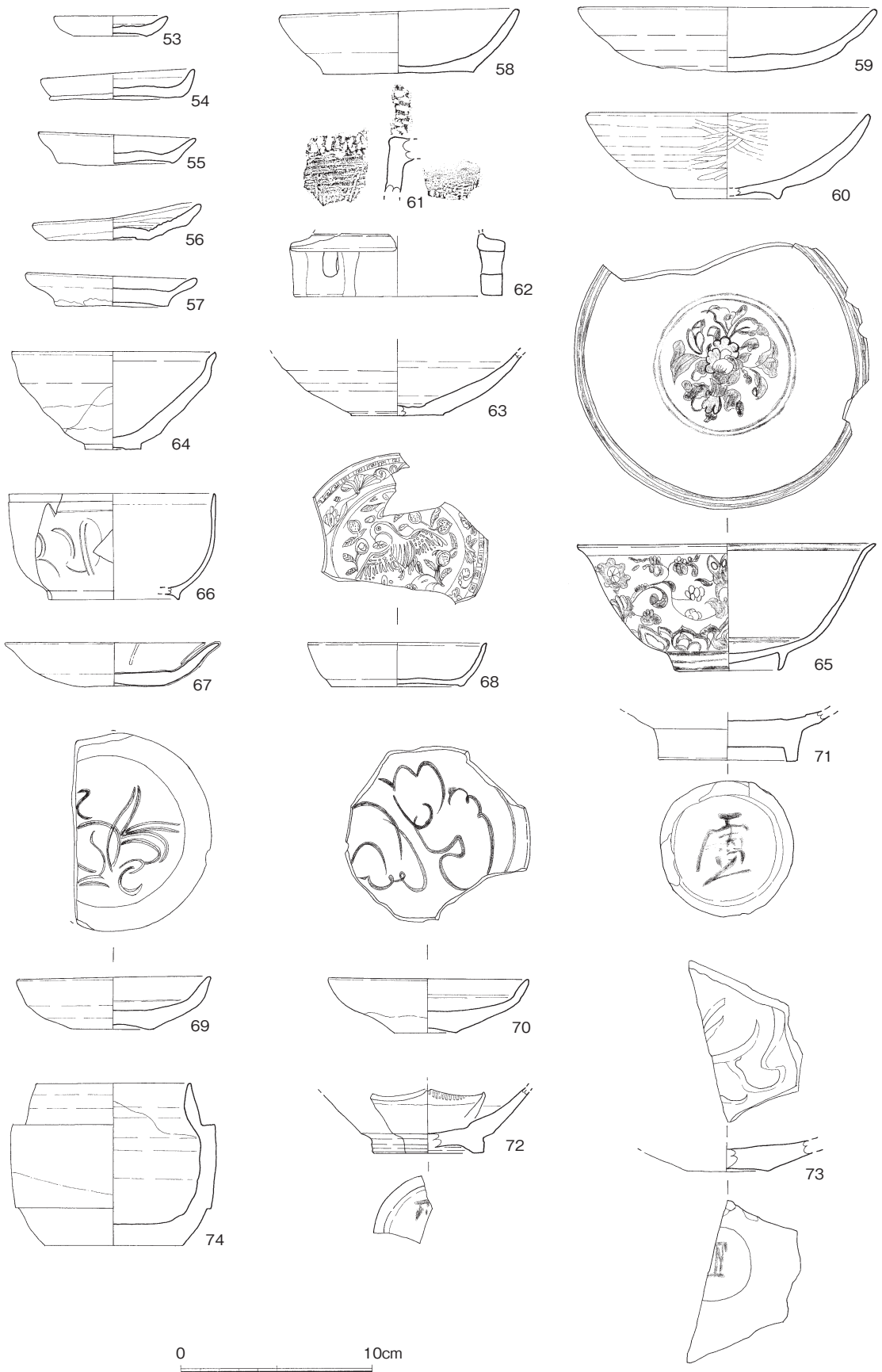
第11图 第1面包含层出土遗物 (1/3)
