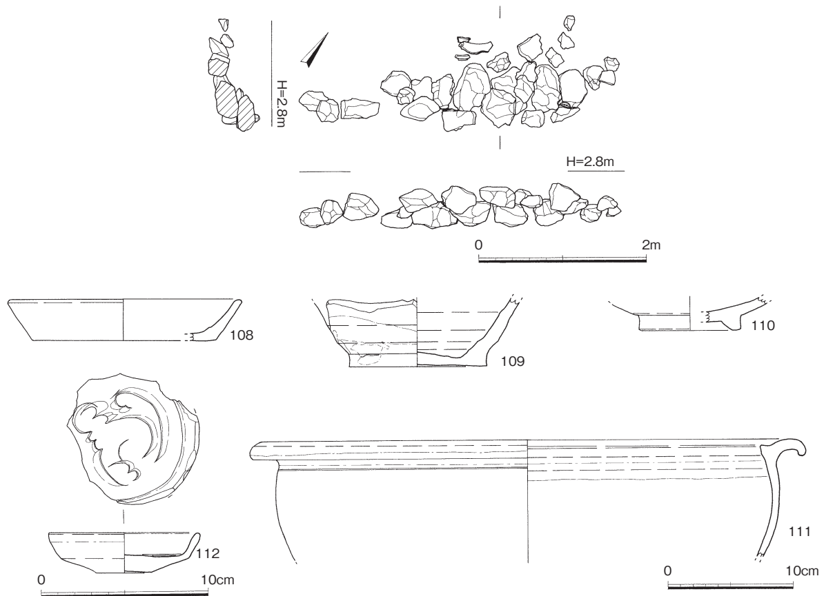
第18図 SX72実測図 (1/30) および出土遺物実測図 (111は1/4、その他は1/3)
