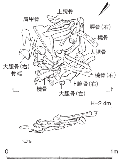
第36図 SX78実測図 (1/20)
