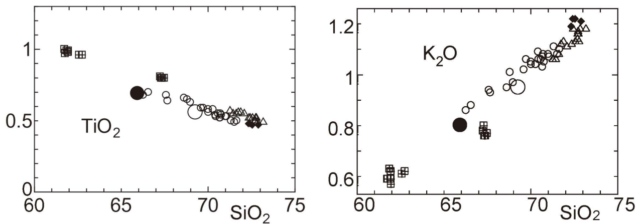
図9 軽石B及び軽石Cの全岩化学組成
