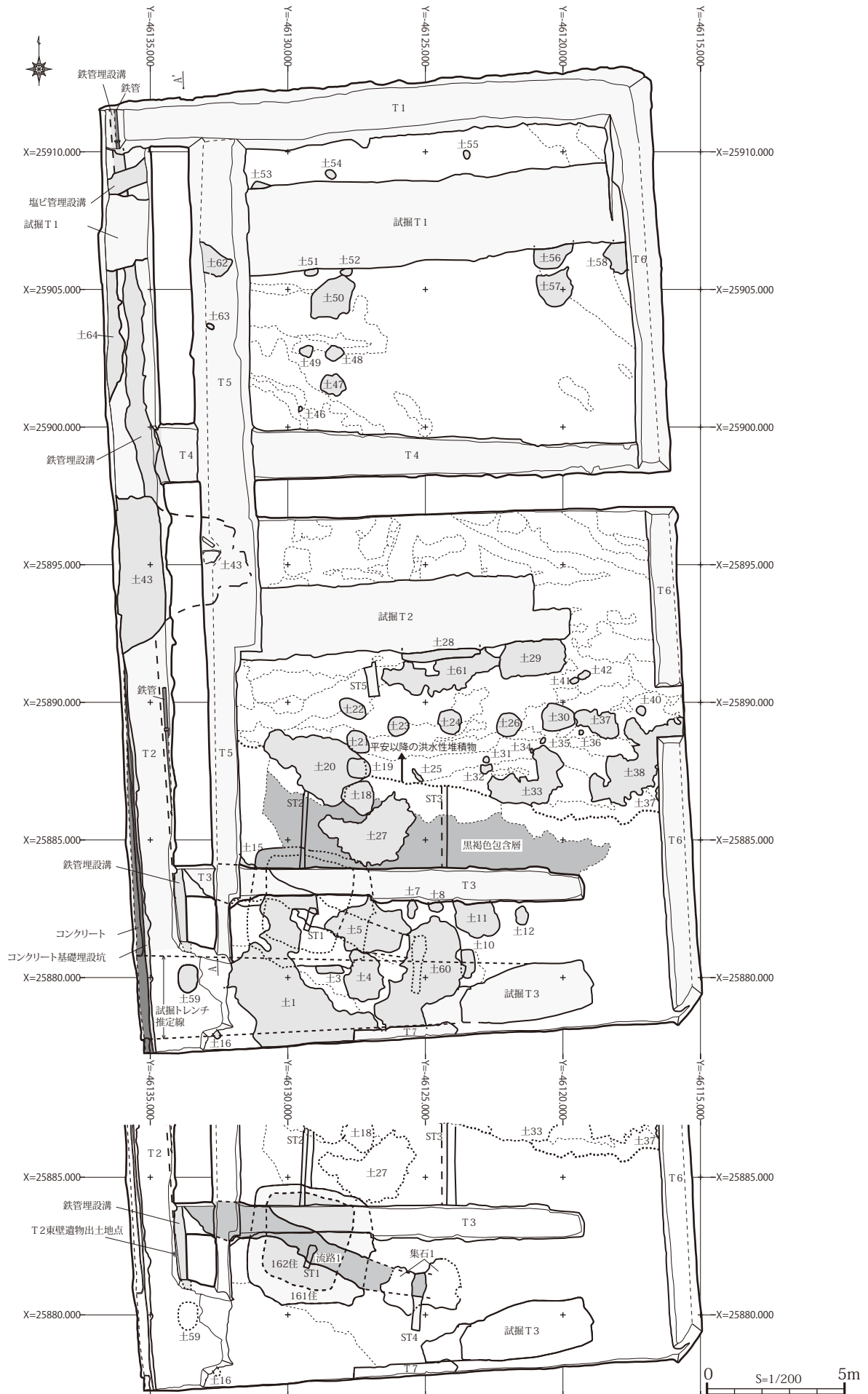
第4図 県町遺跡第15次調査全体図(下: 竪穴建物址周辺図)
