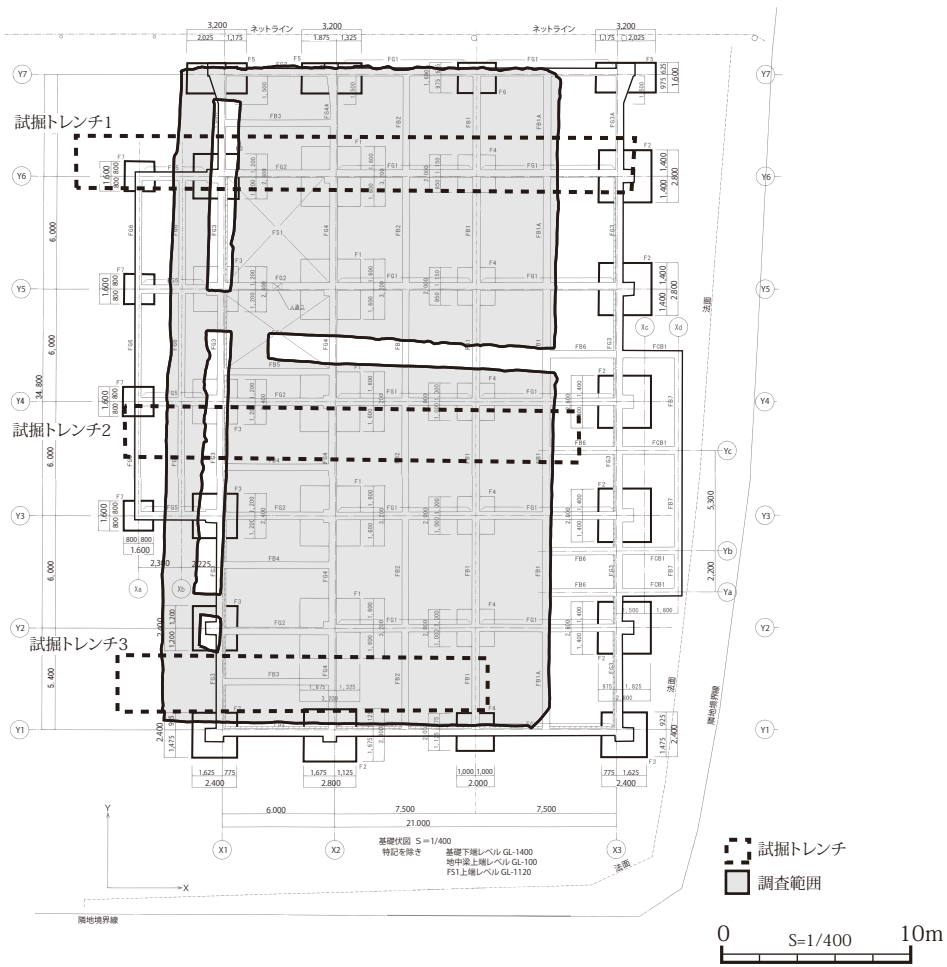
第2図 調査範囲
