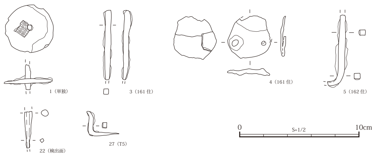
第9図 金属製品実測図
