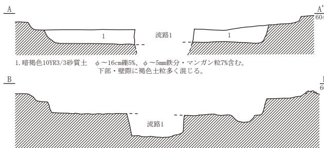
第6図 遺構実測図
