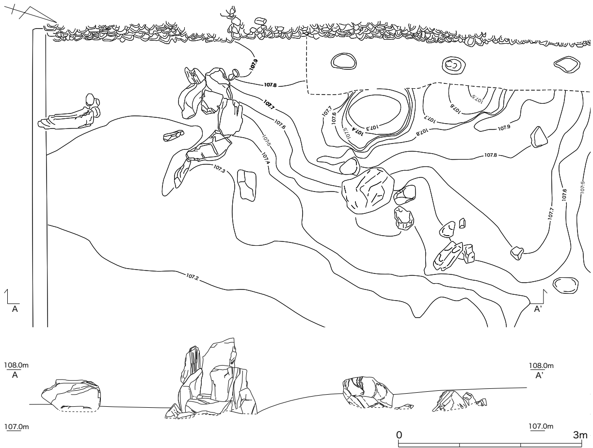
Fig.55 庭園遺構詳細図
