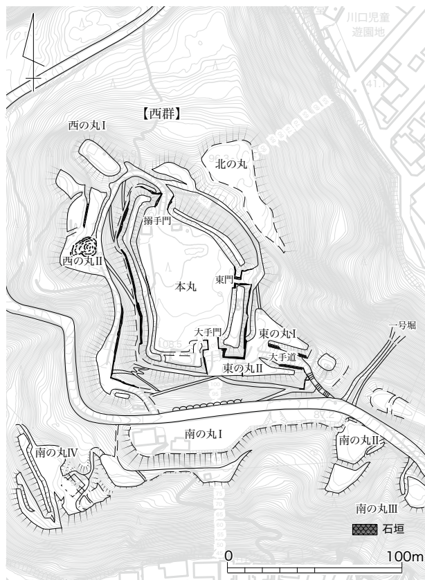
Fig.35 鳥羽山城における石垣配置図
