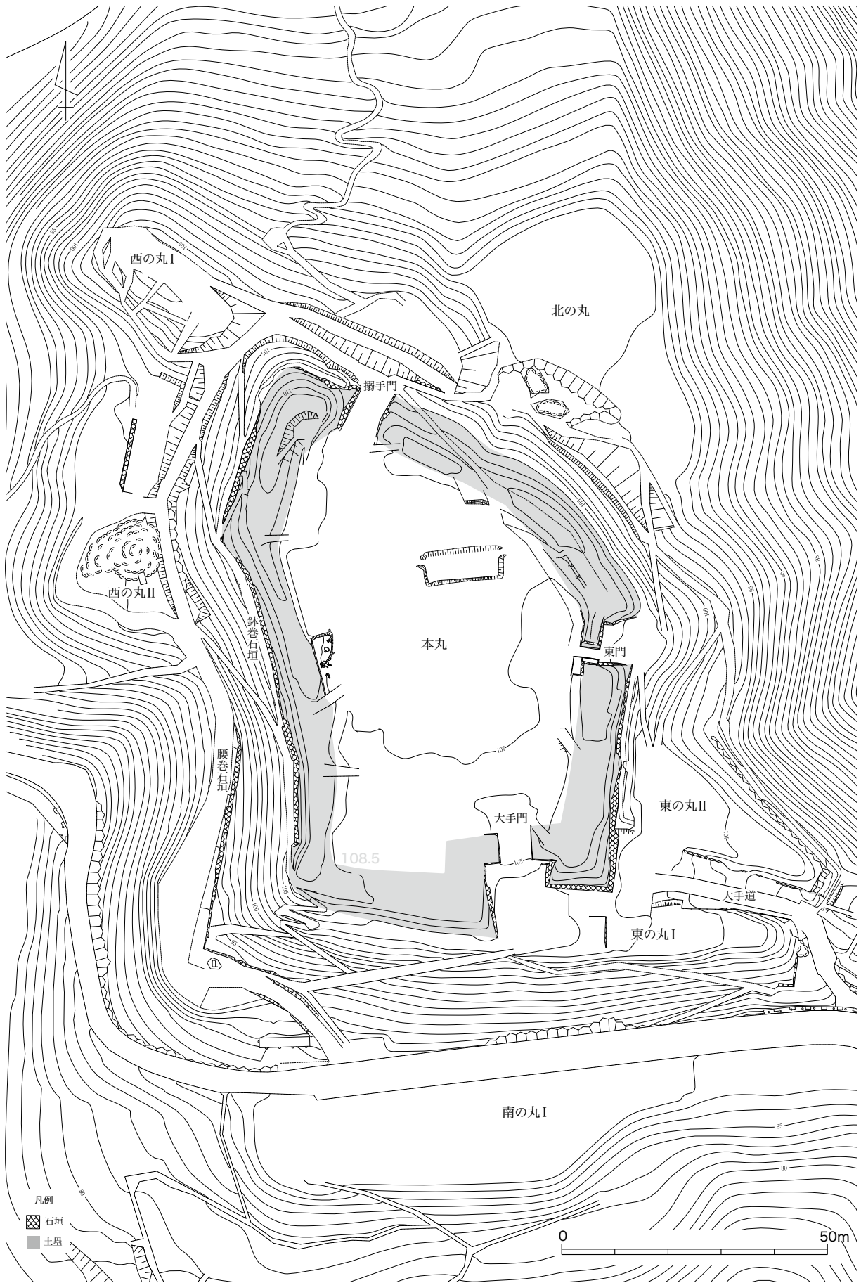
Fig.40 鳥羽山城跡遺構復元図 (拡大図)
