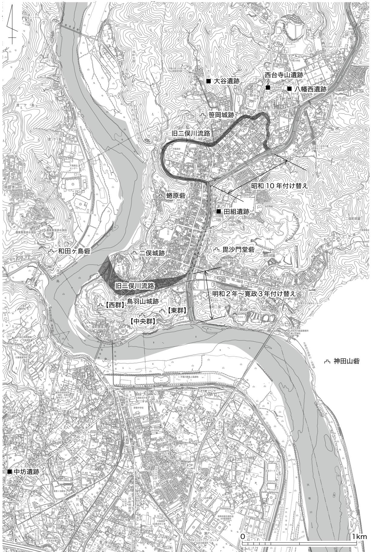
Fig.9 二侯城跡・鳥羽山城跡の位置と周辺城郭関連遺跡分布図
