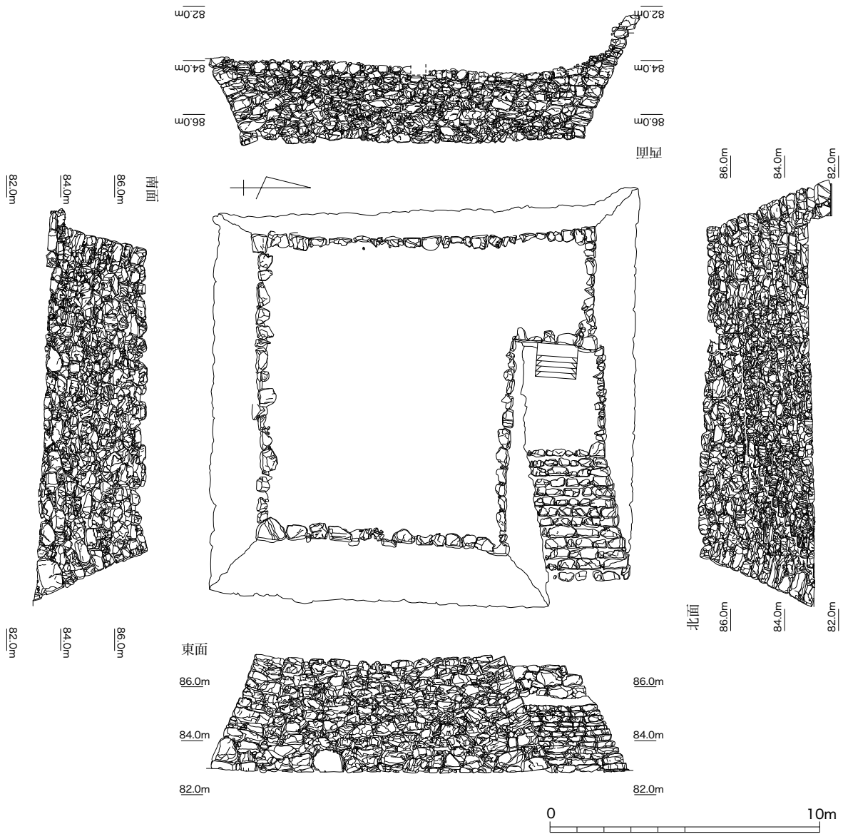
Fig.47 天守台の構造
