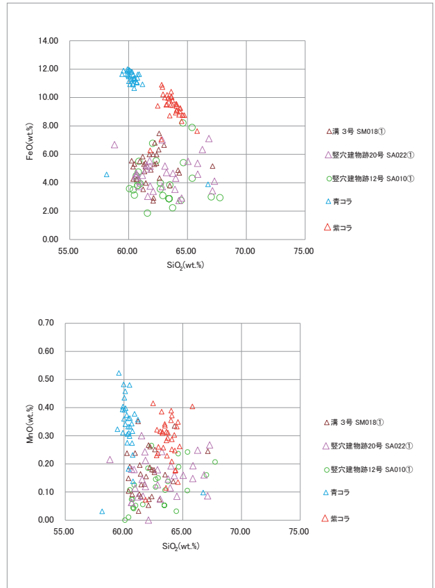
図6 スコリアの科学組成散布図(1)
