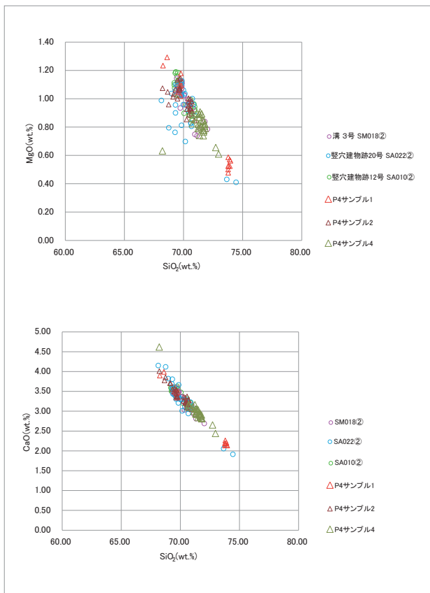
図11 軽石の科学組成散布図(3)
