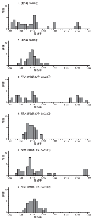
図3 斜方輝石の屈折率測定結果(1)
