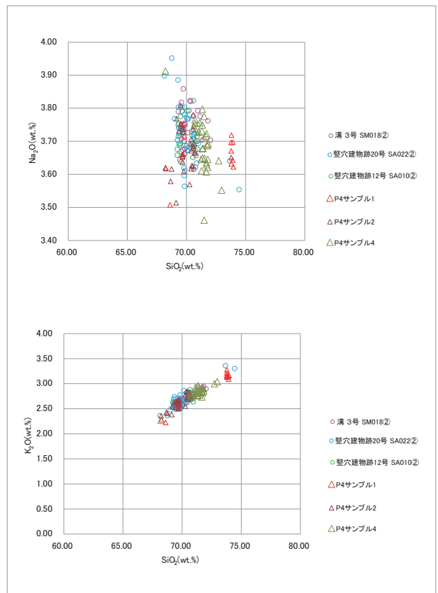
図12 軽石の科学組成散布図(4)
