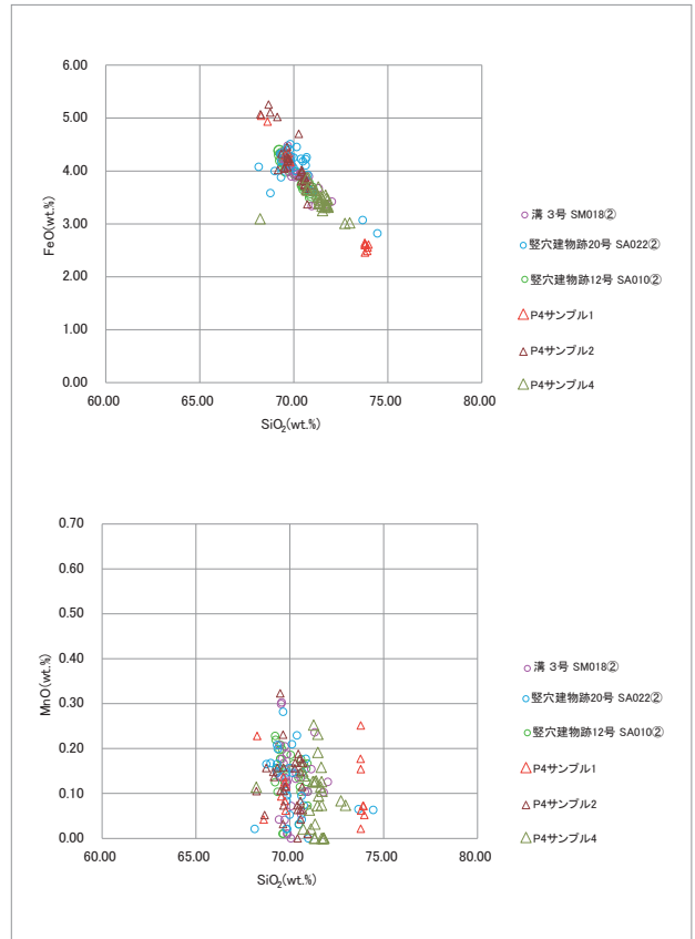
図10 軽石の科学組成散布図(2)
