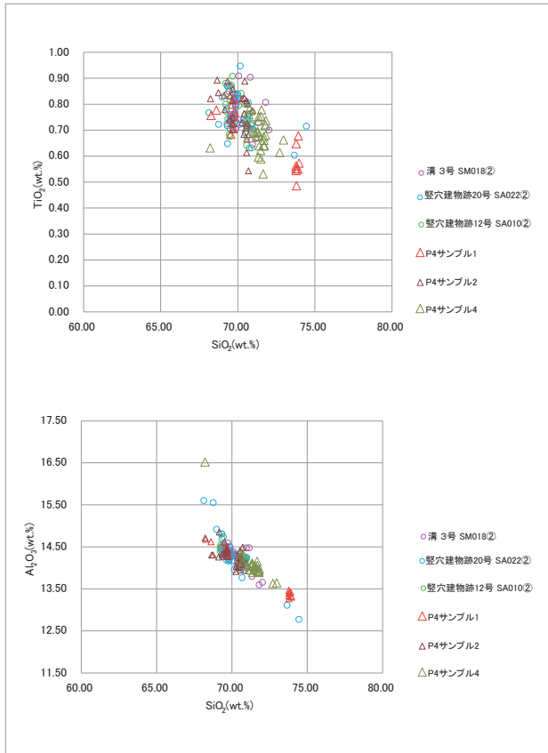
図9 軽石の科学組成散布図(1)
