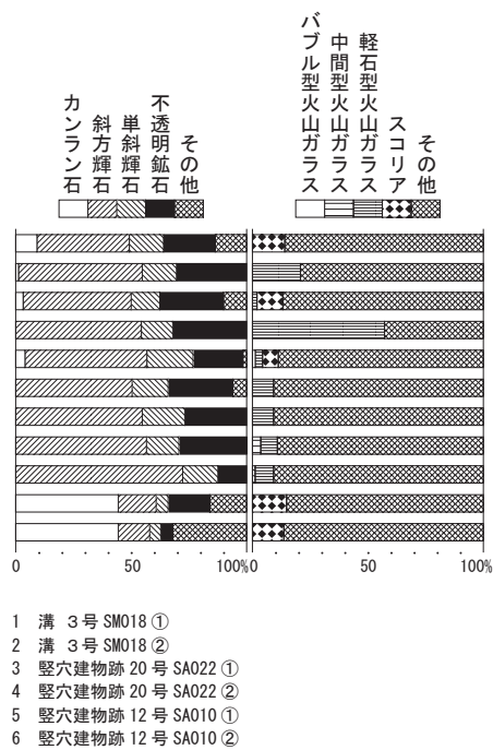
図1 重鉱物組成および火山ガラス比
