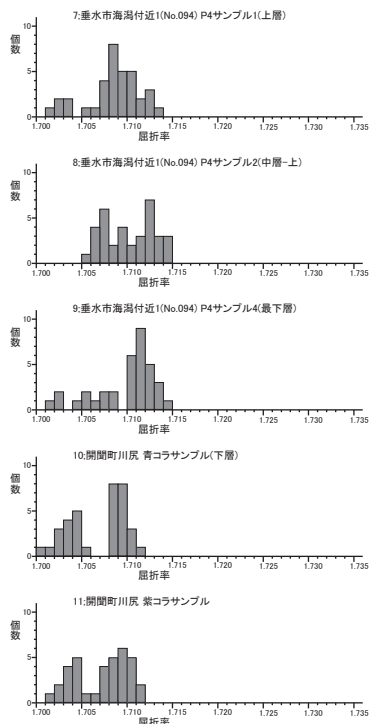
図4 斜方輝石の屈折率測定結果(2)
