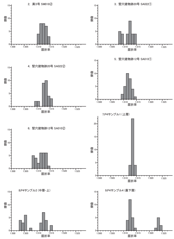
図2 火山ガラスの屈折率測定結果
