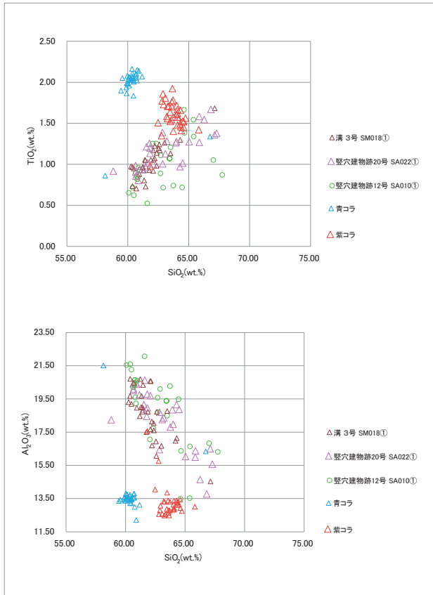
図5 スコリアの科学組成散布図(1)
