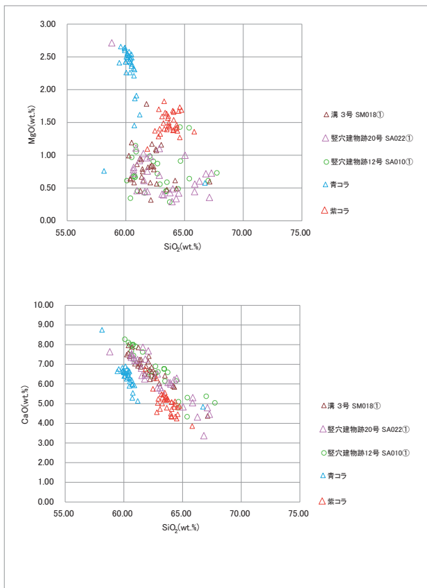
図7 スコリアの科学組成散布図(3)
