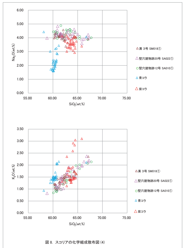
図8 スコリアの科学組成散布図(4)
