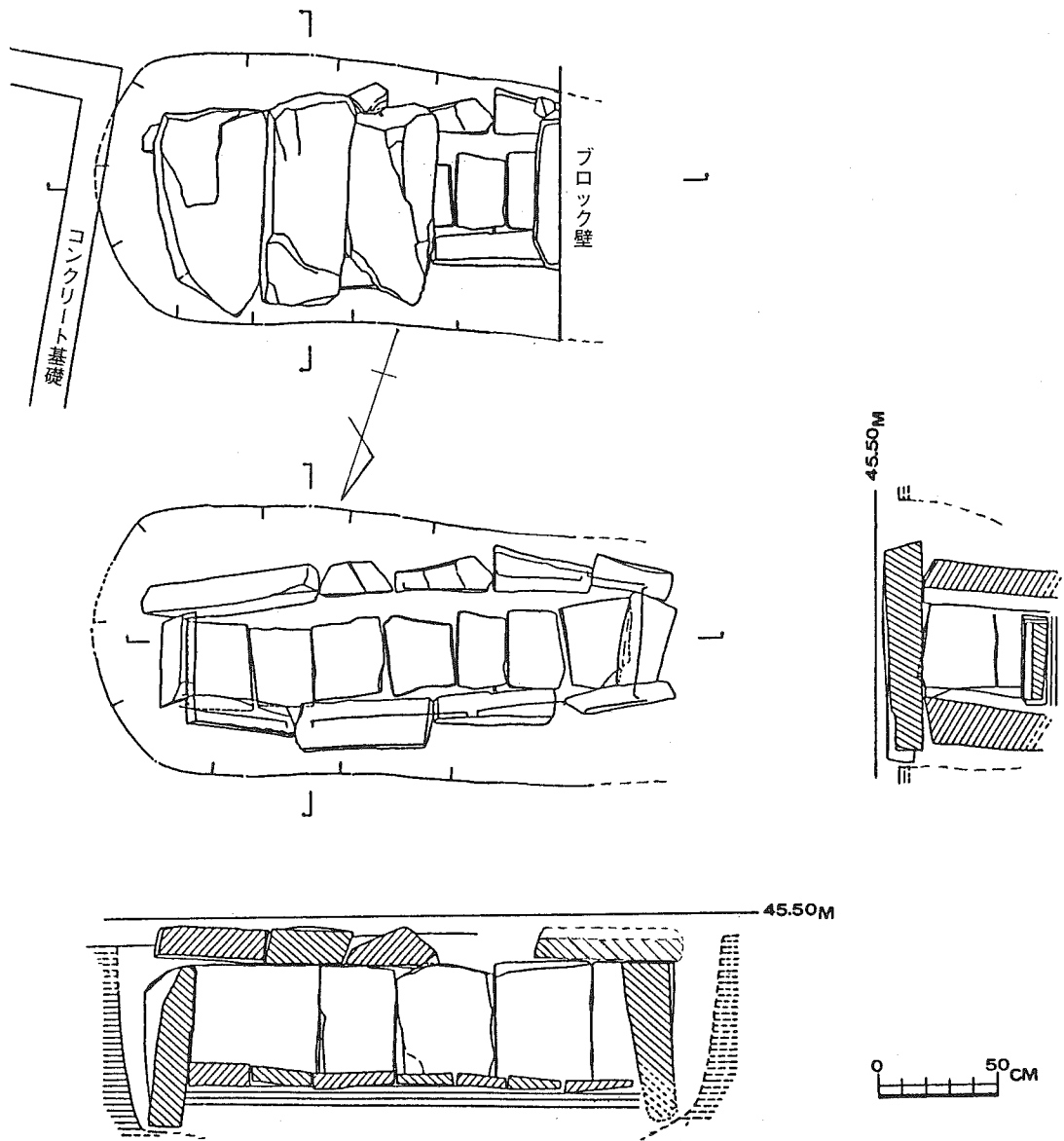
第(3)図 箱式石棺実測図 (1/30)
