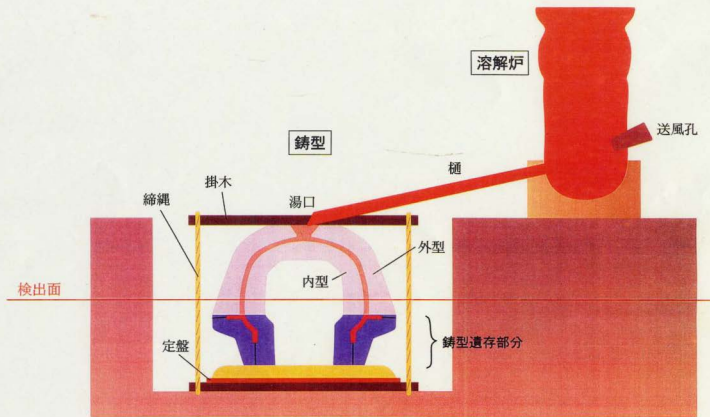
鑄造方法復原図
