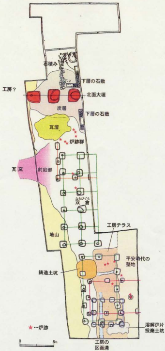
遺構配置図 S=1:200
