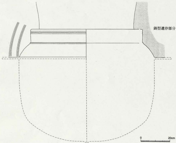
鑄造製品復原図 S=1:6
