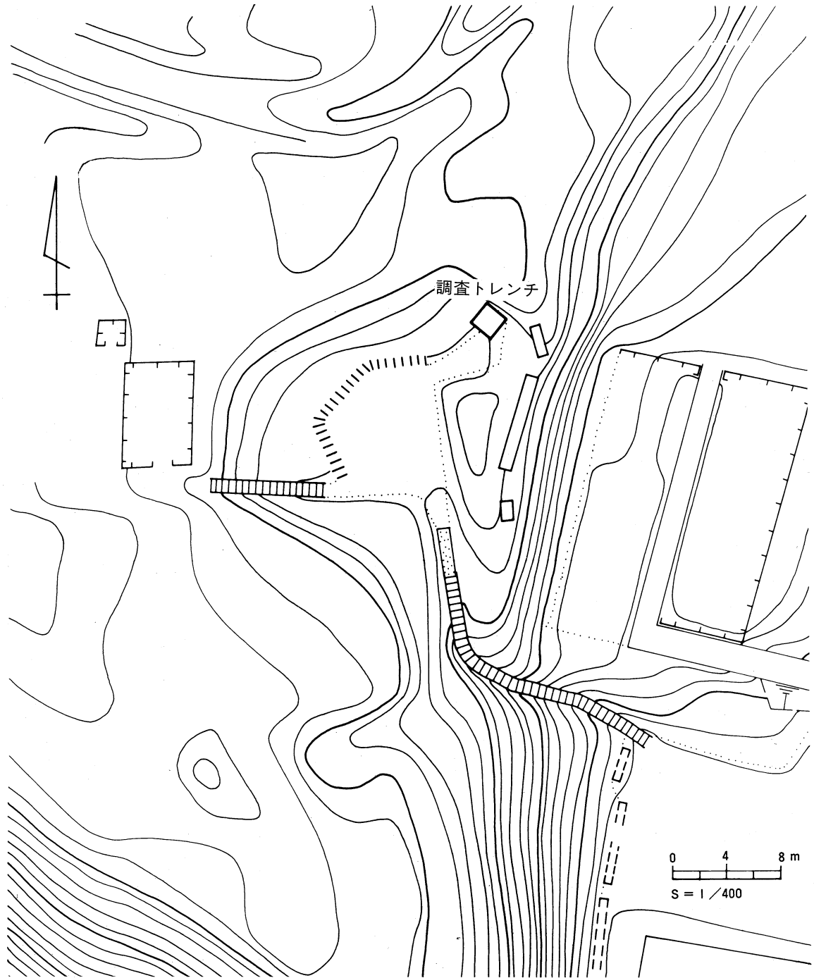
第5図 正覚院館跡 トレンチ配置図
