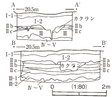
第33図 道地遺跡f地点土層断面図
