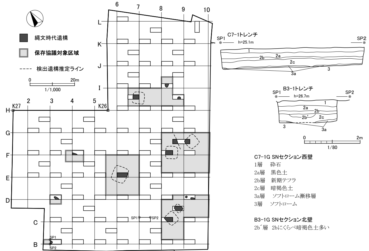
第27図 i 地点トレンチ配置図・土層断面図
