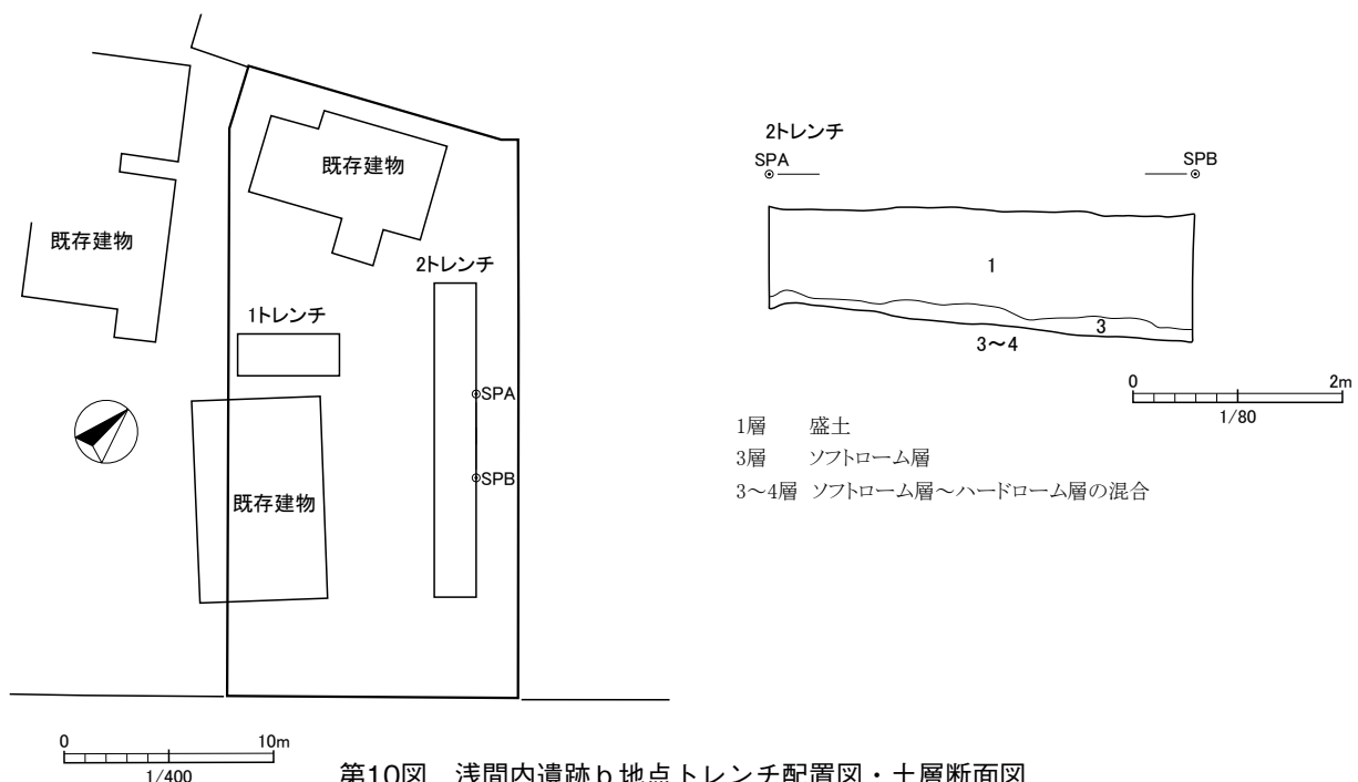
第10図 浅間内遺跡b地点トレンチ配置図・土層断面図
