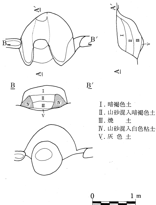
第12図 第2号住居址カマド実測図
