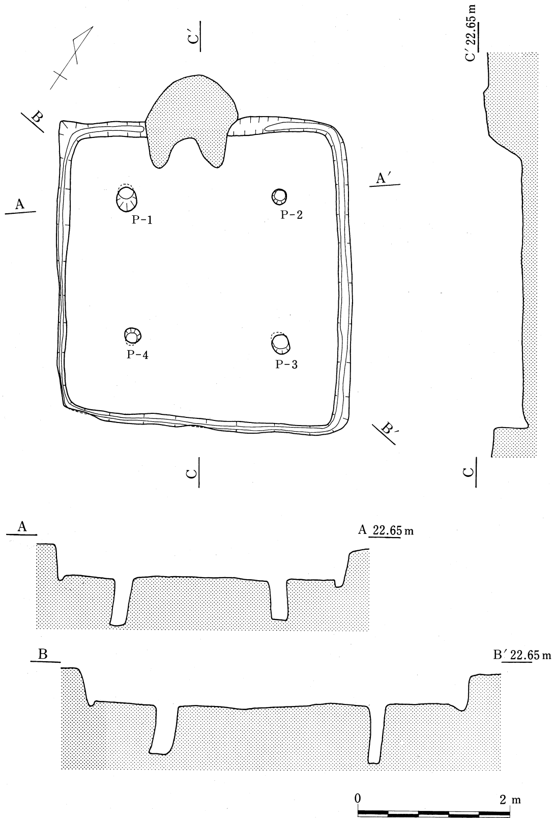
第10图 第2号住居址実測図
