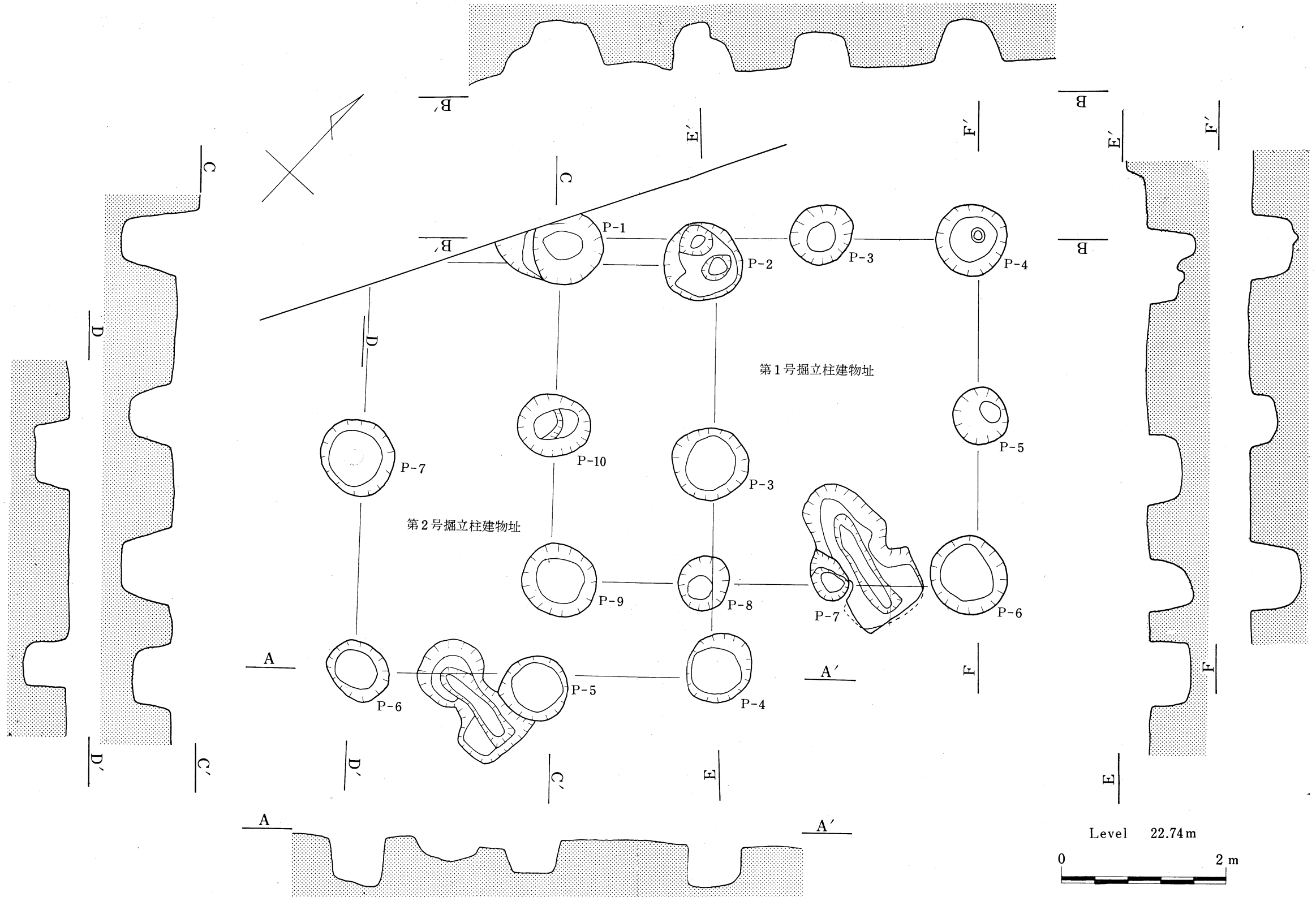
第15图 掘立柱建物址实测图
