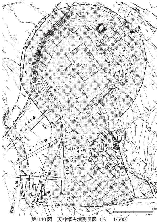
第140図 天神塚古墳測量図 (S = 1/500)
