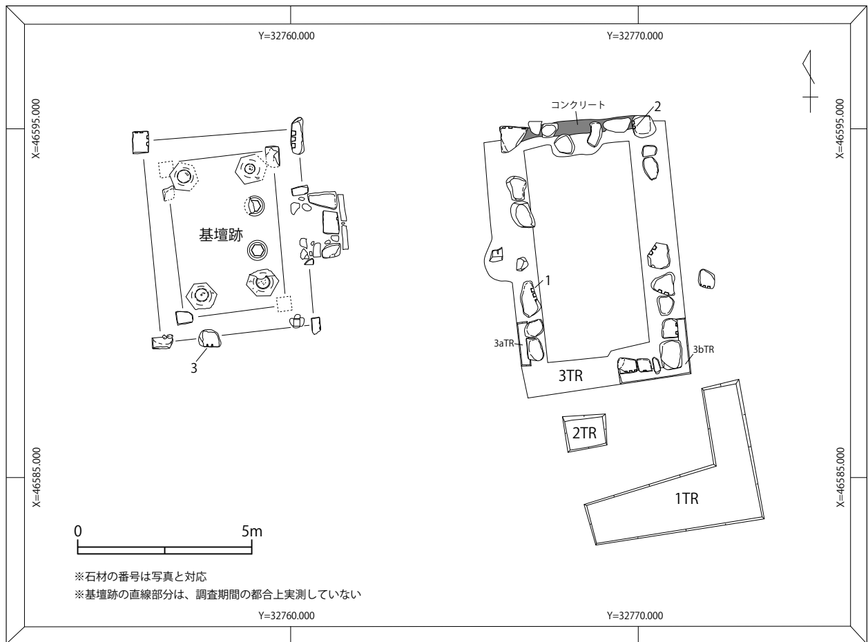
第7図 竜王城跡遺構配置図 (S=1/150)
