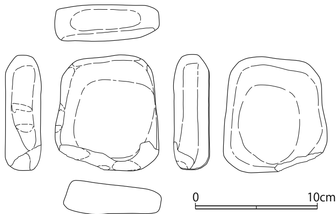
第8図 SI-01出土砥石実測図(S=1/3)
