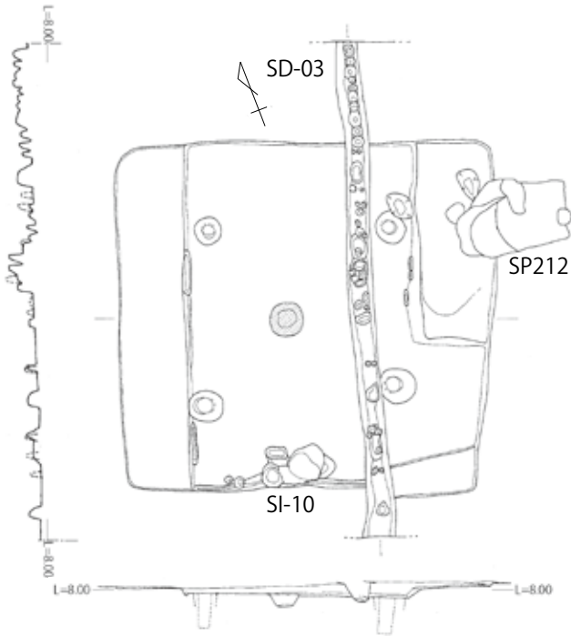
第9図 SI-10 実測図(S=1/80、第7次調査時の平面図と合成)
