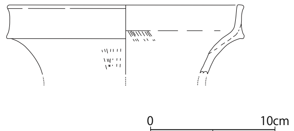
第15図 表面採集遺物実測図(S=1/3)
