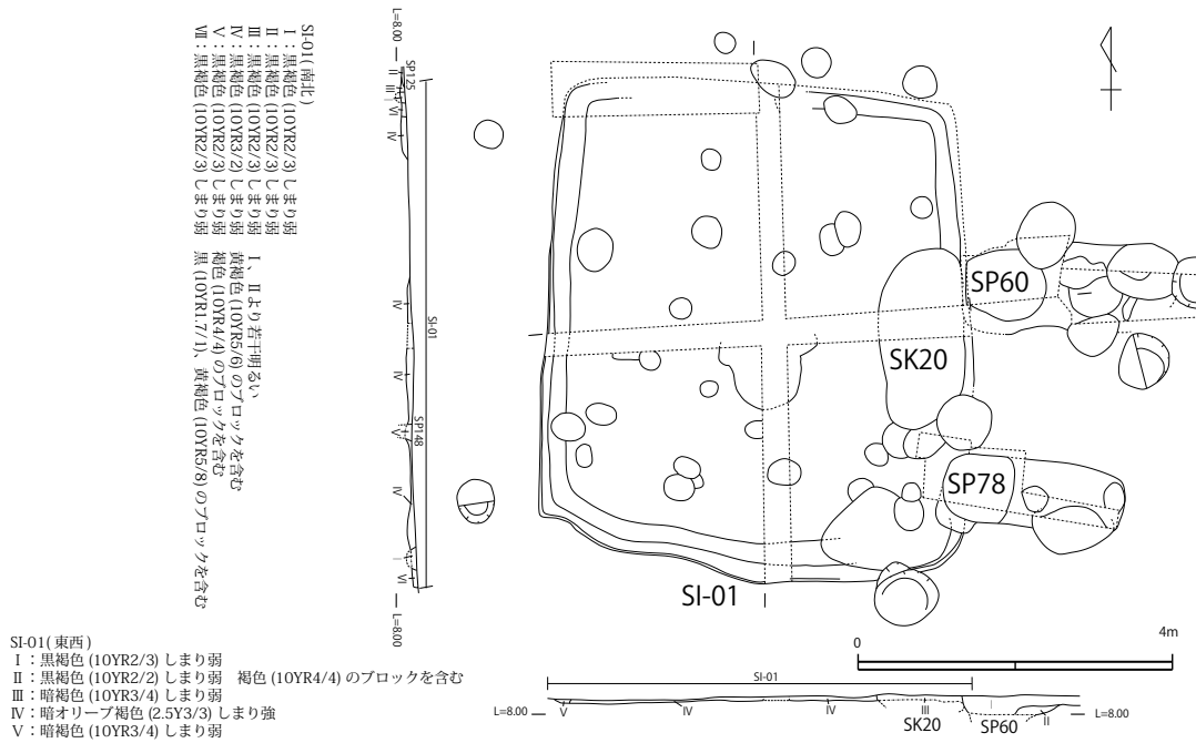
第10図 SI-01 実測図(S=1/80)
