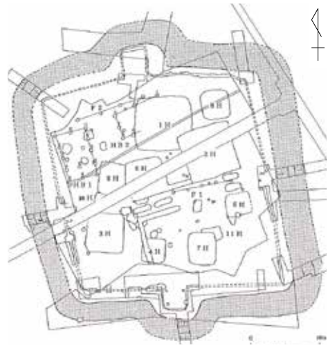
第 24 図 四斗蒔遺跡 1 号遺構平面図 (橋本編 2000 より、S=1/750)
