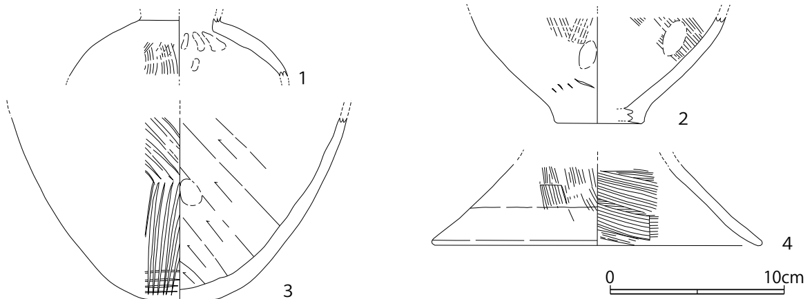
第11図 SI-01 出土遺物実測図(S=1/3)
