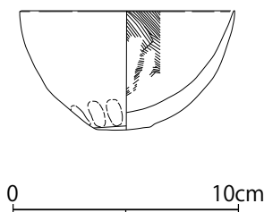
第14図 SK-16出土遺物実測図(S=1/3)
