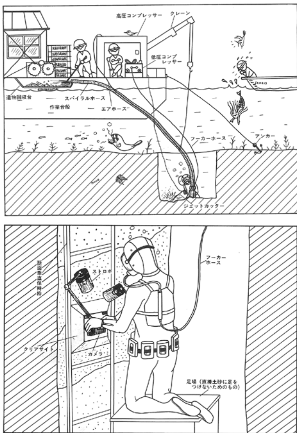
図3 潜水調査の概要図（大沼ほか 1987 より転載）
