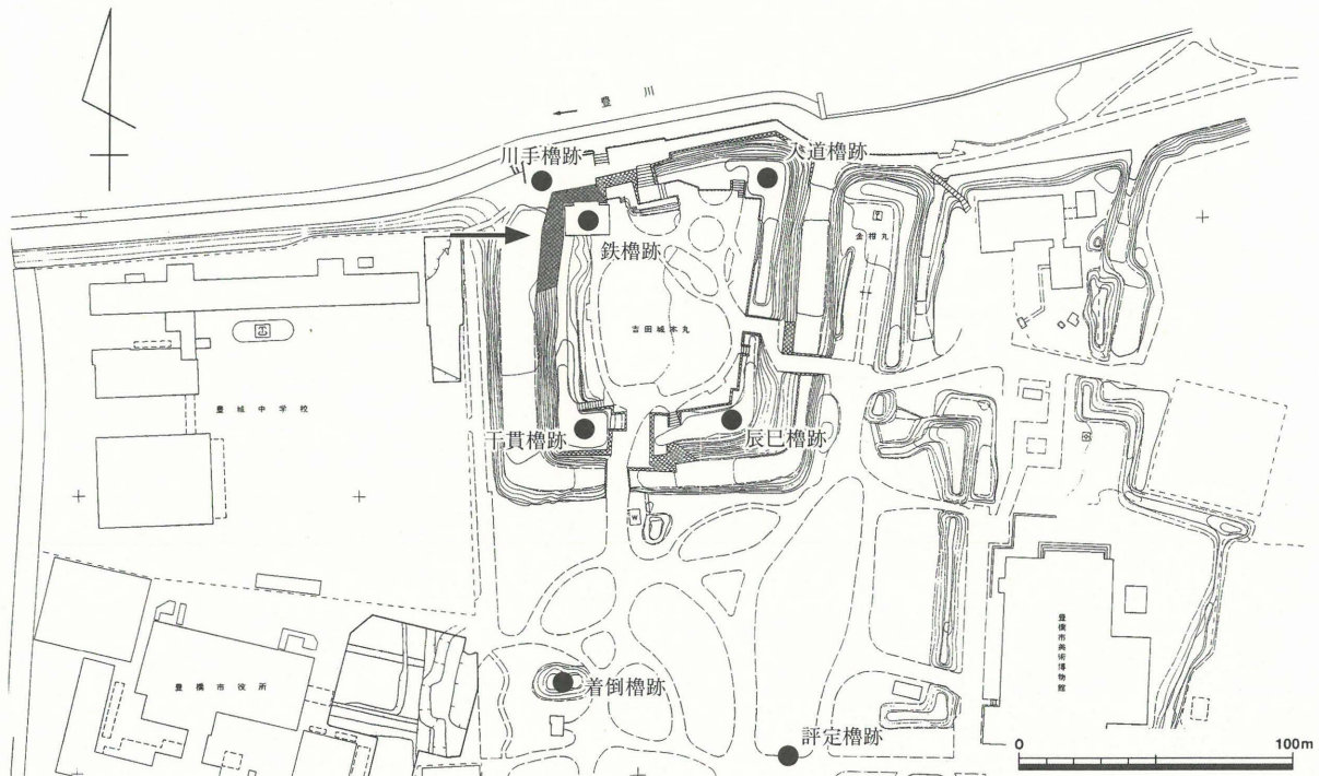
第28図 鉄櫓下石垣の位置（1 / 3,000）
