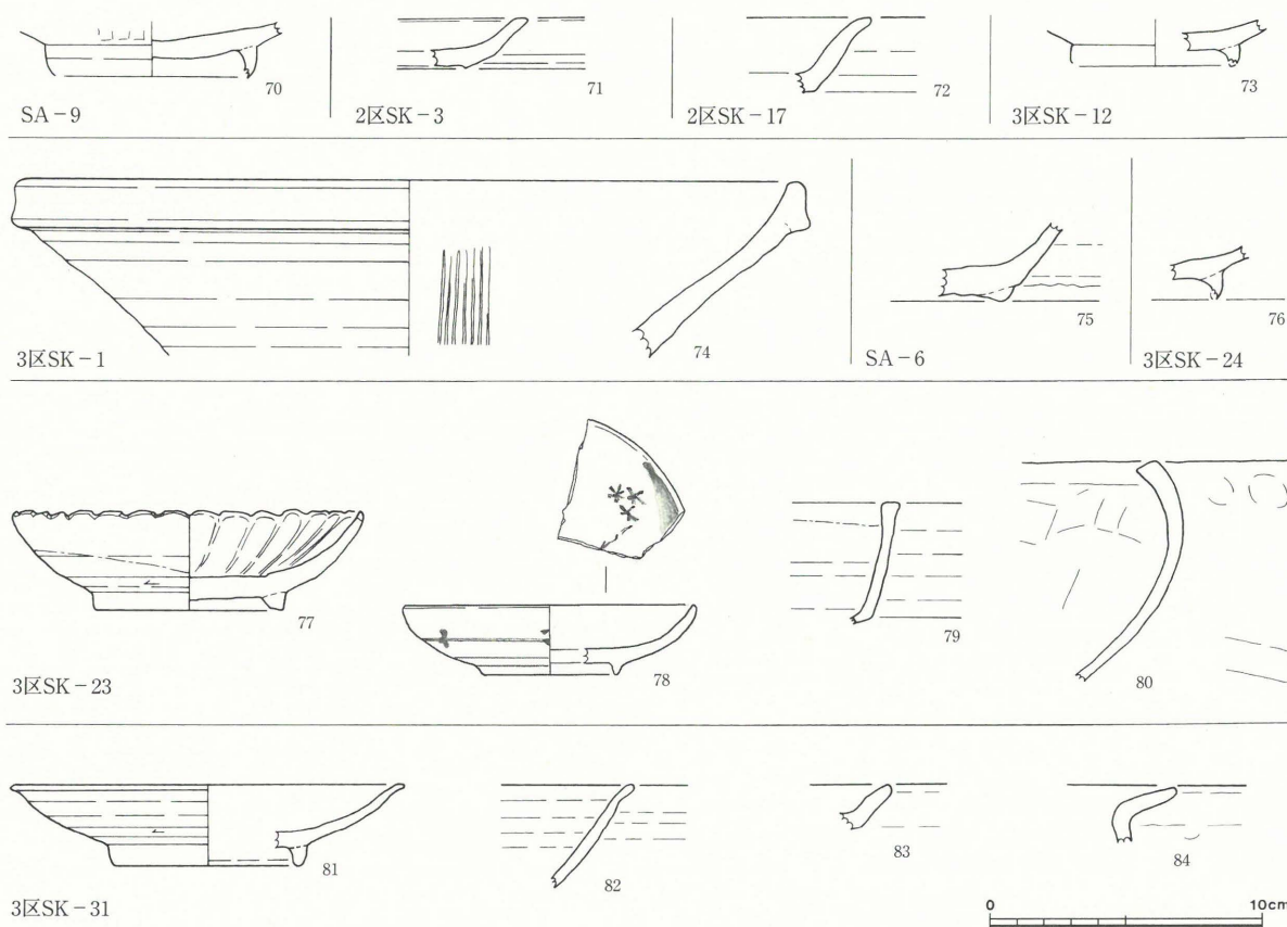
第19図 出土遺物-6 (1/3)
