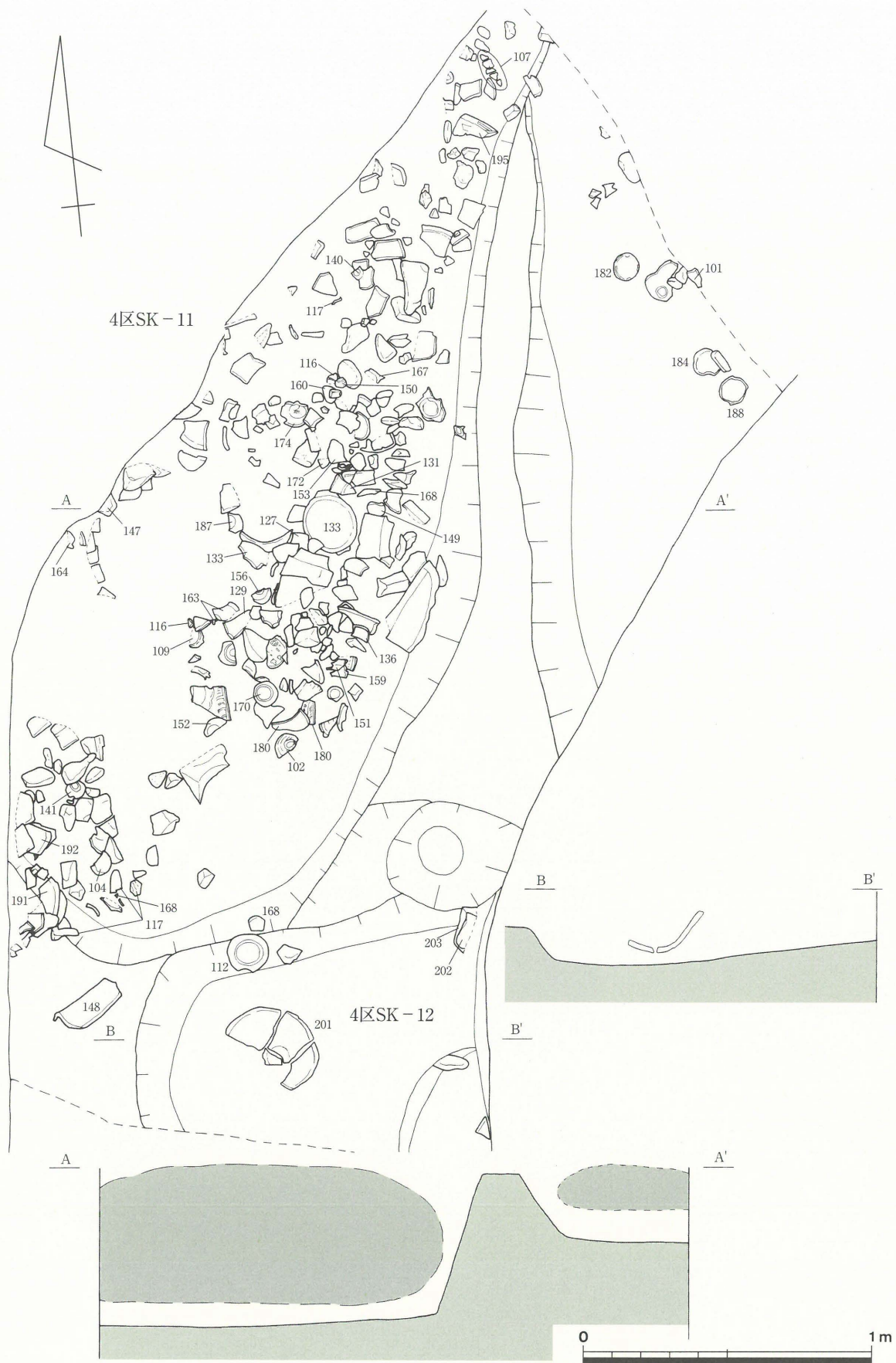
第13図 4区SK-11・12出土状況 (1/20)
