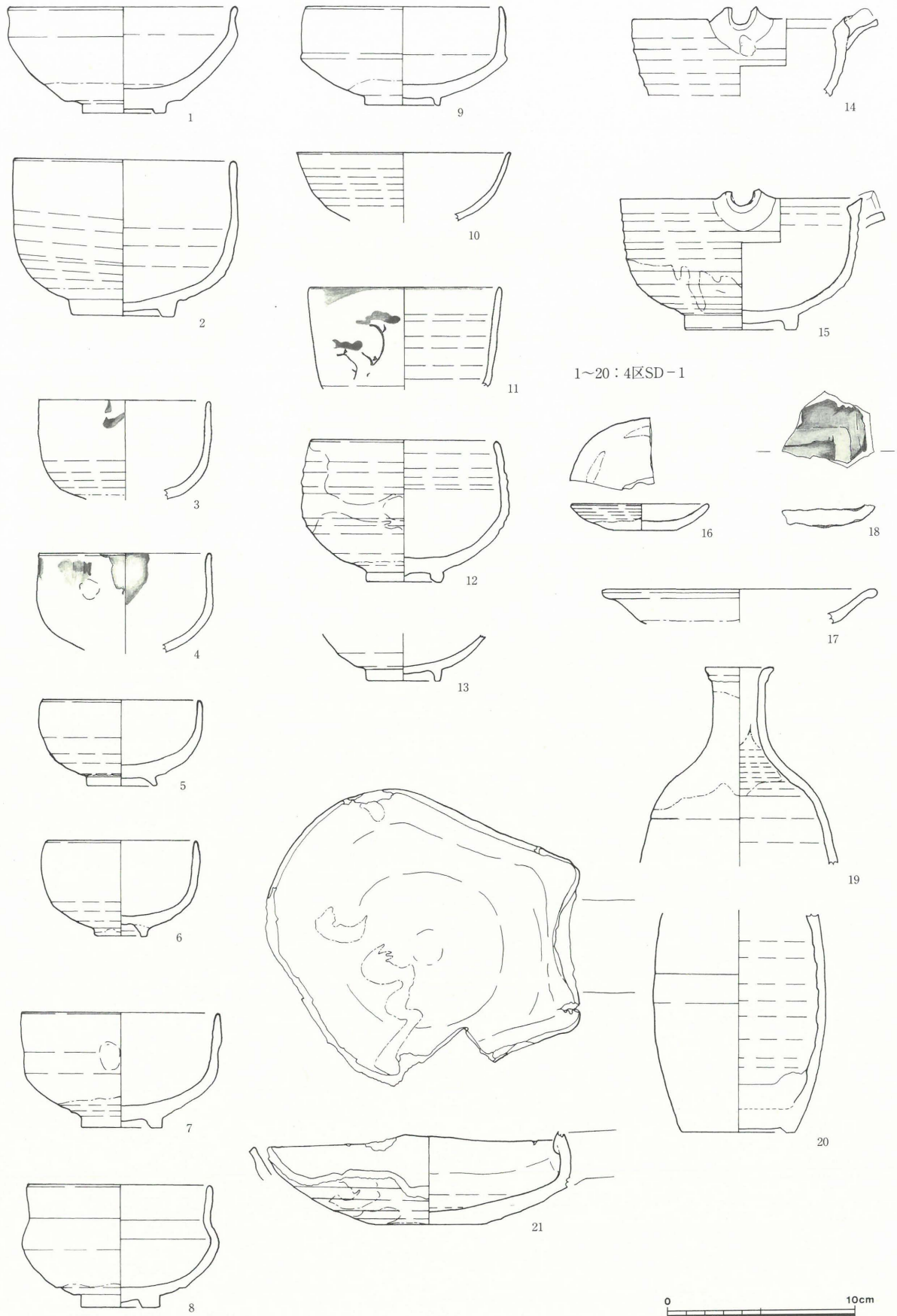
第14図 出土遺物-1 (1/3)
