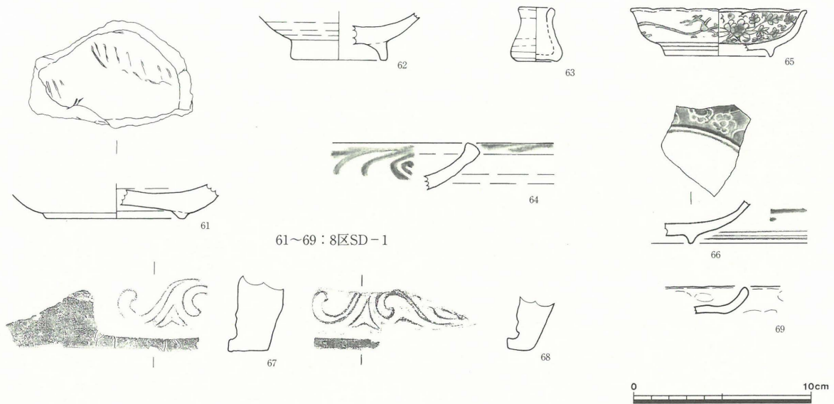
第18図 出土遺物-5 (1/3)
