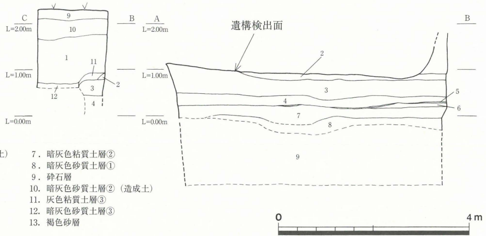
第34図 調査区平面図・土層図 (1/80)
