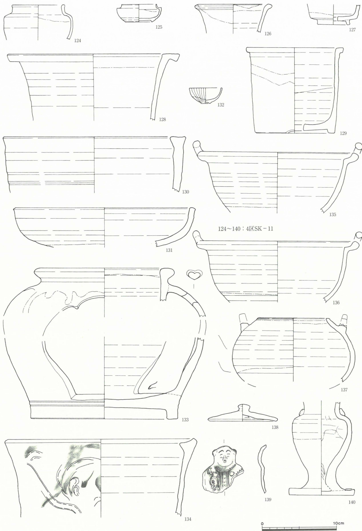
第22図 出土遺物一9 (1/3)
