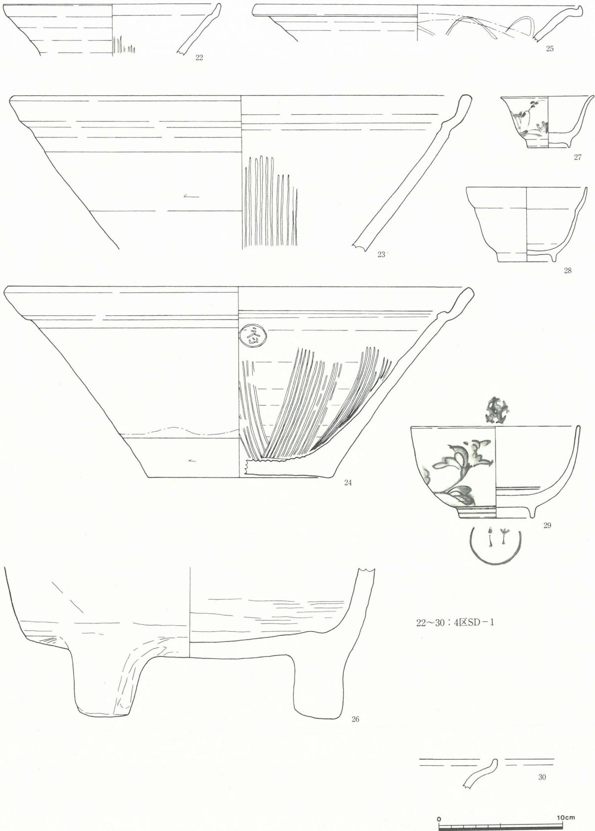
第15図 出土遺物-2 (1/3)
