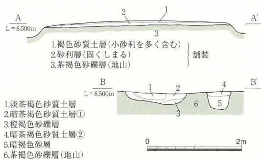
第6図 八幡小路・8区SD-1・2土層図(1/80)
