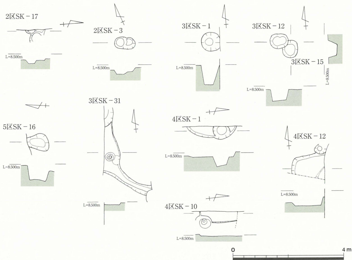
第11図 土壙-1 (1 / 80)
