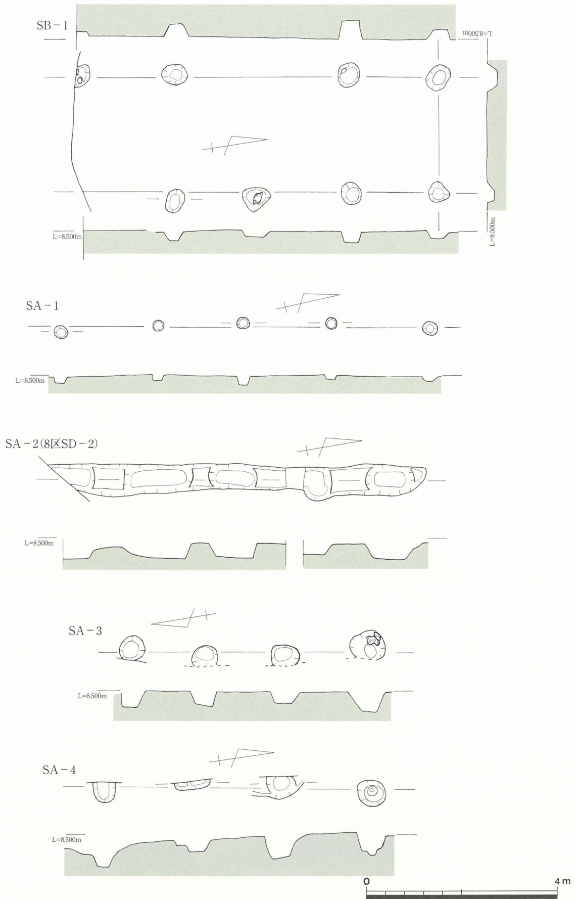
第8図 掘立柱建物・柵-1 (1/80)
