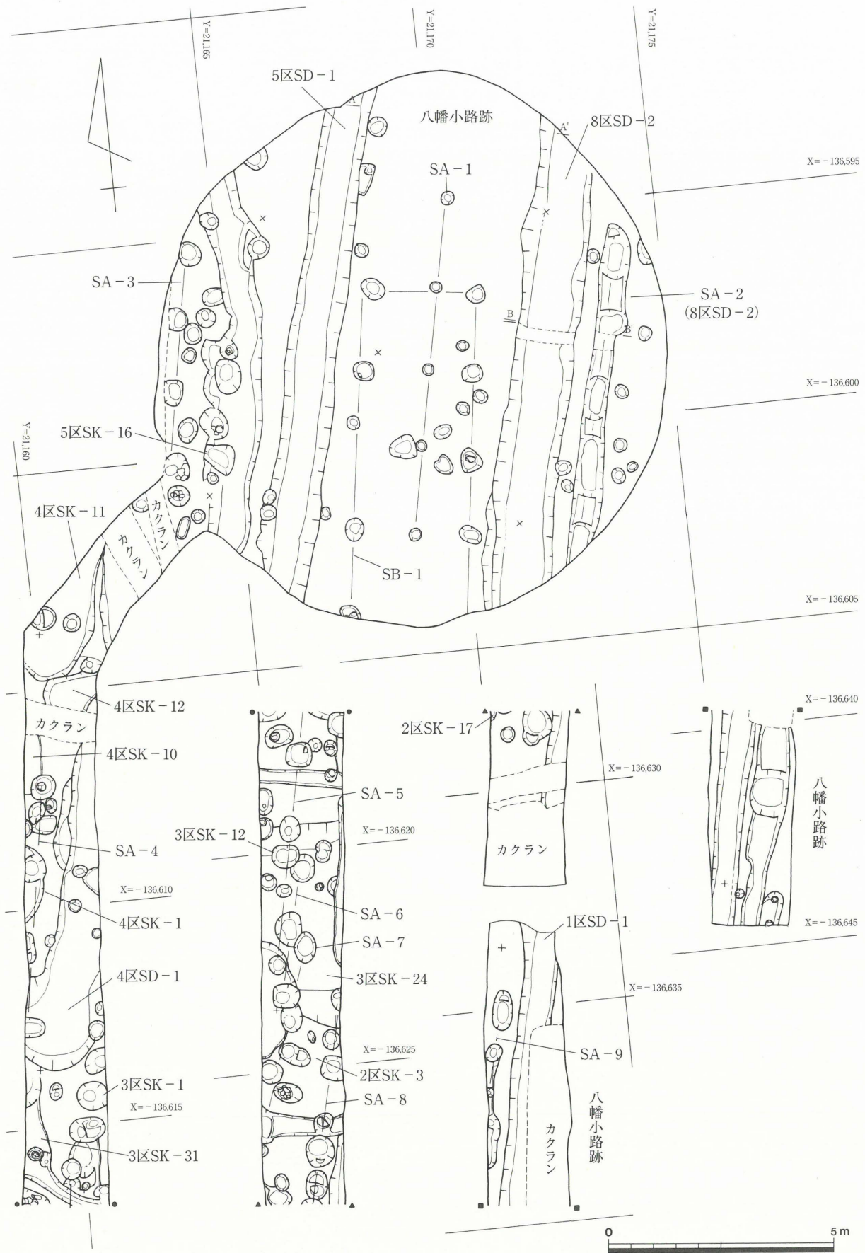
第7図 調査区平面図 (1 / 120)
