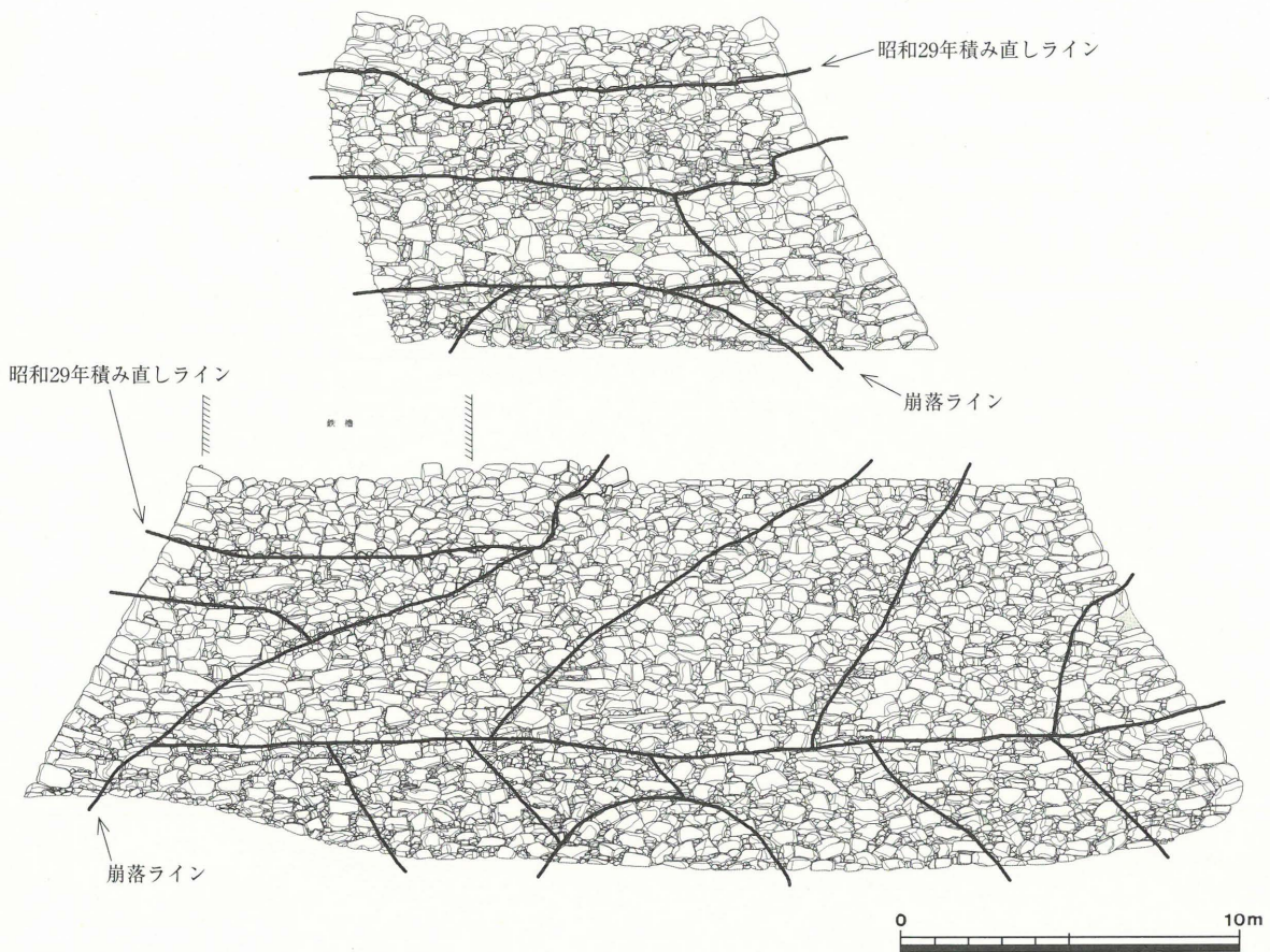
第31図 石垣の目地 (1 / 240)
