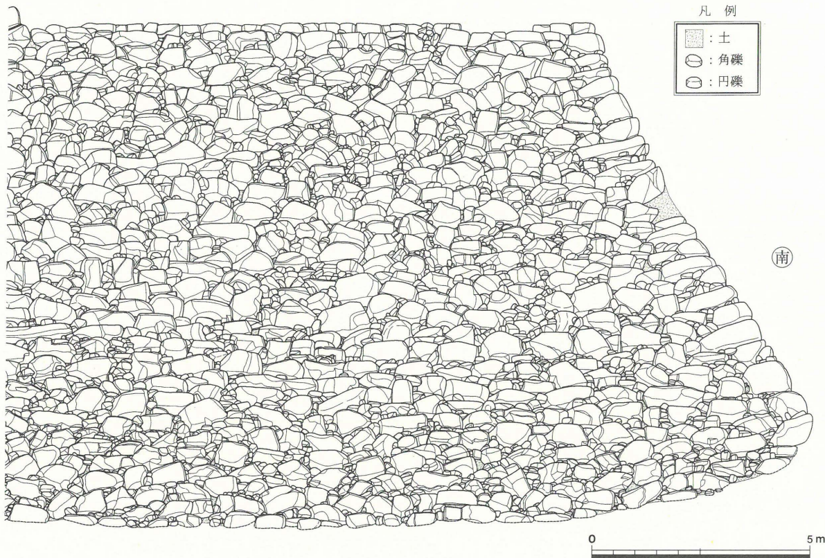
第29図 鉄櫓下石垣実測図 (1 / 120)
