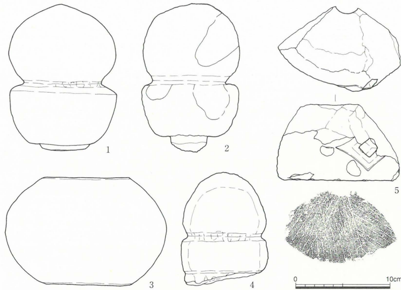
第30図 櫓台の裏込めに使われた石塔等（1／4）
