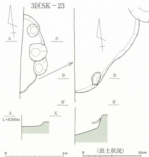
第12図 土壌-2 (1/20・1/80)
