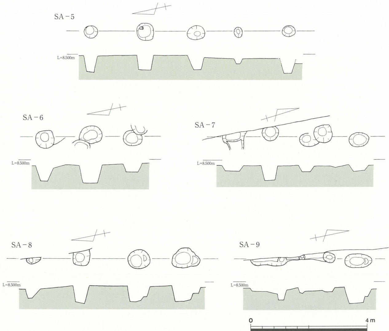
第9図 柵-2 (1/80)
