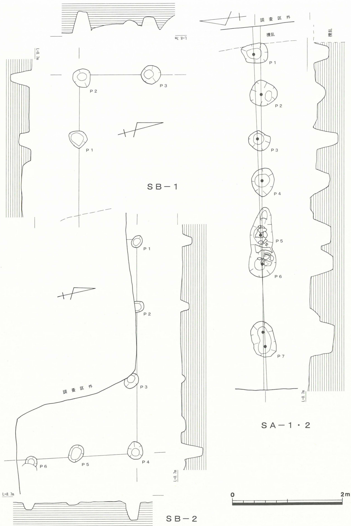
第3図 第19次遺構実測図-1 (1/40)
