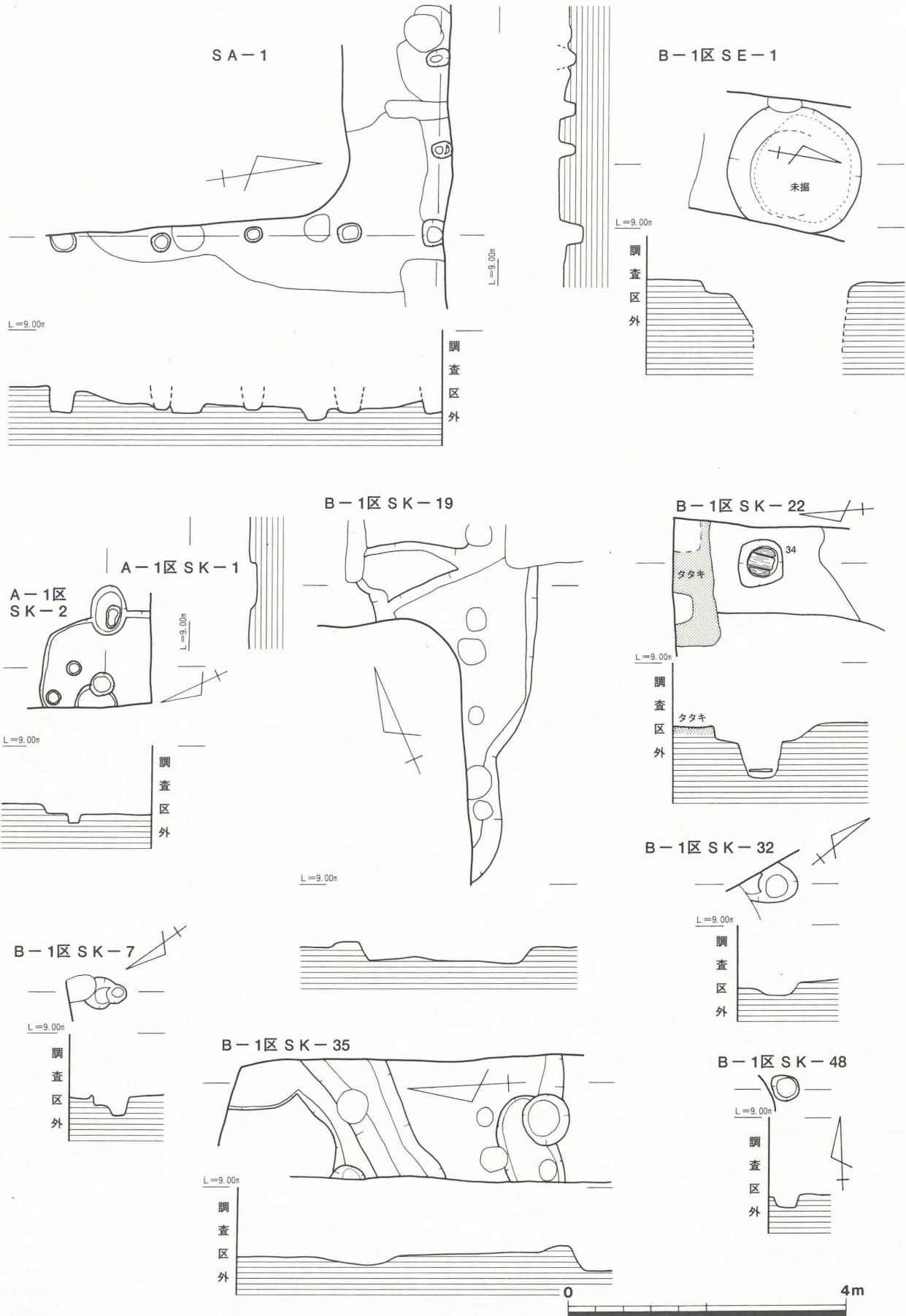
第6図 第15次調査遺構実測図 (1/80)
