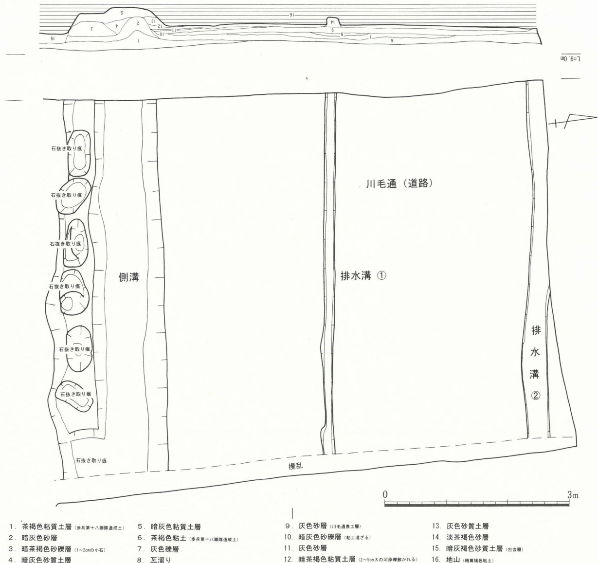
第4図 第19次調査遺構実測図-2 (1/60)
