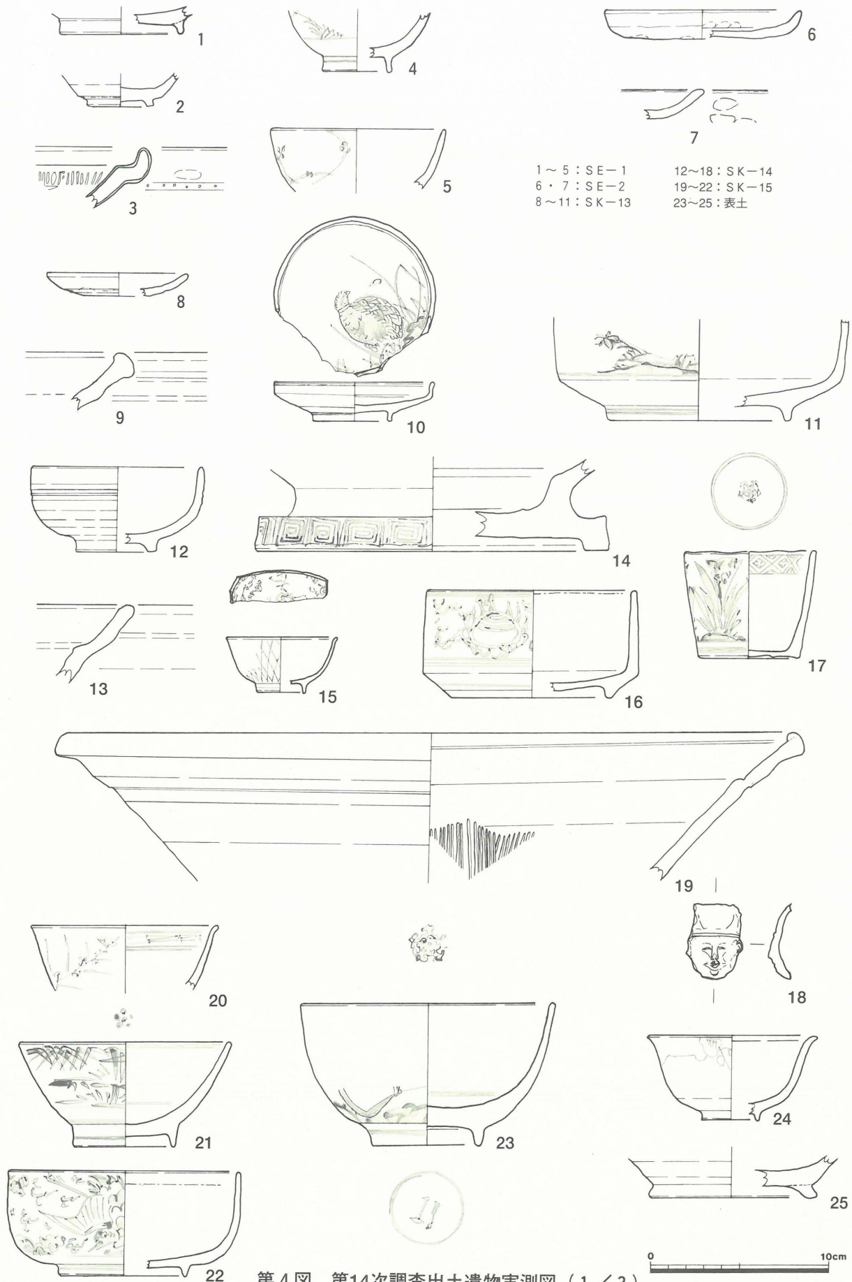
第4図 第14次調査出土遺物実測図 (1 / 3)
