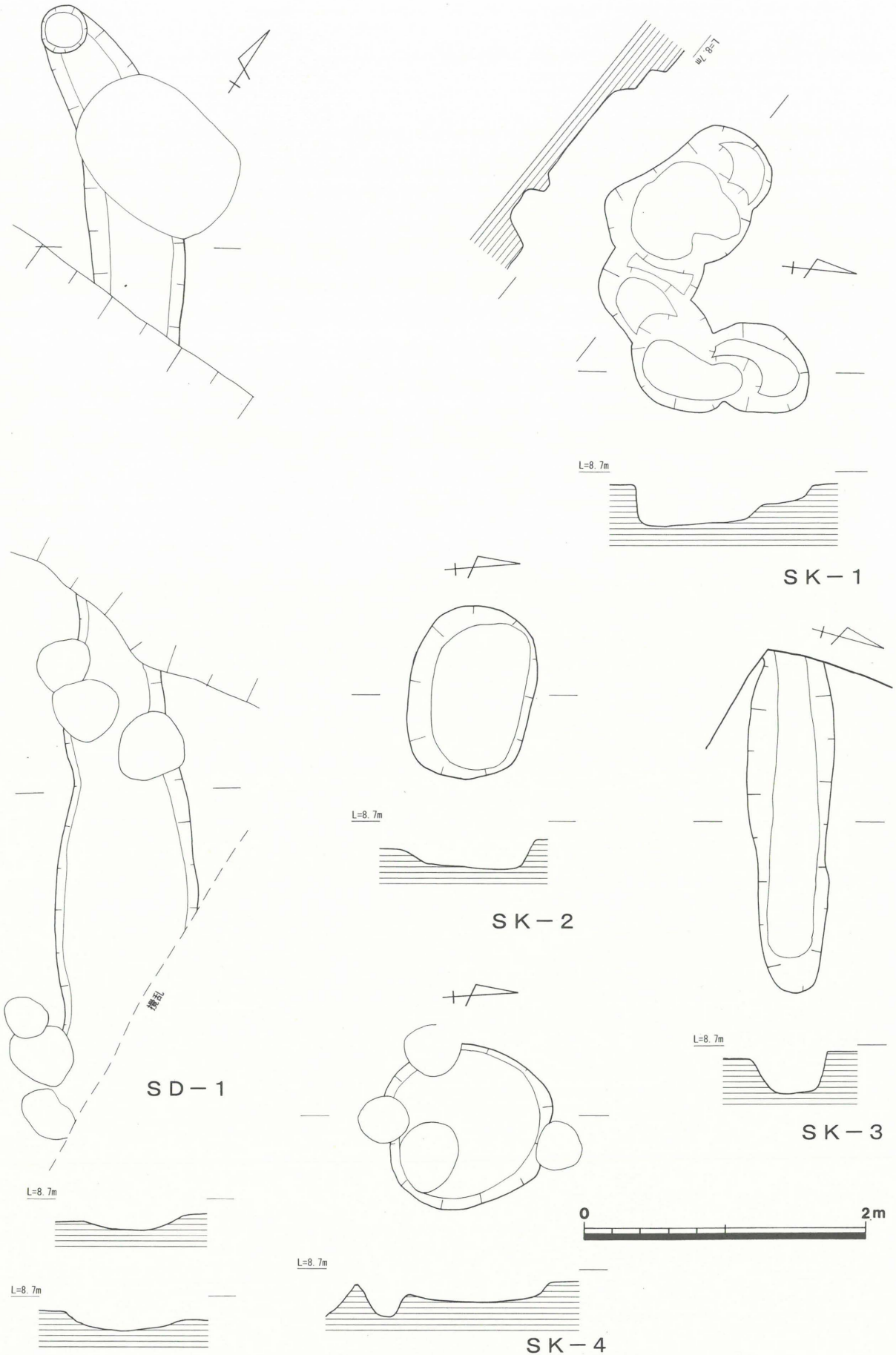
第5図 第19次調査遺構実測図-3 (1/40)
