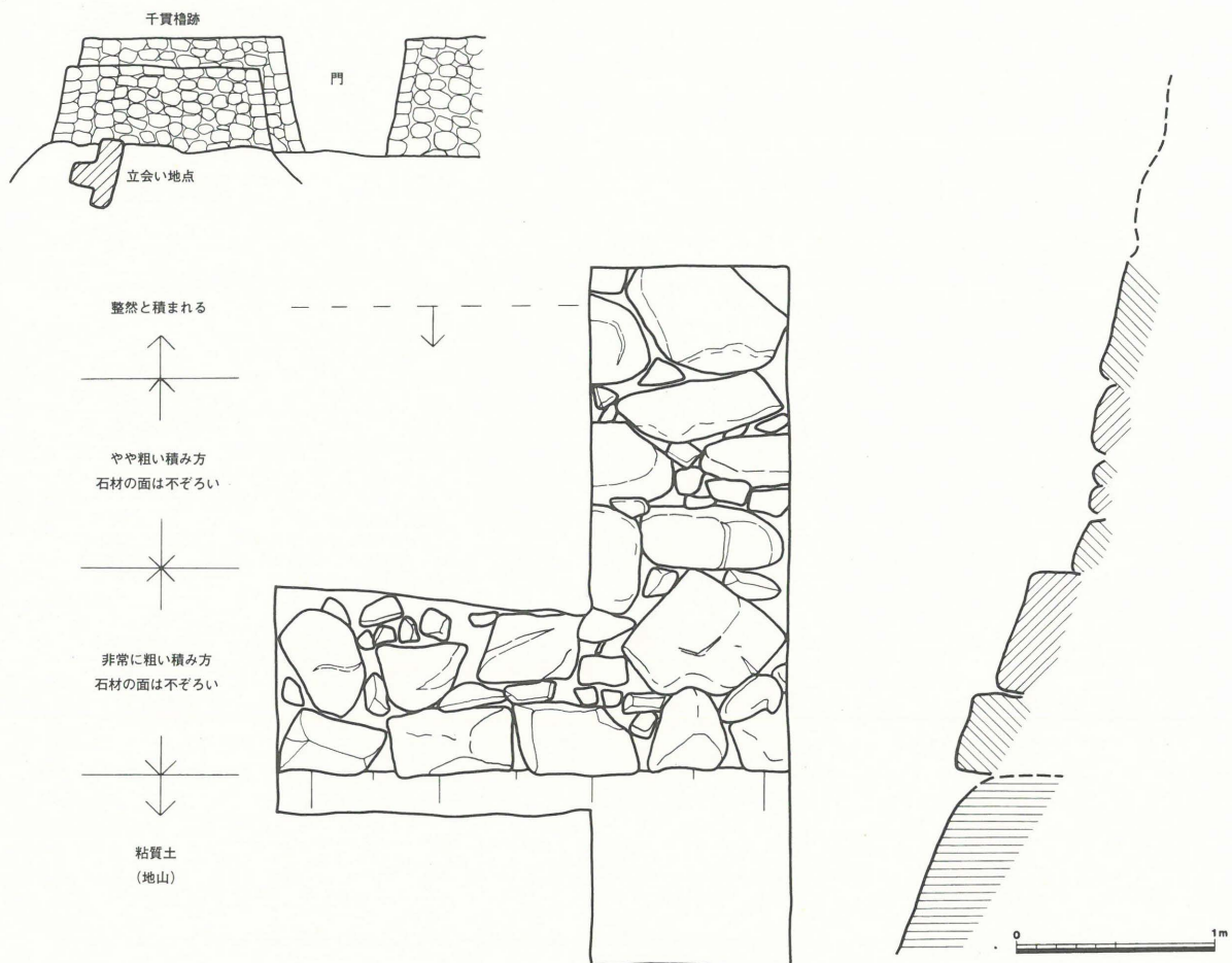
第5図 本丸南側石垣地点略測図 (1/40)
