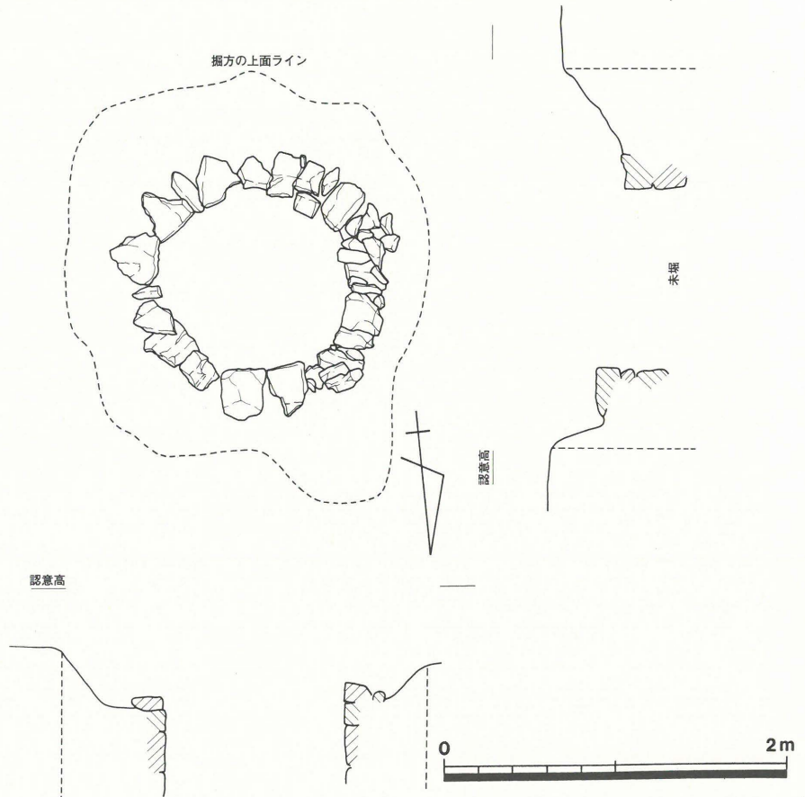
第3図 石組み井戸実測図 (1/40)
