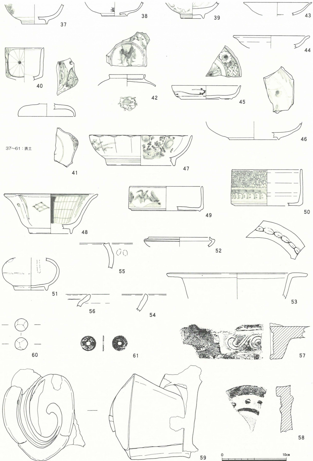
第7図 第19次調査出土遺物実測図-2 (1/3)
