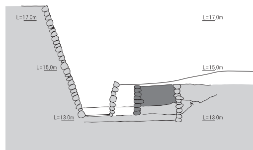
第16図 東内惣構跡(枯木橋南地点)における惣構変遷図(S=1/150)
