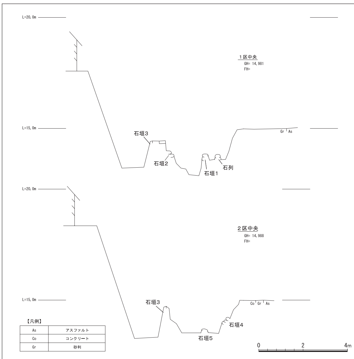
第10図 石垣エレベーション図(S=1/100)
