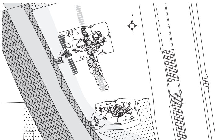
第16図 東内惣構跡(枯木橋南地点)における惣構変遷図(S=1/150)
